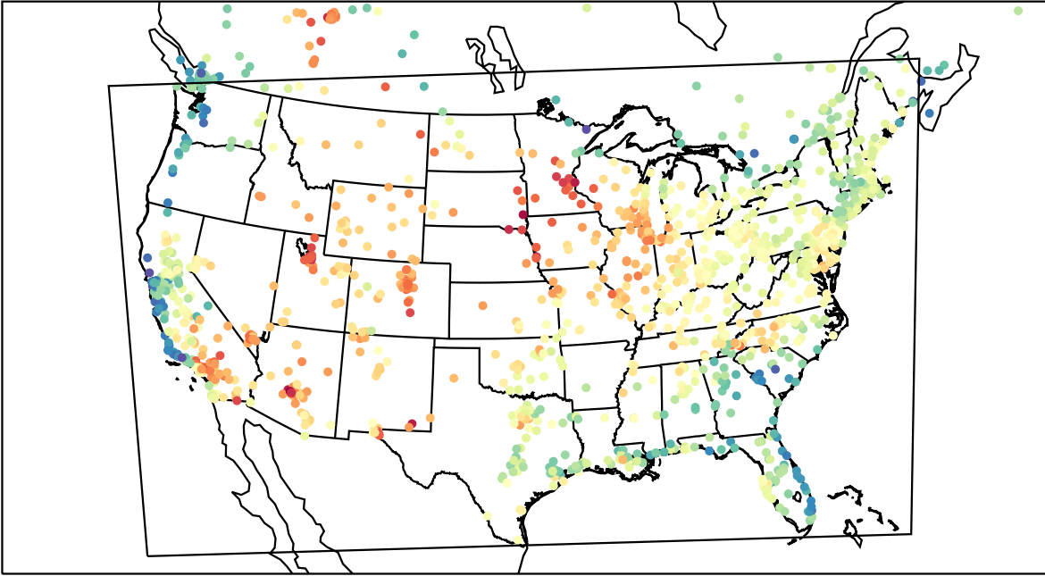
AirNOW (2023-05-21_20:00:00)
