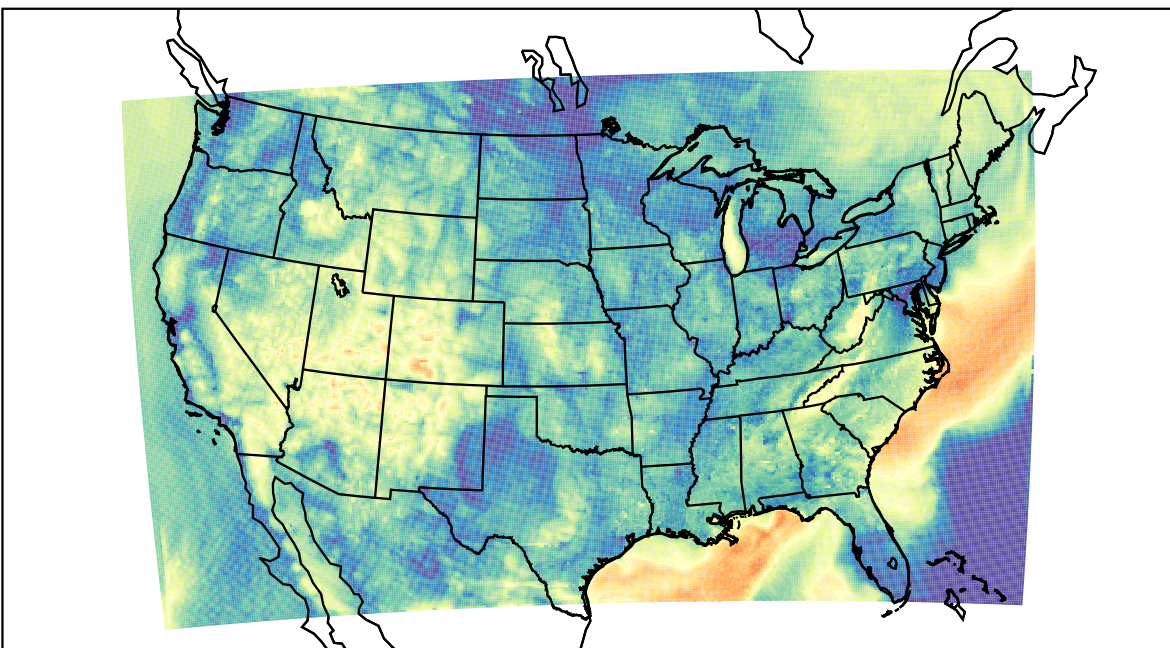
WRF (2023-05-22_13:00:00)
