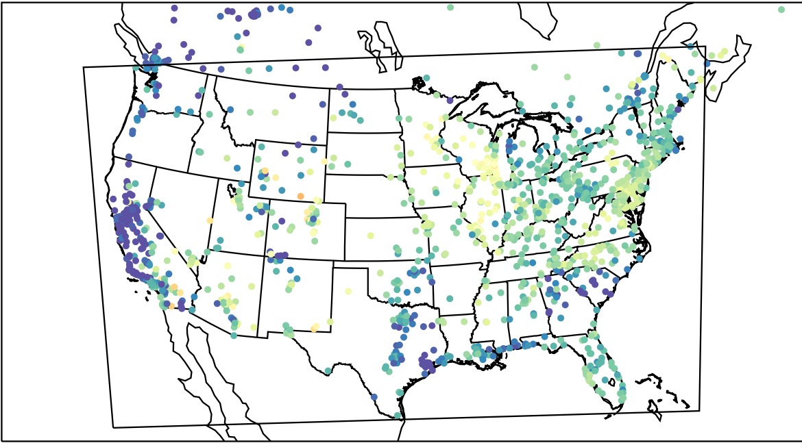
AirNOW (2023-05-21_14:00:00)
