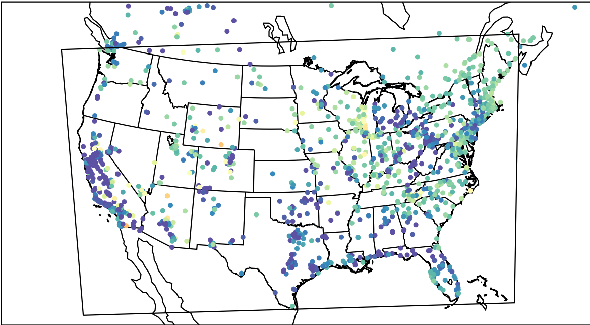
AirNOW (2023-05-22_13:00:00)
