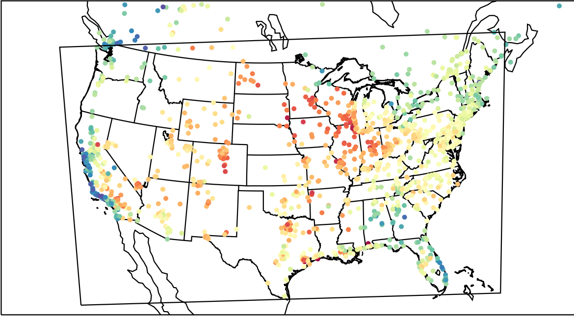
AirNOW (2023-05-22_18:00:00)
