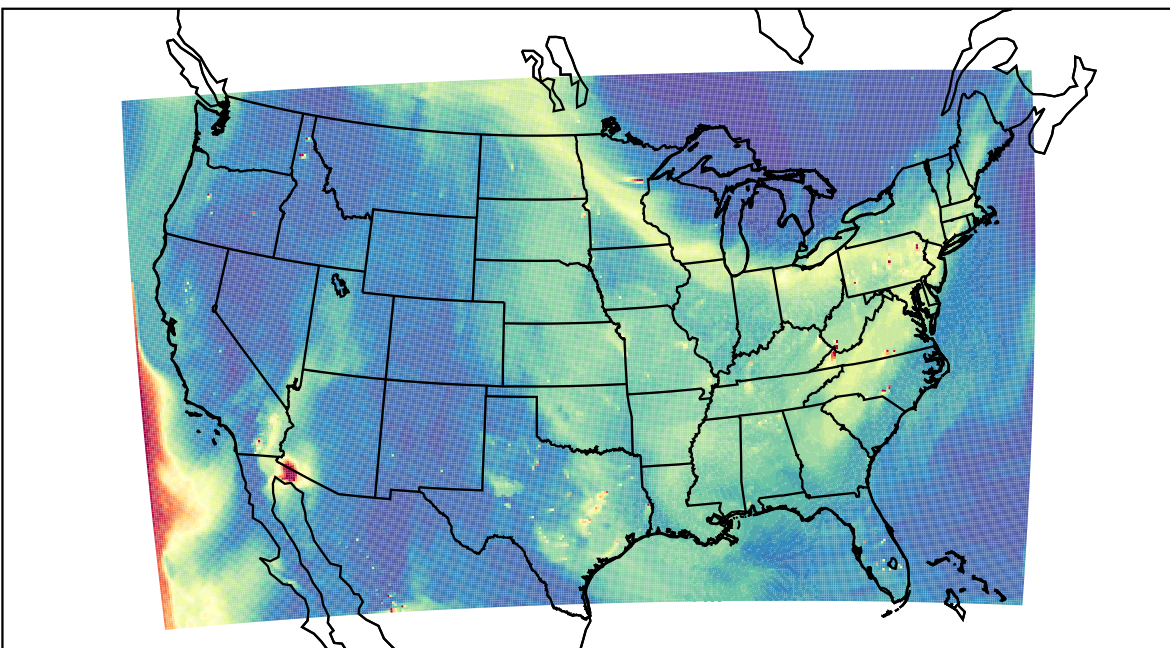
WRF 2023-05-24_22:00:00
