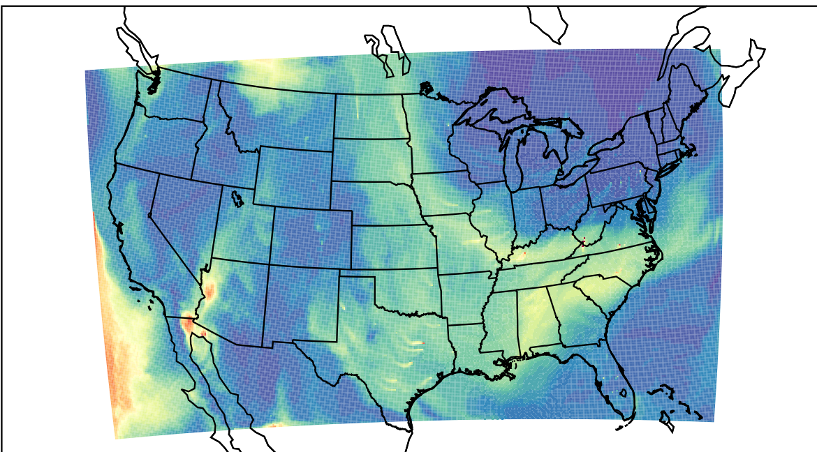
WRF 2023-05-25_18:00:00
