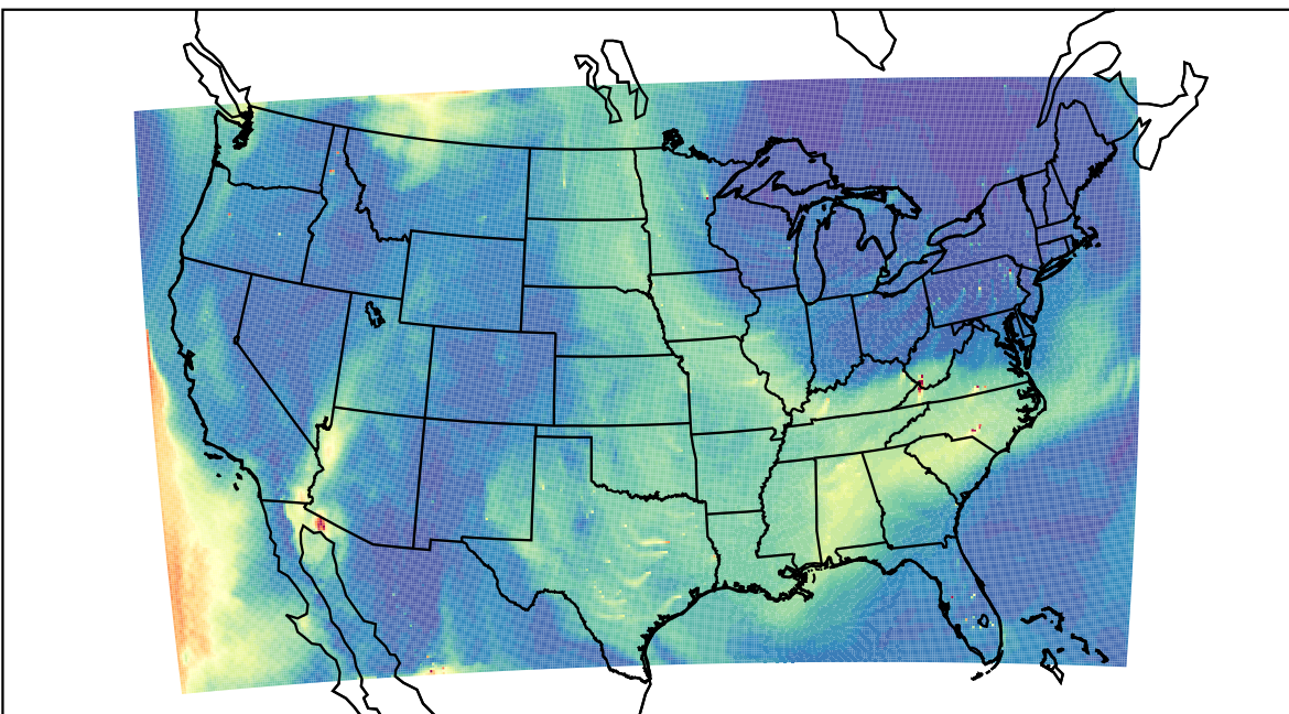
WRF 2023-05-25_20:00:00
