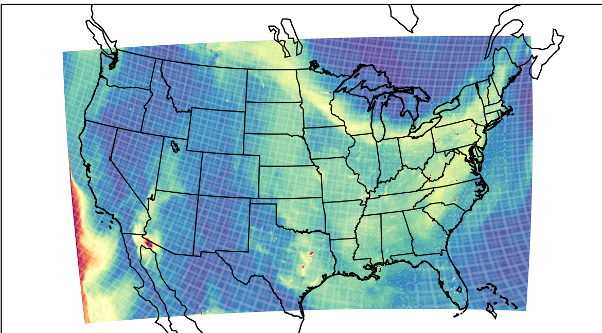
WRF 2023-05-24_20:00:00
