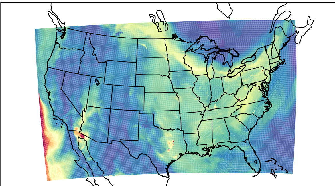
WRF 2023-05-24_18:00:00
