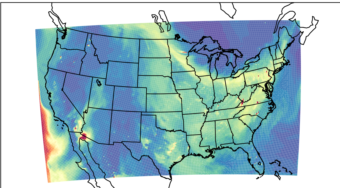
WRF 2023-05-24_23:00:00
