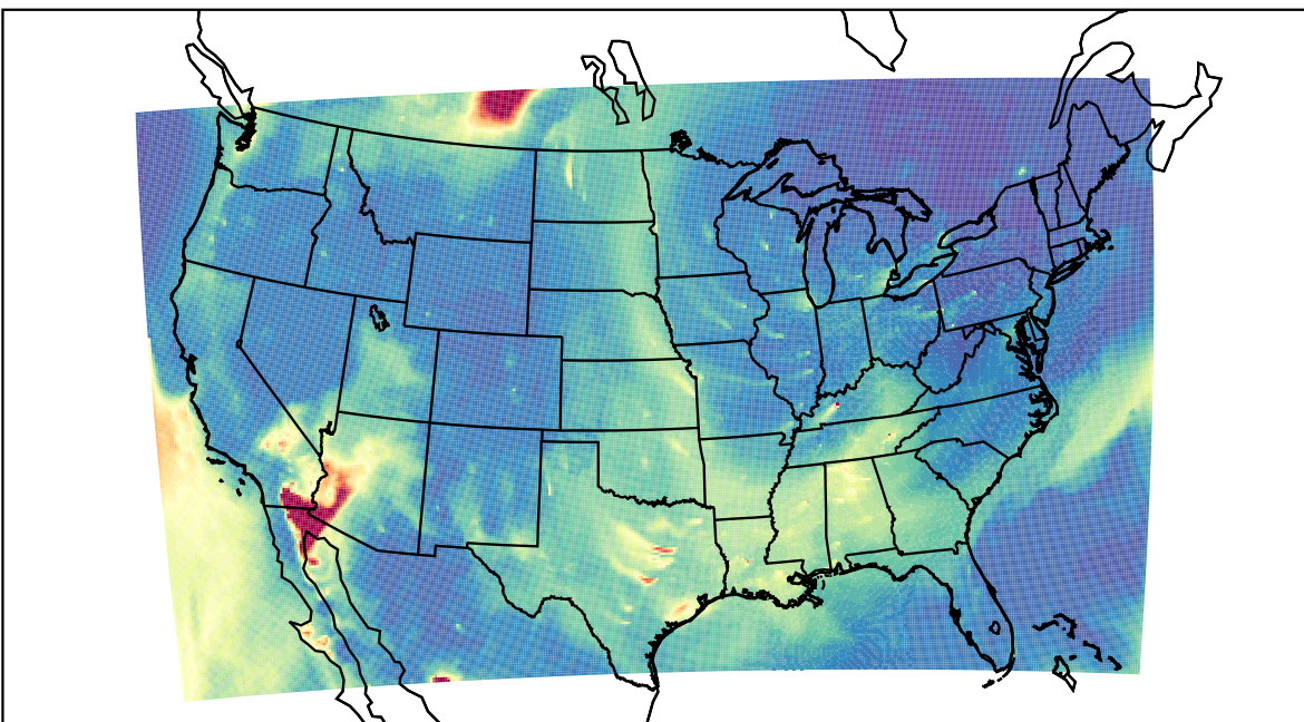
WRF 2023-05-26_13:00:00
