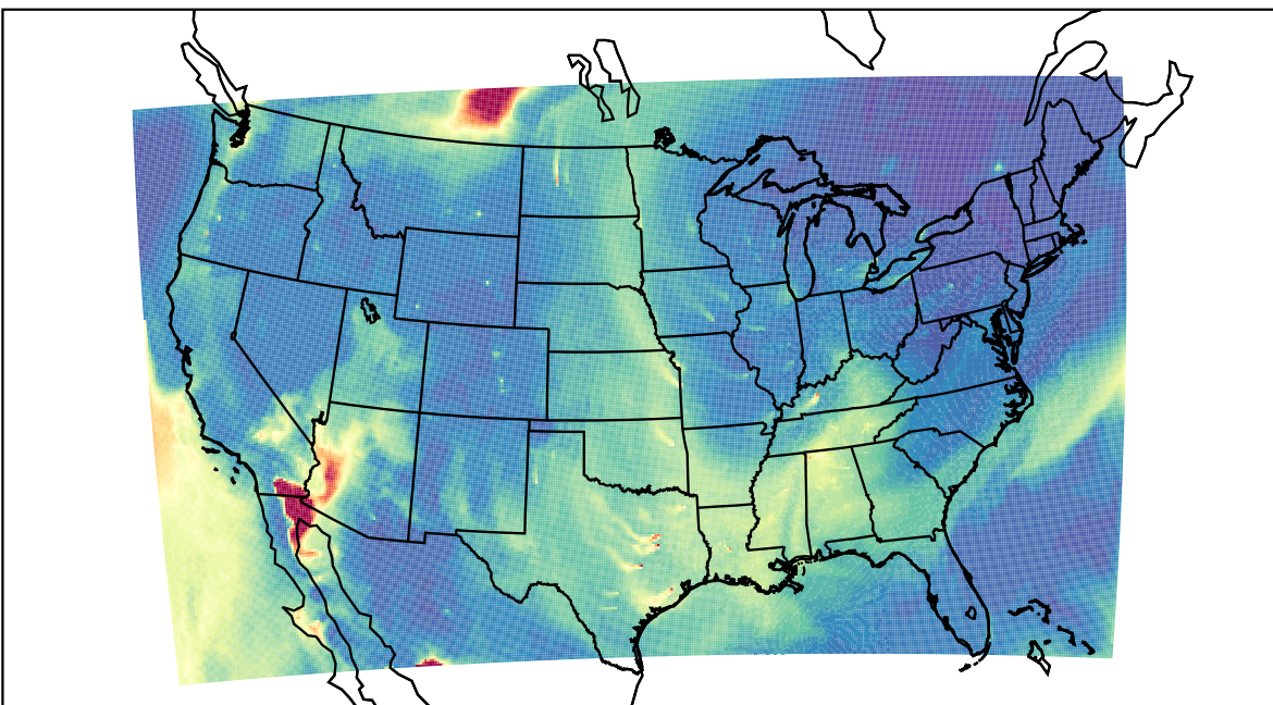
WRF 2023-05-26_15:00:00
