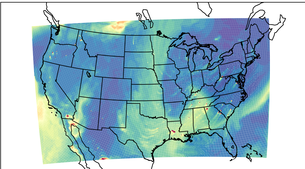
WRF 2023-05-26_23:00:00
