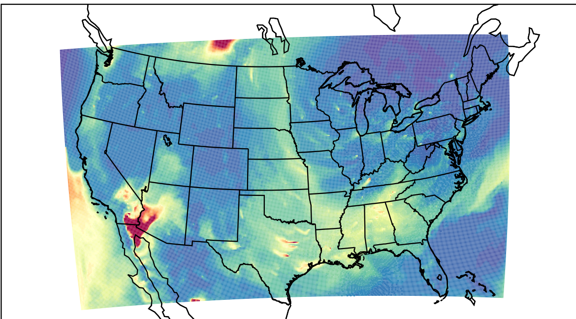
WRF 2023-05-26_10:00:00
