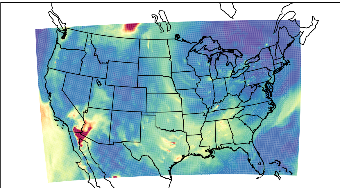
WRF 2023-05-26_12:00:00
