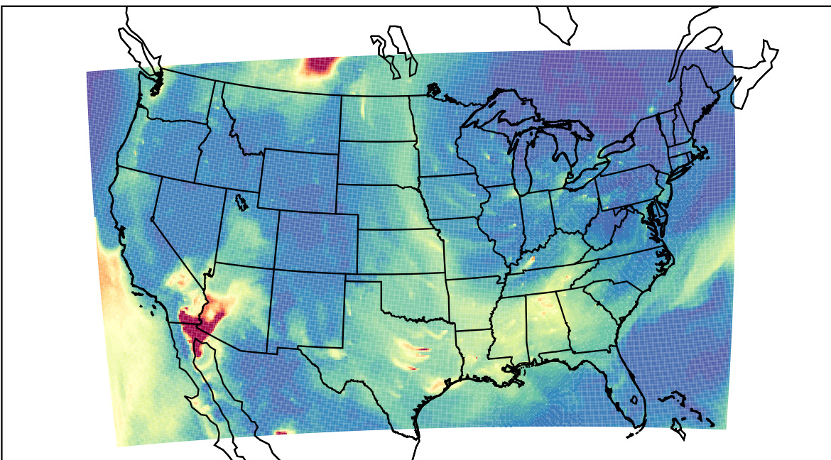
WRF 2023-05-26_11:00:00
