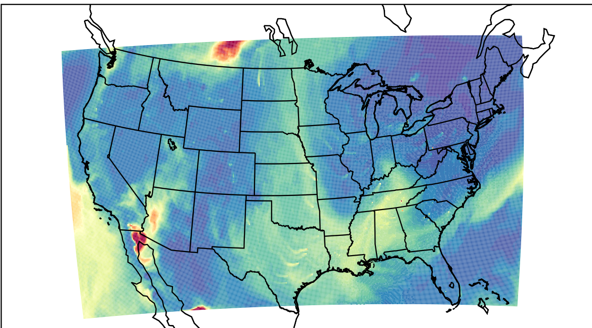
WRF 2023-05-26_17:00:00
