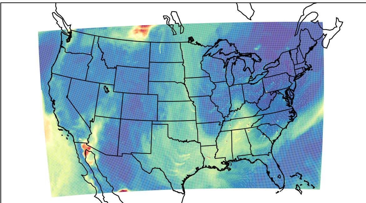
WRF 2023-05-26_19:00:00
