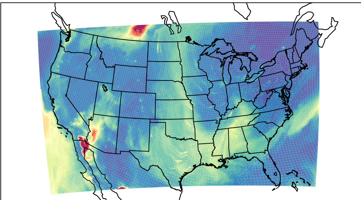
WRF 2023-05-26_16:00:00
