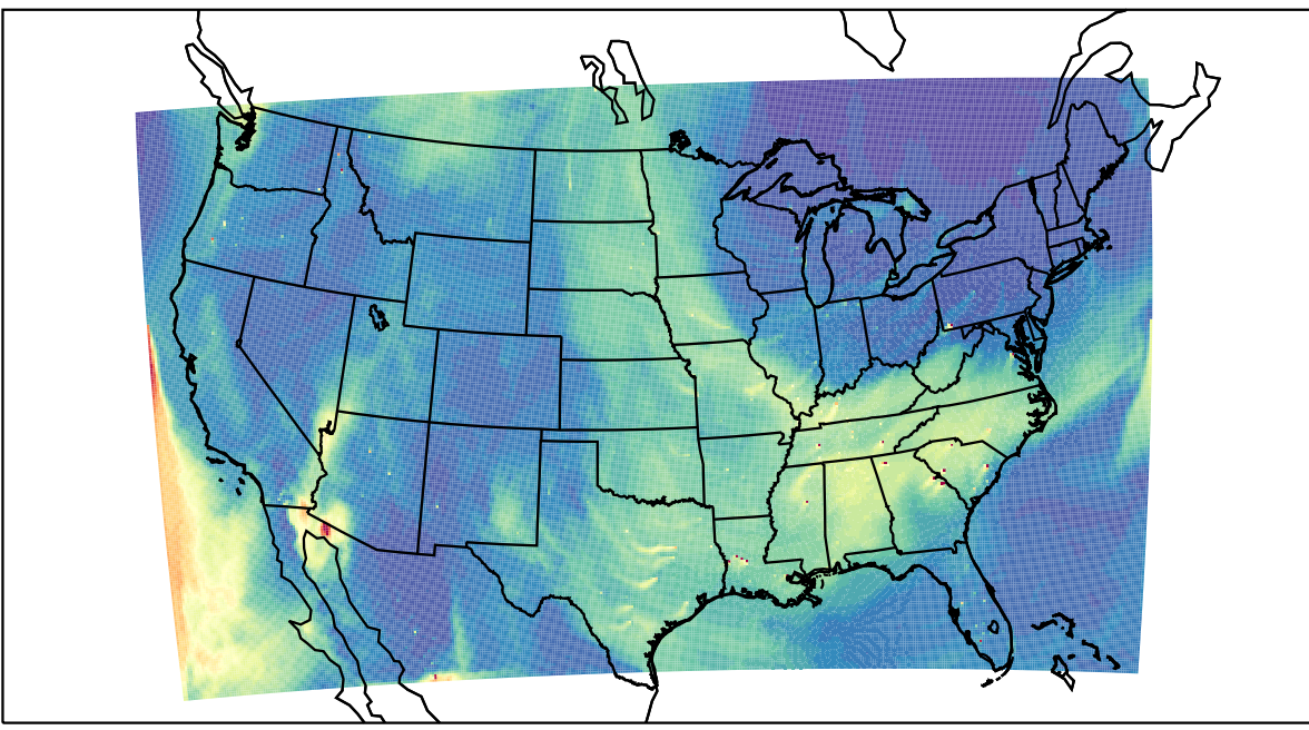
WRF 2023-05-25_20:00:00
