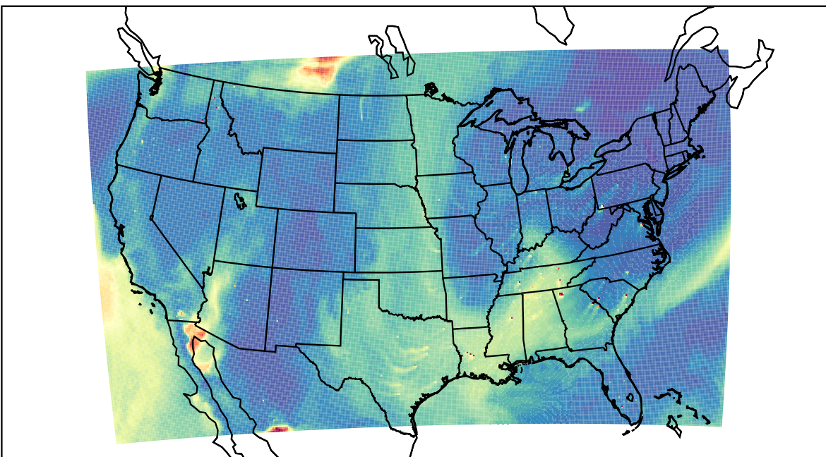
WRF 2023-05-26_20:00:00
