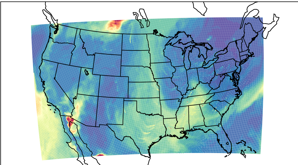
WRF 2023-05-26_18:00:00
