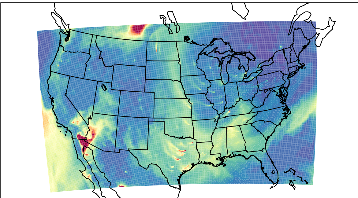
WRF 2023-05-26_14:00:00
