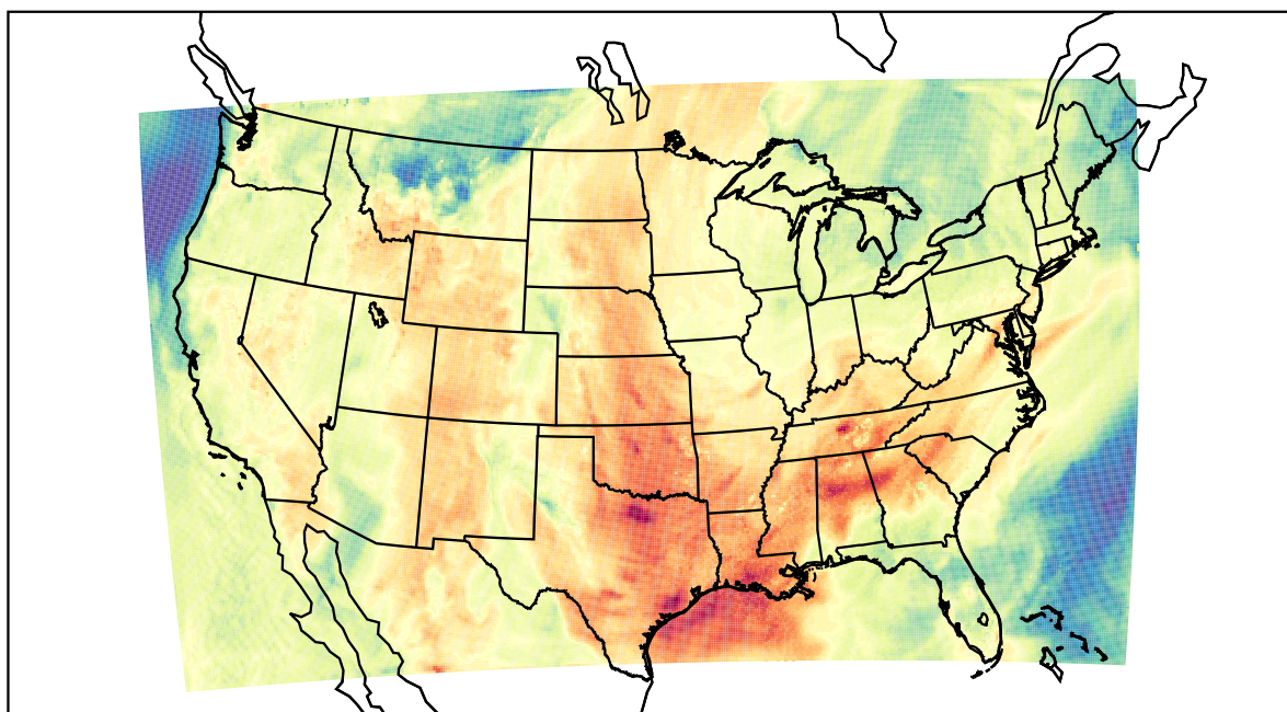
WRF (2023-05-26_19:00:00)
