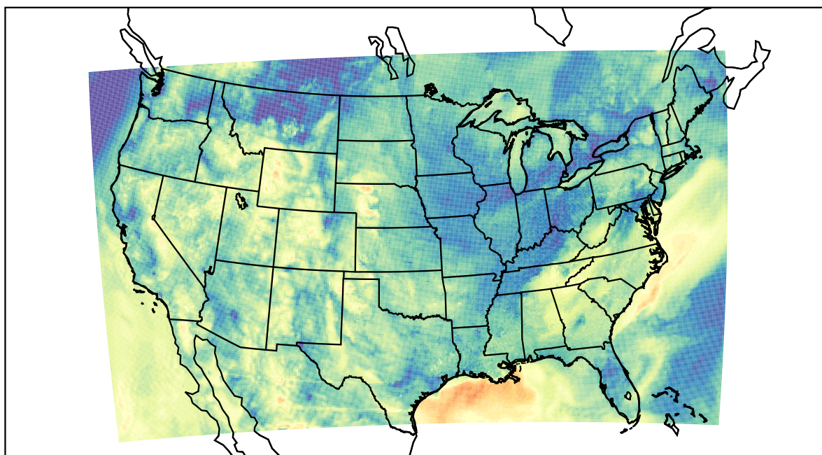
WRF (2023-05-26_13:00:00)
