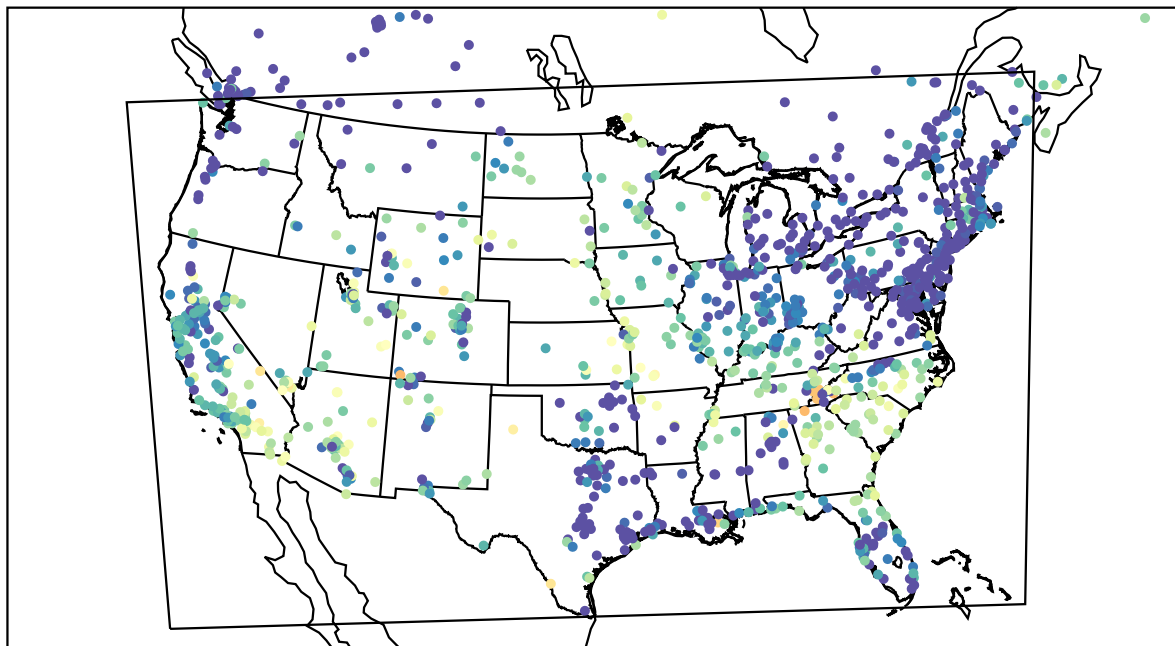
AirNOW (2023-05-26_10:00:00)
