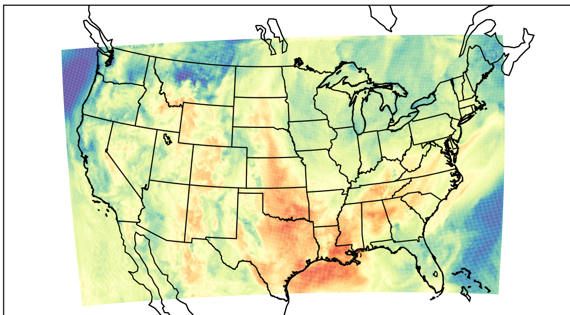
WRF (2023-05-26_16:00:00)
