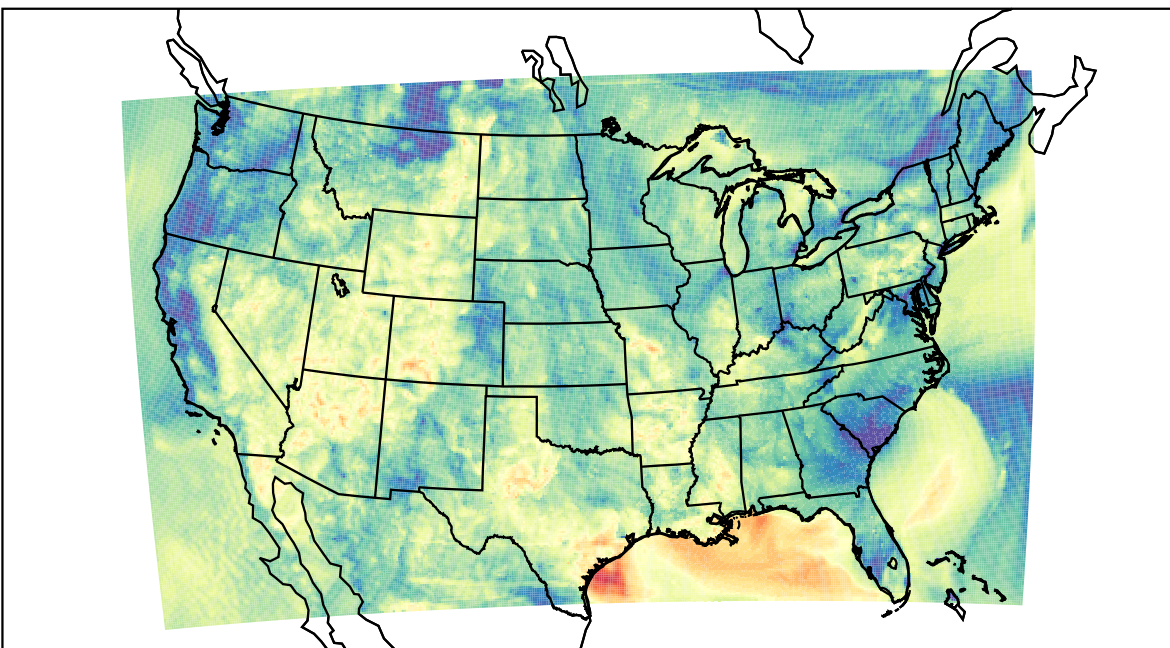
WRF (2023-05-28_10:00:00)
