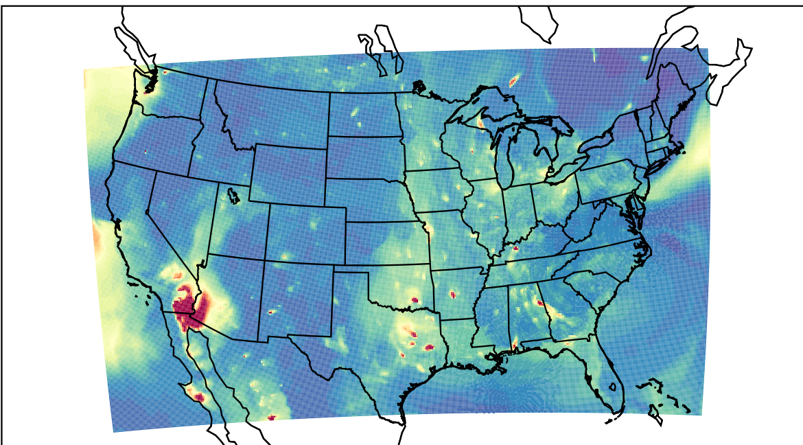
WRF 2023-05-30_03:00:00
