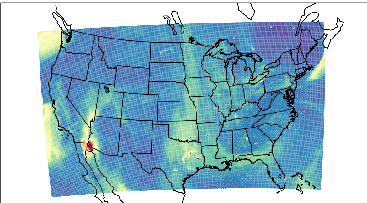
WRF 2023-05-29_20:00:00
