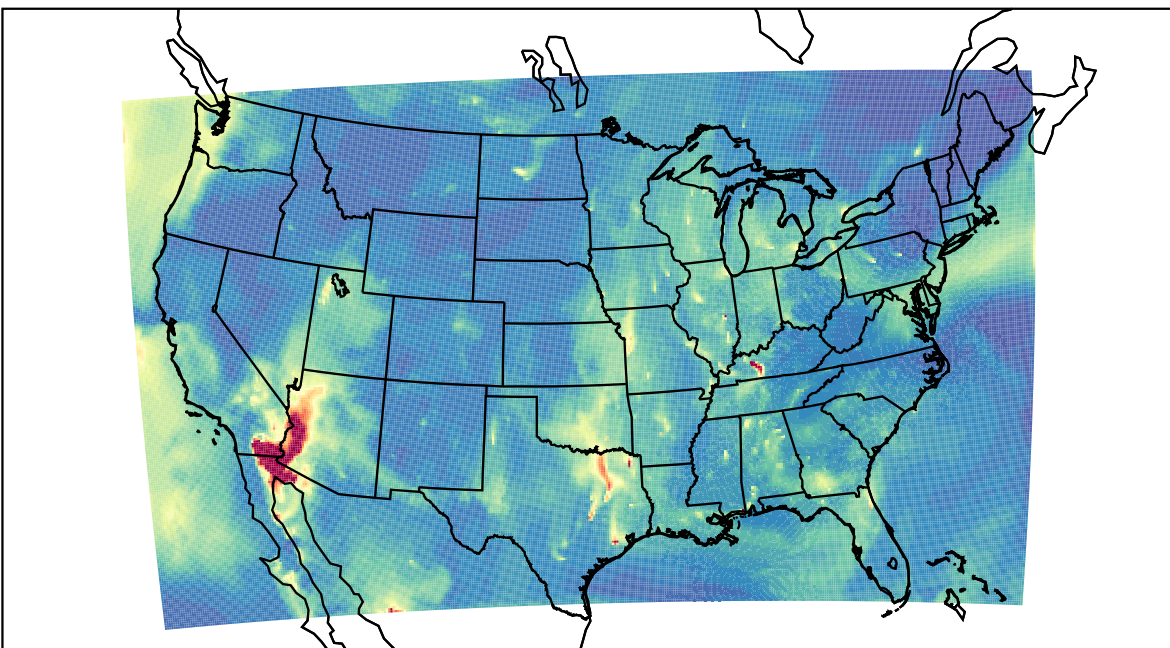
WRF 2023-05-30_13:00:00
