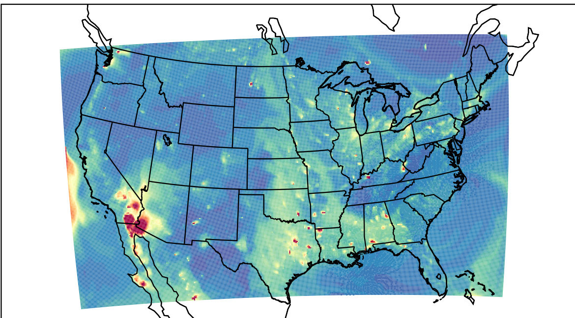
WRF 2023-05-29_03:00:00
