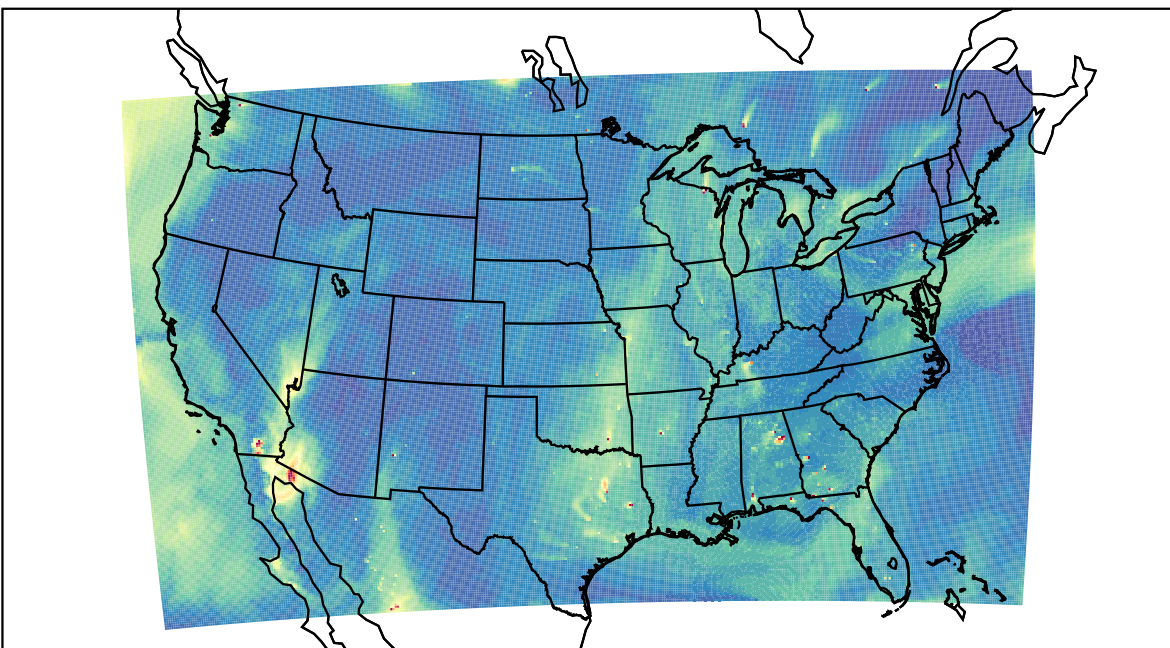
WRF 2023-05-30_22:00:00
