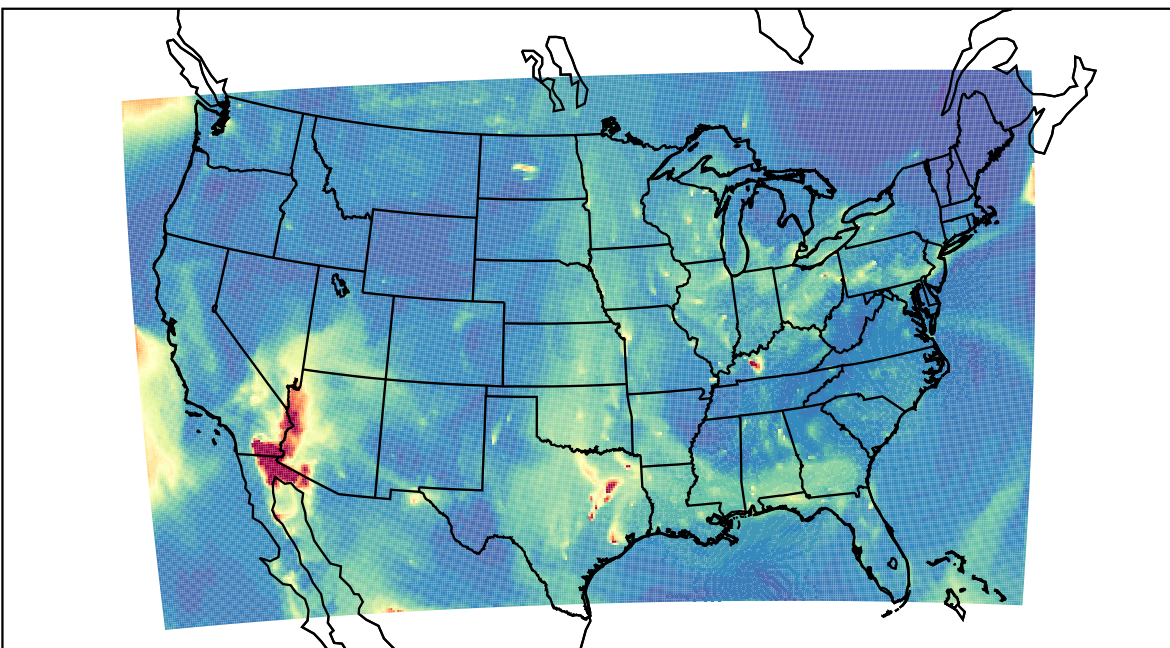
WRF 2023-05-29_13:00:00
