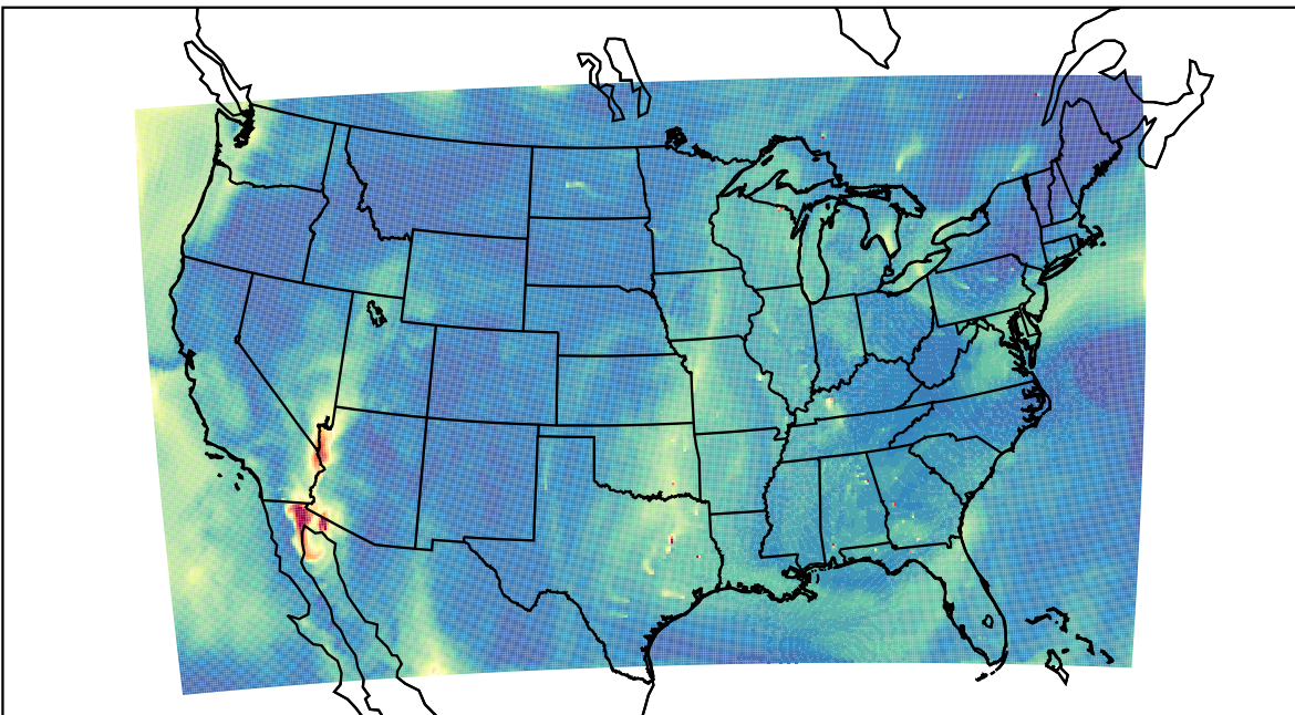
WRF 2023-05-30_18:00:00
