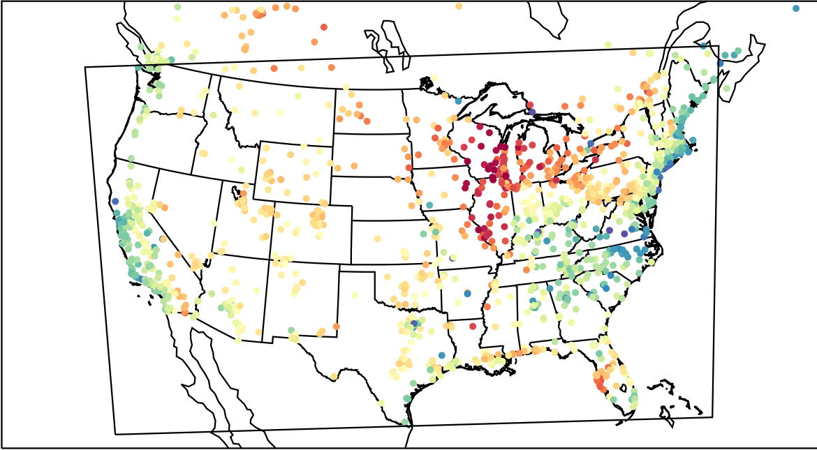
AirNOW (2023-05-30_23:00:00)
