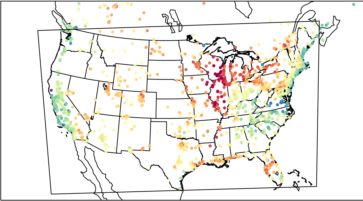
AirNOW (2023-05-30_20:00:00)
