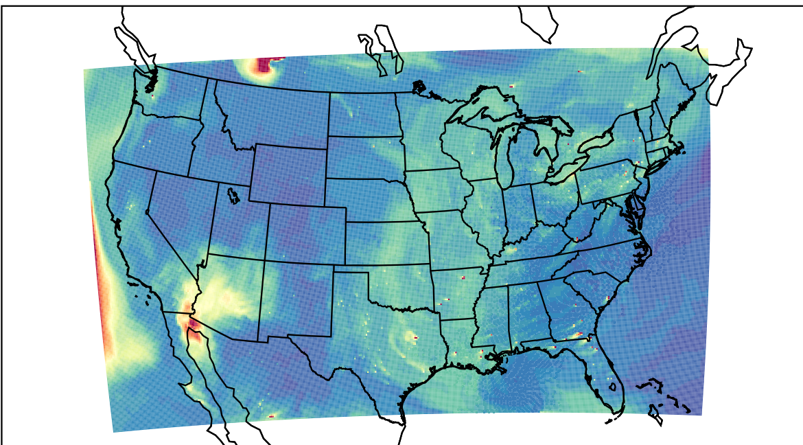
WRF 2023-06-01_22:00:00
