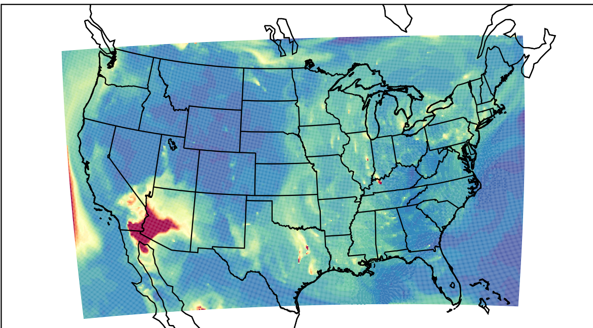
WRF 2023-06-01_12:00:00
