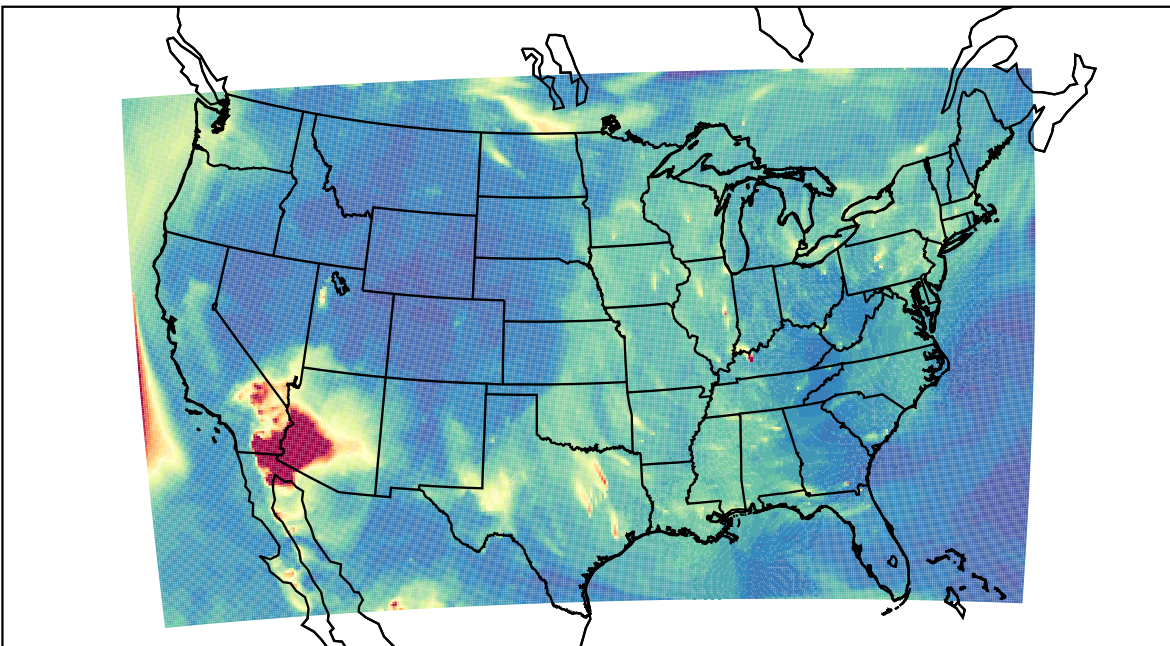
WRF 2023-06-01_08:00:00
