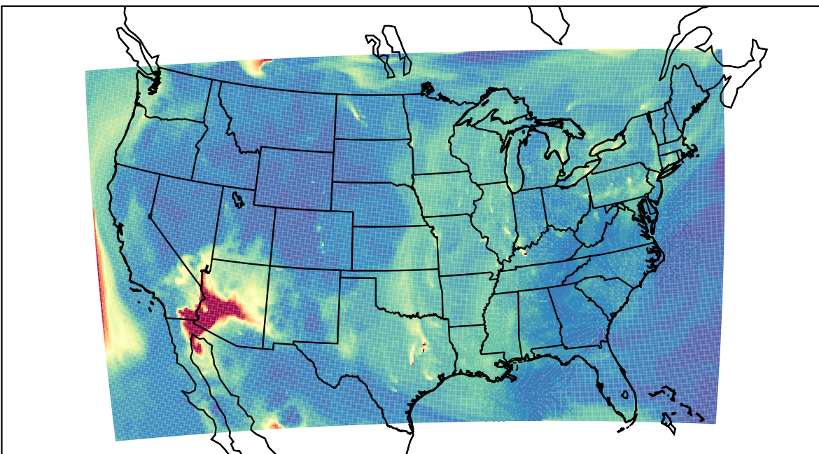
WRF 2023-06-01_15:00:00
