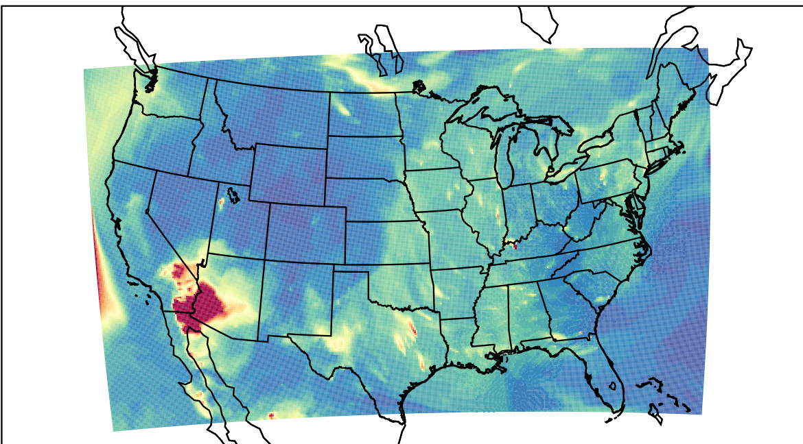
WRF 2023-06-01_07:00:00
