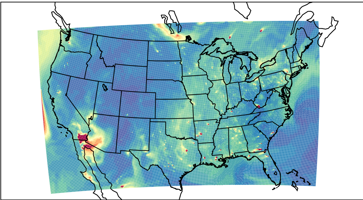
WRF 2023-06-01_01:00:00
