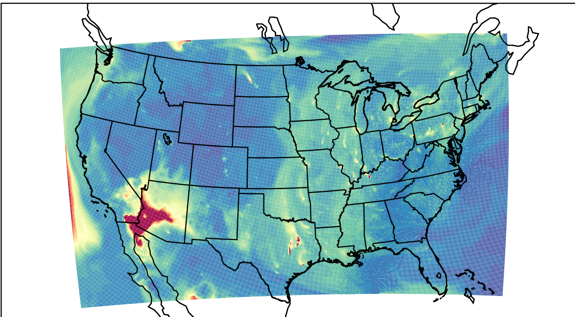
WRF 2023-06-01_14:00:00
