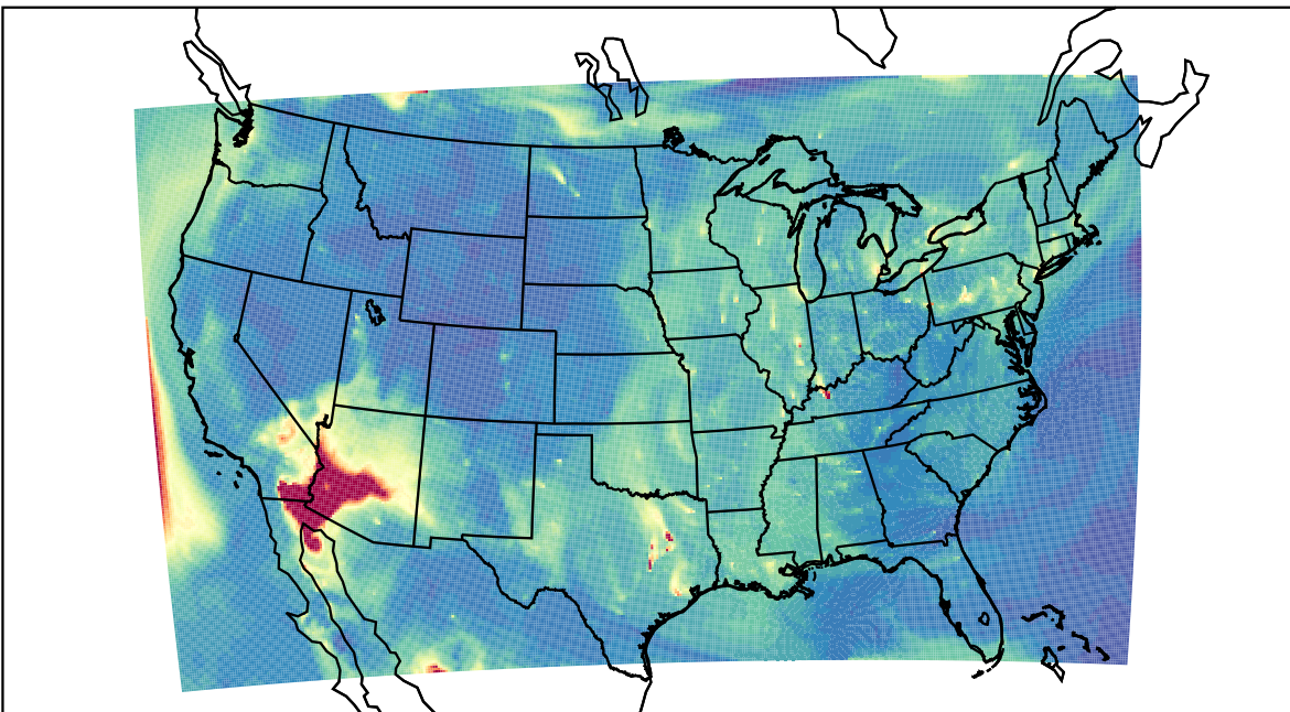
WRF 2023-06-01_13:00:00
