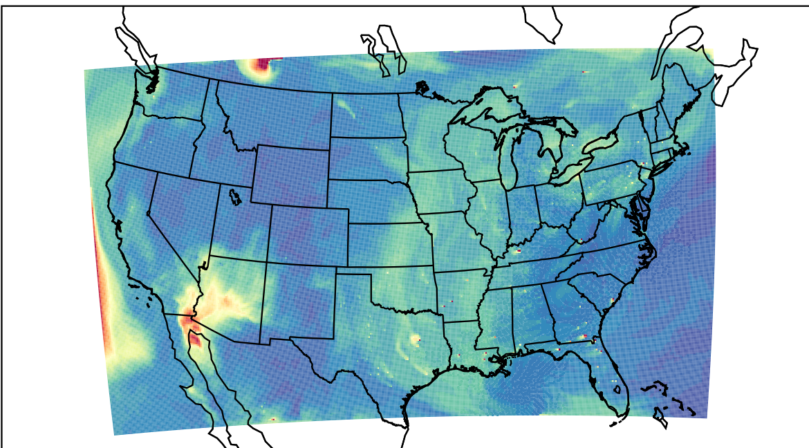
WRF 2023-06-01_20:00:00
