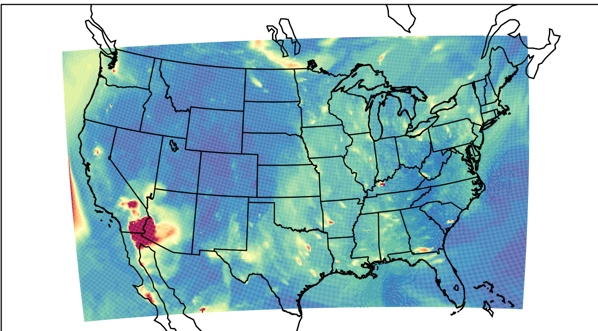
WRF 2023-06-01_04:00:00
