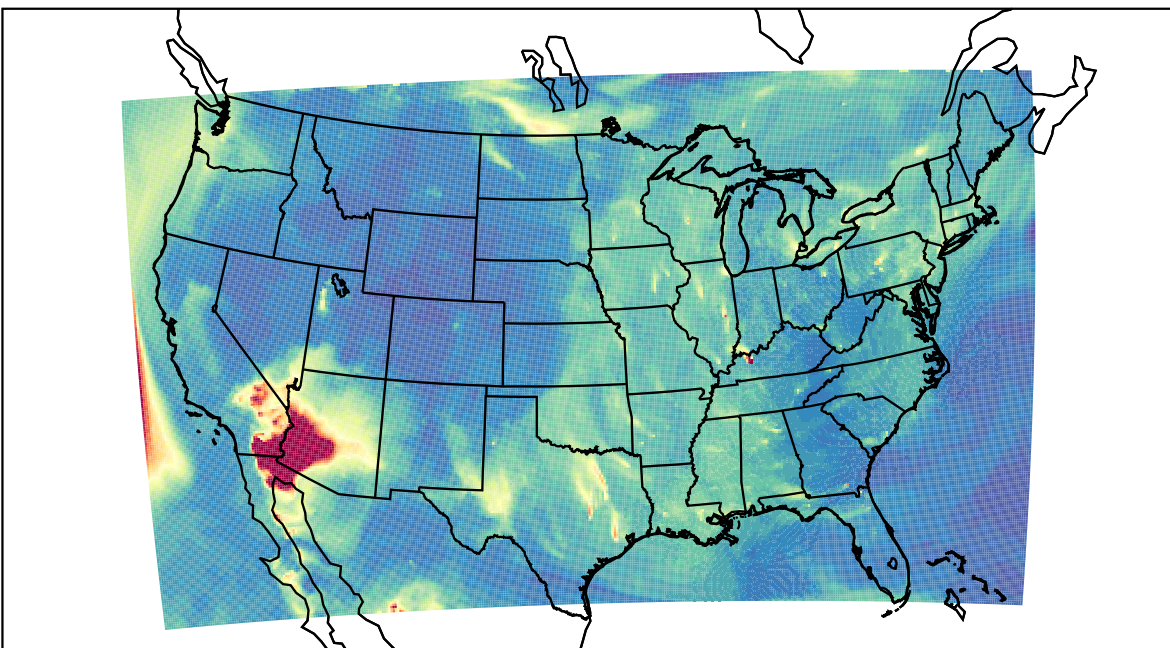
WRF 2023-06-01_09:00:00
