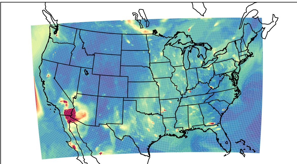
WRF 2023-06-01_03:00:00
