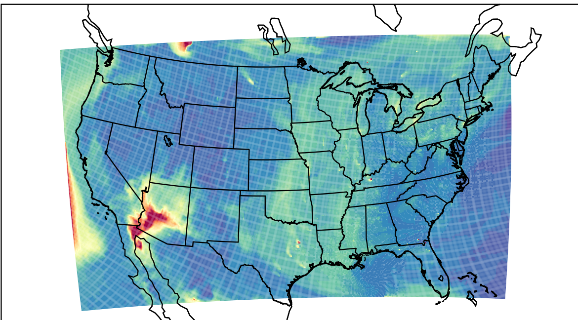
WRF 2023-06-01_17:00:00
