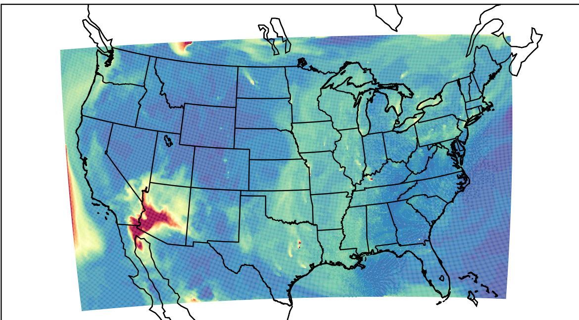
WRF 2023-06-01_16:00:00
