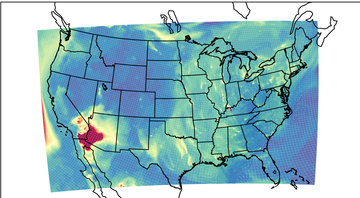
WRF 2023-06-01_10:00:00
