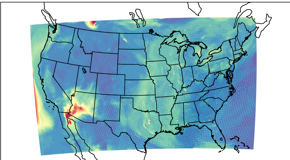
WRF 2023-06-01_18:00:00
