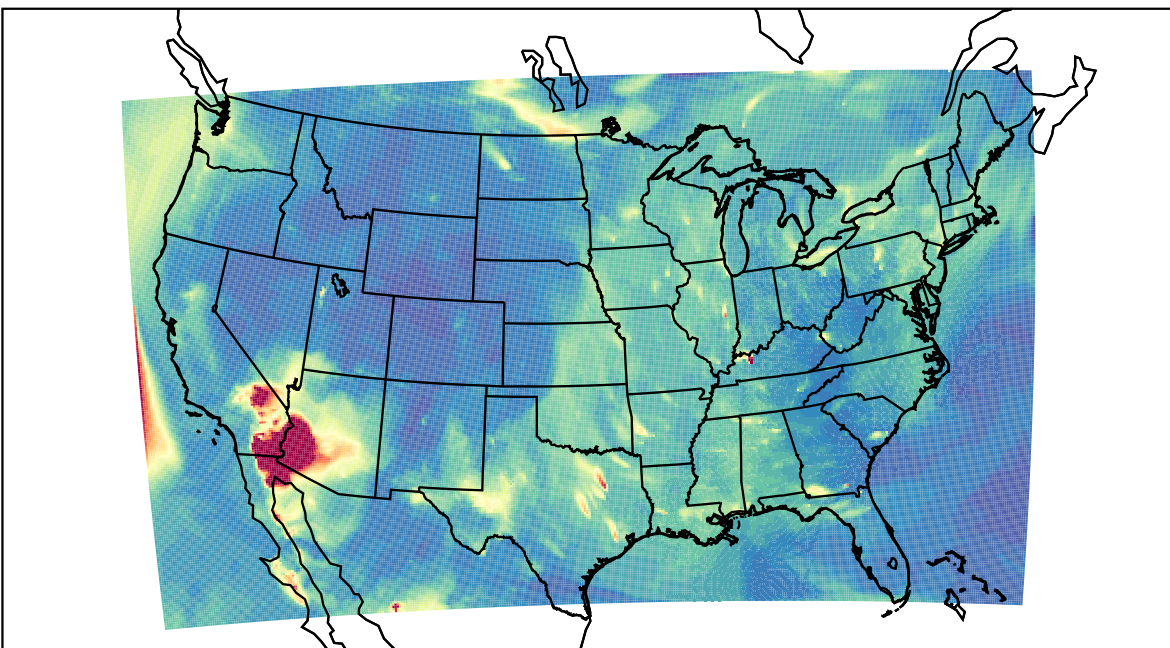
WRF 2023-06-01_06:00:00
