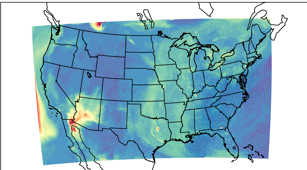
WRF 2023-06-01_19:00:00
