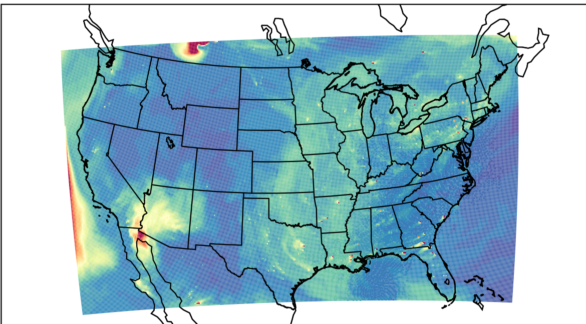
WRF 2023-06-01_23:00:00
