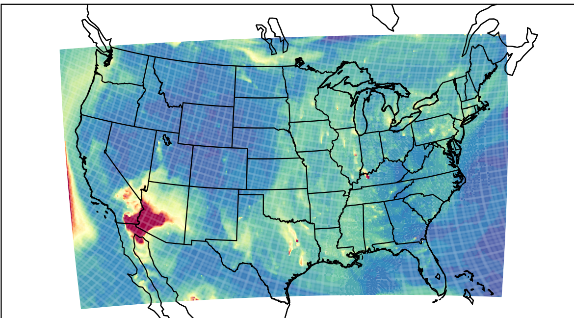
WRF 2023-06-01_11:00:00
