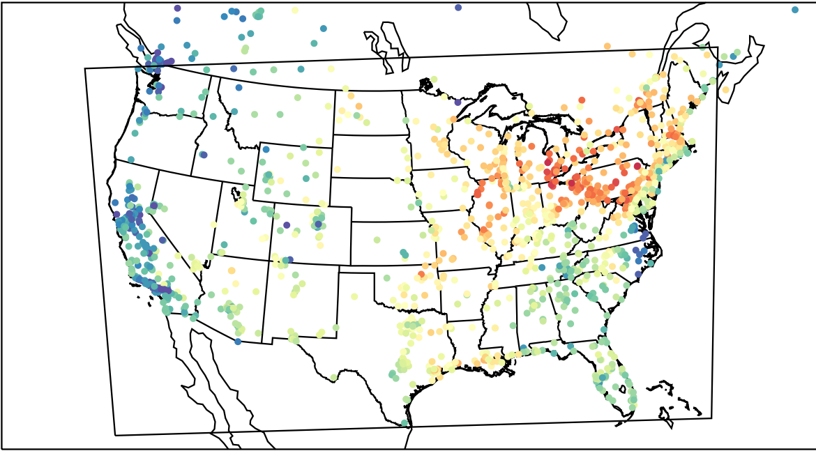
AirNOW (2023-06-01_15:00:00)
