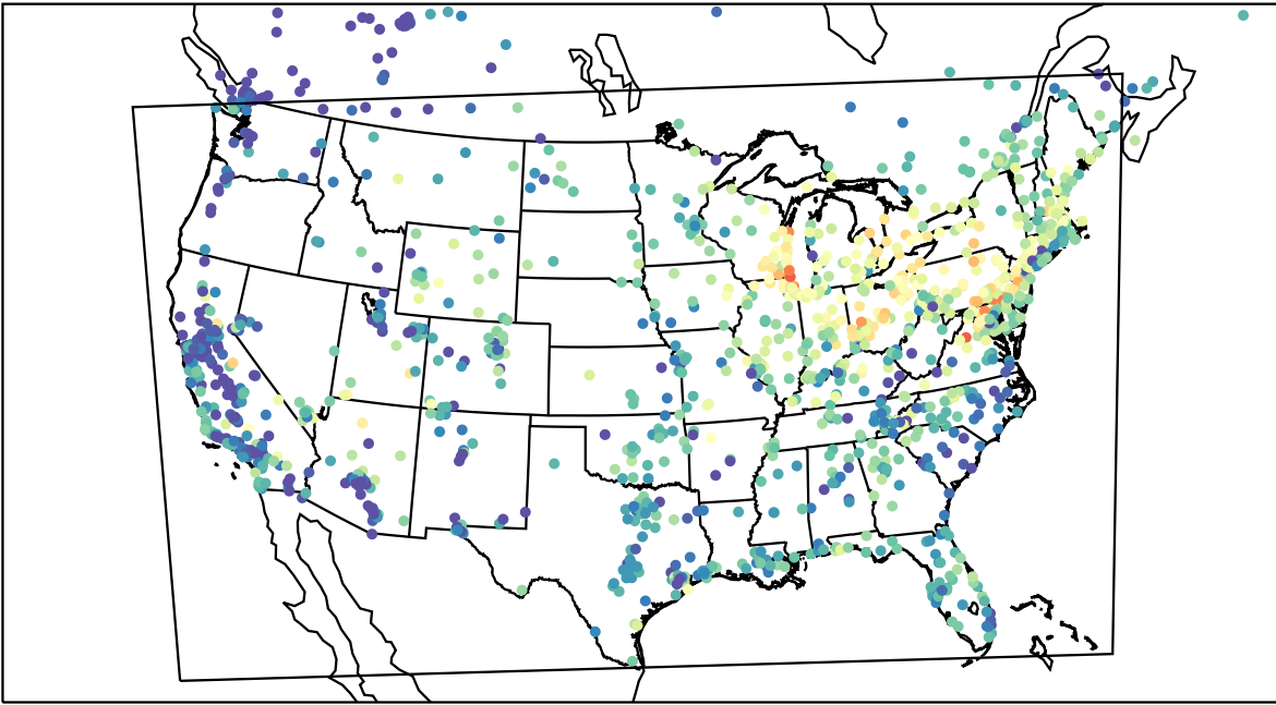
AirNOW (2023-06-02_13:00:00)
