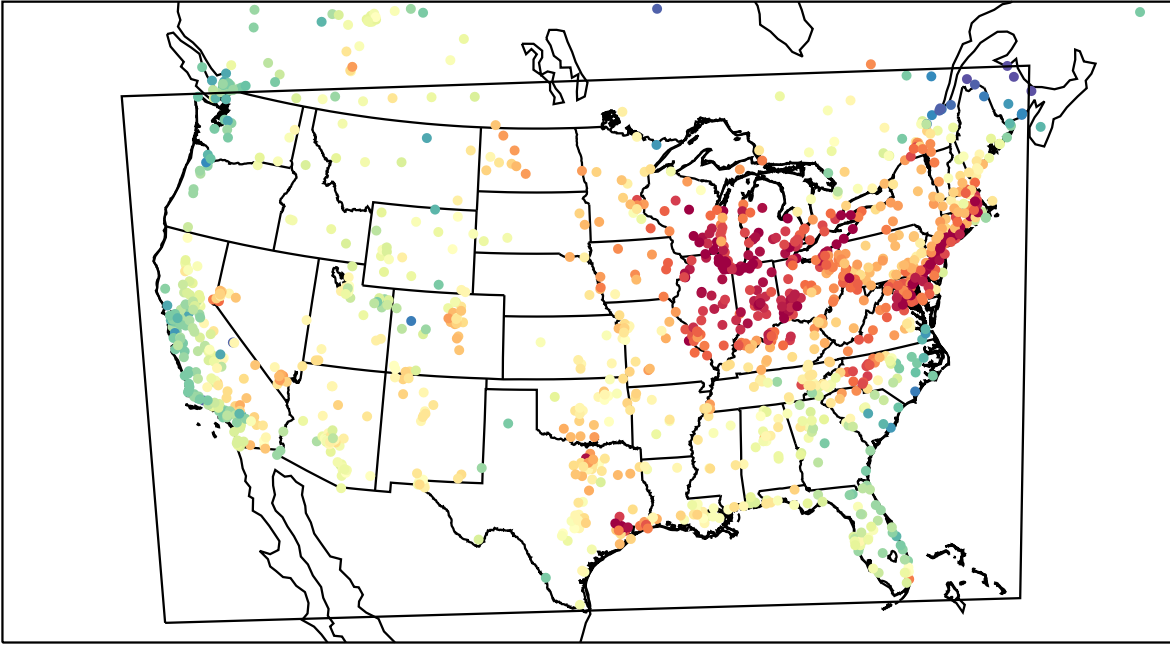
AirNOW (2023-06-02_18:00:00)
