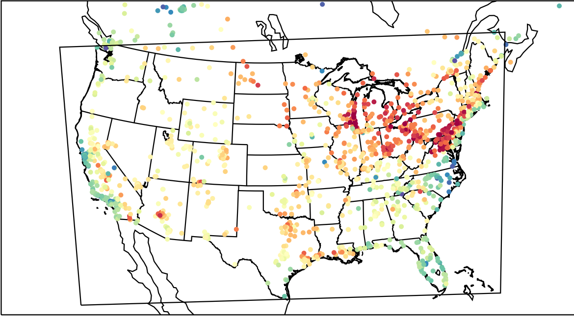
AirNOW (2023-06-01_22:00:00)
