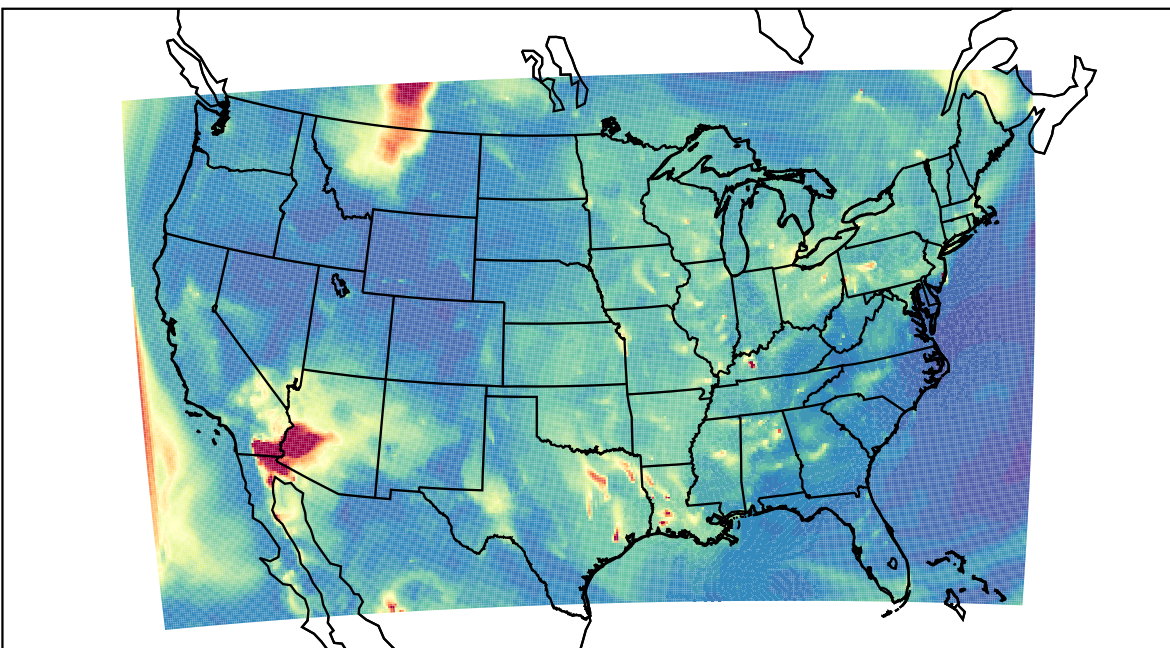
WRF 2023-06-02_10:00:00
