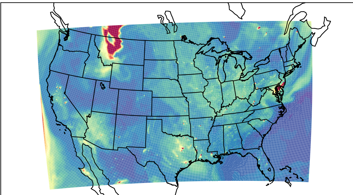
WRF 2023-06-03_23:00:00
