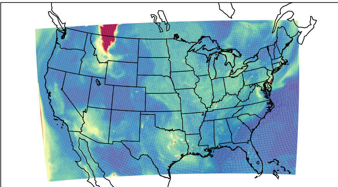
WRF 2023-06-03_19:00:00
