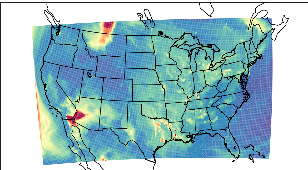
WRF 2023-06-02_12:00:00
