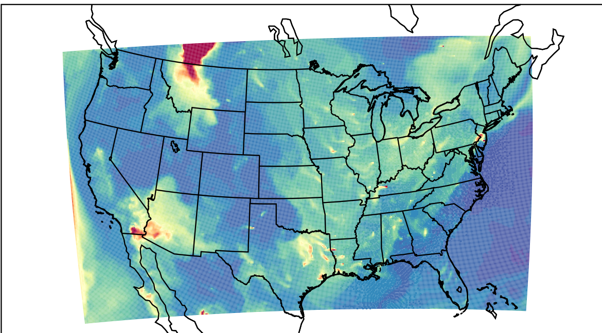
WRF 2023-06-03_10:00:00
