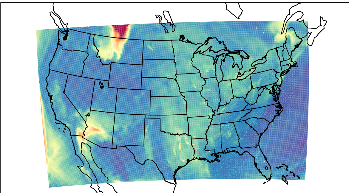
WRF 2023-06-02_18:00:00
