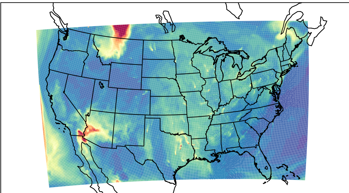
WRF 2023-06-02_16:00:00
