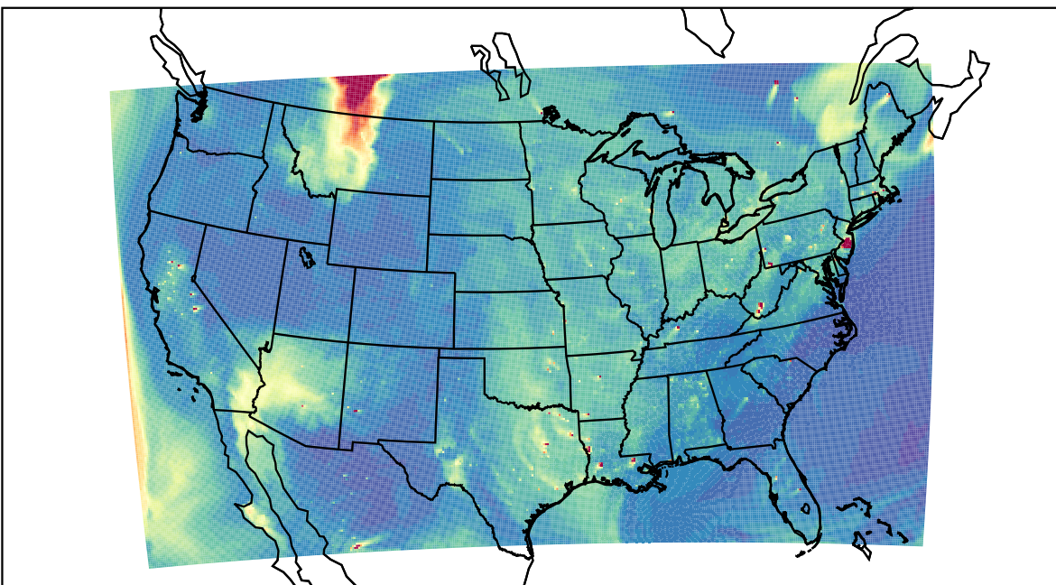
WRF 2023-06-02_23:00:00
