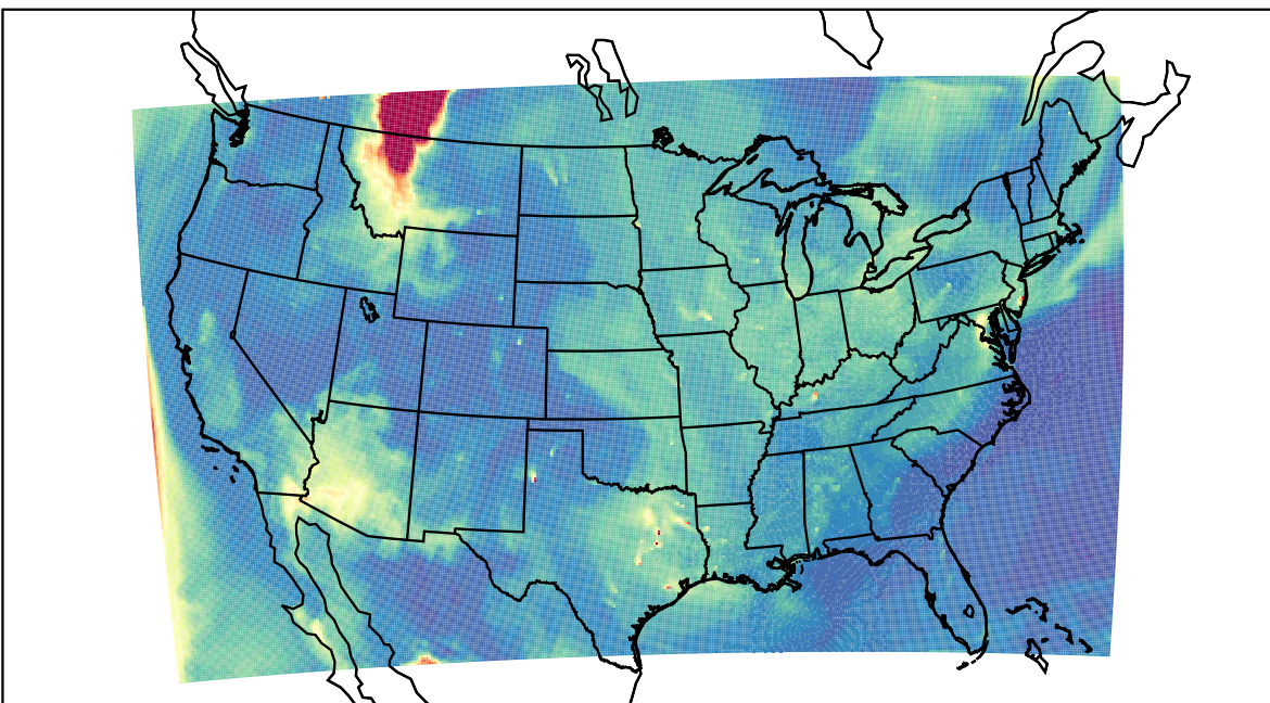
WRF 2023-06-03_16:00:00
