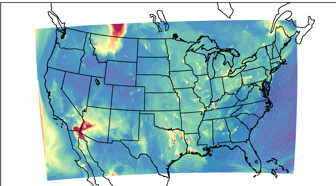
WRF 2023-06-02_14:00:00
