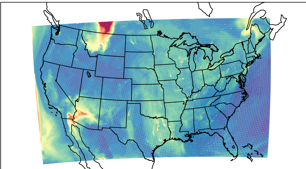
WRF 2023-06-02_17:00:00
