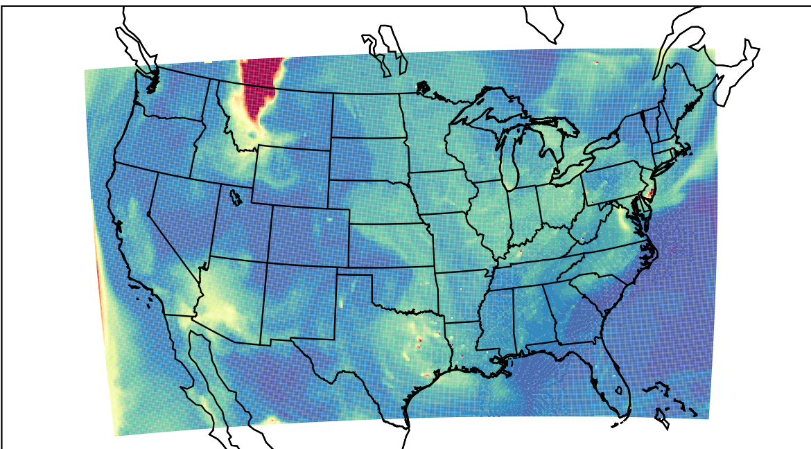
WRF 2023-06-03_18:00:00
