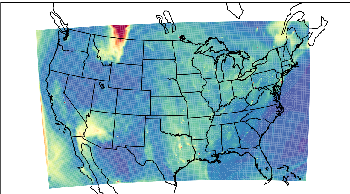
WRF 2023-06-02_20:00:00
