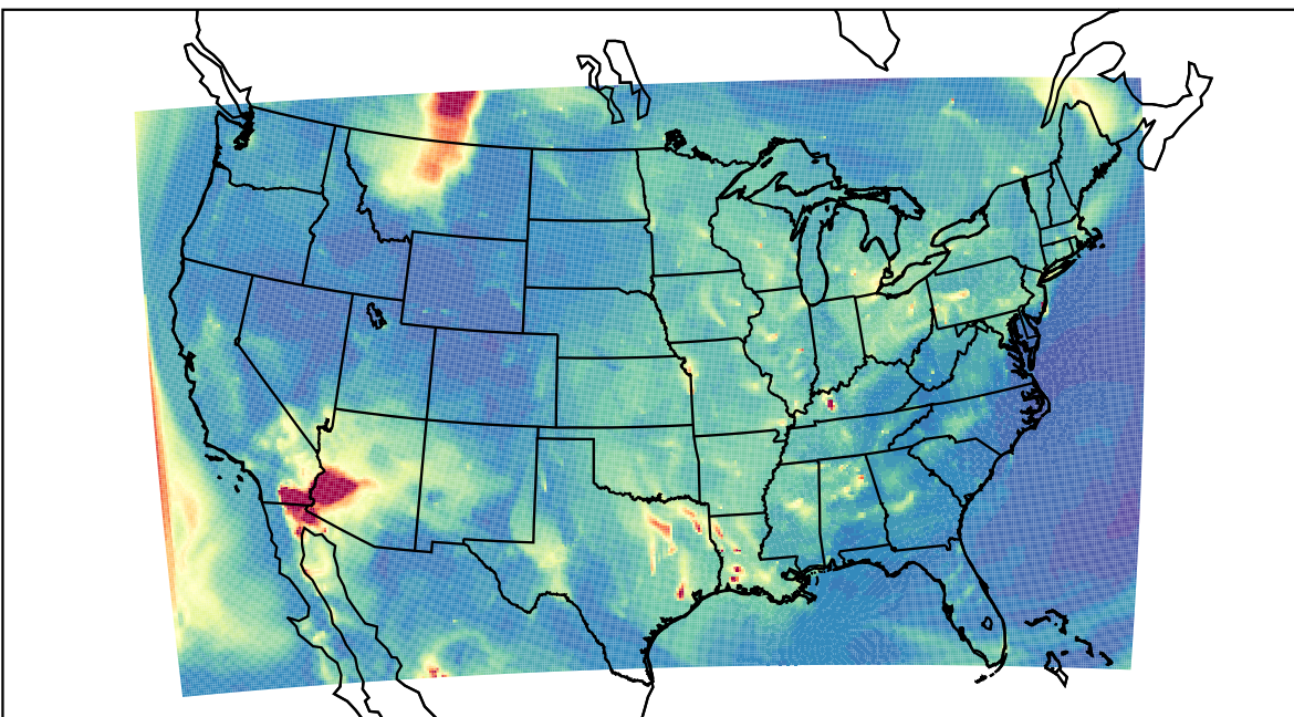
WRF 2023-06-02_11:00:00
