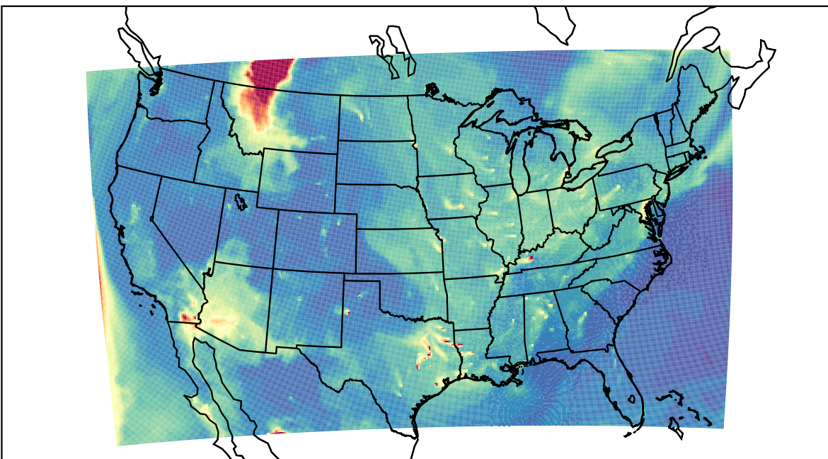
WRF 2023-06-03_14:00:00
