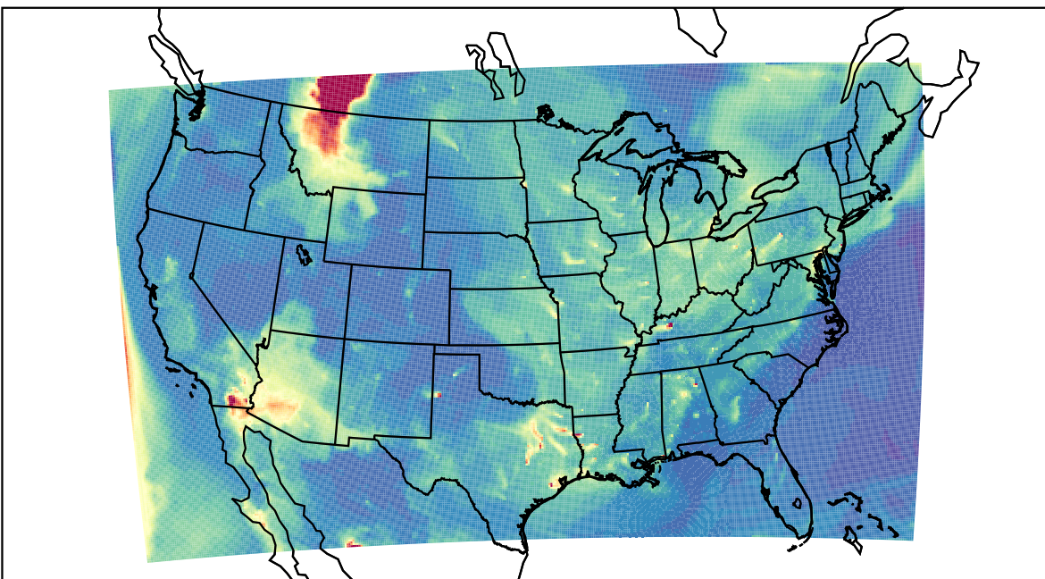
WRF 2023-06-03_13:00:00
