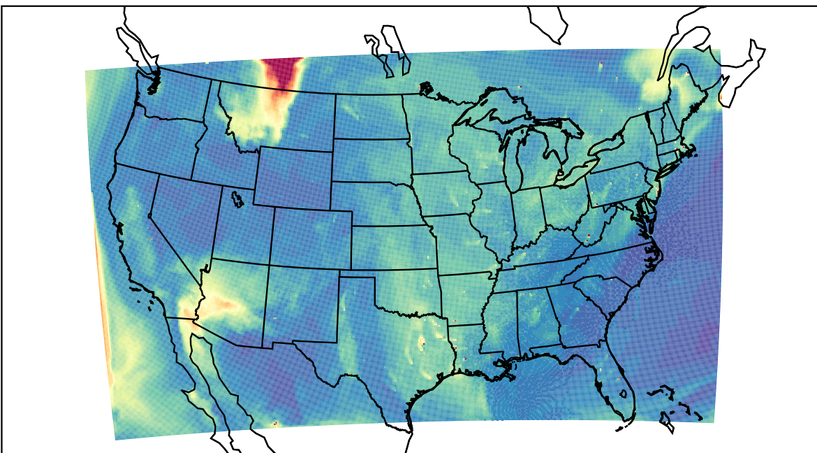
WRF 2023-06-02_19:00:00
