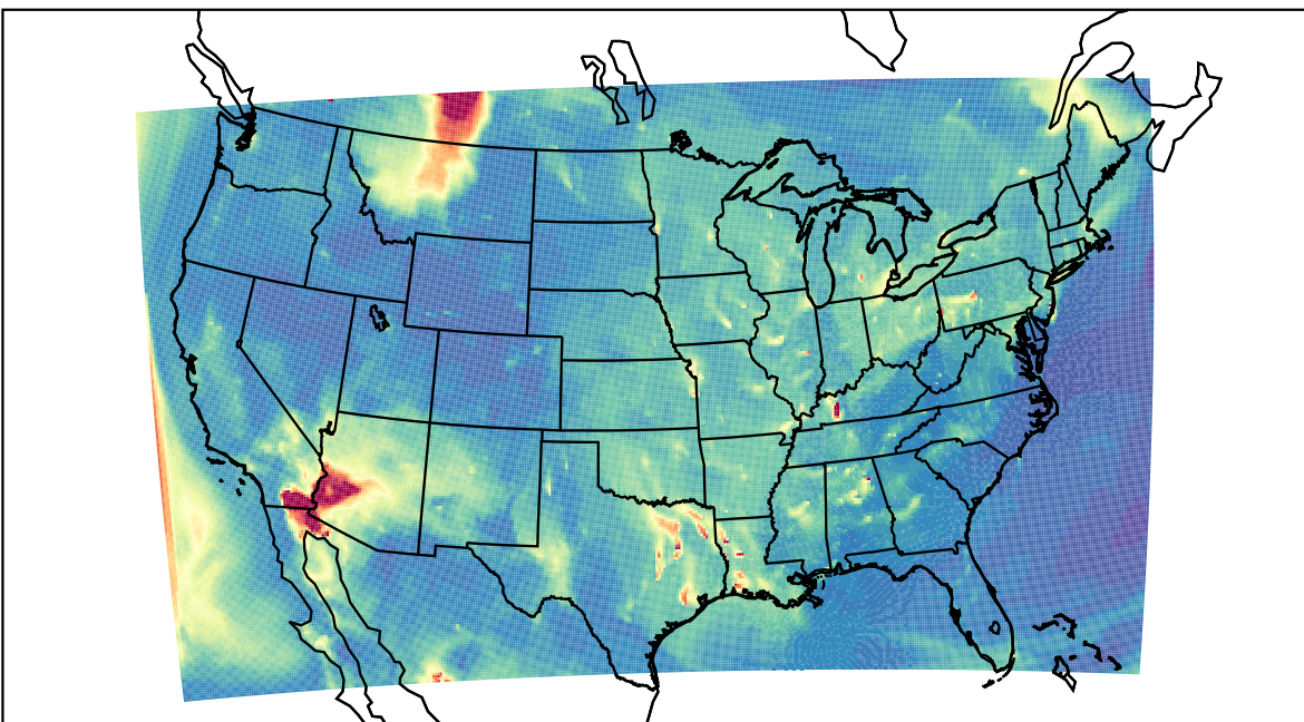
WRF 2023-06-02_13:00:00
