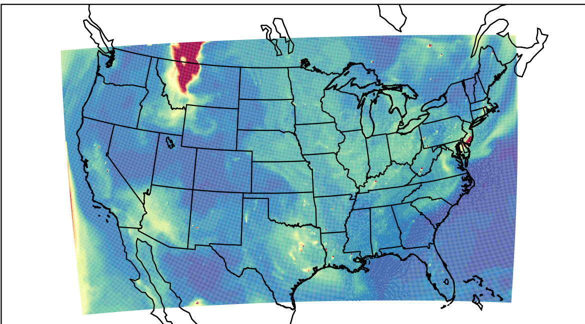
WRF 2023-06-03_20:00:00
