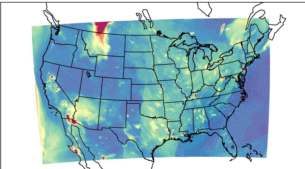
WRF 2023-06-03_03:00:00
