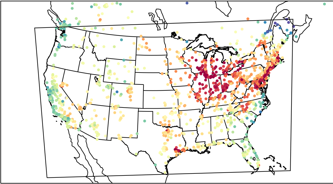
AirNOW (2023-06-02_18:00:00)
