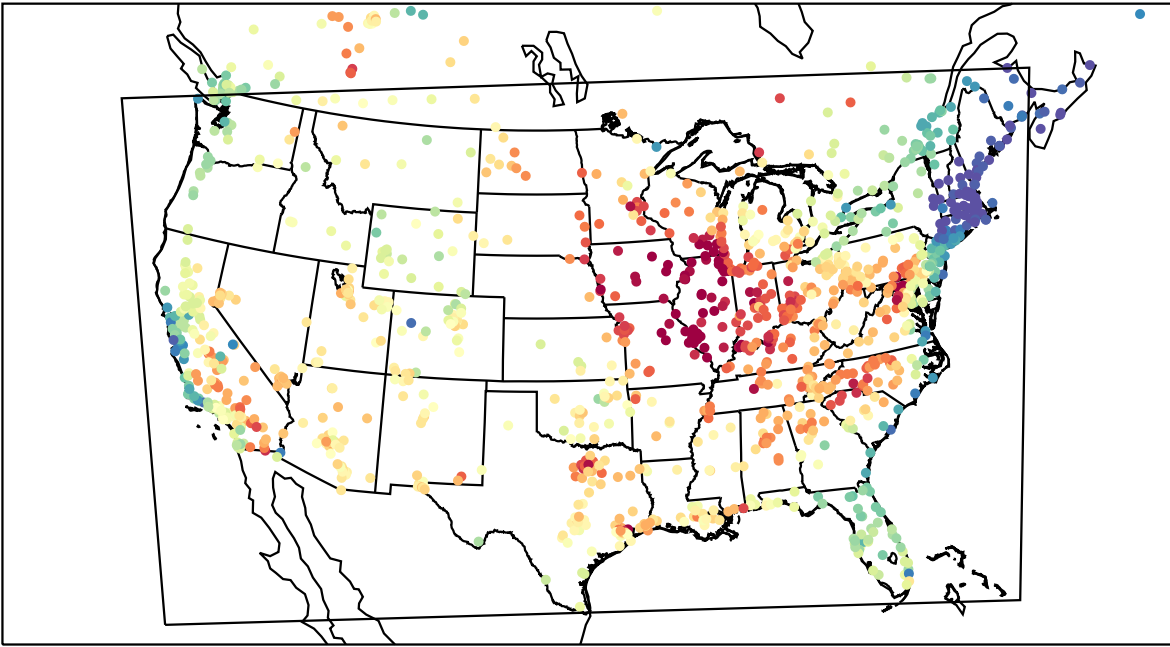
AirNOW (2023-06-03_18:00:00)
