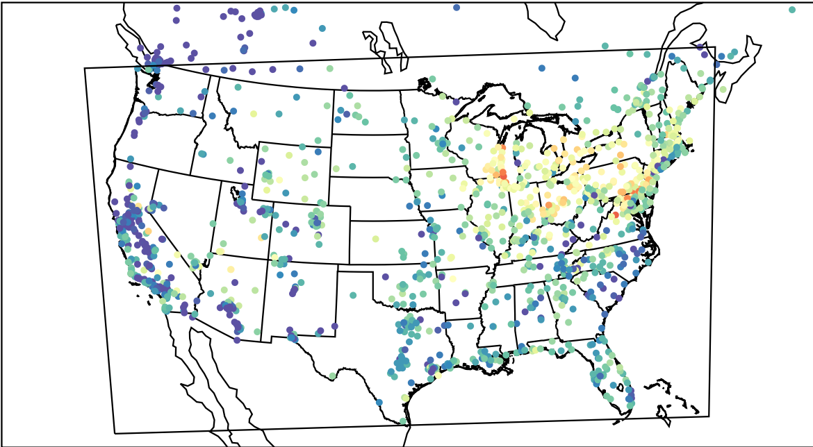
AirNOW (2023-06-02_13:00:00)
