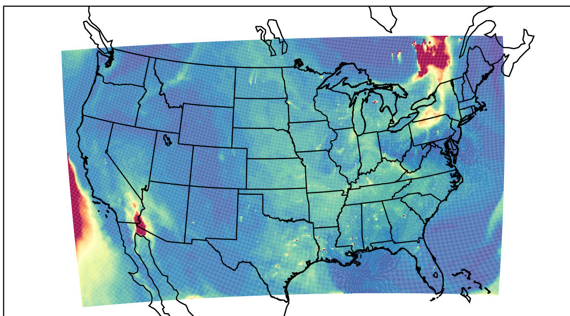
WRF 2023-06-05_20:00:00
