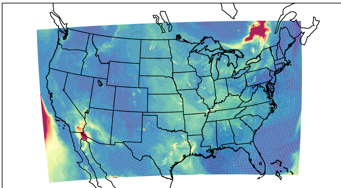
WRF 2023-06-05_16:00:00
