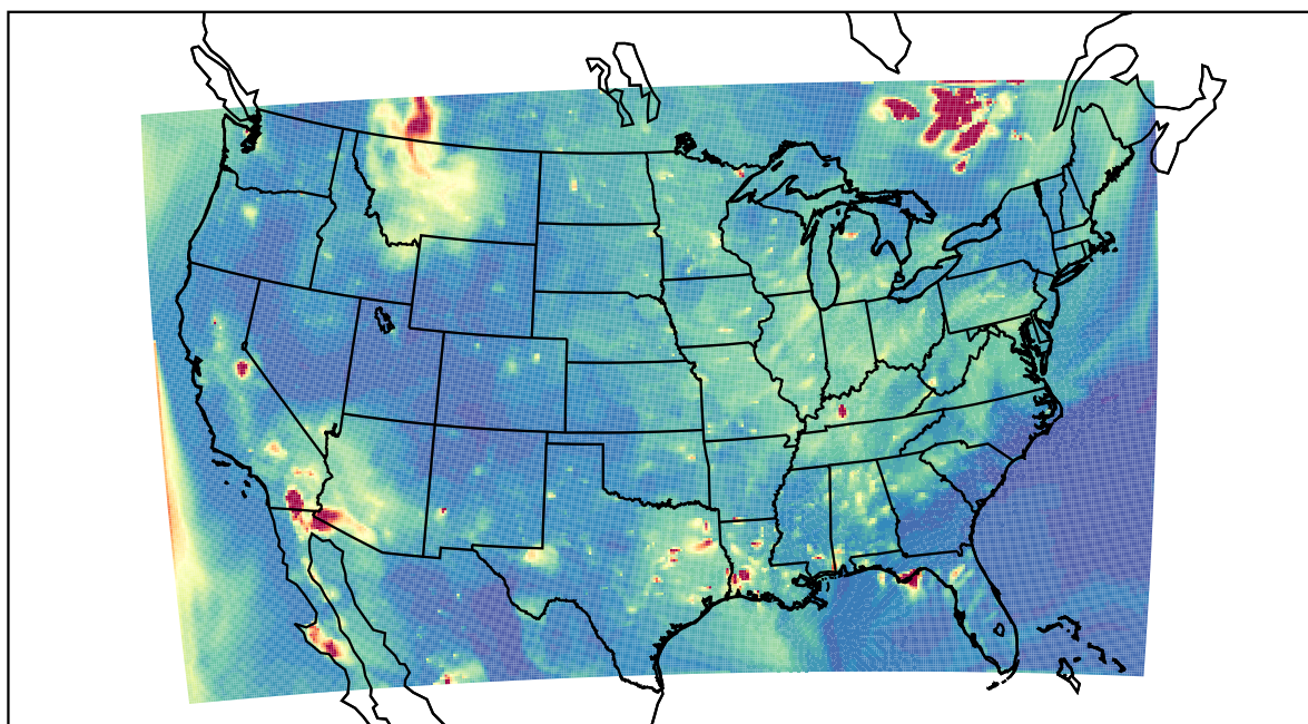
WRF 2023-06-04_03:00:00
