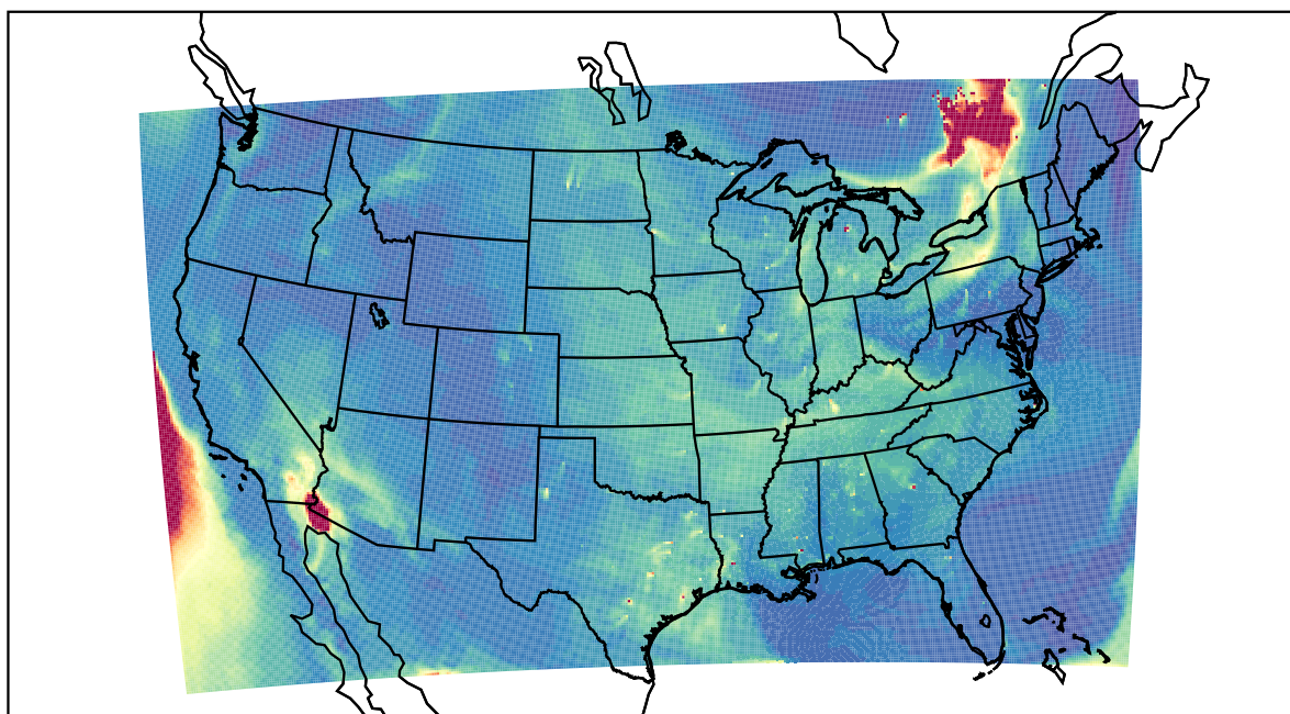
WRF 2023-06-05_18:00:00
