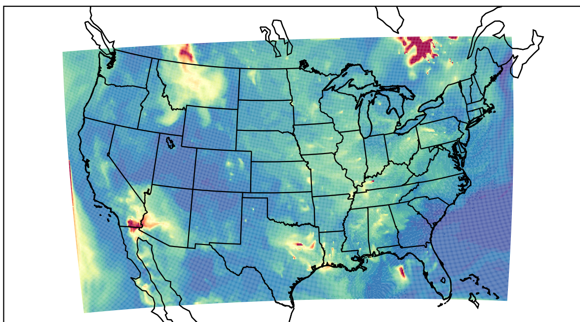
WRF 2023-06-04_10:00:00
