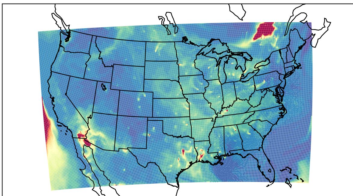
WRF 2023-06-05_13:00:00
