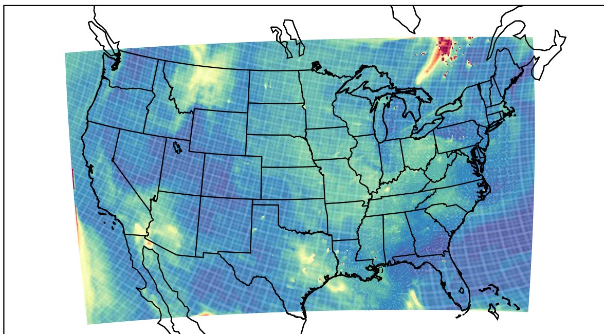
WRF 2023-06-04_18:00:00
