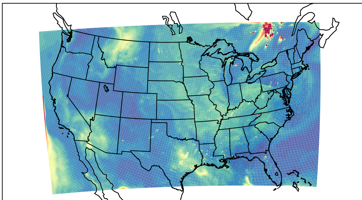
WRF 2023-06-04_20:00:00
