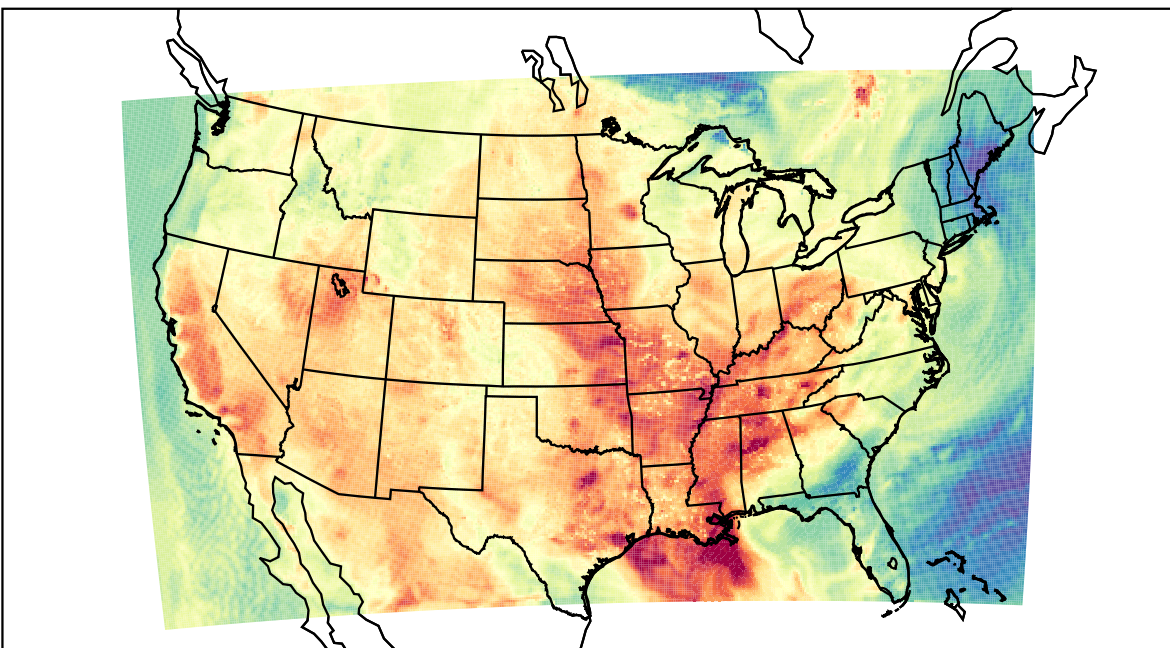
WRF (2023-06-04_20:00:00)
