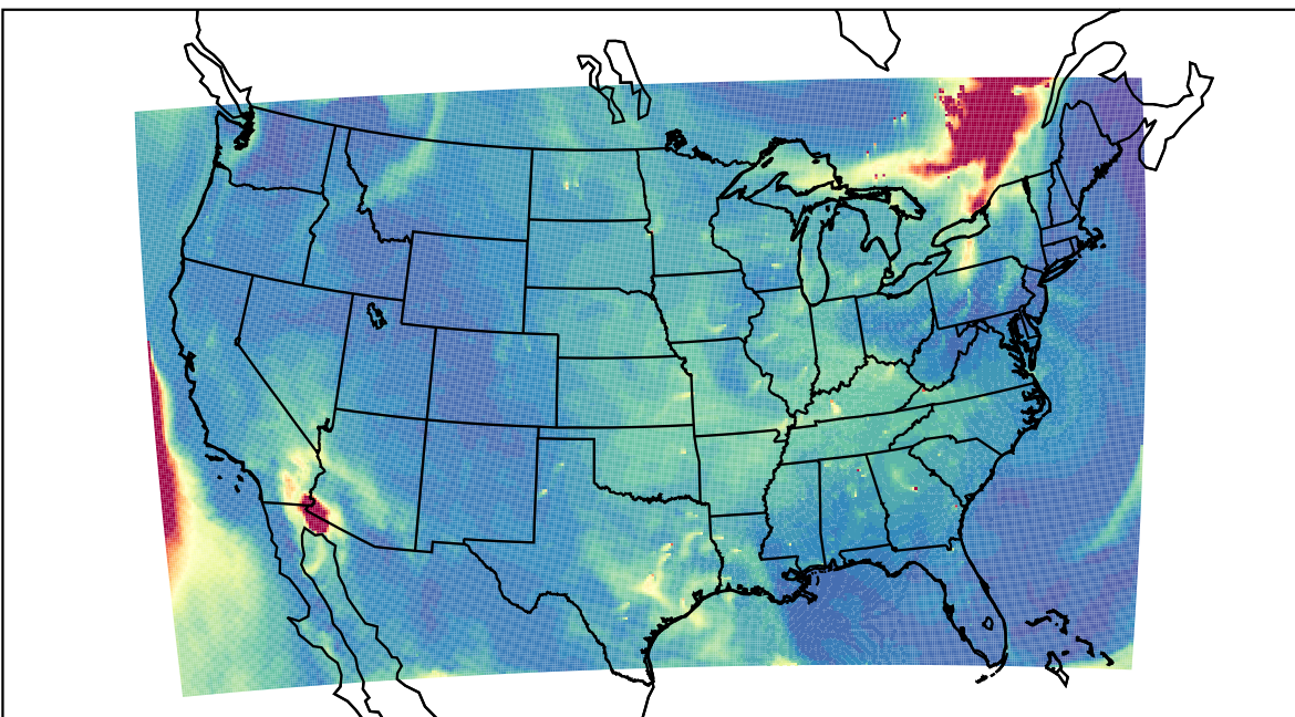
WRF 2023-06-05_18:00:00
