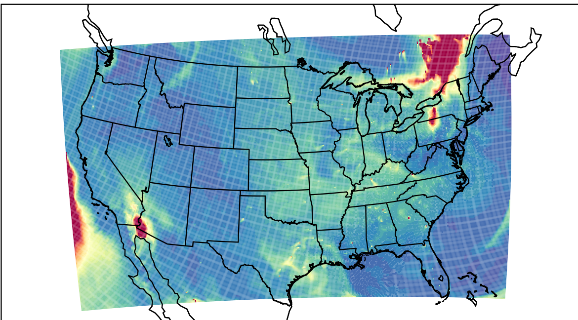
WRF 2023-06-05_20:00:00
