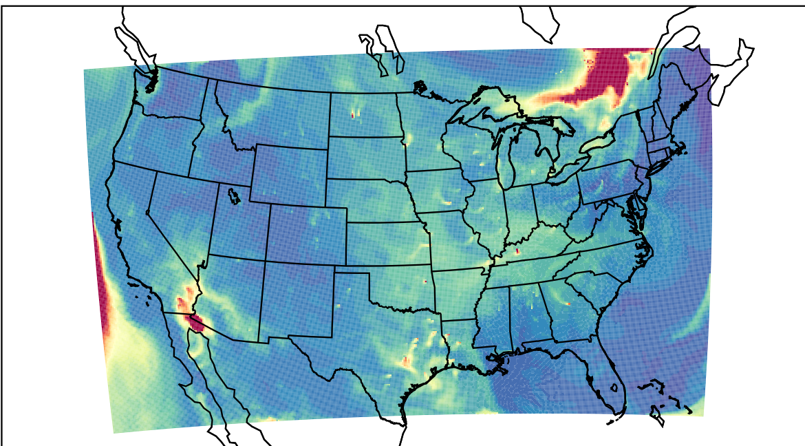
WRF 2023-06-05_16:00:00
