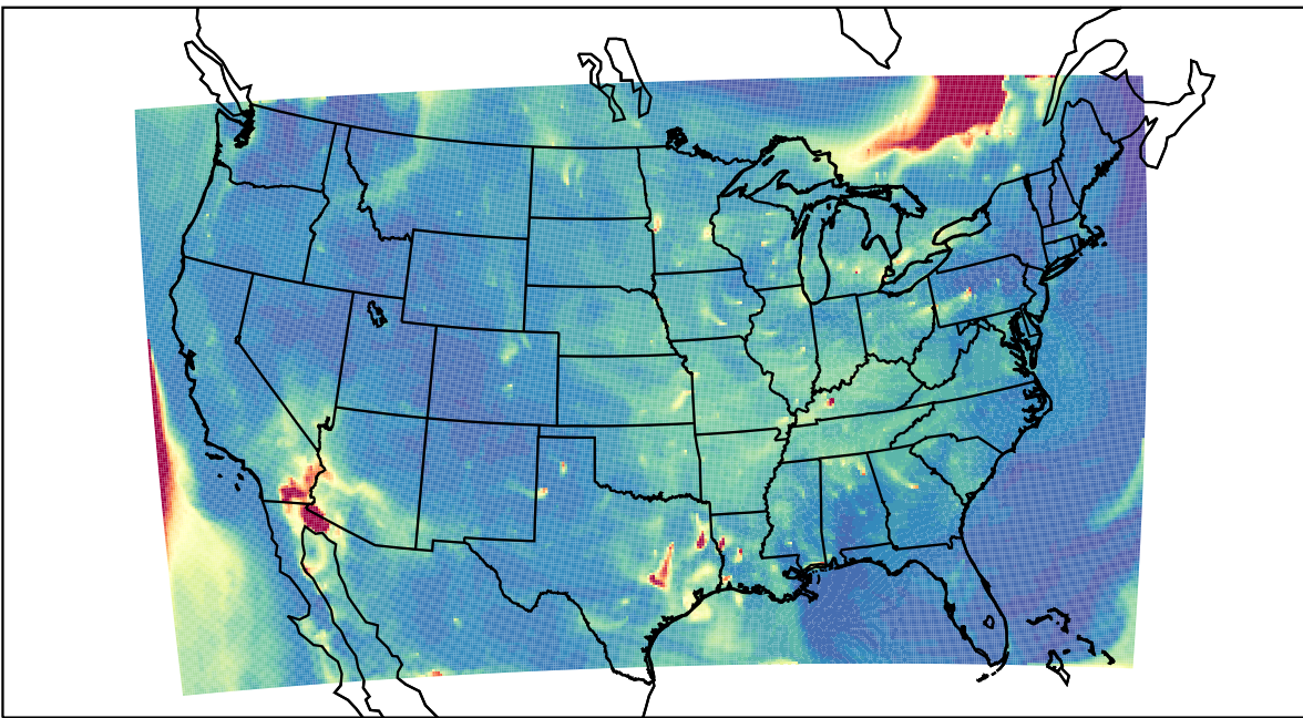
WRF 2023-06-05_13:00:00
