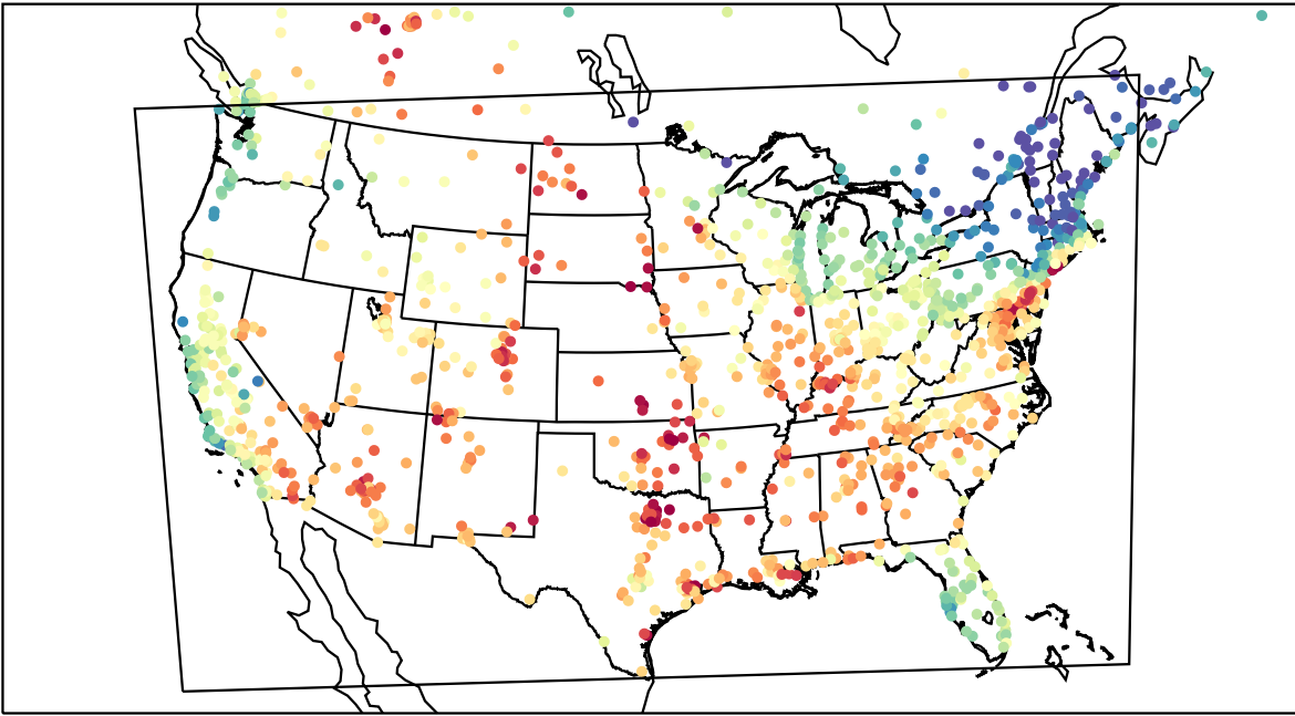
AirNOW (2023-06-08_20:00:00)
