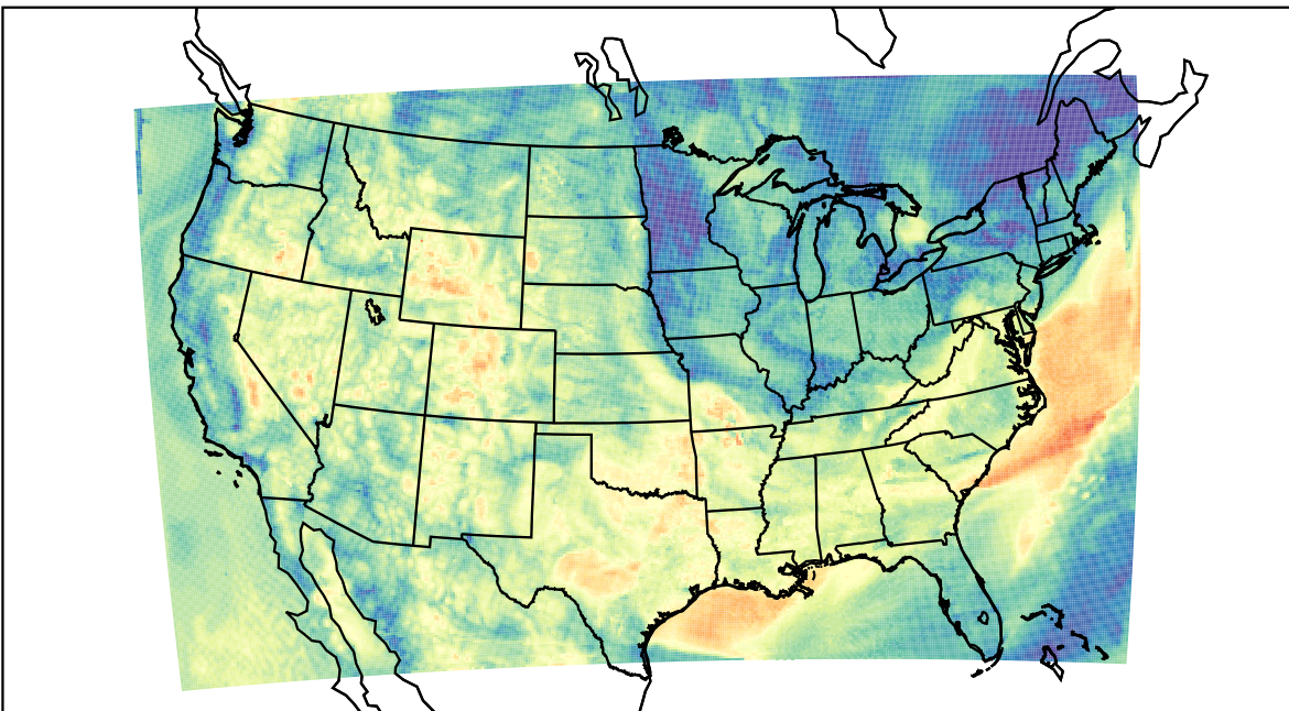
WRF (2023-06-08_14:00:00)
