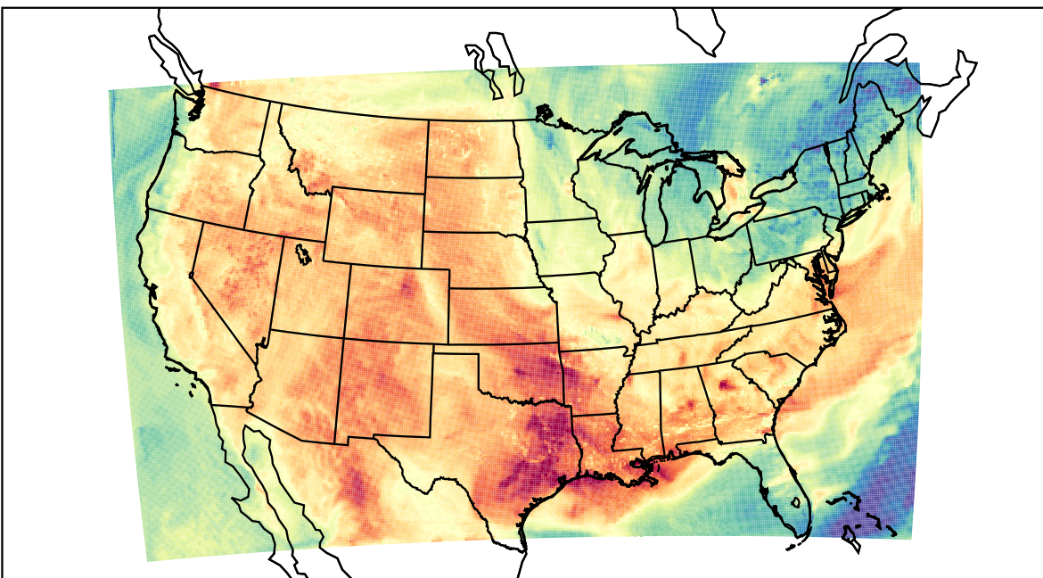
WRF (2023-06-08_20:00:00)
