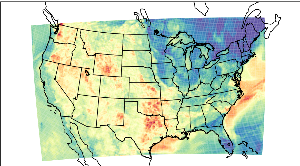
WRF (2023-06-08_04:00:00)
