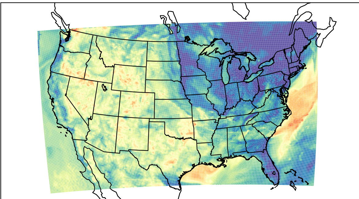
WRF (2023-06-08_11:00:00)
