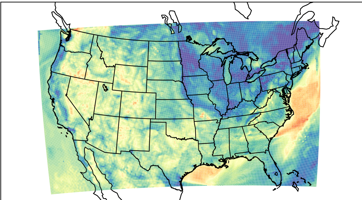
WRF (2023-06-08_13:00:00)
