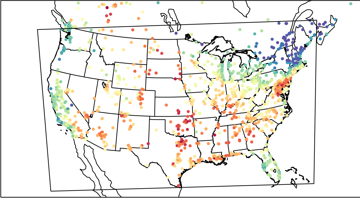
AirNOW (2023-06-08_18:00:00)
