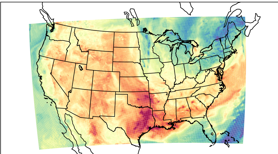
WRF (2023-06-08_18:00:00)
