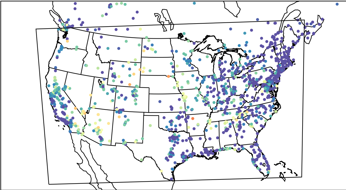
AirNOW (2023-06-08_10:00:00)
