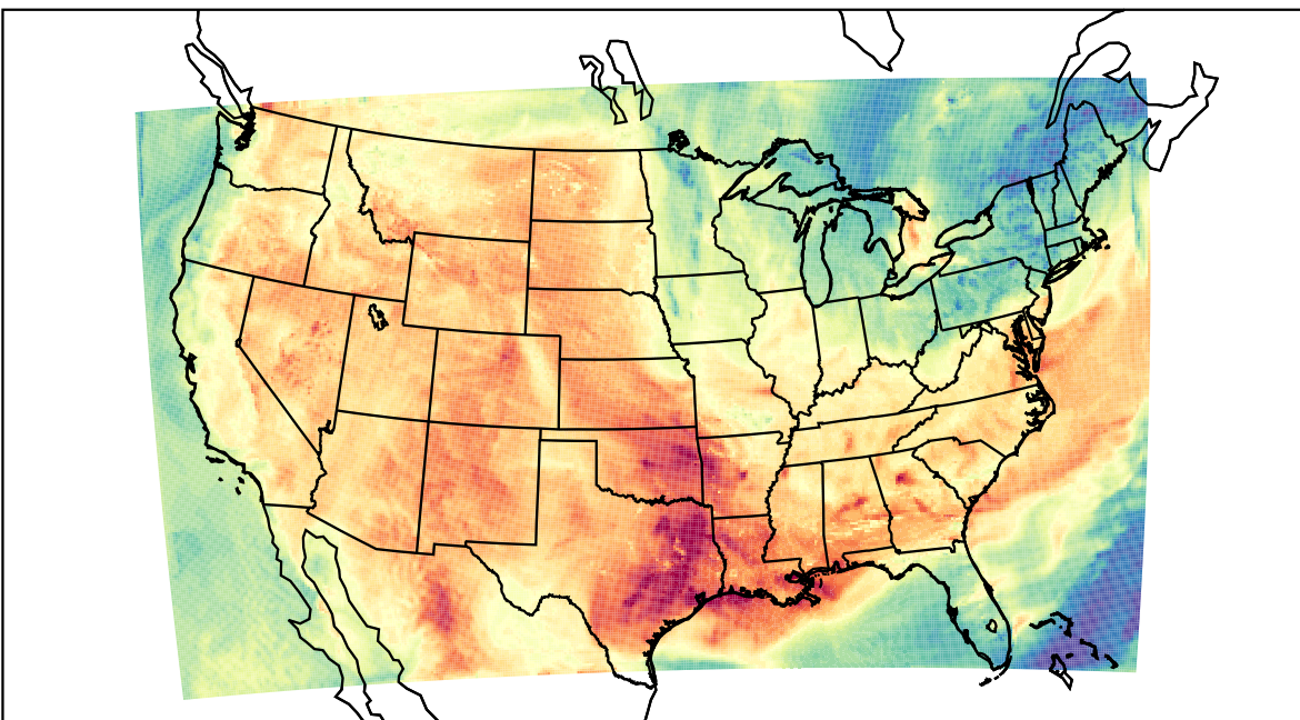
WRF (2023-06-08_19:00:00)
