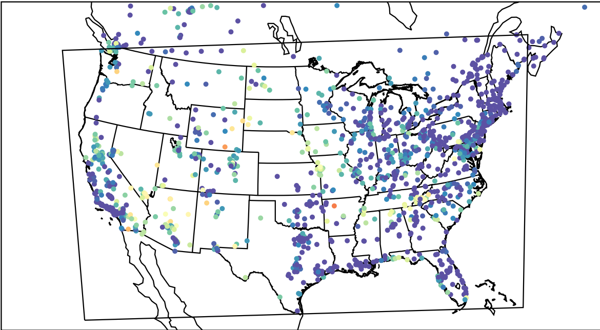
AirNOW (2023-06-08_11:00:00)
