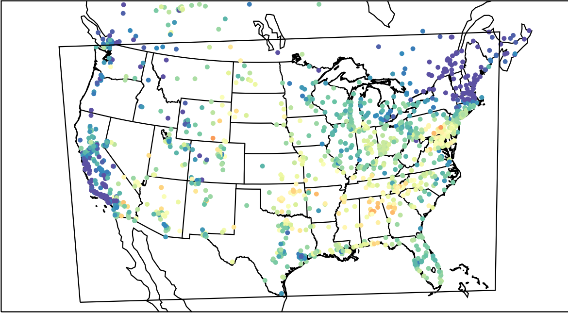
AirNOW (2023-06-08_14:00:00)
