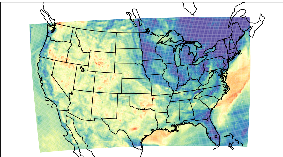
WRF (2023-06-08_10:00:00)
