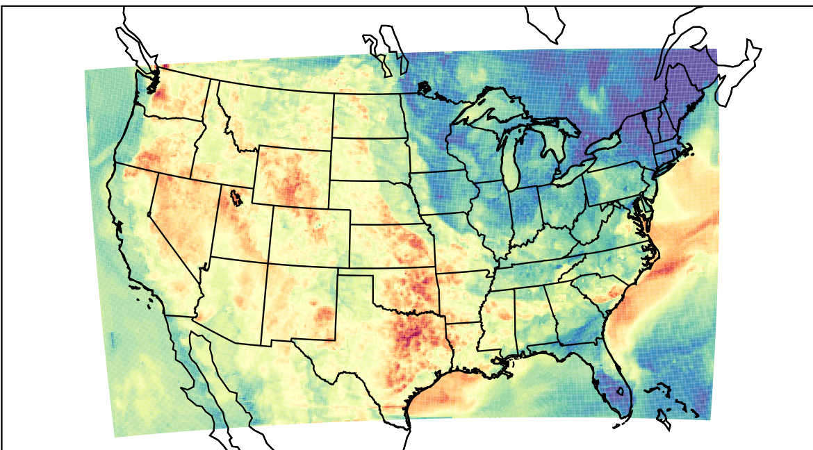
WRF (2023-06-08_03:00:00)
