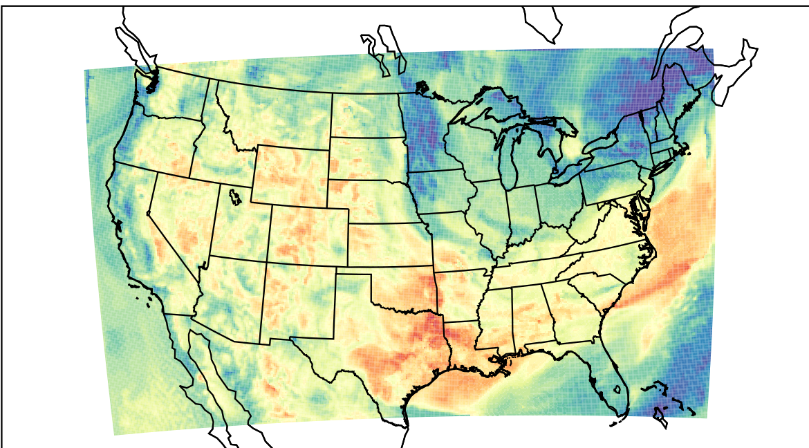
WRF (2023-06-08_15:00:00)
