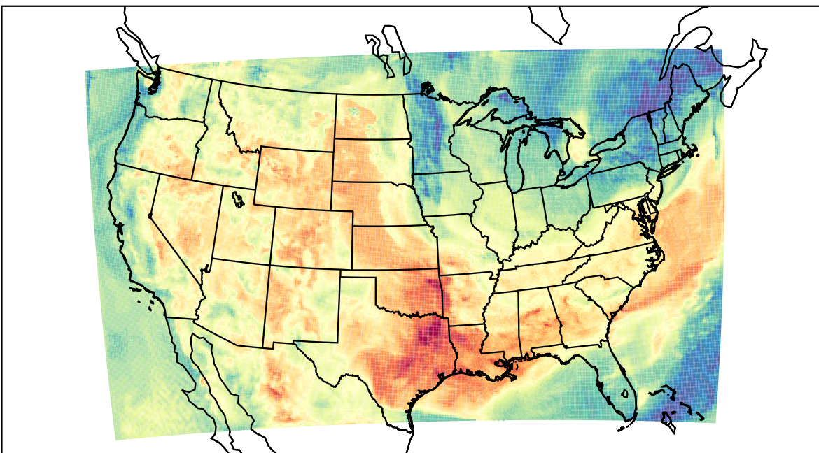
WRF (2023-06-08_16:00:00)
