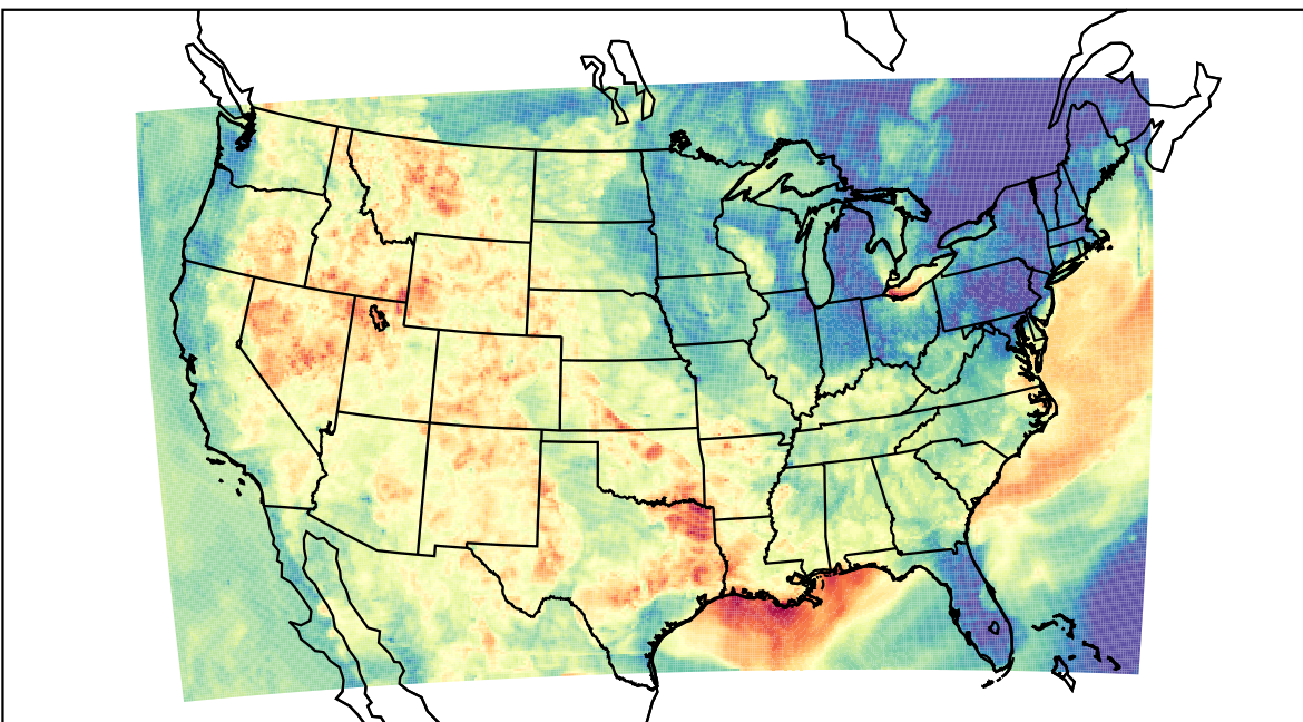
WRF (2023-06-09_04:00:00)
