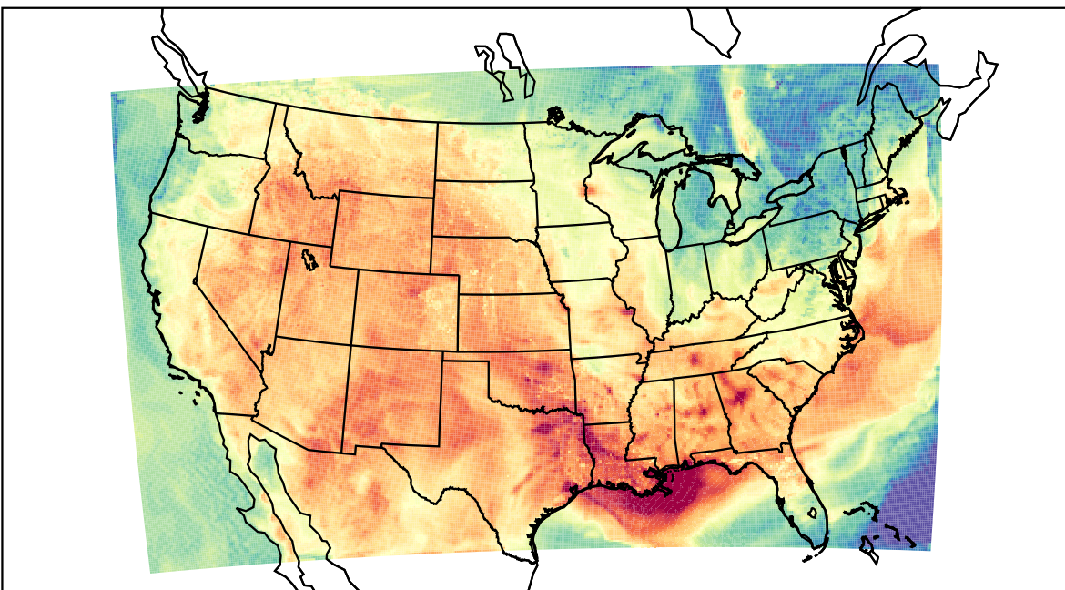
WRF (2023-06-09_20:00:00)
