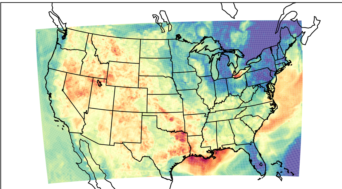
WRF (2023-06-09_03:00:00)
