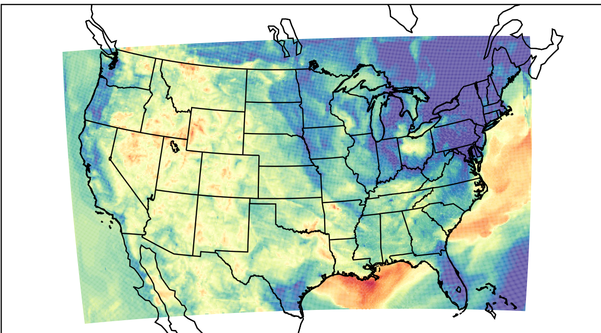
WRF (2023-06-09_10:00:00)
