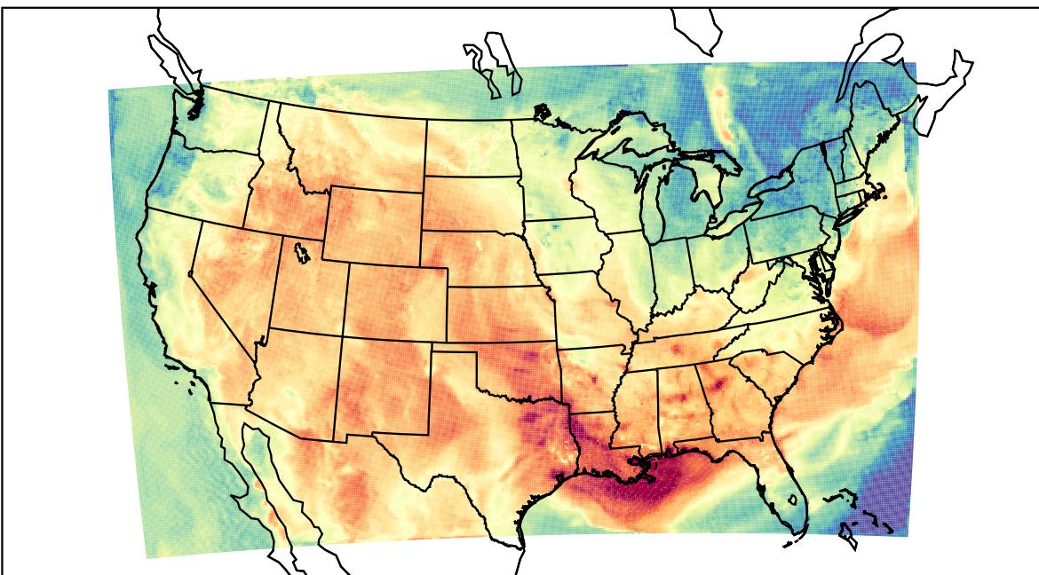
WRF (2023-06-09_18:00:00)
