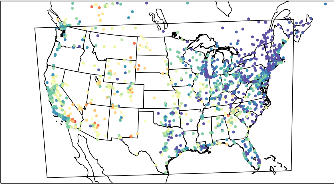
AirNOW (2023-06-09_04:00:00)
