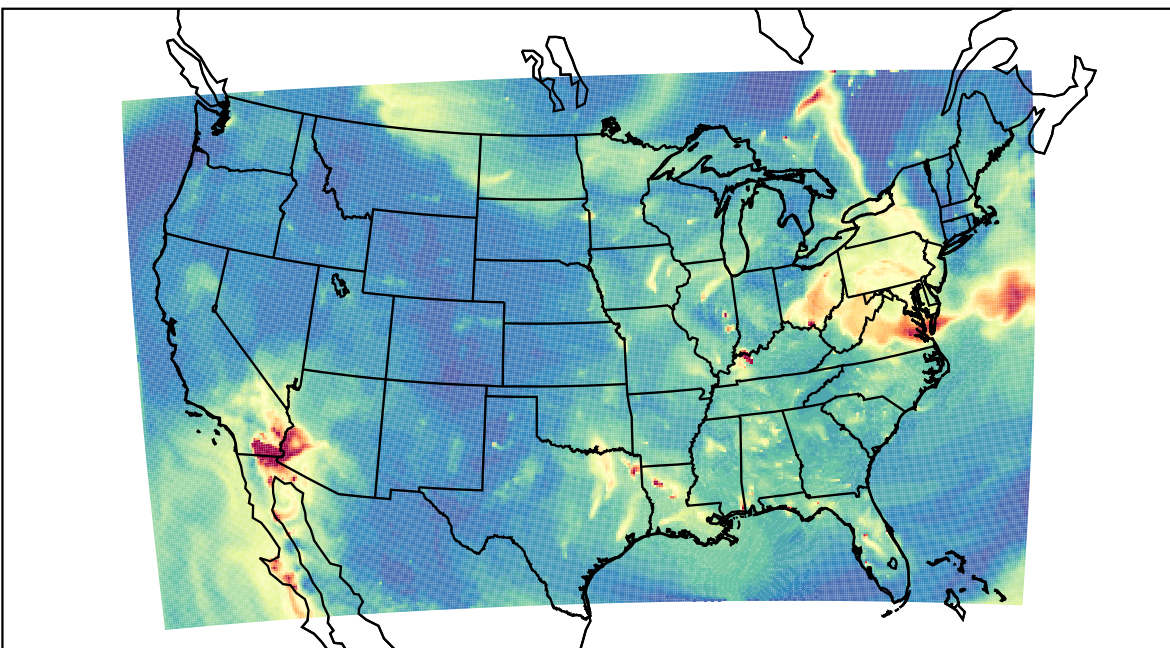
WRF 2023-06-10_11:00:00
