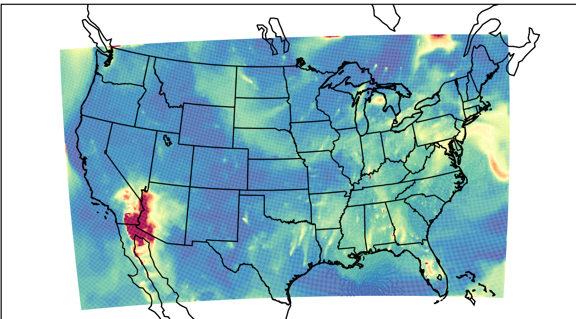
WRF 2023-06-11_11:00:00
