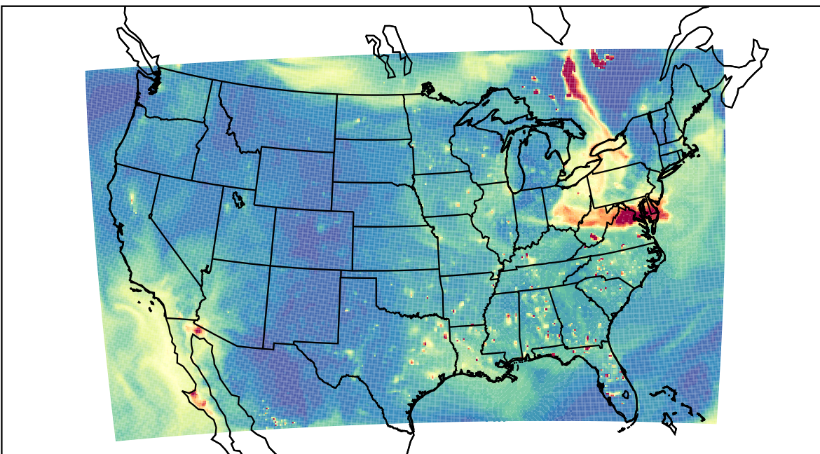
WRF 2023-06-10_01:00:00
