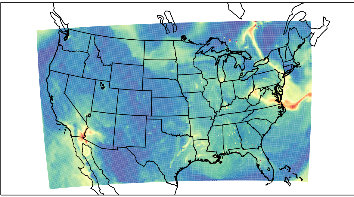
WRF 2023-06-10_17:00:00
