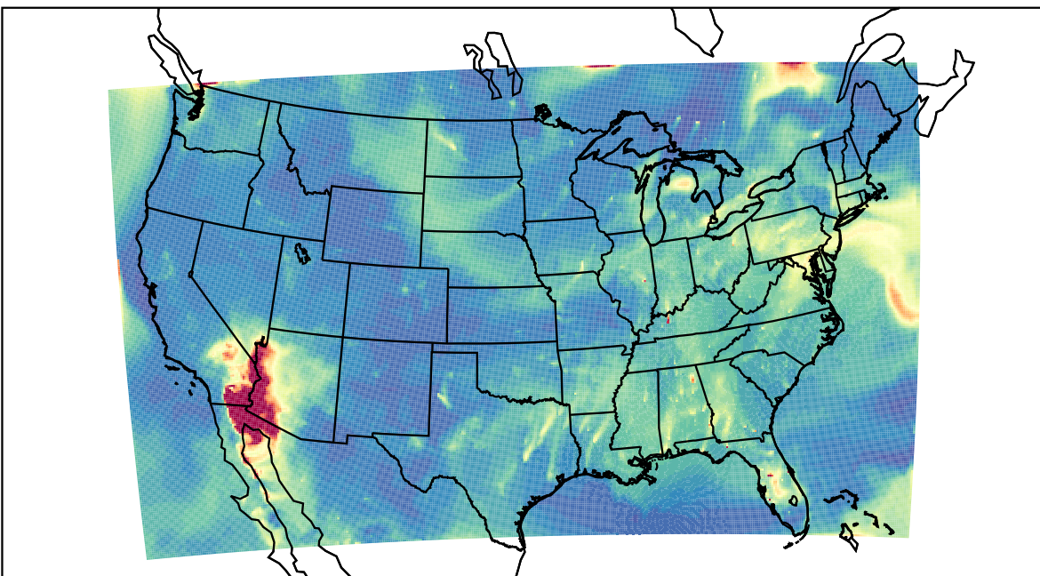
WRF 2023-06-11_12:00:00
