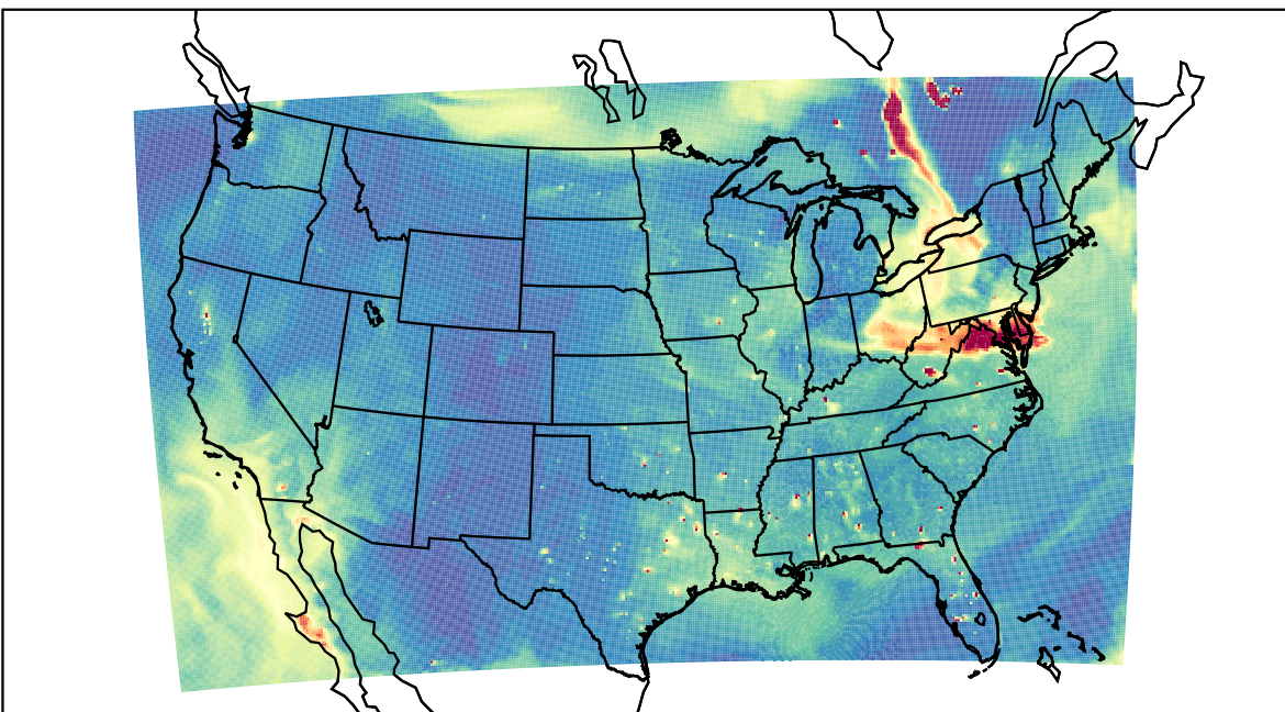
WRF 2023-06-10_00:00:00
