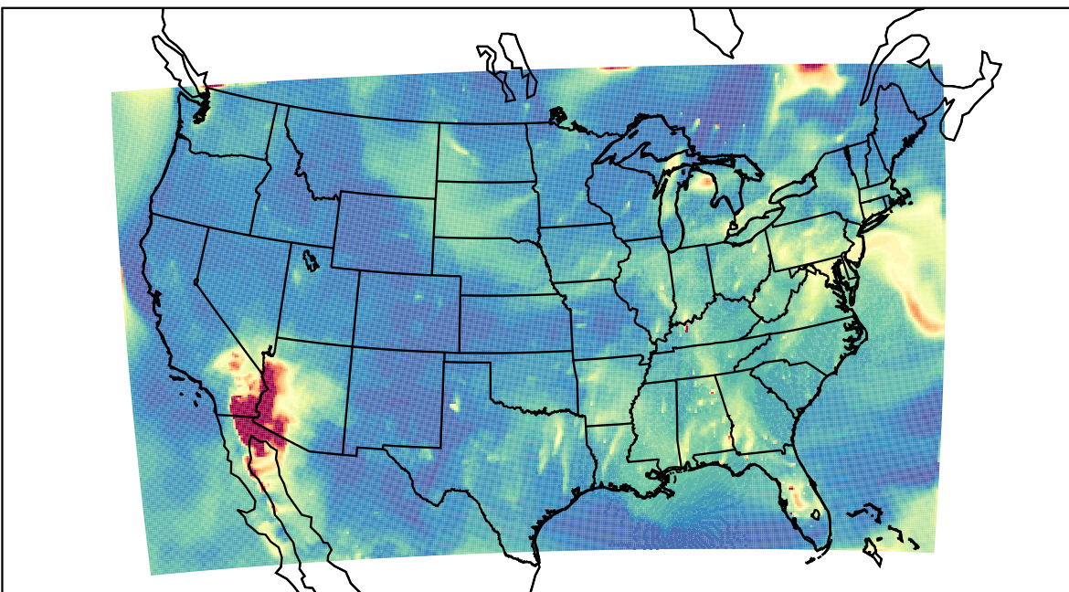
WRF 2023-06-11_10:00:00
