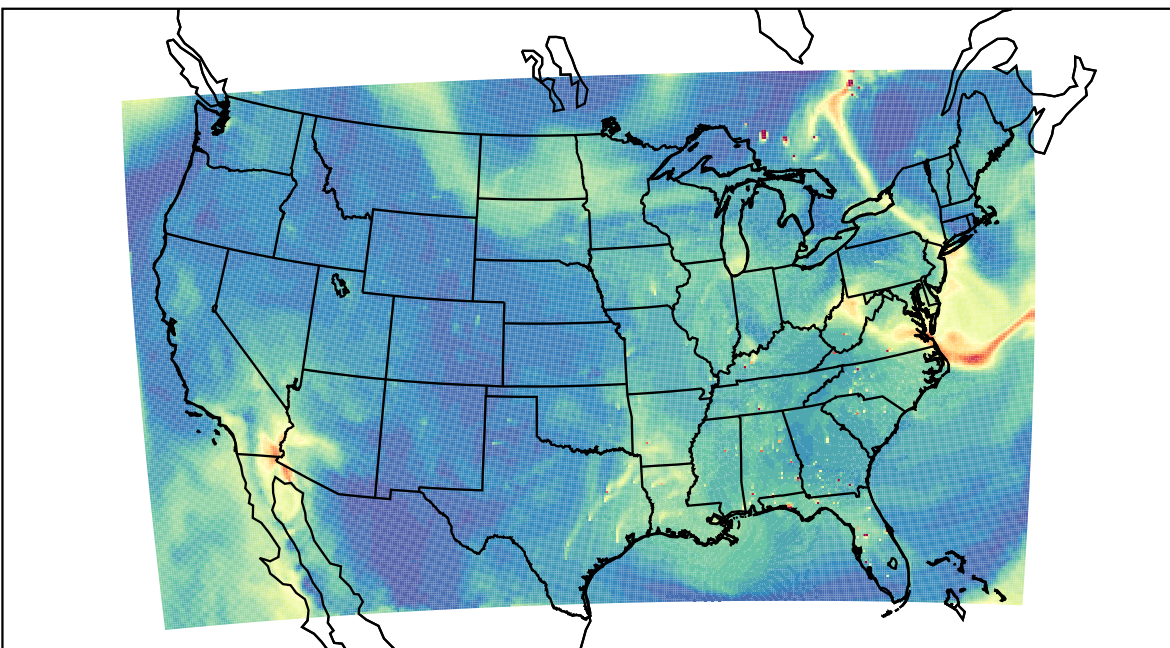
WRF 2023-06-10_18:00:00
