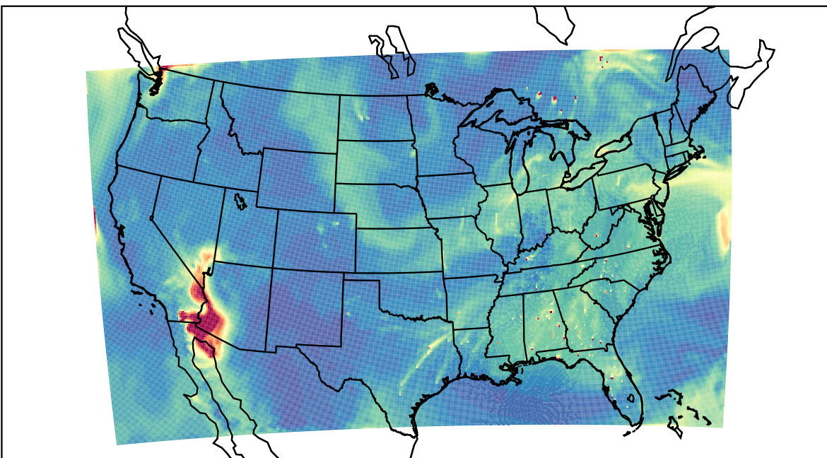
WRF 2023-06-11_18:00:00
