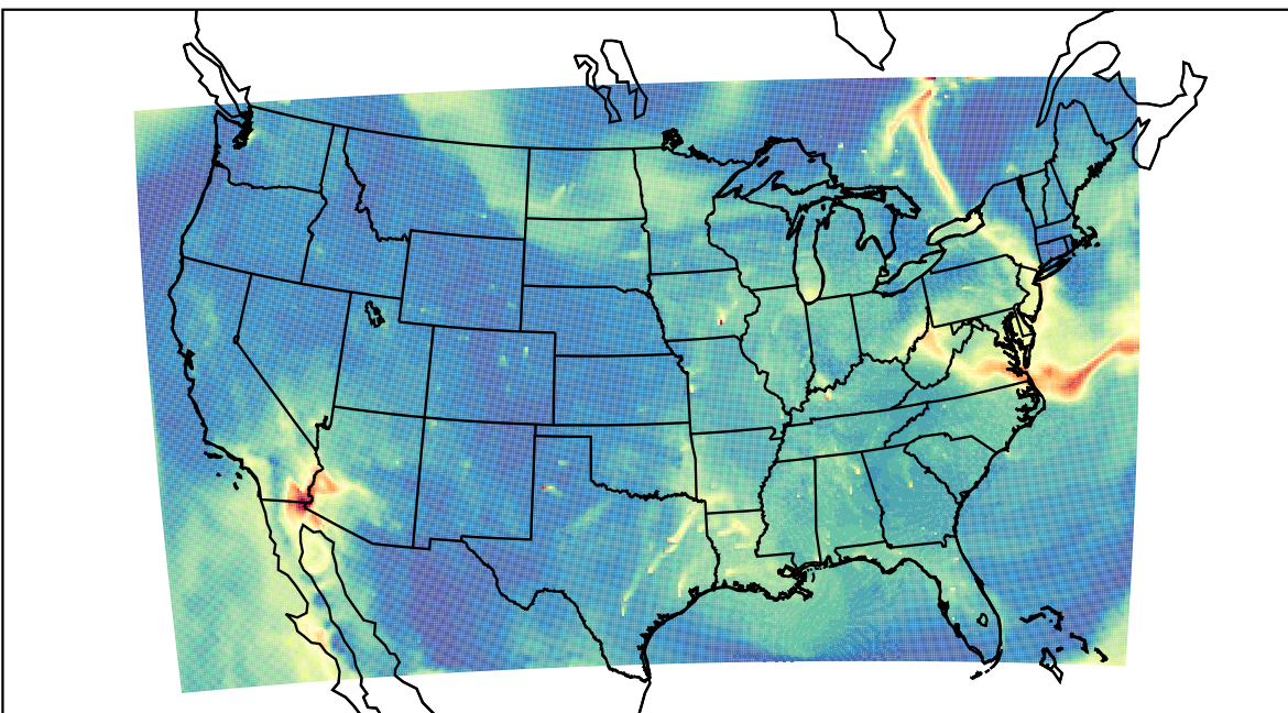
WRF 2023-06-10_16:00:00
