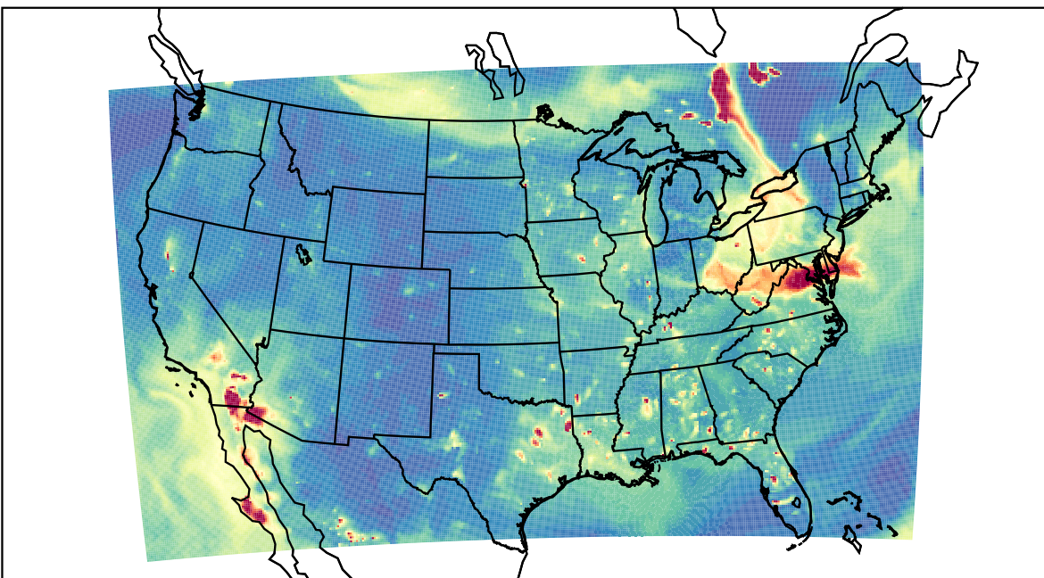
WRF 2023-06-10_03:00:00
