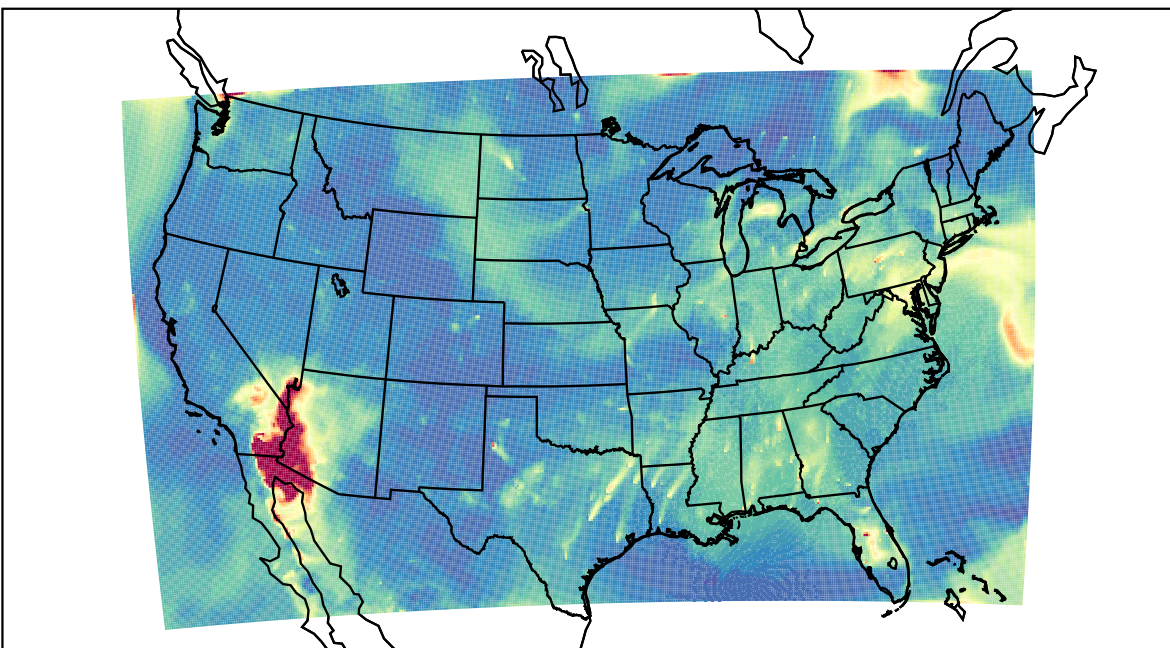
WRF 2023-06-11_13:00:00
