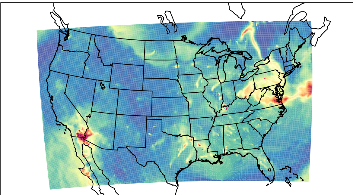
WRF 2023-06-10_13:00:00
