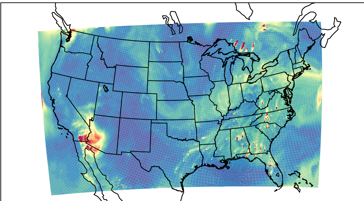
WRF 2023-06-11_23:00:00
