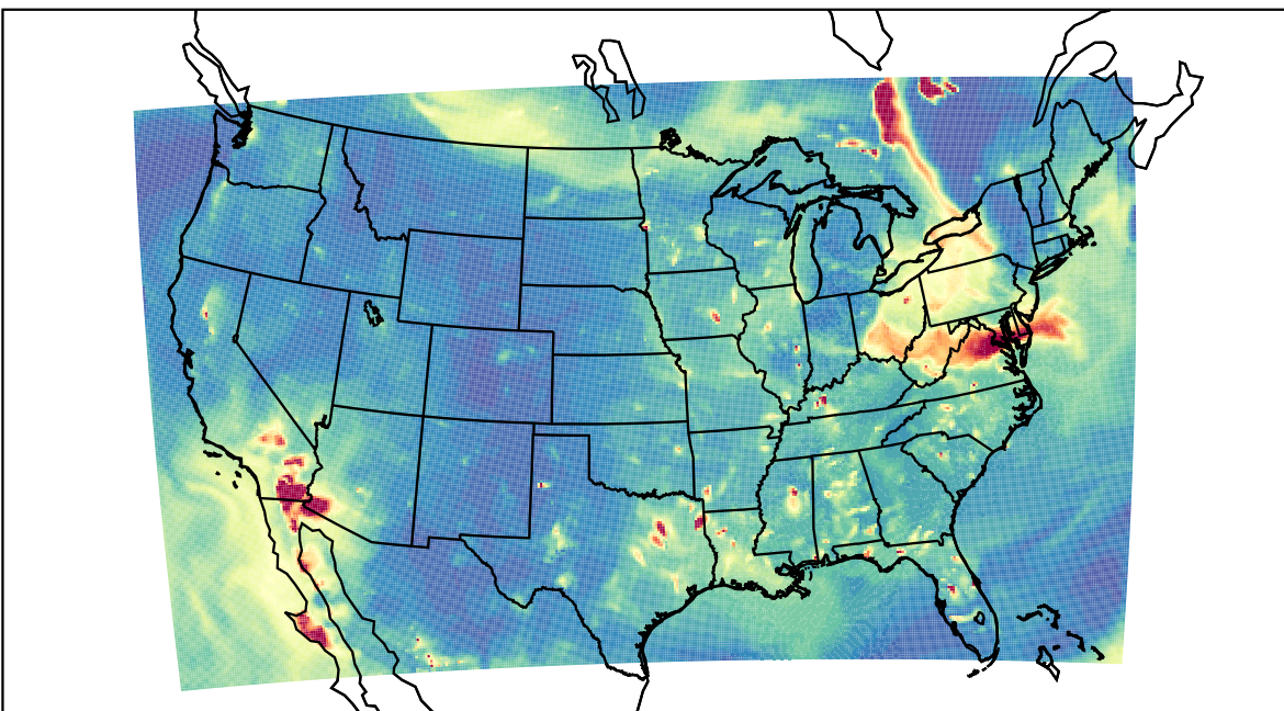
WRF 2023-06-10_04:00:00
