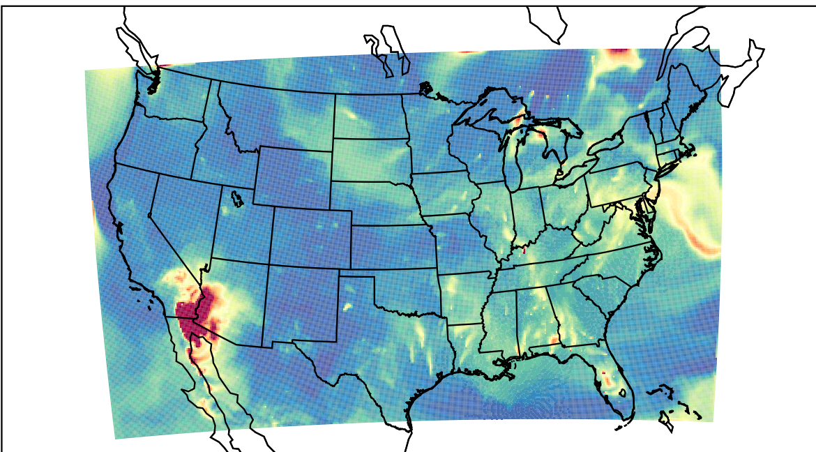
WRF 2023-06-11_08:00:00
