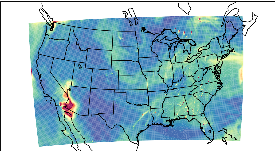
WRF 2023-06-11_19:00:00
