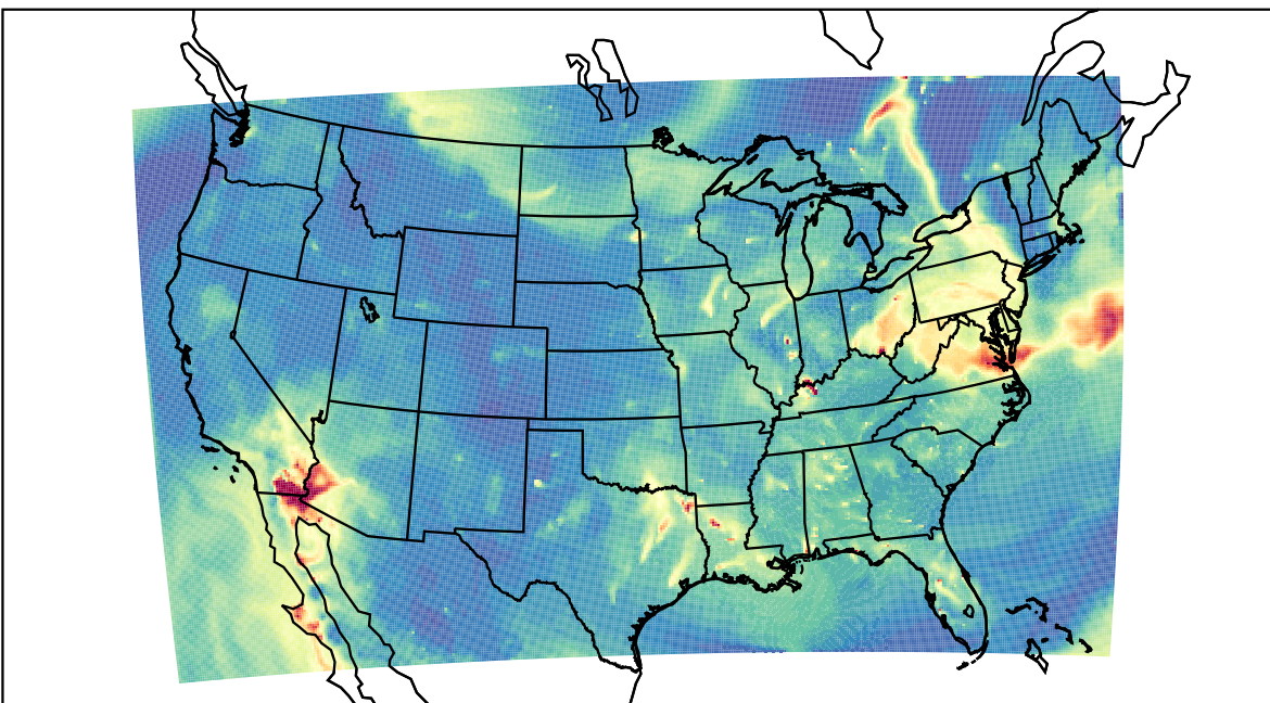
WRF 2023-06-10_12:00:00
