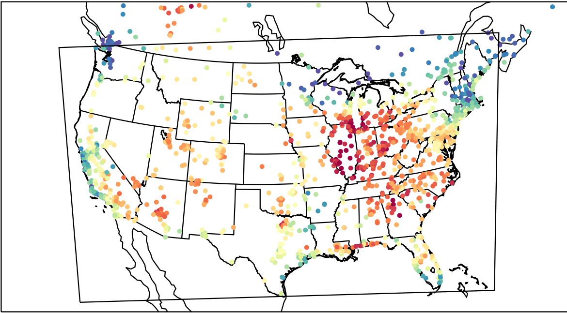
AirNOW (2023-06-10_22:00:00)
