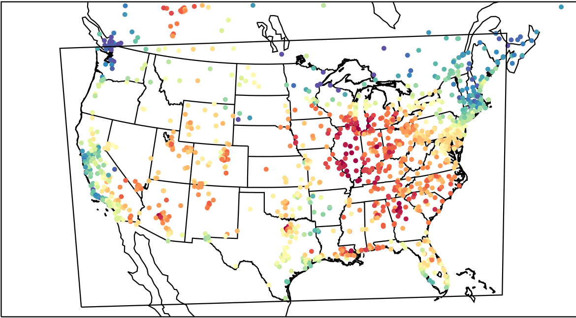
AirNOW (2023-06-10_20:00:00)
