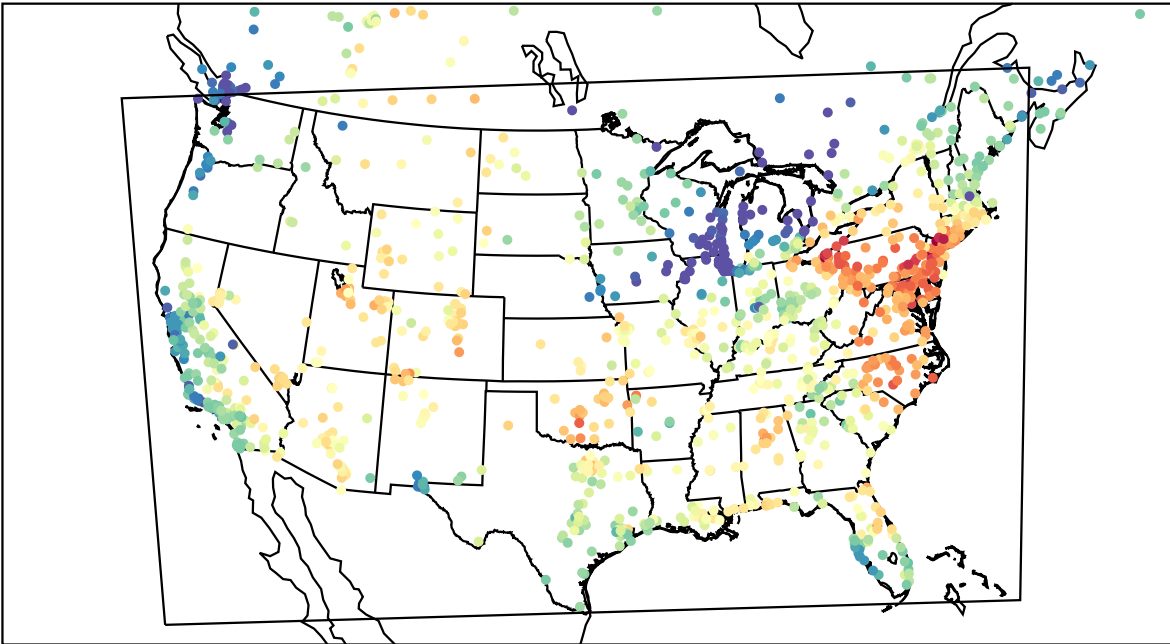
AirNOW (2023-06-11_18:00:00)
