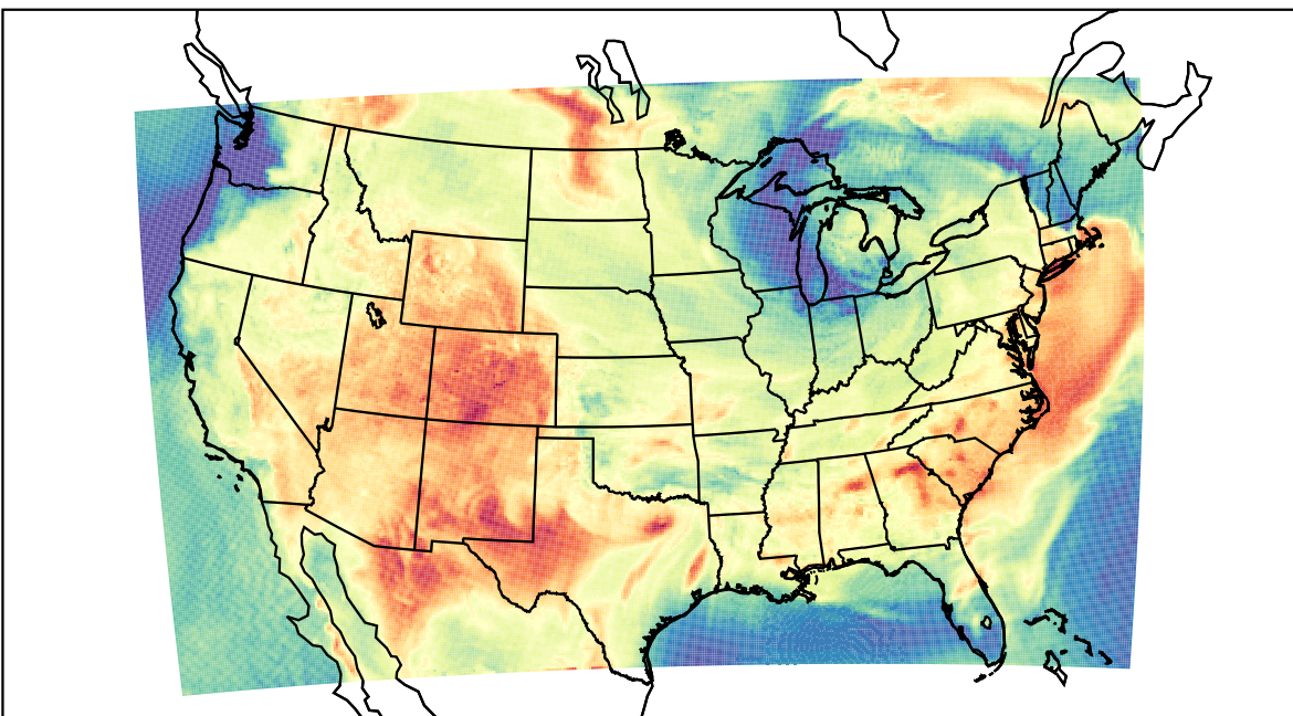
WRF (2023-06-13_18:00:00)
