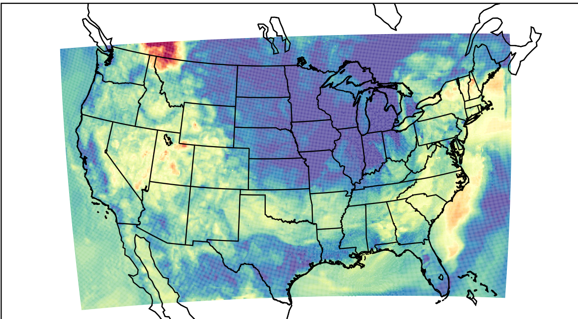
WRF (2023-06-12_13:00:00)
