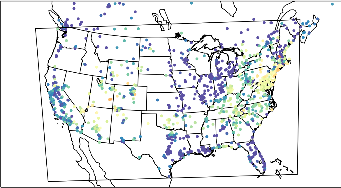
AirNOW (2023-06-12_10:00:00)
