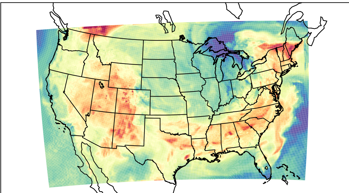
WRF (2023-06-12_18:00:00)
