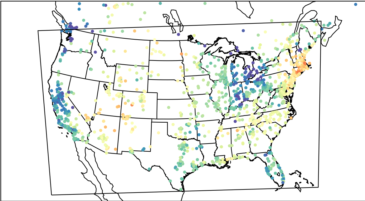
AirNOW (2023-06-12_16:00:00)
