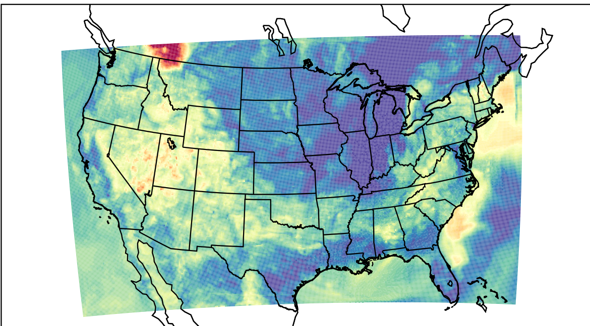
WRF (2023-06-12_10:00:00)
