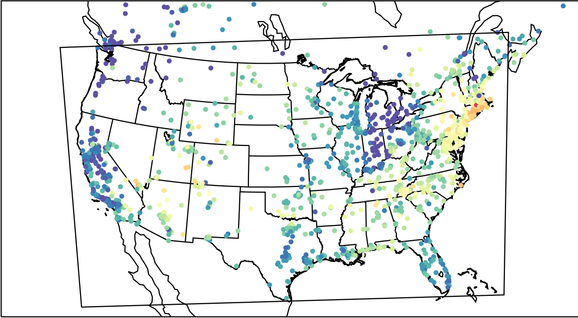
AirNOW (2023-06-12_14:00:00)
