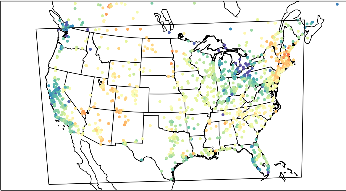
AirNOW (2023-06-12_18:00:00)
