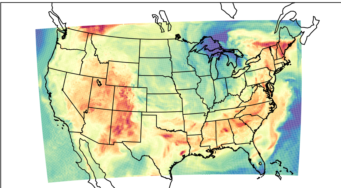
WRF (2023-06-12_19:00:00)
