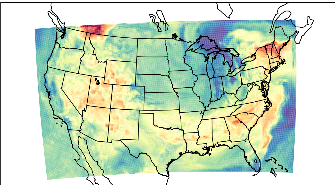
WRF (2023-06-12_16:00:00)
