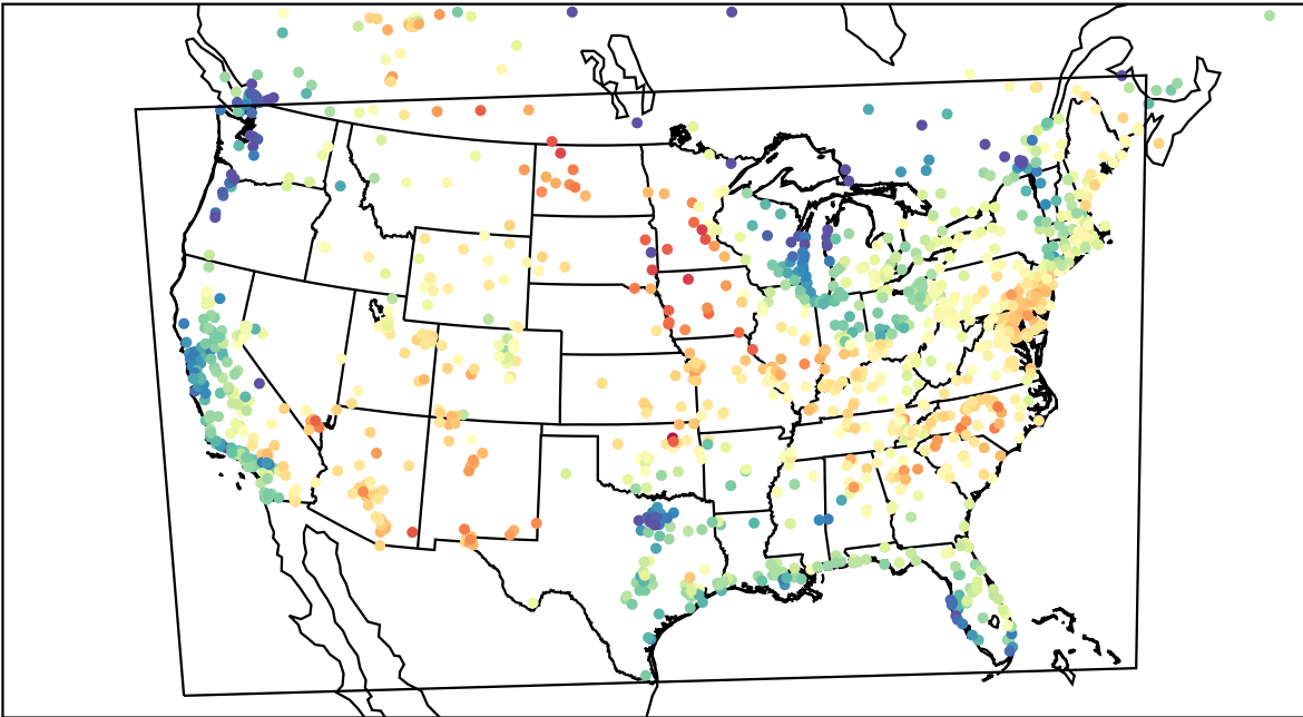
AirNOW (2023-06-13_18:00:00)
