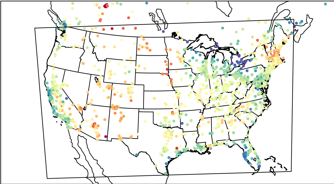
AirNOW (2023-06-12_23:00:00)
