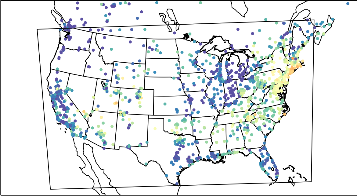
AirNOW (2023-06-12_13:00:00)
