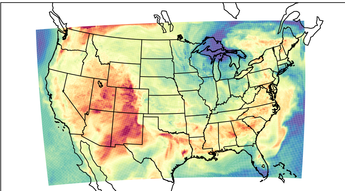
WRF (2023-06-12_23:00:00)
