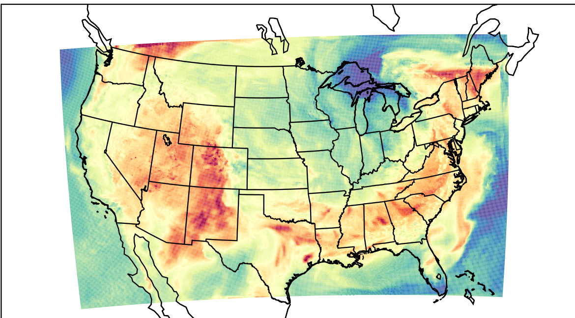
WRF (2023-06-12_20:00:00)
