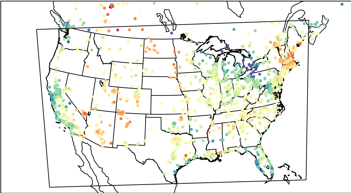
AirNOW (2023-06-12_20:00:00)
