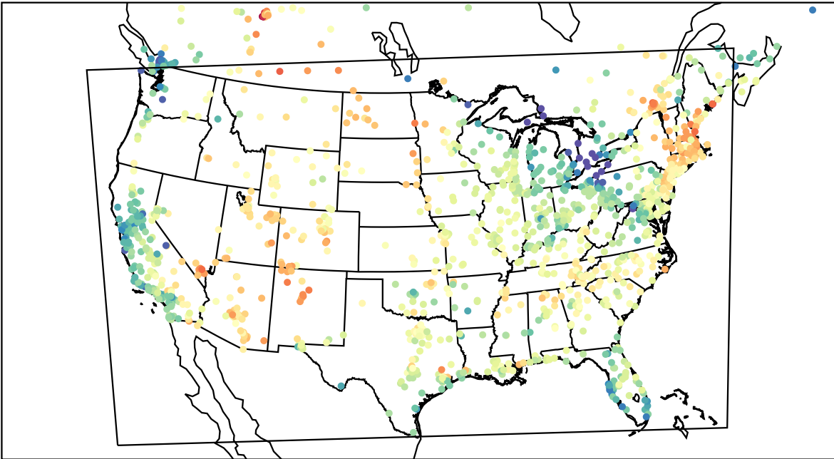
AirNOW (2023-06-12_19:00:00)
