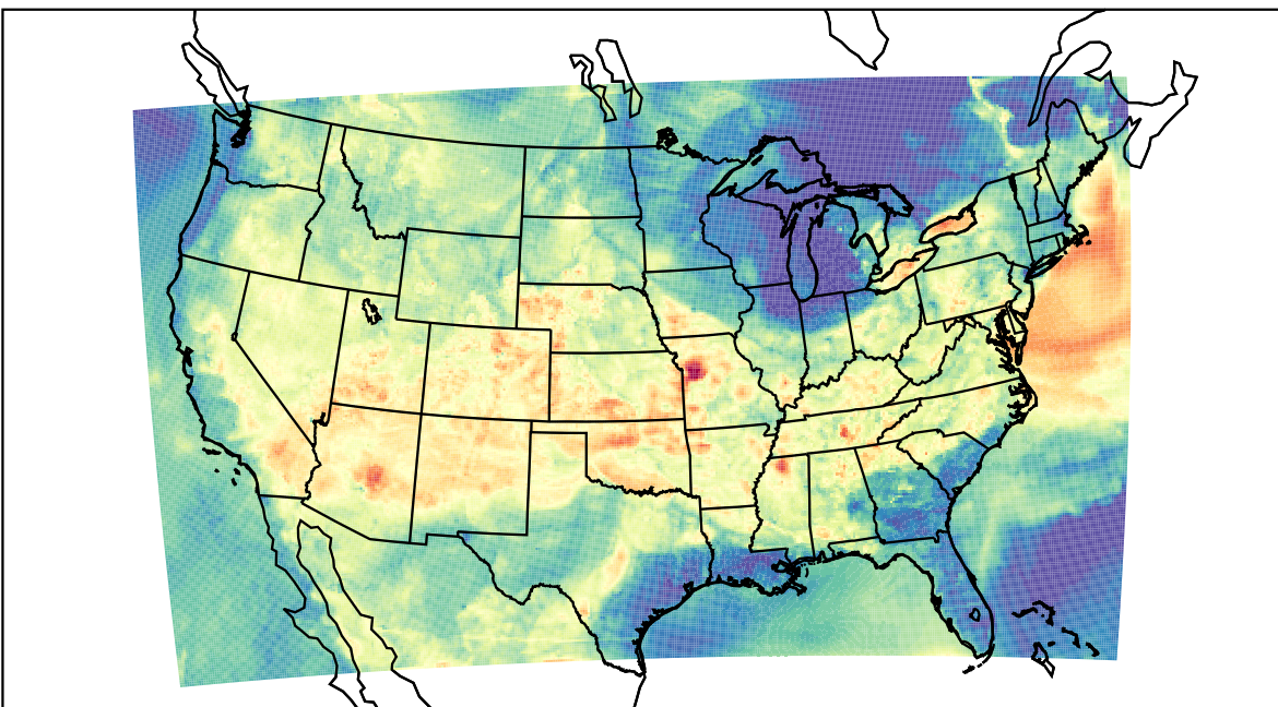
WRF (2023-06-16_03:00:00)
