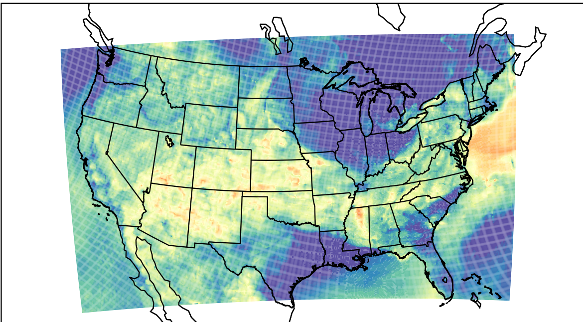
WRF (2023-06-16_10:00:00)
