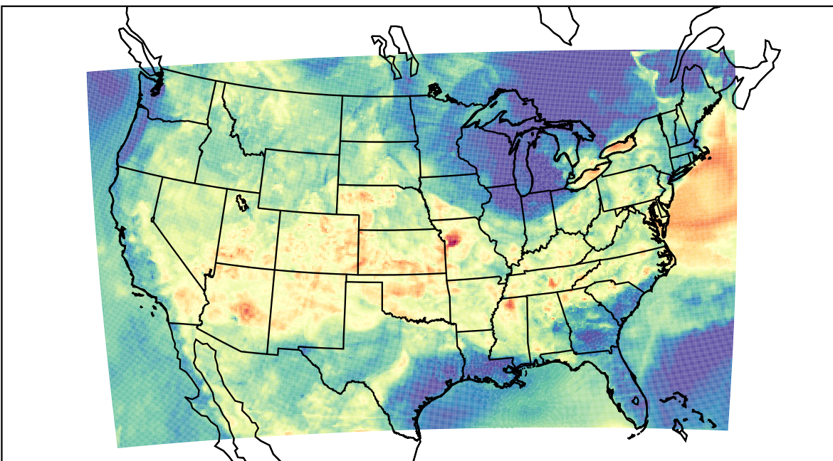
WRF (2023-06-16_04:00:00)
