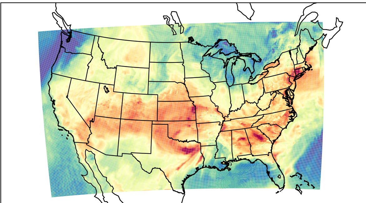
WRF (2023-06-16_20:00:00)
