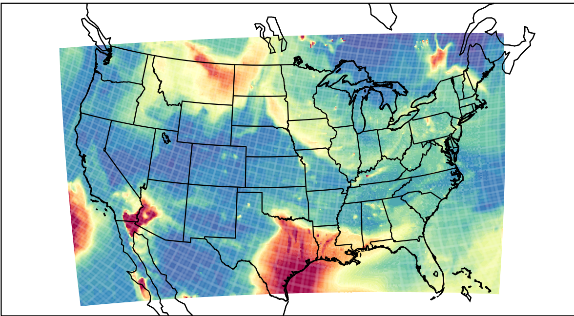
WRF 2023-06-16_10:00:00
