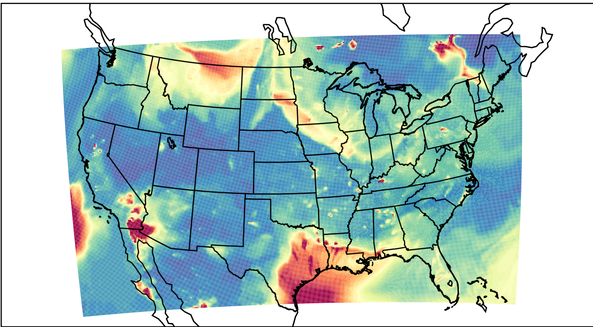
WRF 2023-06-16_04:00:00
