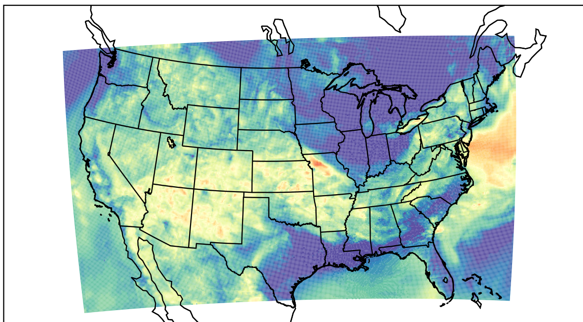
WRF (2023-06-16_10:00:00)
