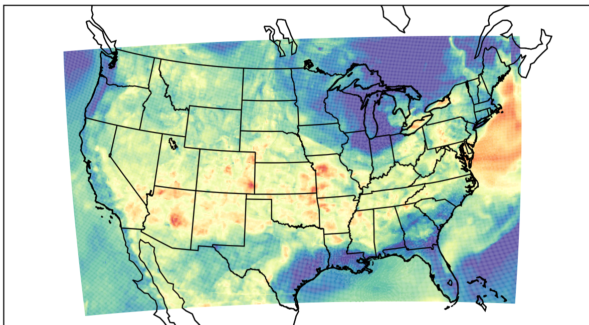
WRF (2023-06-16_04:00:00)
