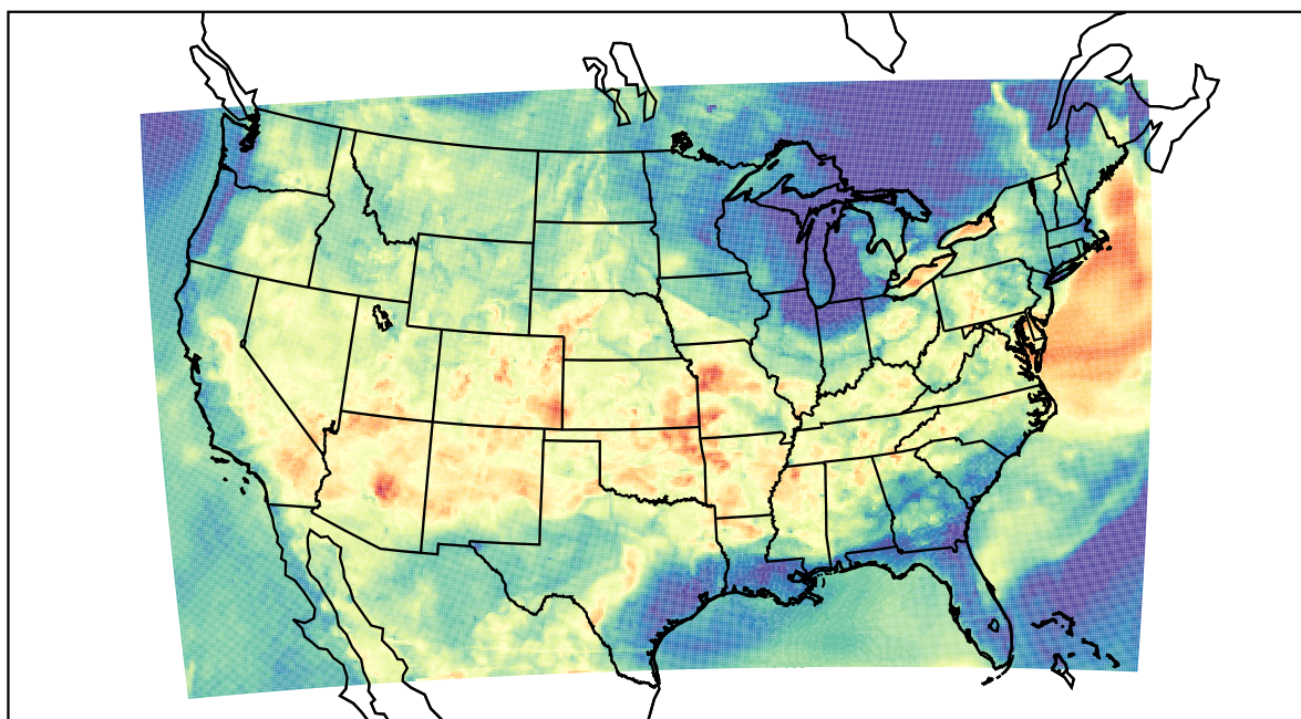
WRF (2023-06-16_03:00:00)
