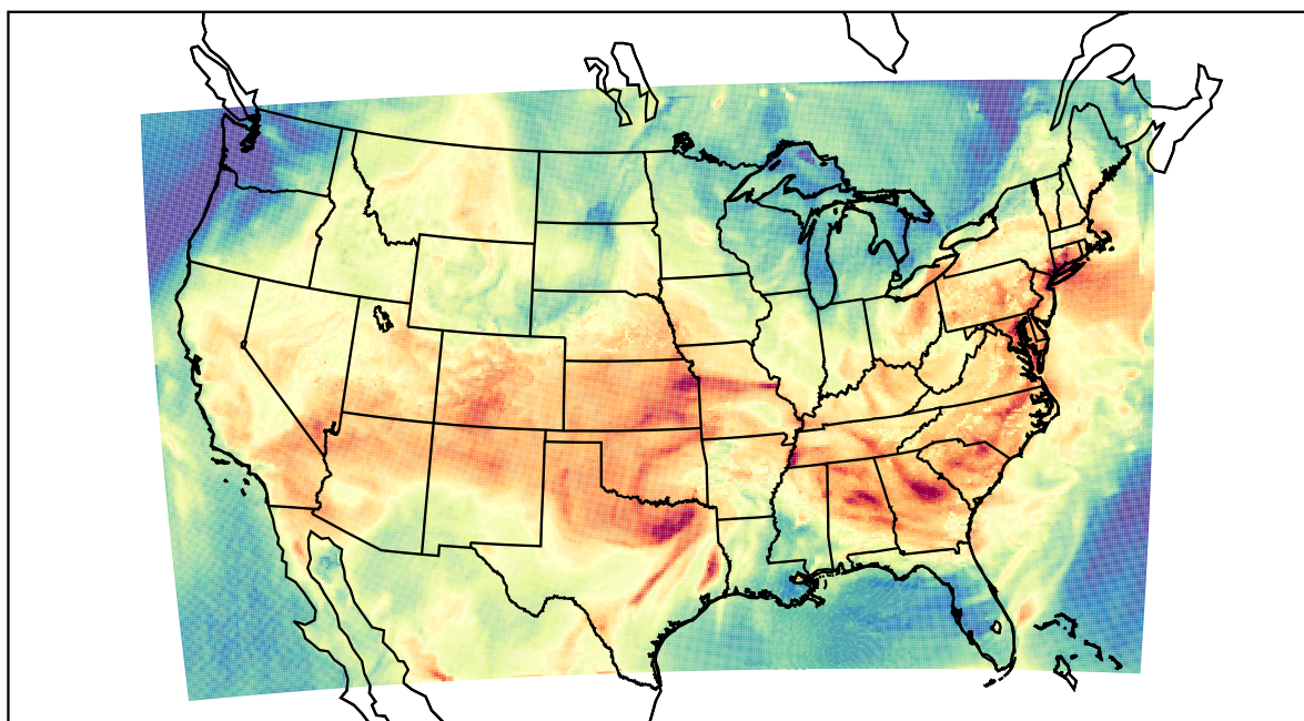
WRF (2023-06-16_20:00:00)
