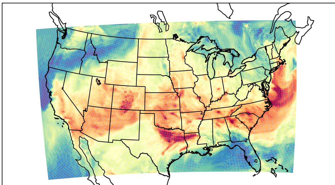
WRF (2023-06-17_20:00:00)
