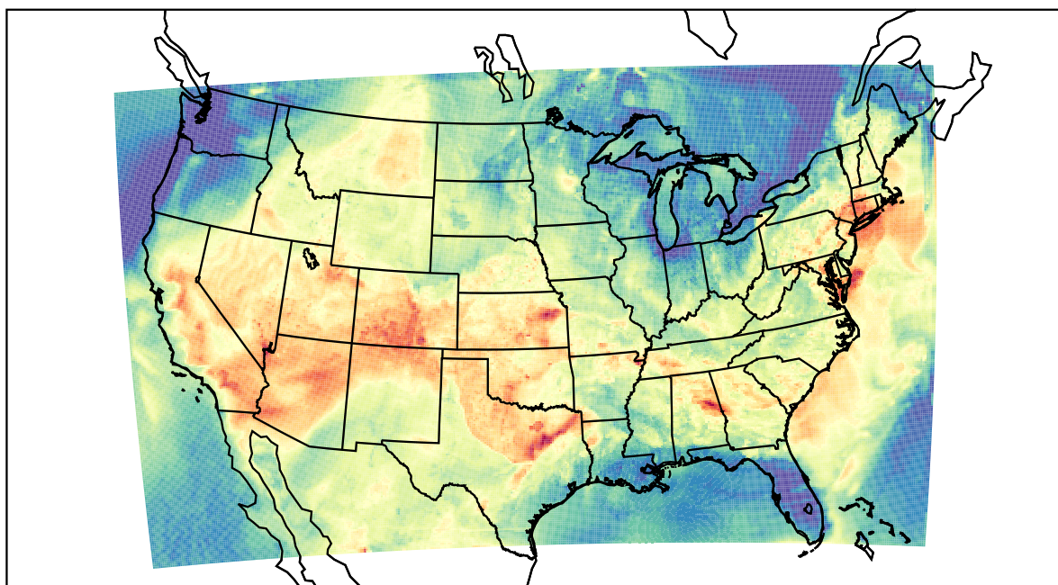
WRF (2023-06-17_01:00:00)
