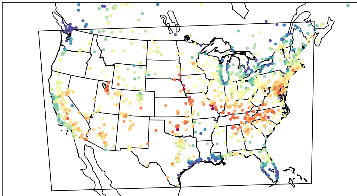
AirNOW (2023-06-16_20:00:00)
