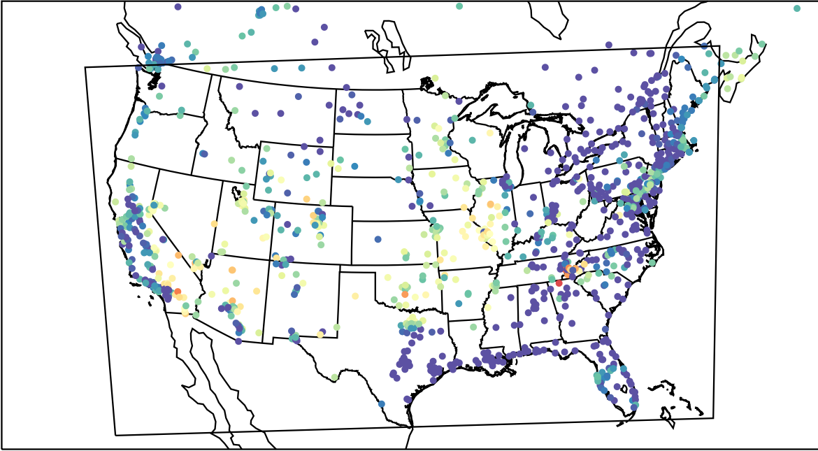
AirNOW (2023-06-18_10:00:00)
