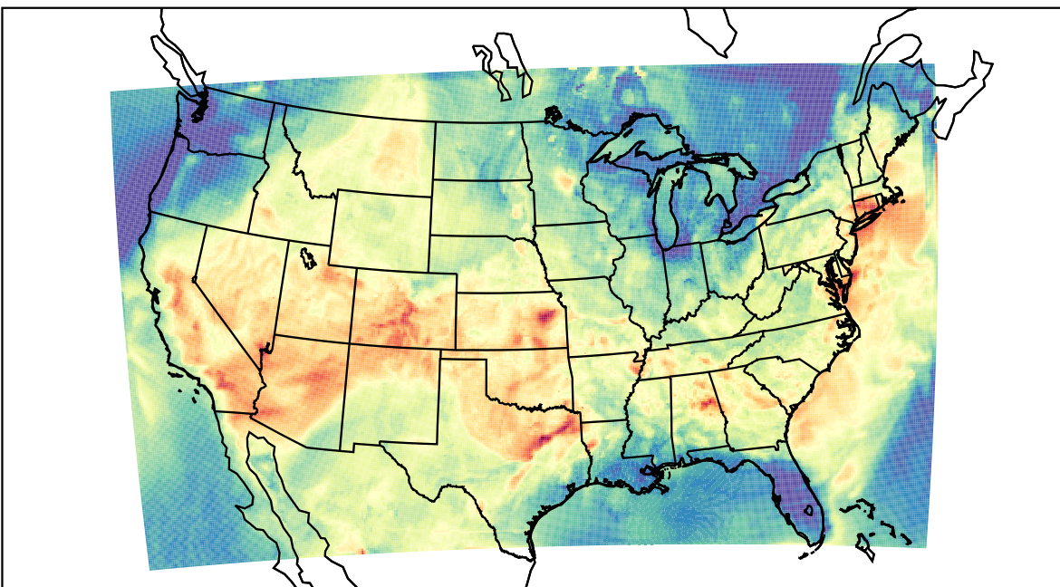
WRF (2023-06-17_01:00:00)
