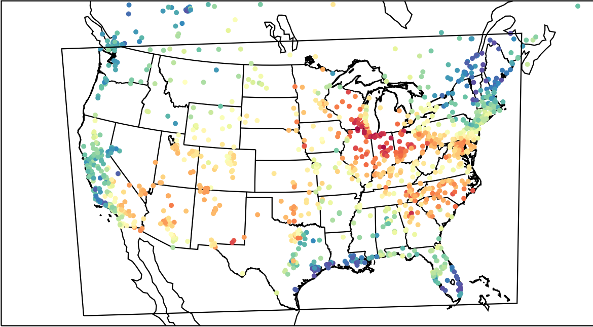
AirNOW (2023-06-18_18:00:00)
