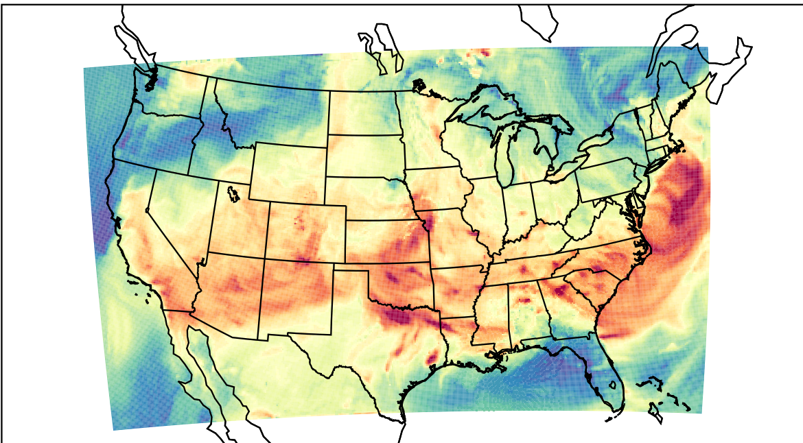
WRF (2023-06-17_20:00:00)
