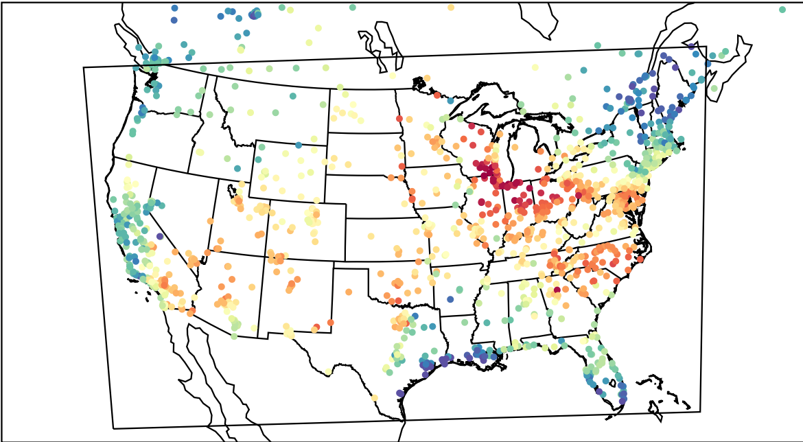
AirNOW (2023-06-18_20:00:00)
