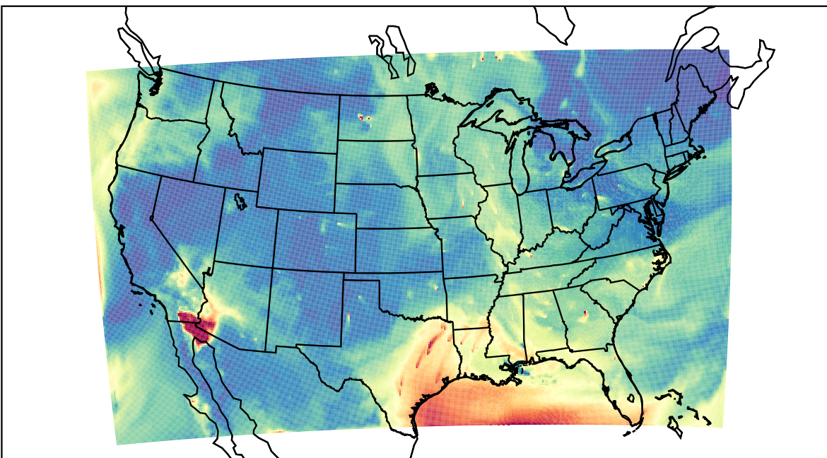
WRF 2023-06-18_15:00:00
