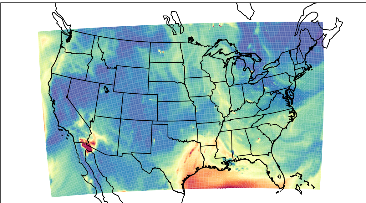
WRF 2023-06-18_16:00:00
