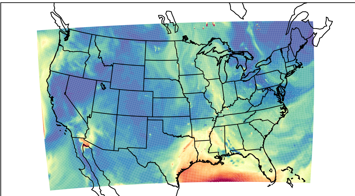
WRF 2023-06-18_18:00:00
