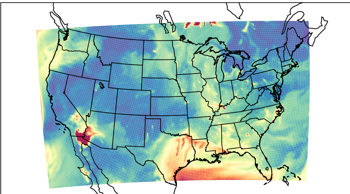
WRF 2023-06-18_11:00:00
