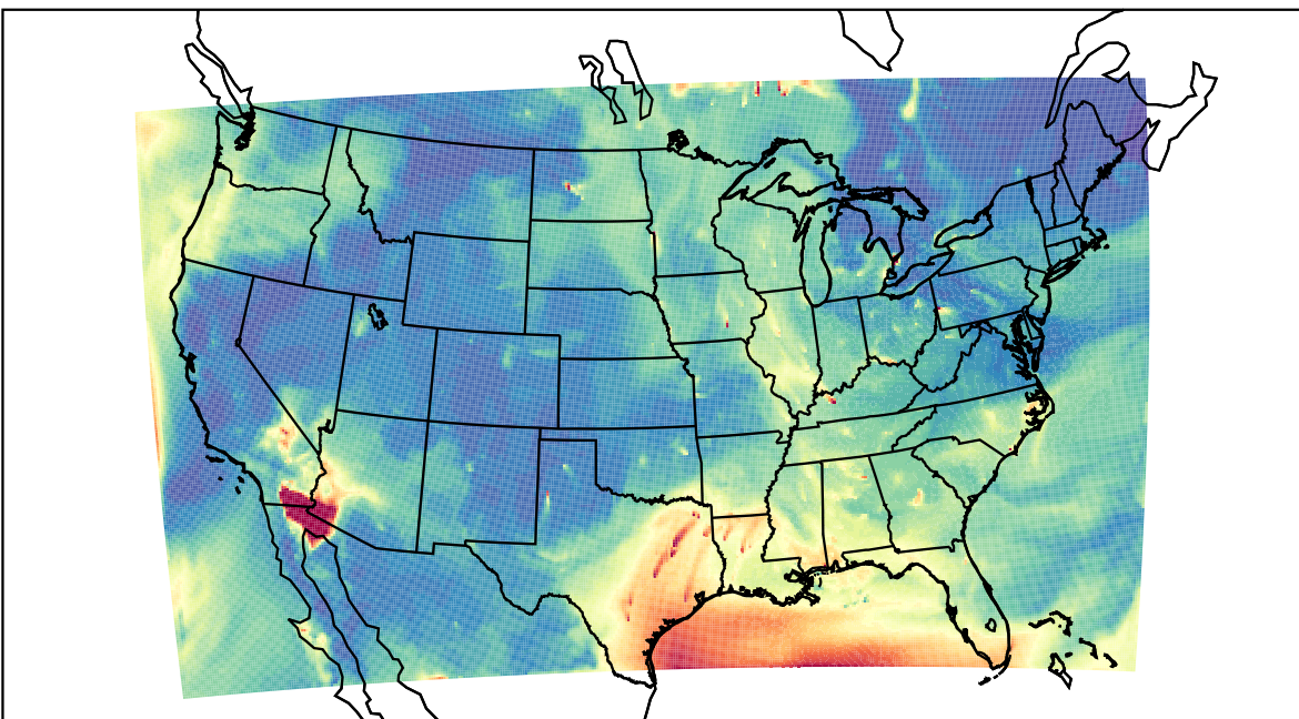
WRF 2023-06-18_14:00:00
