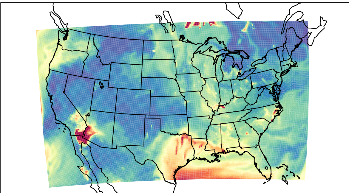
WRF 2023-06-18_10:00:00
