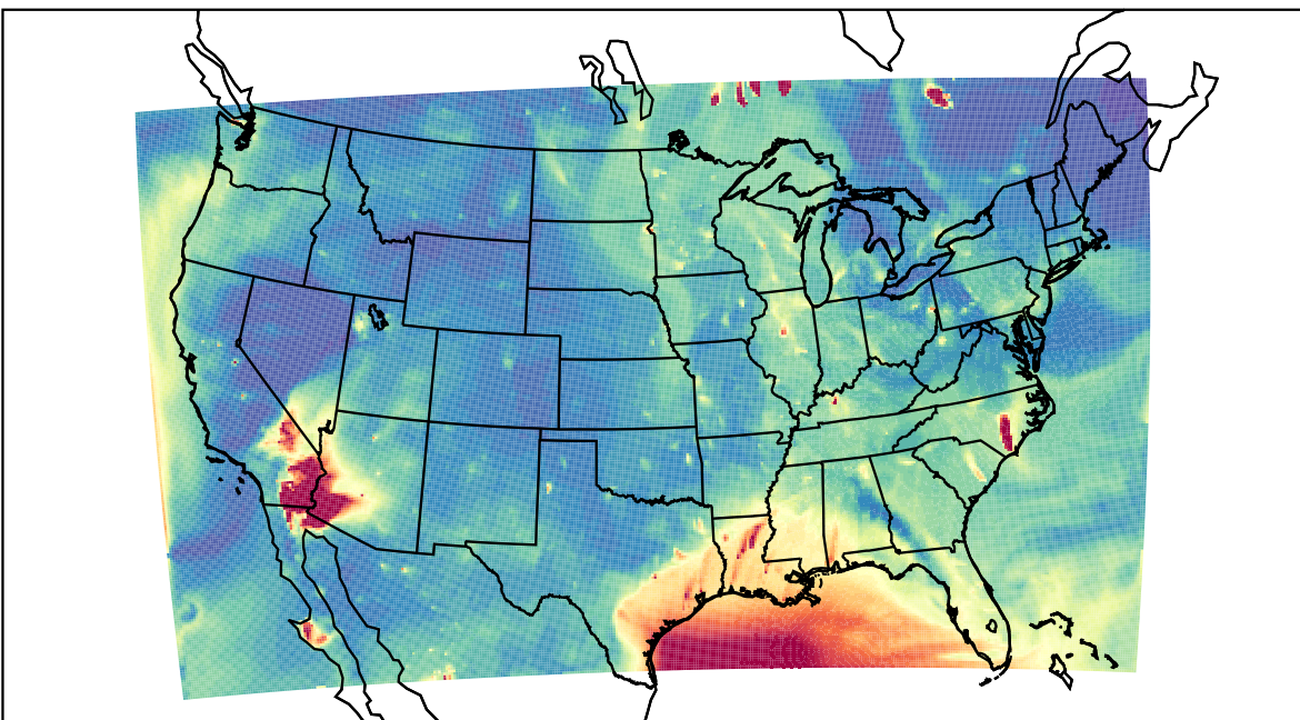
WRF 2023-06-19_03:00:00
