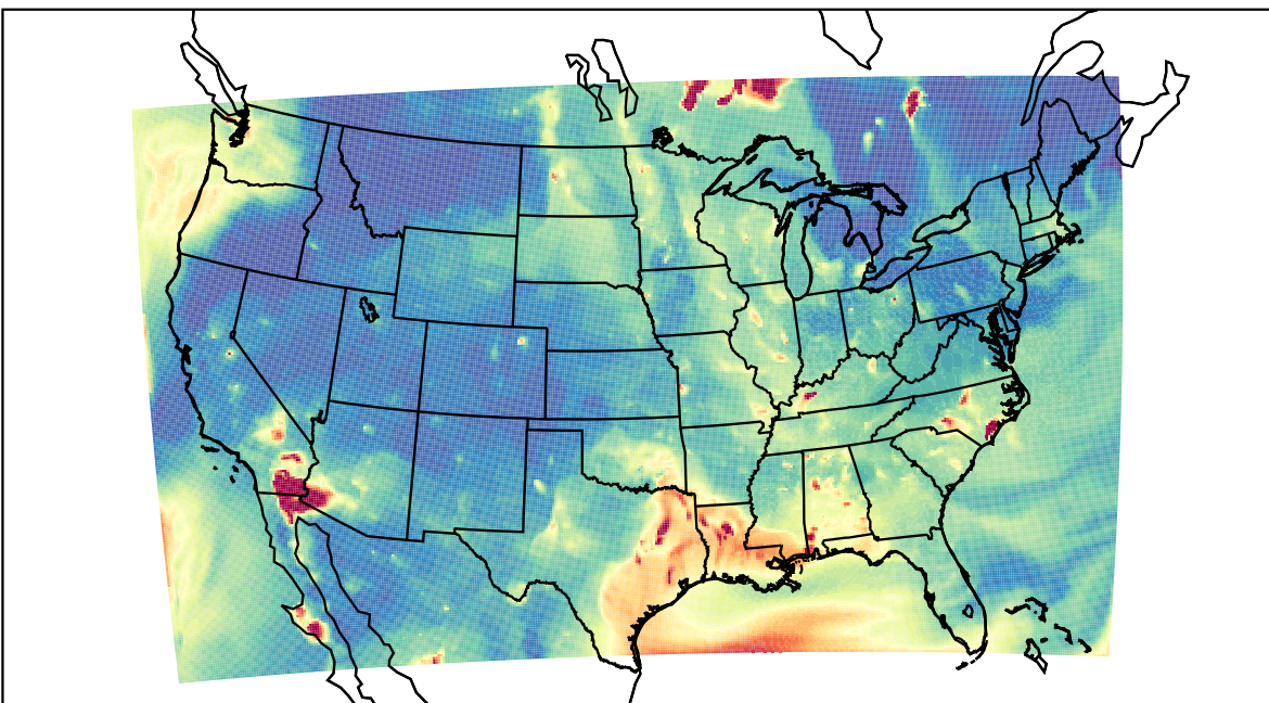
WRF 2023-06-18_04:00:00
