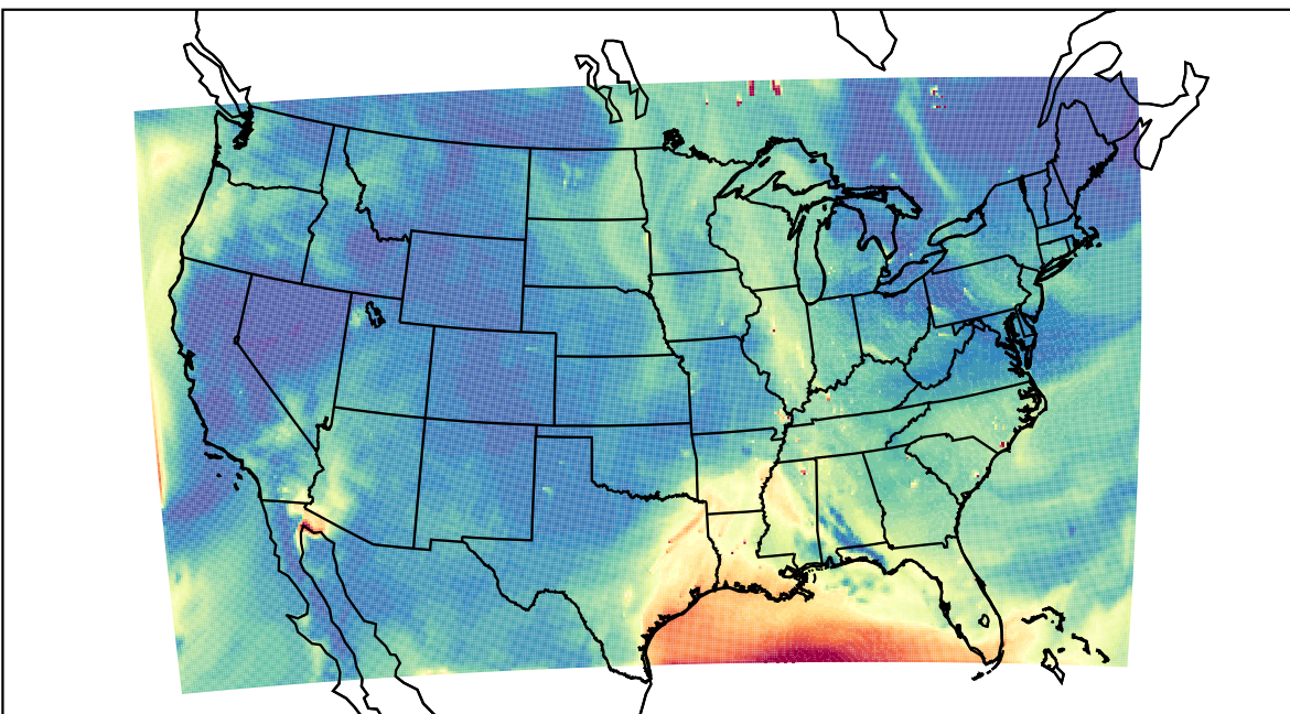
WRF 2023-06-18_19:00:00
