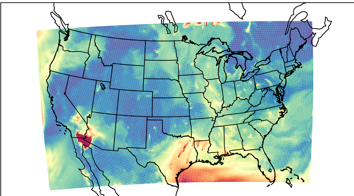
WRF 2023-06-18_13:00:00
