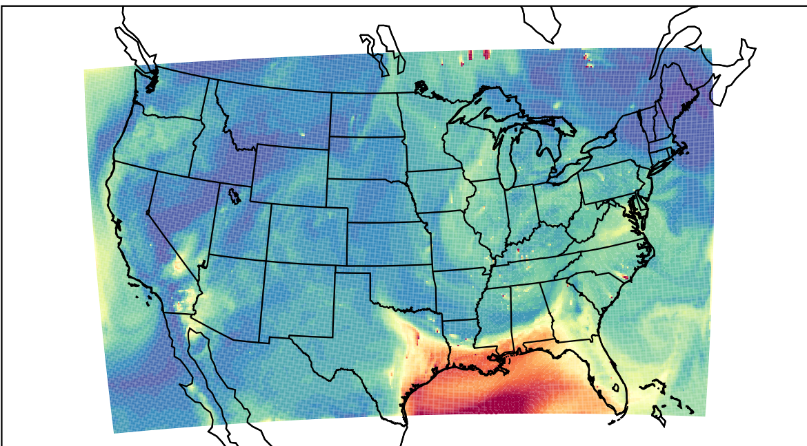
WRF 2023-06-19_20:00:00
