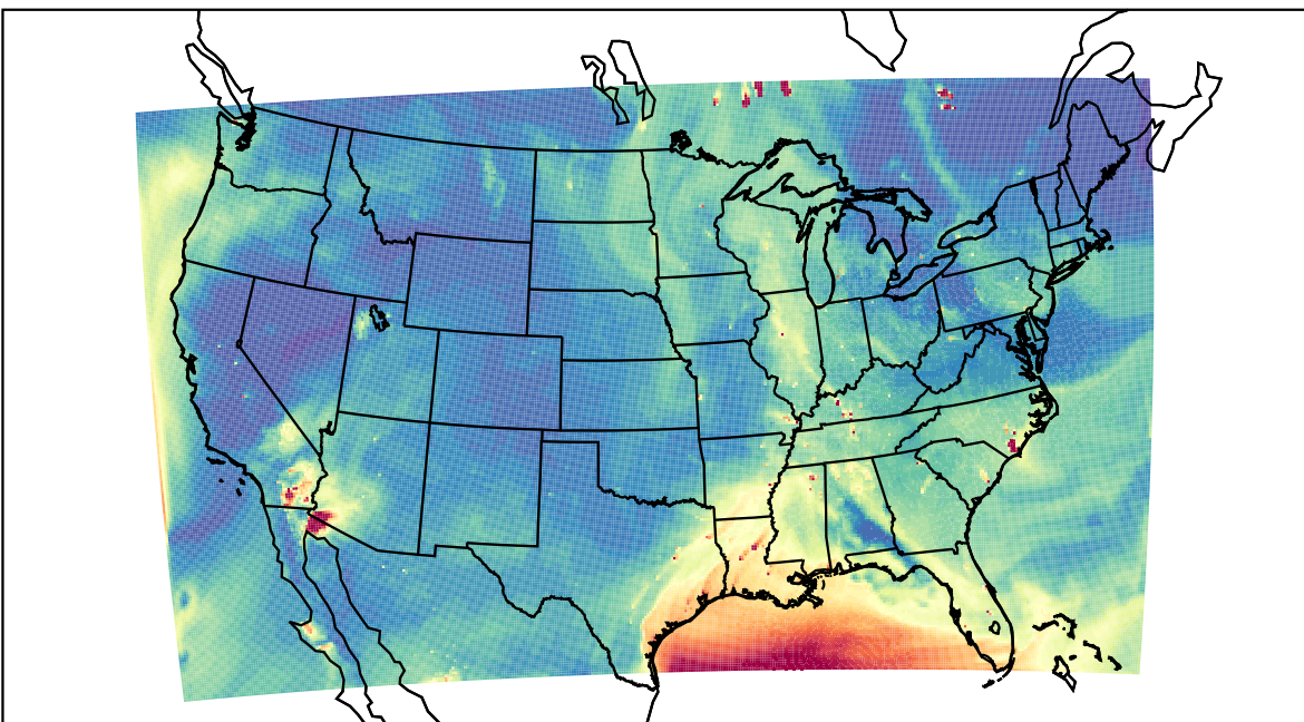
WRF 2023-06-18_23:00:00
