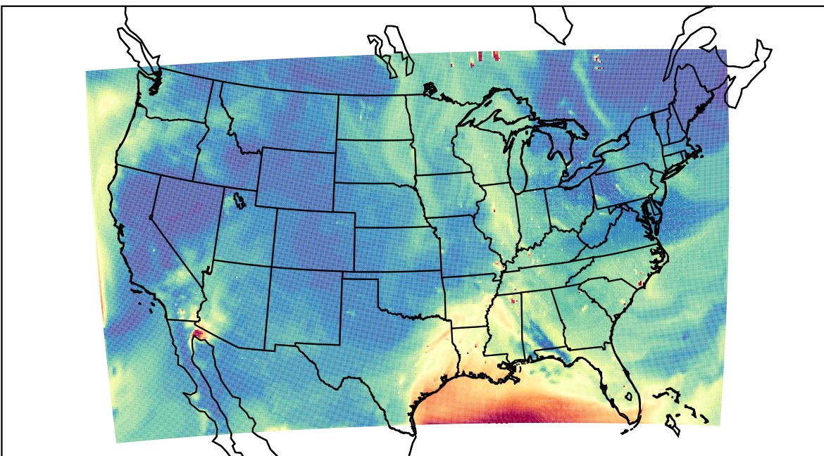
WRF 2023-06-18_20:00:00
