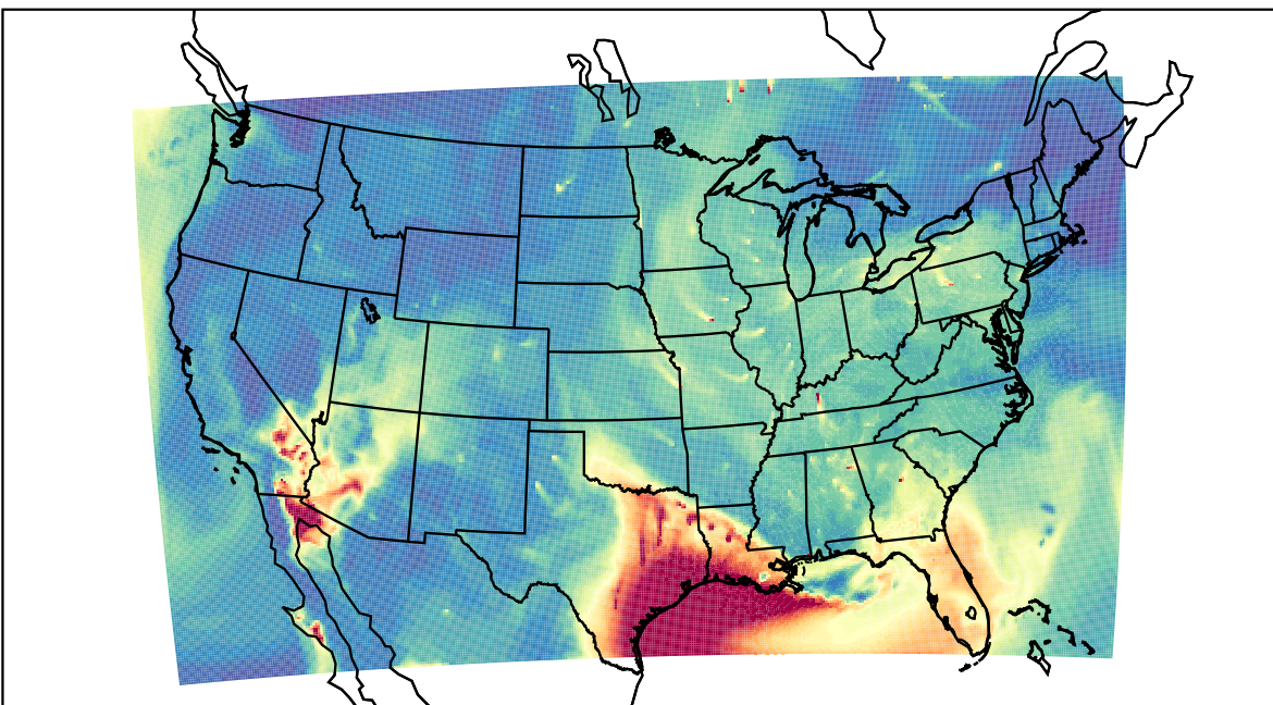
WRF 2023-06-20_14:00:00
