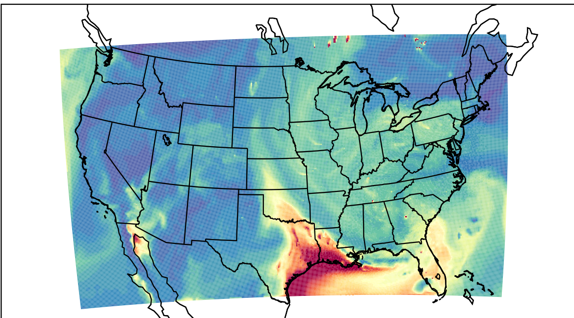
WRF 2023-06-20_19:00:00
