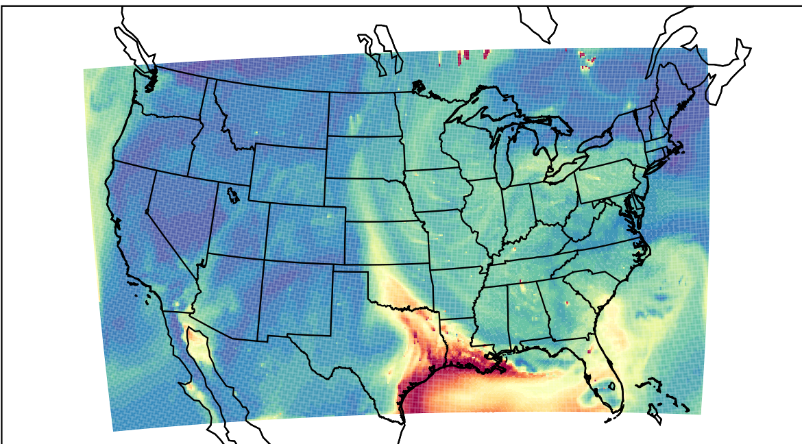
WRF 2023-06-20_22:00:00
