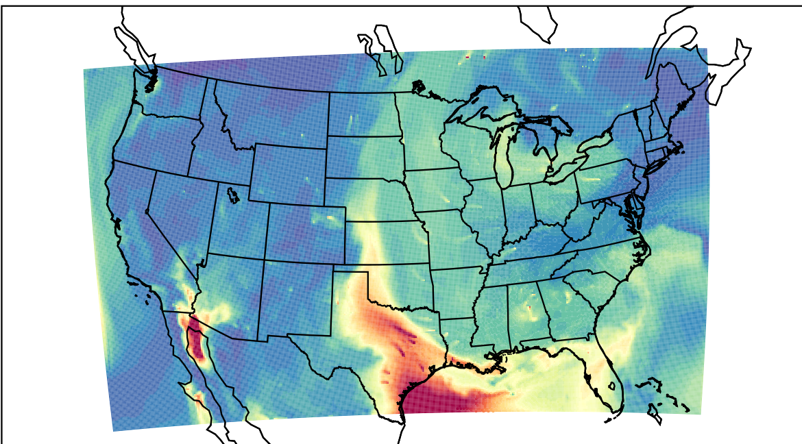
WRF 2023-06-21_16:00:00
