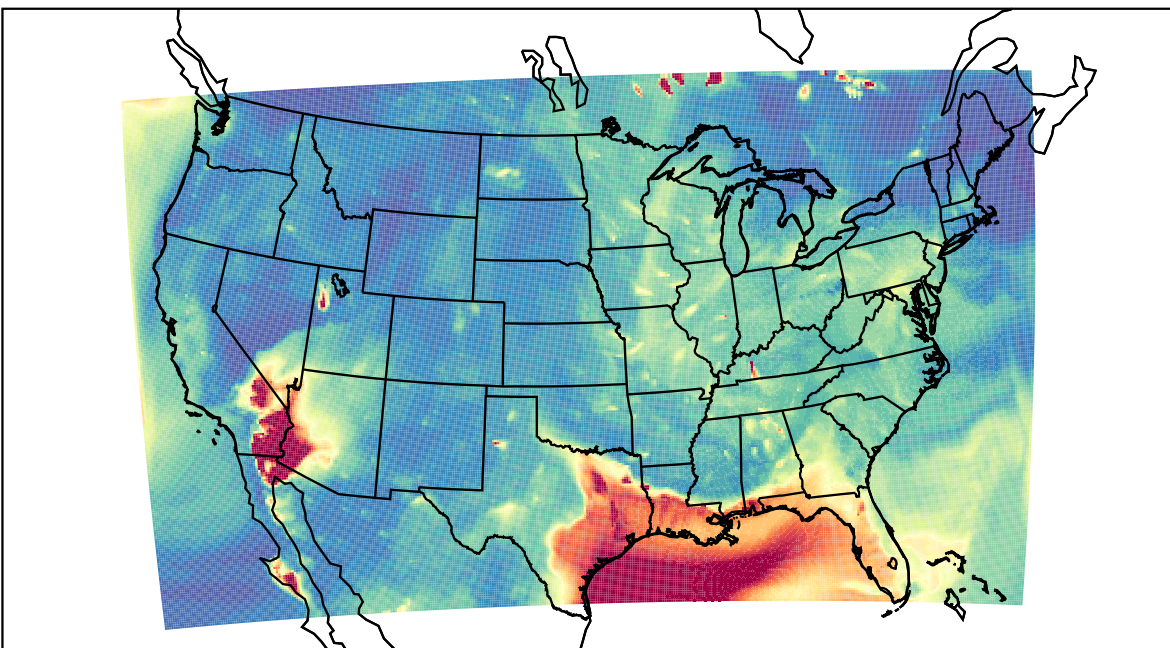
WRF 2023-06-20_04:00:00
