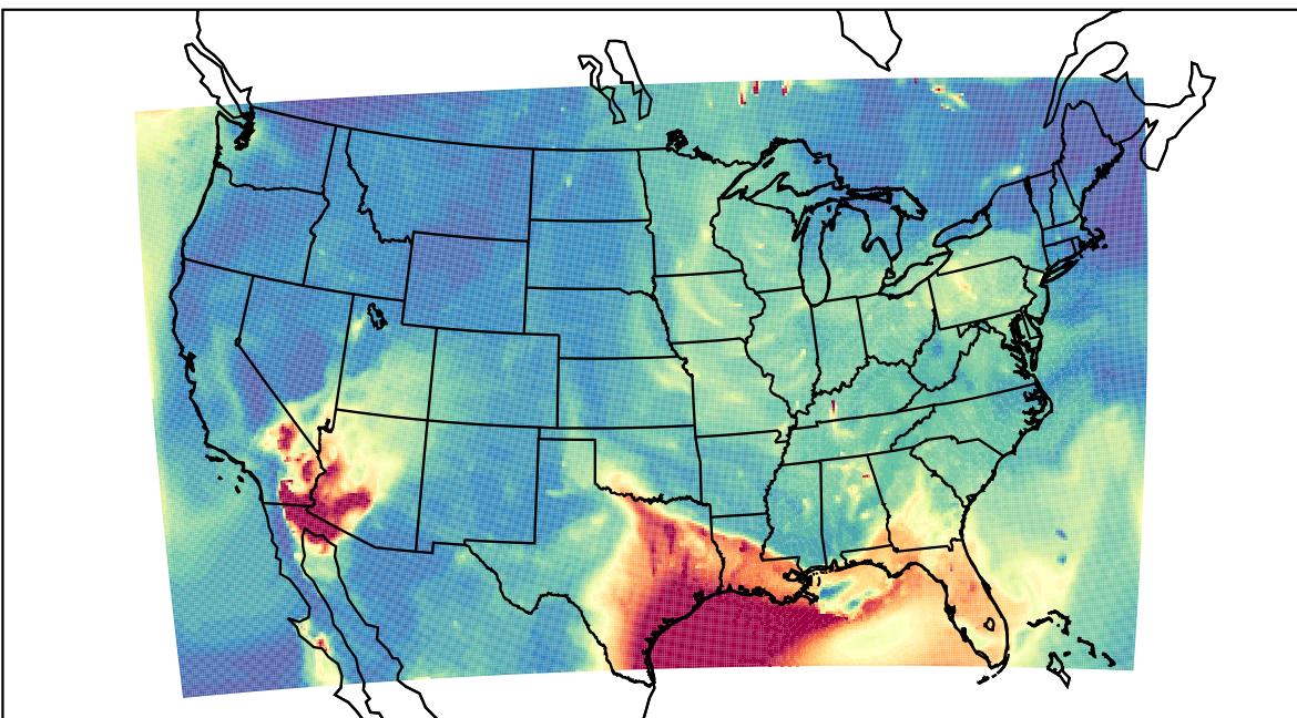
WRF 2023-06-20_10:00:00
