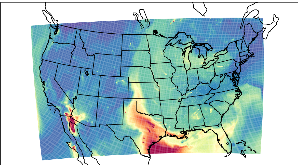
WRF 2023-06-21_15:00:00
