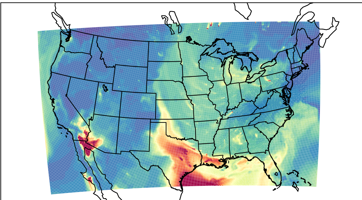
WRF 2023-06-21_12:00:00
