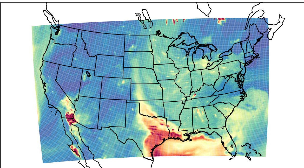
WRF 2023-06-21_04:00:00
