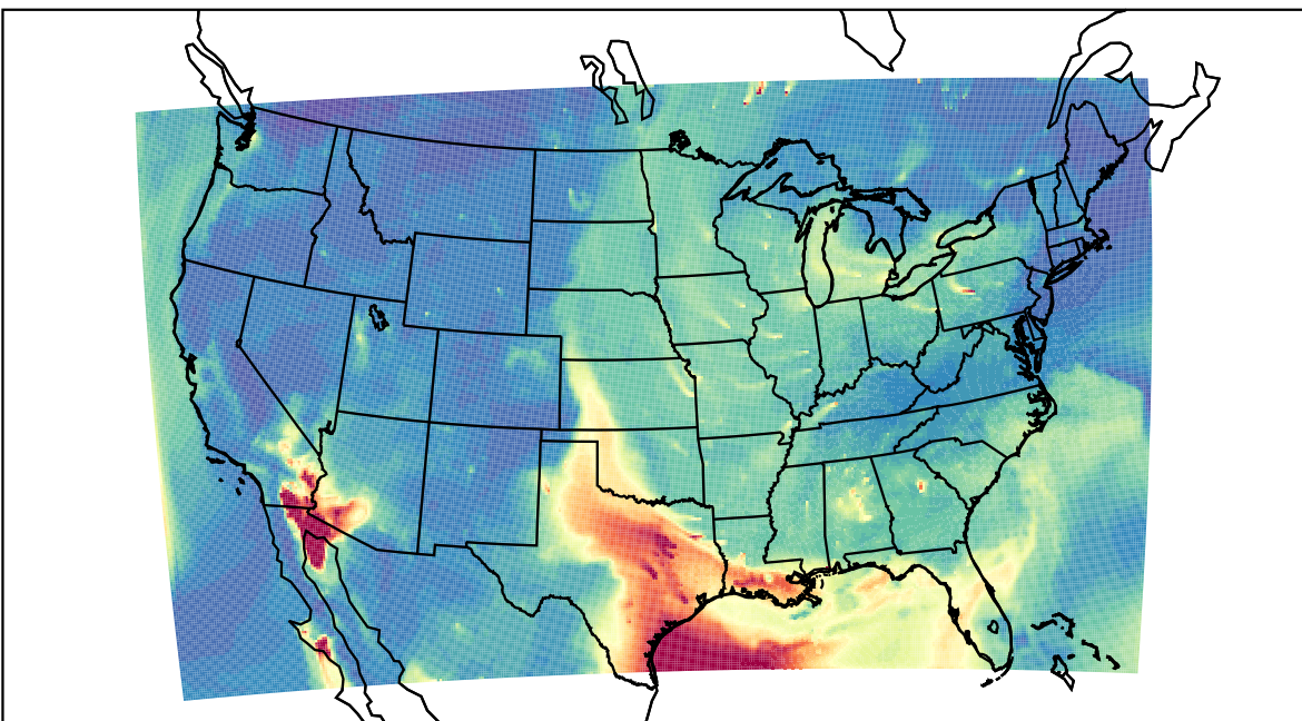
WRF 2023-06-21_13:00:00
