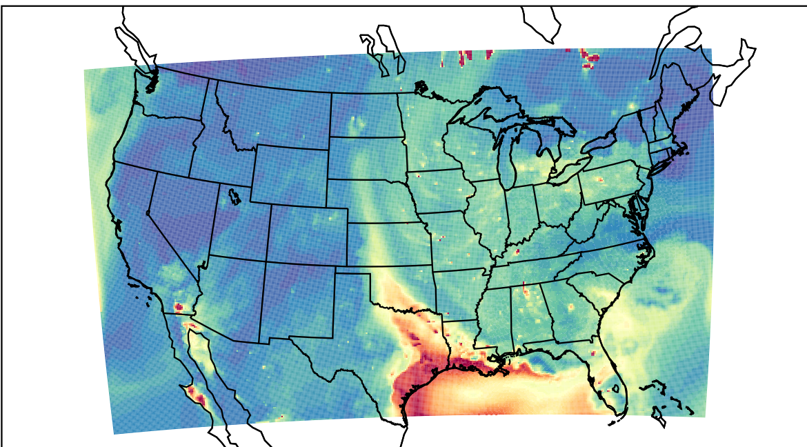
WRF 2023-06-21_01:00:00
