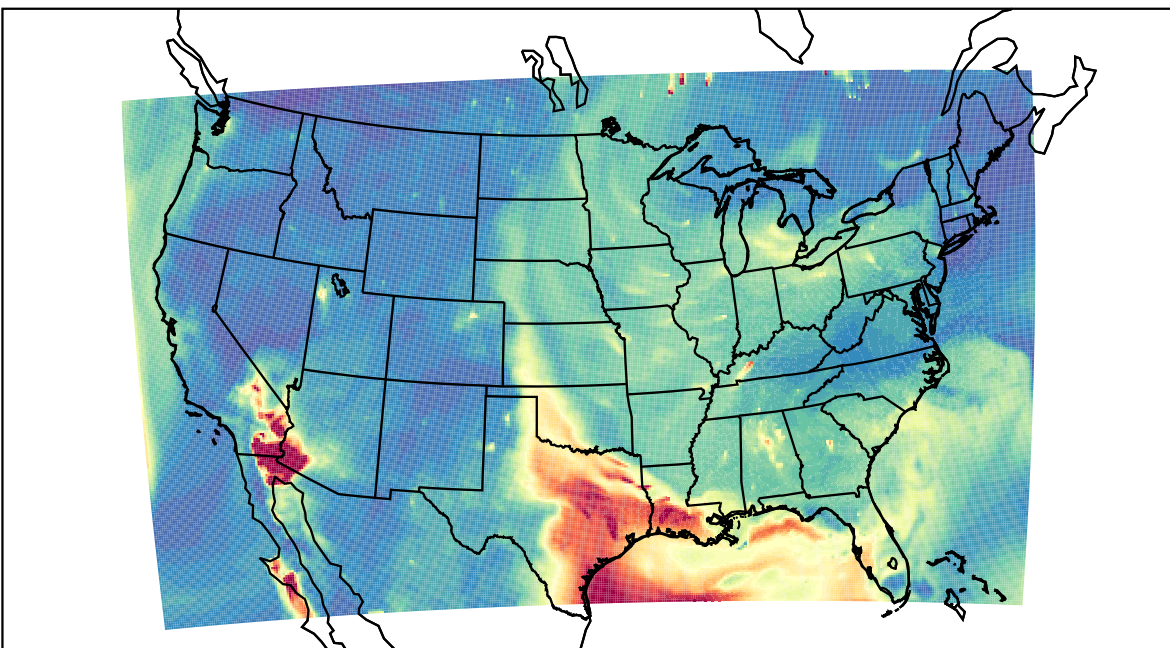
WRF 2023-06-21_07:00:00
