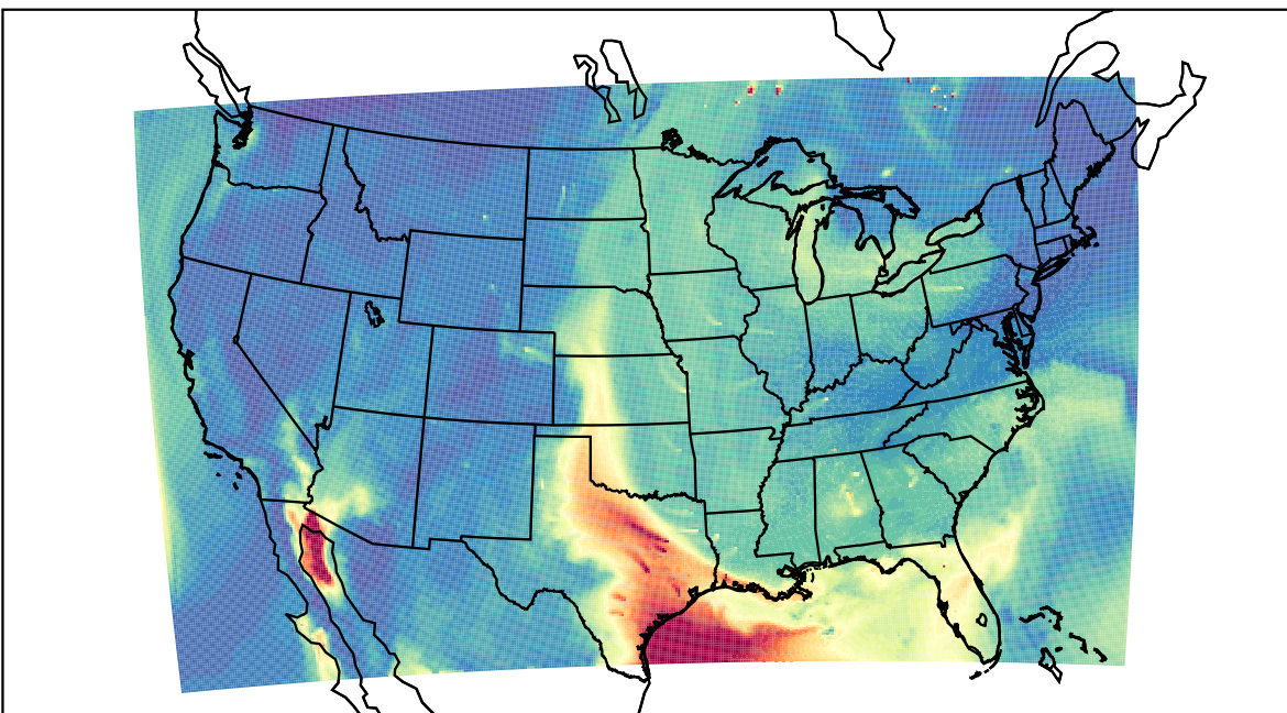
WRF 2023-06-21_17:00:00
