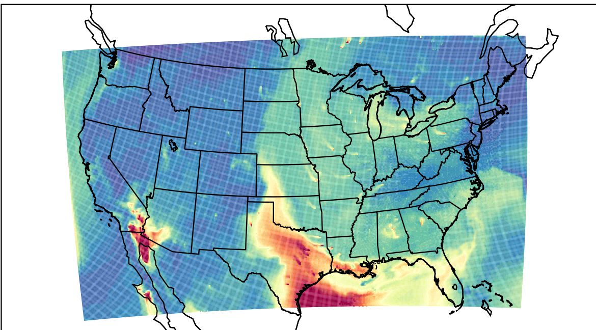
WRF 2023-06-21_14:00:00
