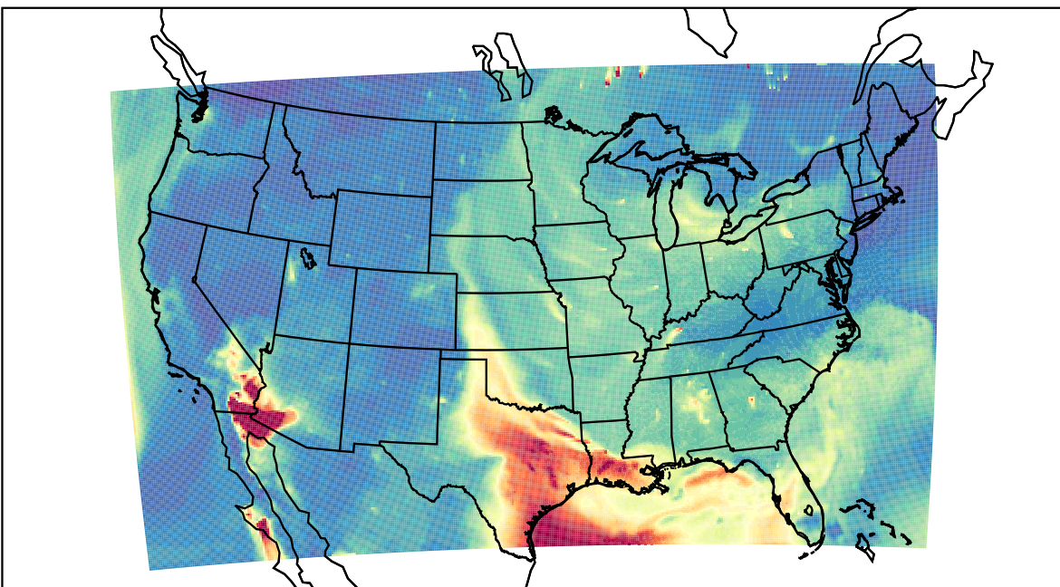
WRF 2023-06-21_09:00:00
