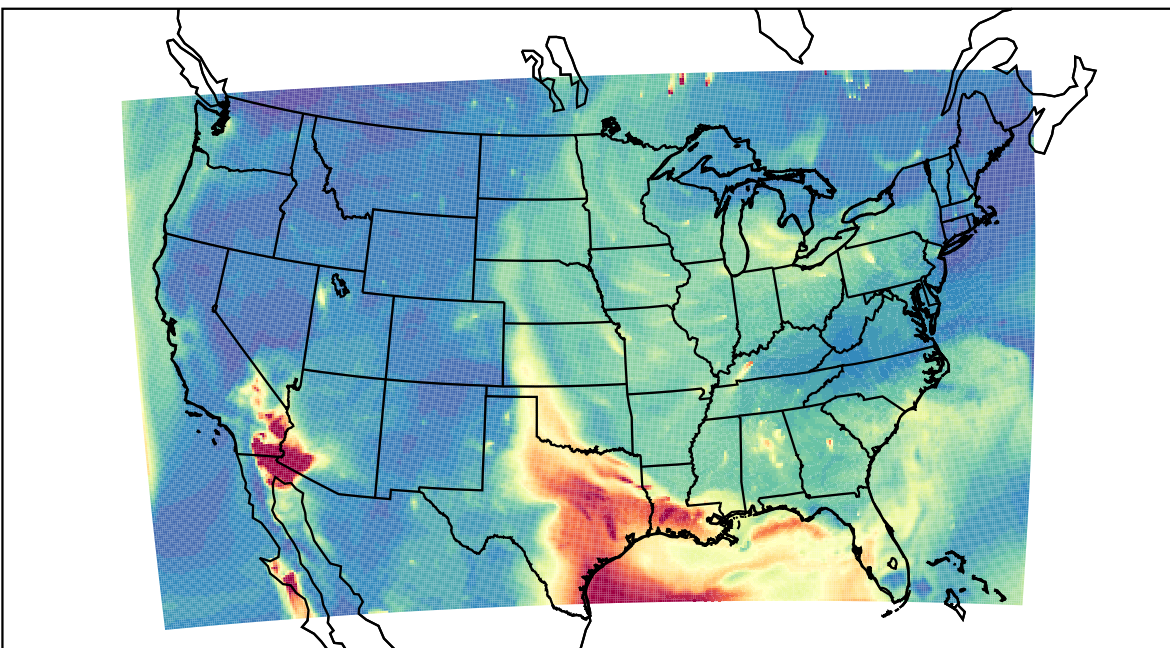
WRF 2023-06-21_08:00:00
