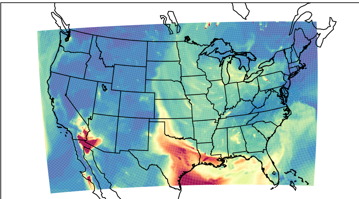
WRF 2023-06-21_11:00:00
