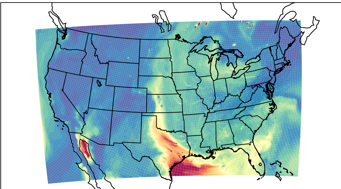
WRF 2023-06-21_19:00:00
