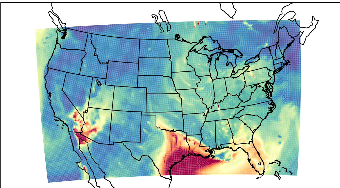
WRF 2023-06-20_13:00:00
