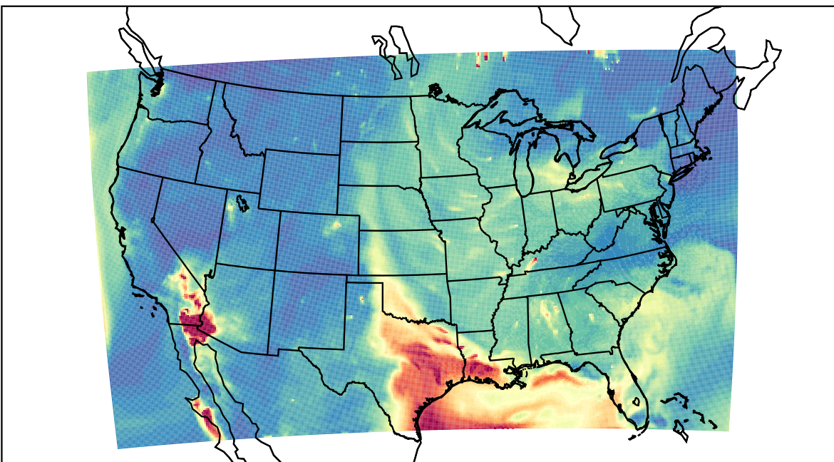
WRF 2023-06-21_06:00:00
