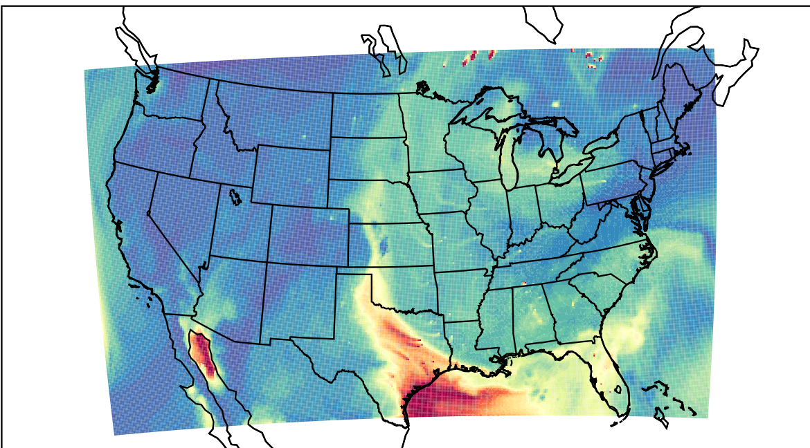
WRF 2023-06-21_20:00:00
