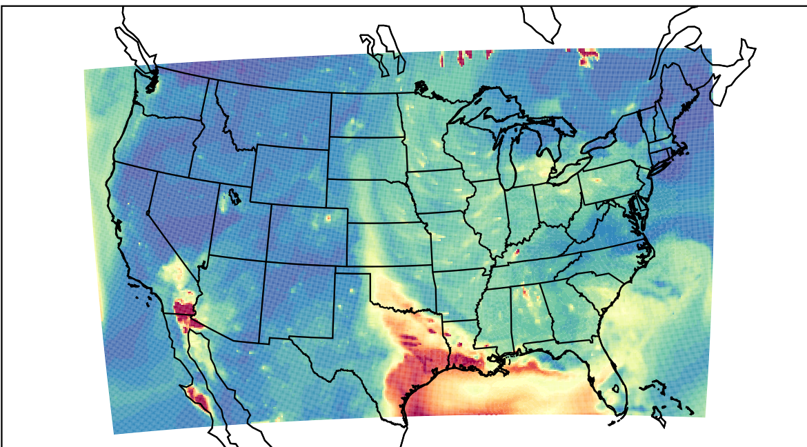
WRF 2023-06-21_03:00:00
