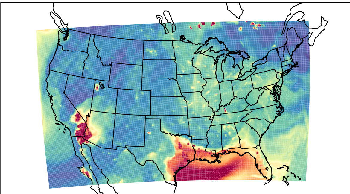
WRF 2023-06-20_03:00:00
