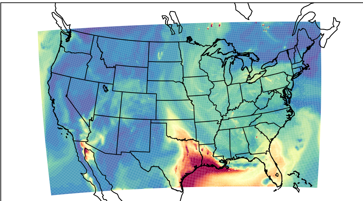
WRF 2023-06-20_18:00:00
