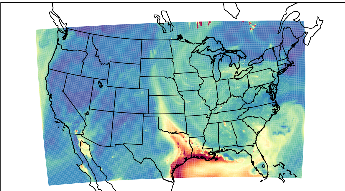
WRF 2023-06-20_23:00:00
