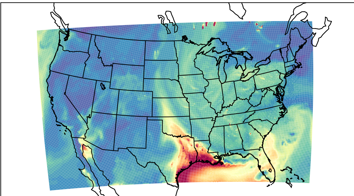
WRF 2023-06-20_20:00:00
