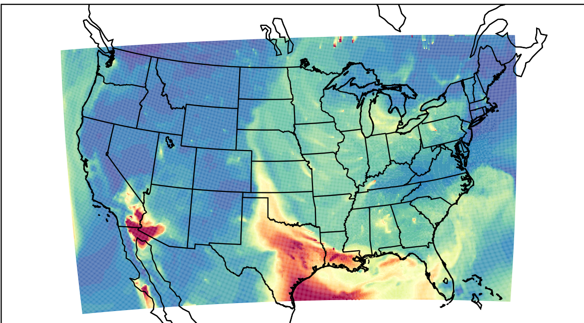
WRF 2023-06-21_10:00:00
