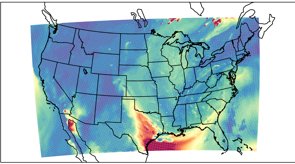
WRF 2023-06-22_20:00:00
