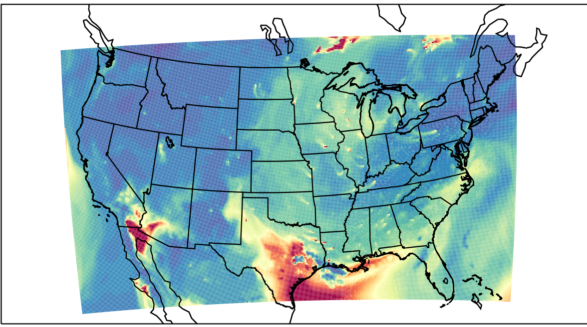
WRF 2023-06-22_14:00:00
