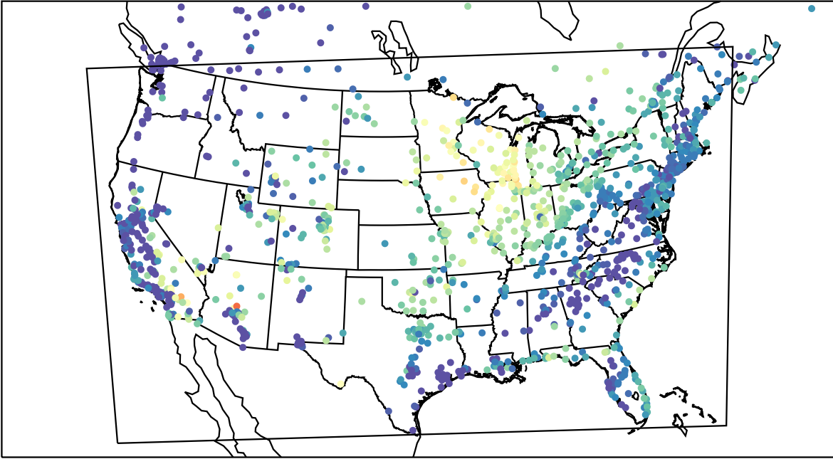
AirNOW (2023-06-22_13:00:00)
