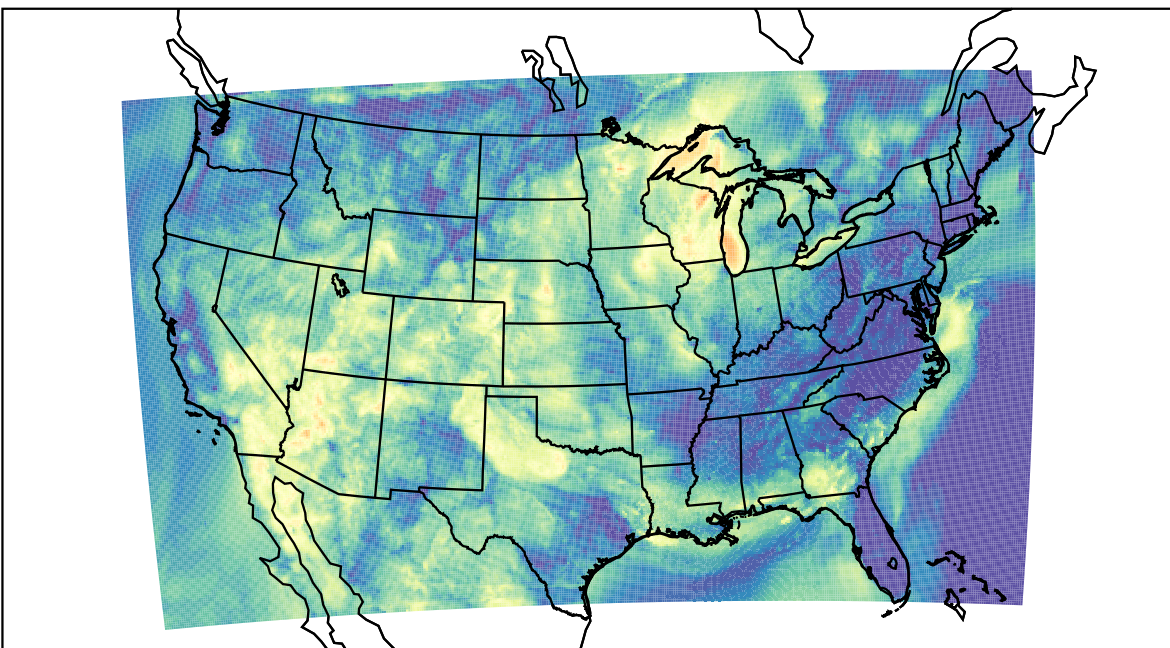
WRF (2023-06-22_10:00:00)
