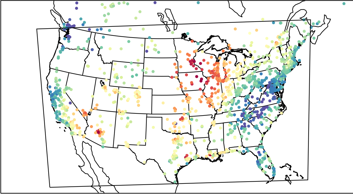
AirNOW (2023-06-22_18:00:00)
