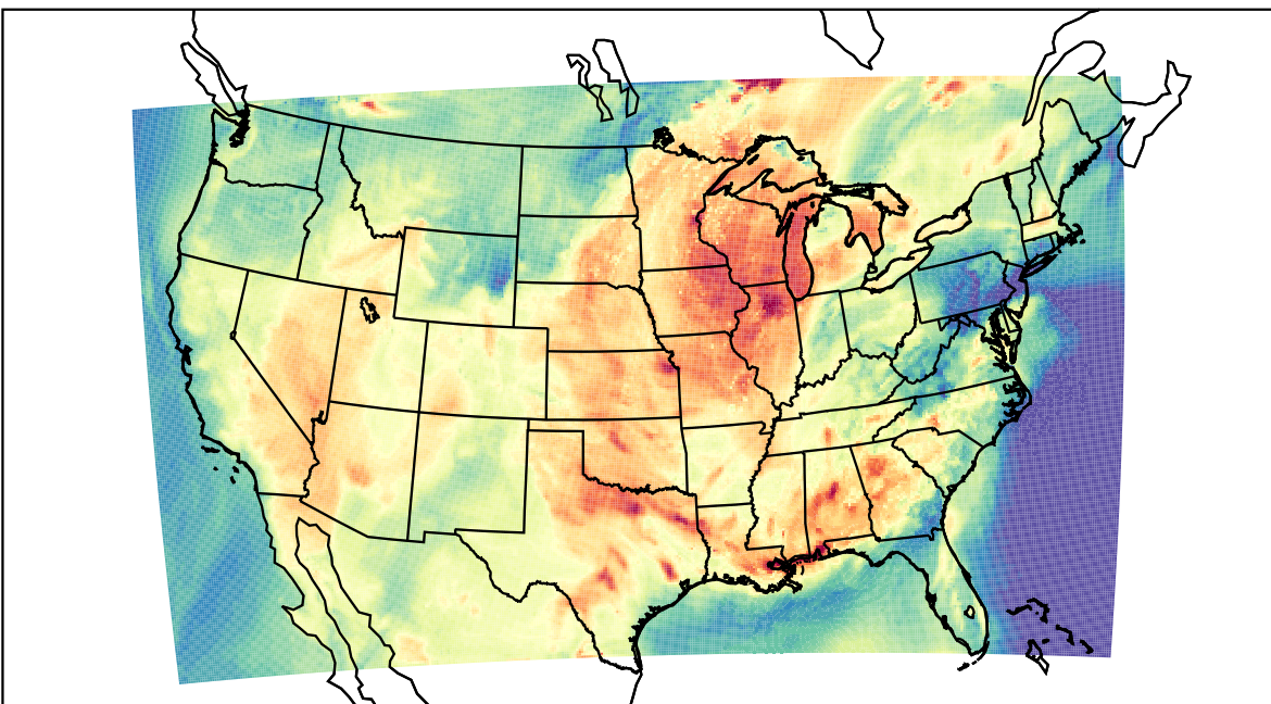
WRF (2023-06-22_20:00:00)
