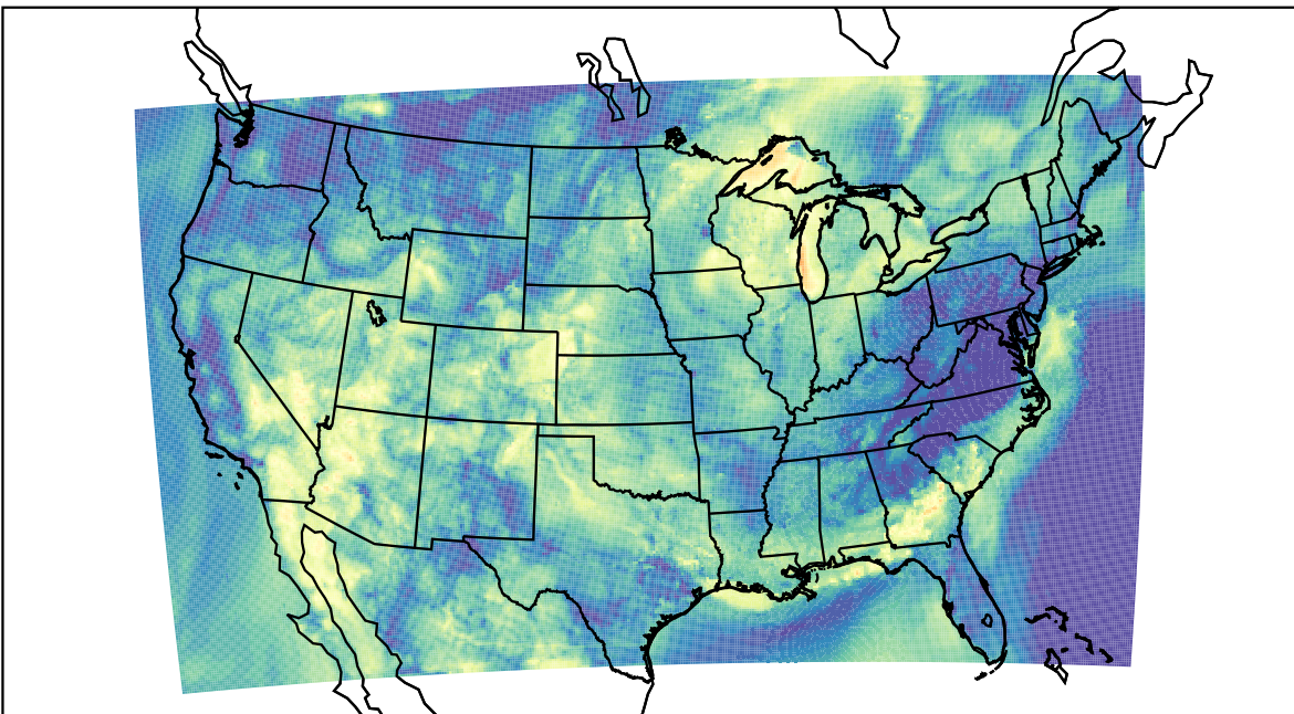
WRF (2023-06-22_13:00:00)
