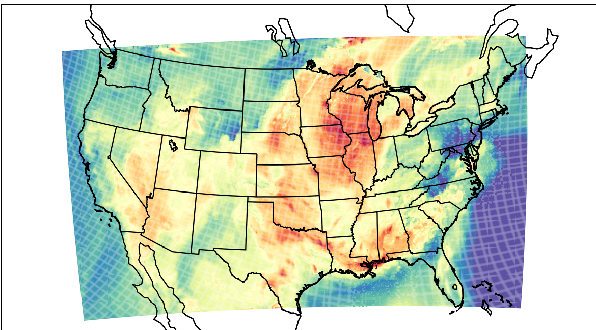
WRF (2023-06-22_18:00:00)
