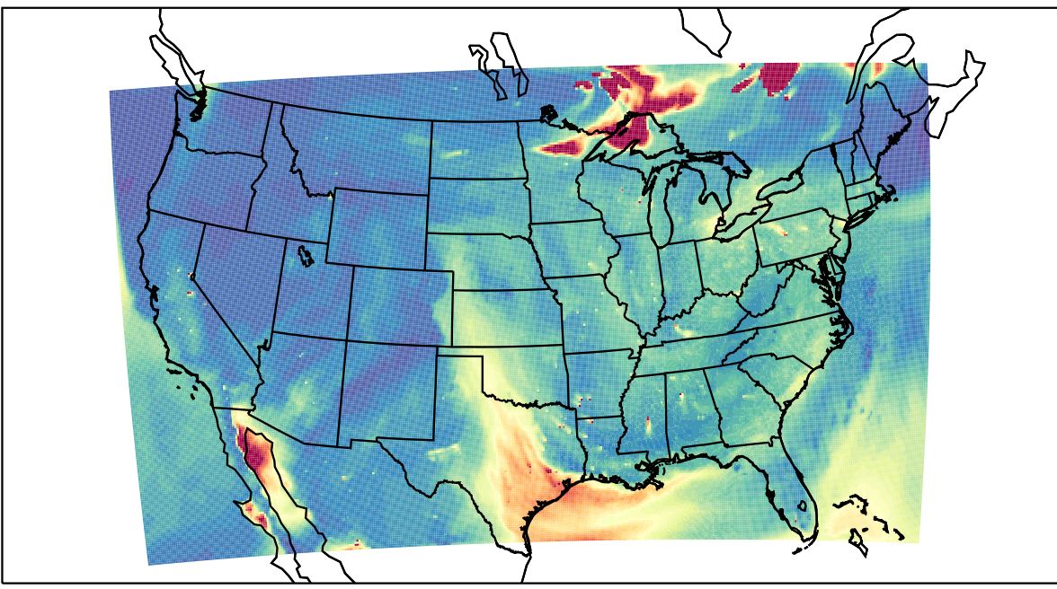
WRF 2023-06-23_23:00:00
