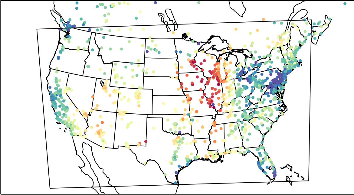
AirNOW (2023-06-23_18:00:00)
