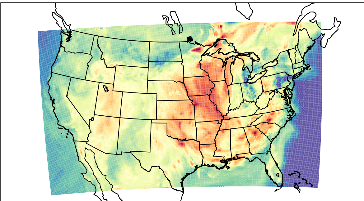
WRF (2023-06-23_18:00:00)
