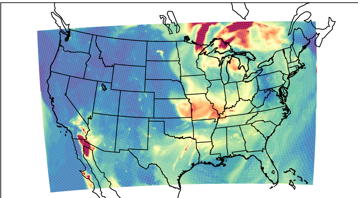
WRF 2023-06-26_14:00:00
