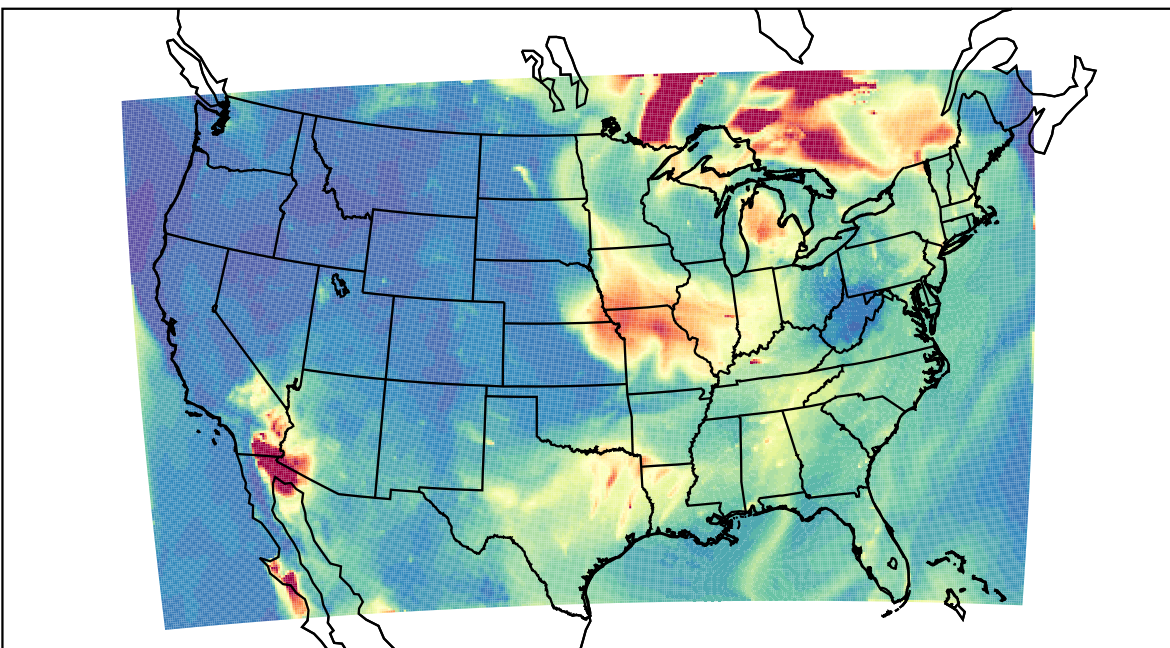
WRF 2023-06-26_10:00:00
