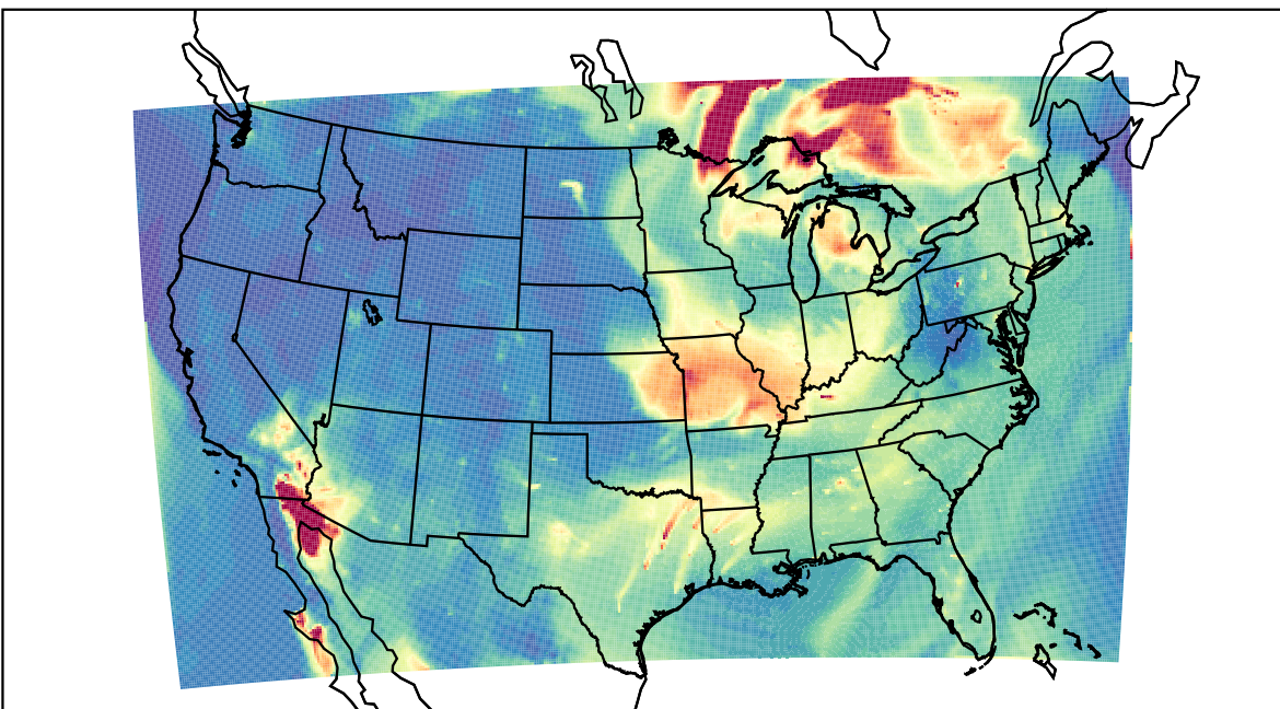
WRF 2023-06-26_13:00:00
