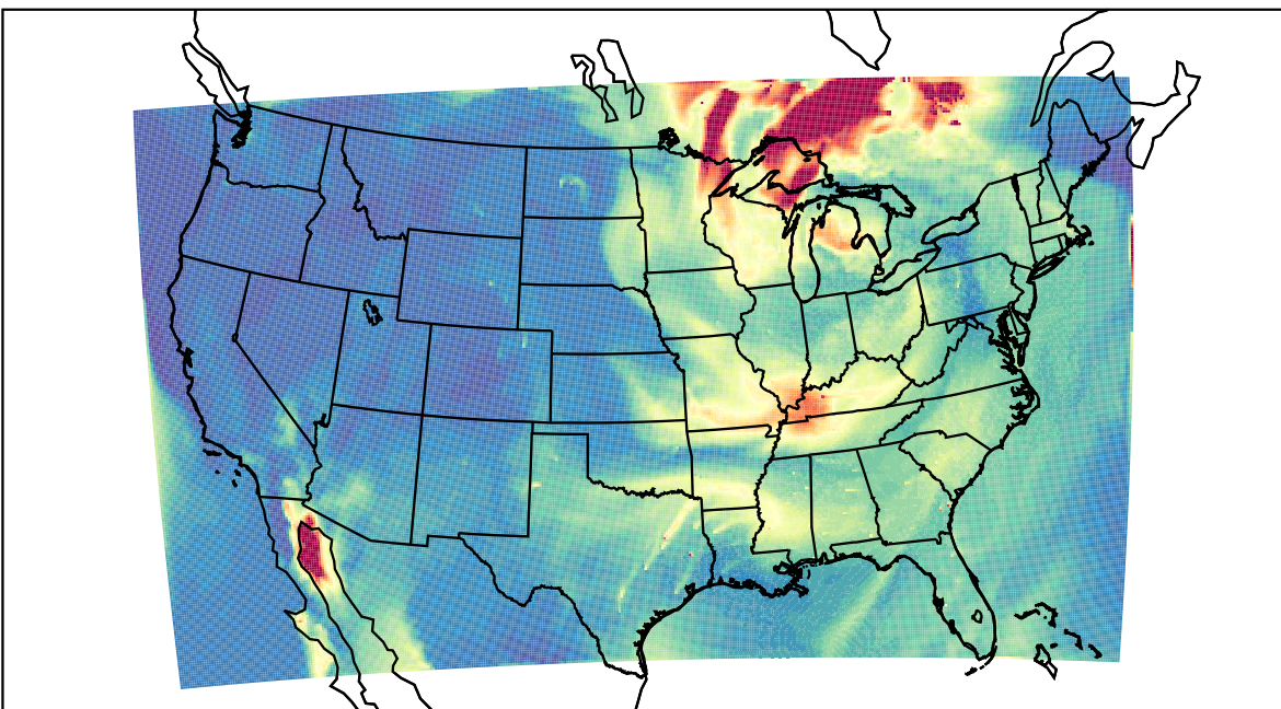
WRF 2023-06-26_18:00:00
