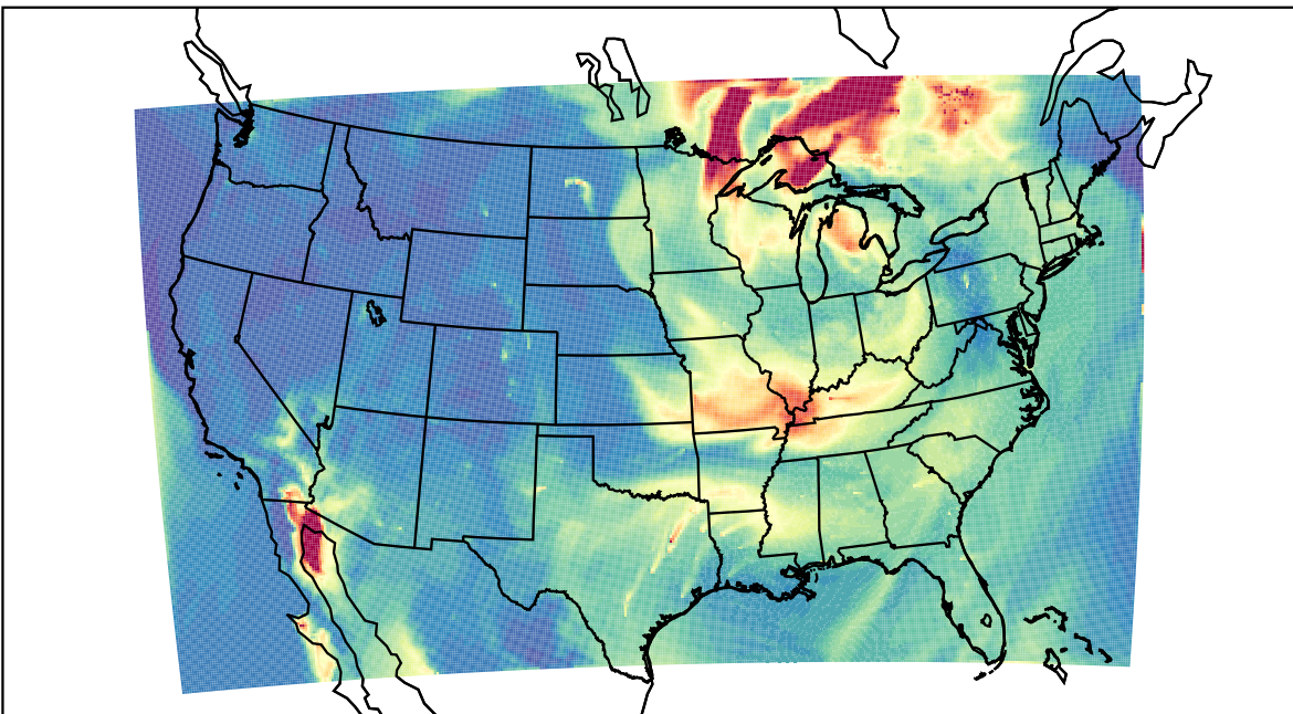
WRF 2023-06-26_16:00:00
