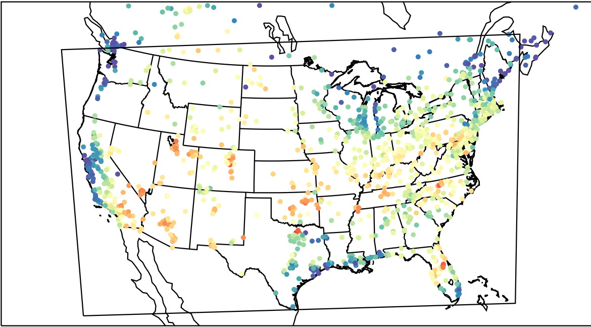
AirNOW (2023-06-26_18:00:00)
