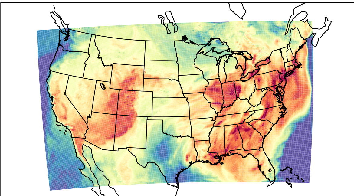
WRF (2023-06-30_19:00:00)
