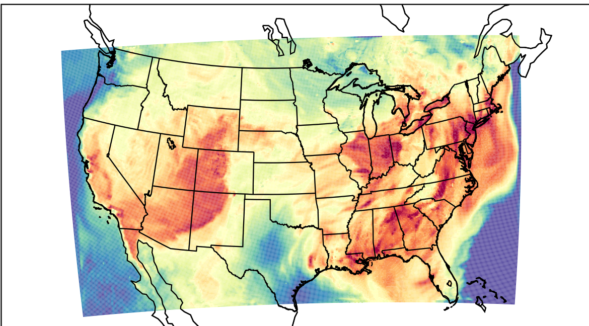
WRF (2023-06-30_20:00:00)
