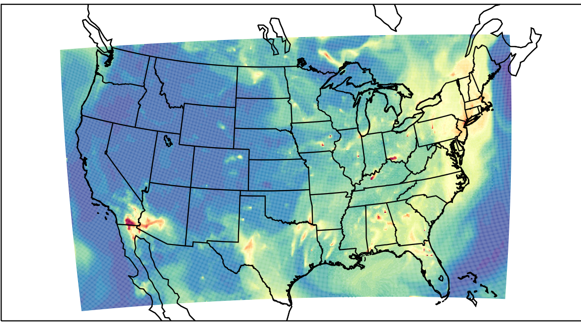
WRF 2023-07-01_10:00:00
