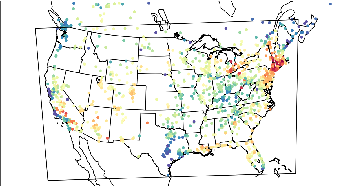
AirNOW (2023-07-01_16:00:00)
