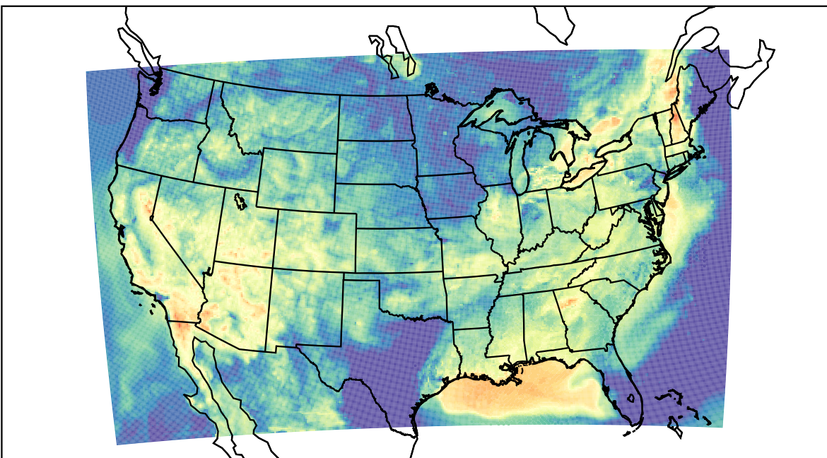
WRF (2023-07-02_13:00:00)
