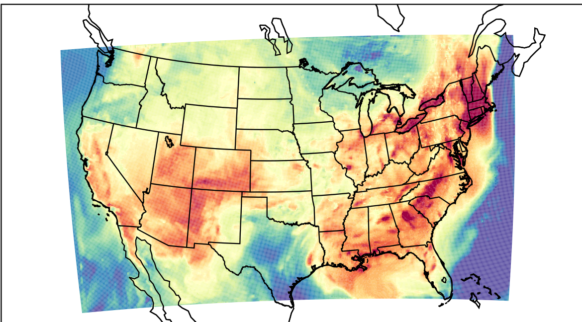
WRF (2023-07-01_18:00:00)
