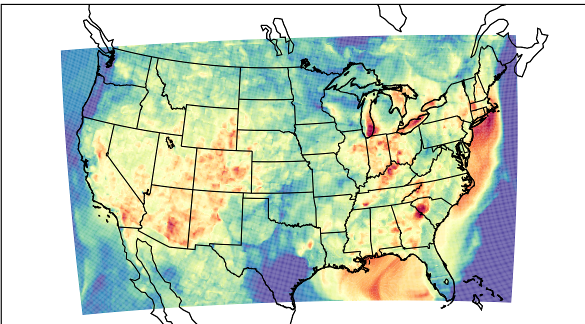
WRF (2023-07-01_04:00:00)
