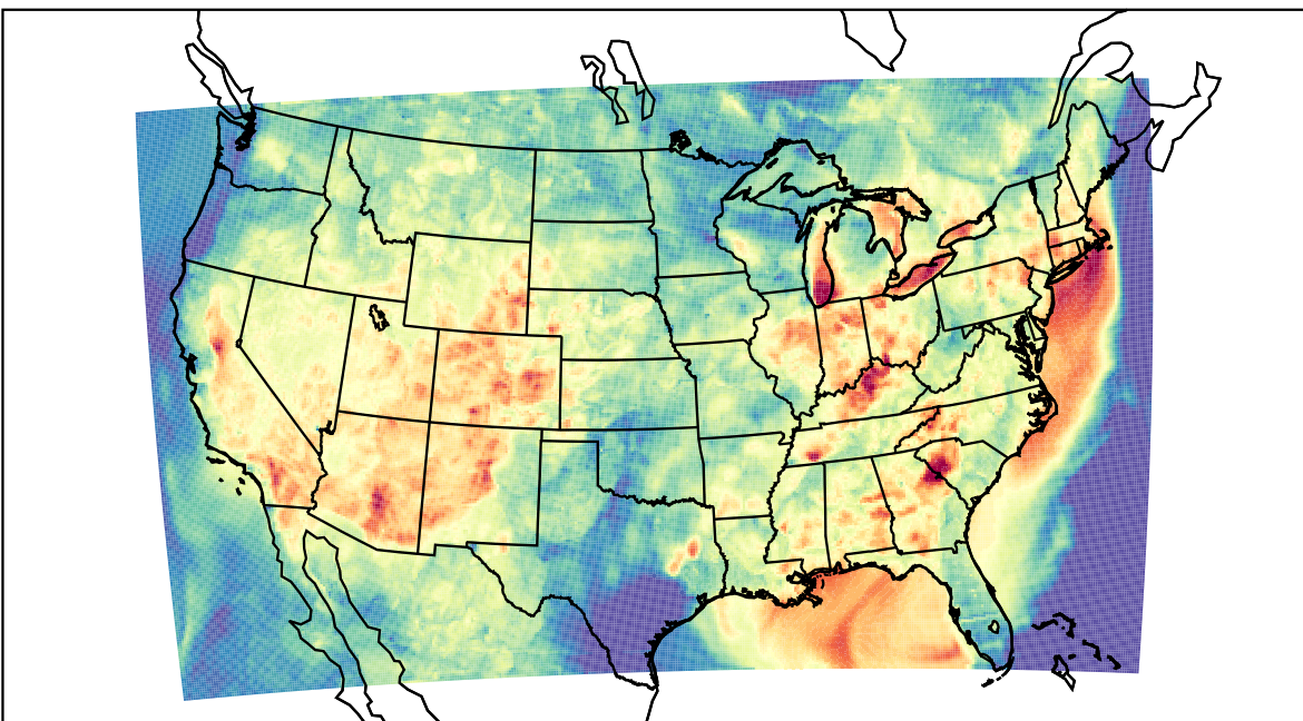
WRF (2023-07-01_03:00:00)
