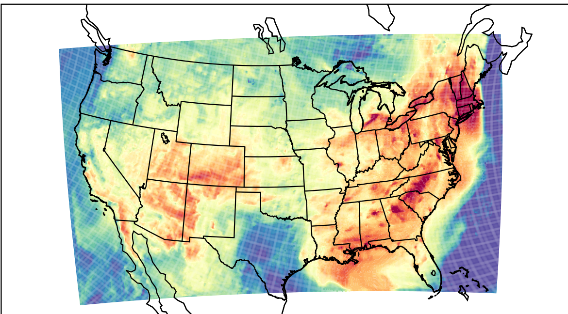
WRF (2023-07-01_16:00:00)
