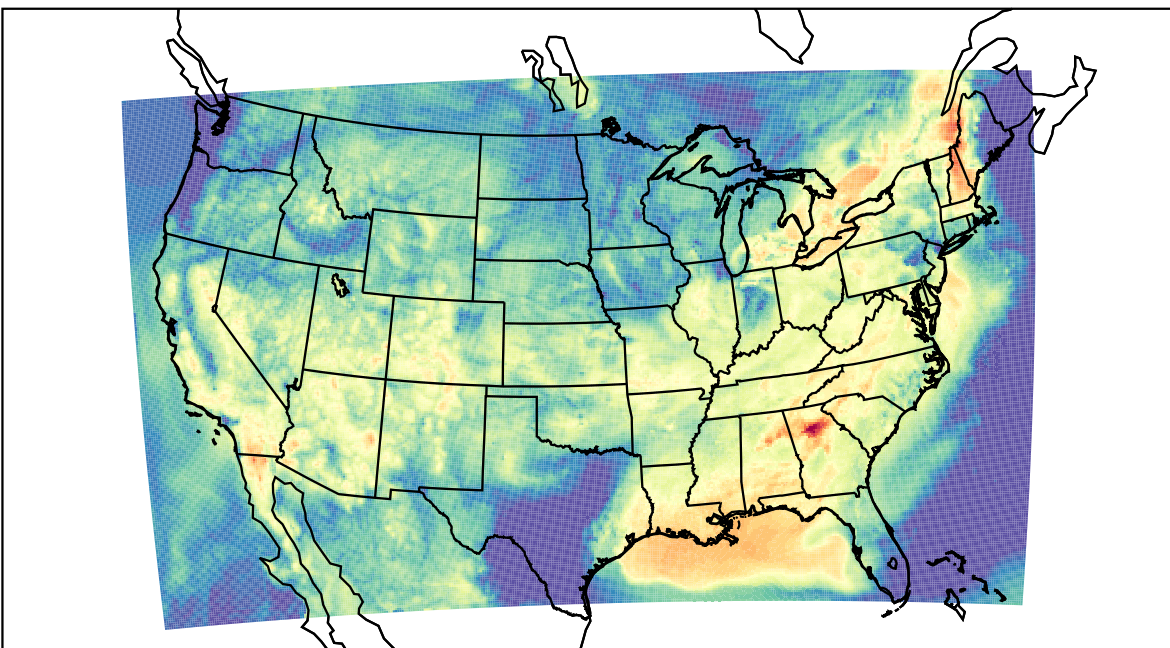
WRF (2023-07-02_14:00:00)
