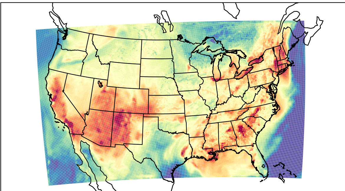
WRF (2023-07-01_23:00:00)
