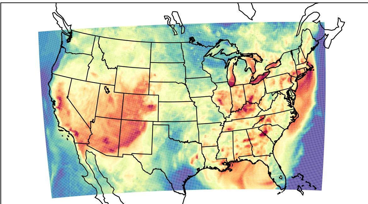
WRF (2023-07-01_01:00:00)
