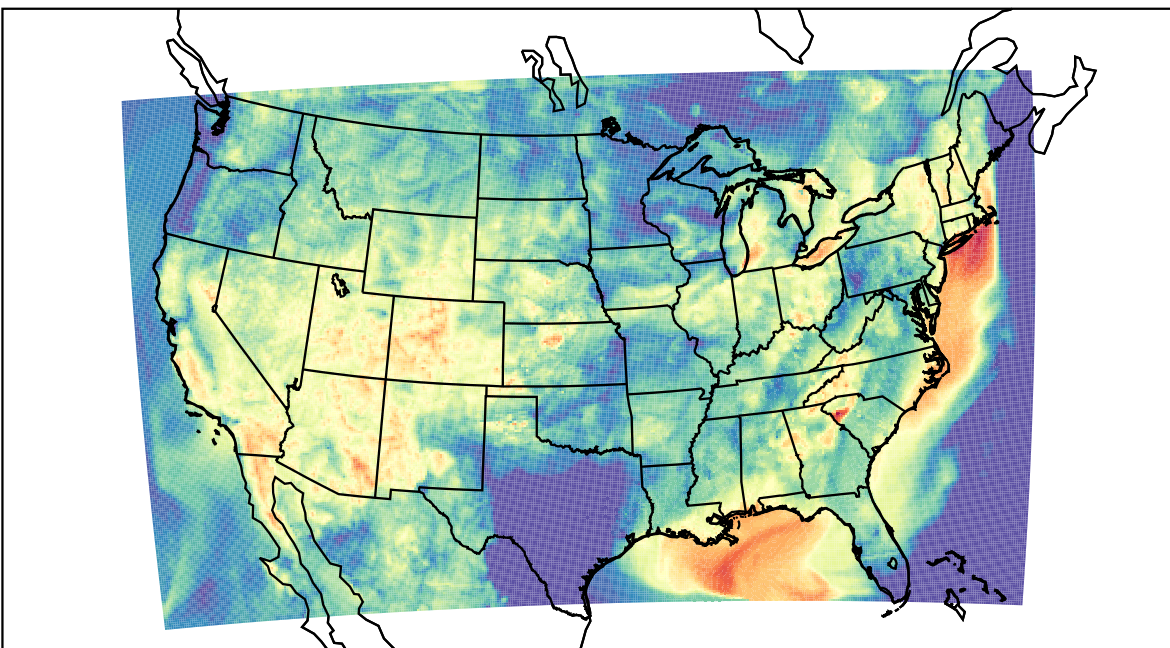
WRF (2023-07-01_10:00:00)
