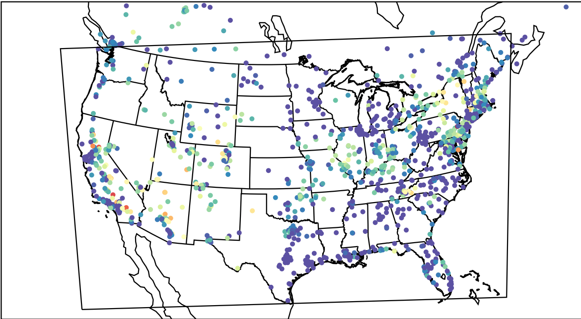
AirNOW (2023-07-01_10:00:00)
