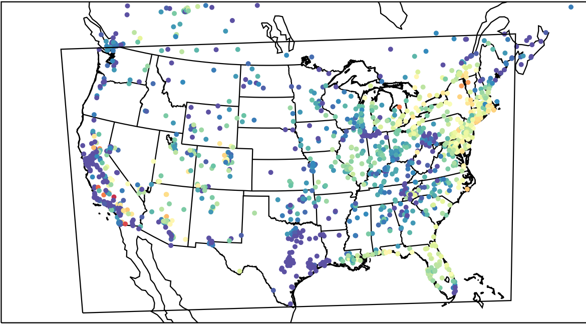
AirNOW (2023-07-01_13:00:00)
