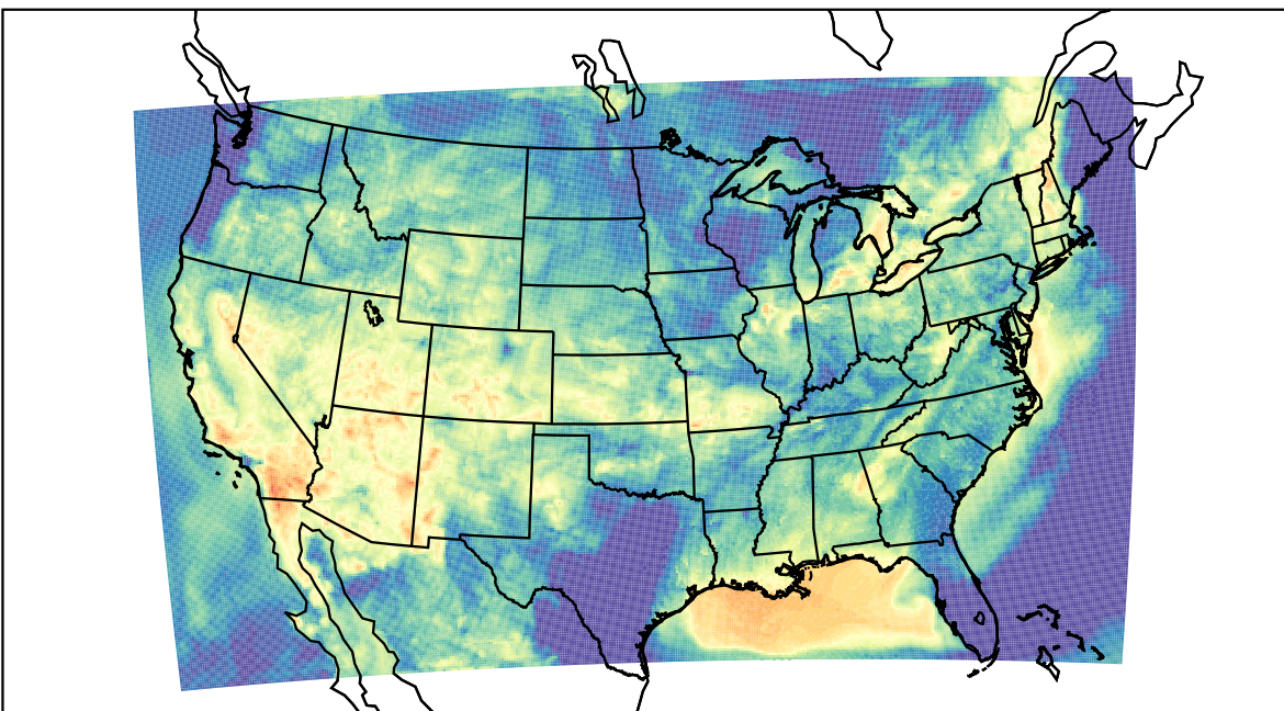
WRF (2023-07-02_10:00:00)
