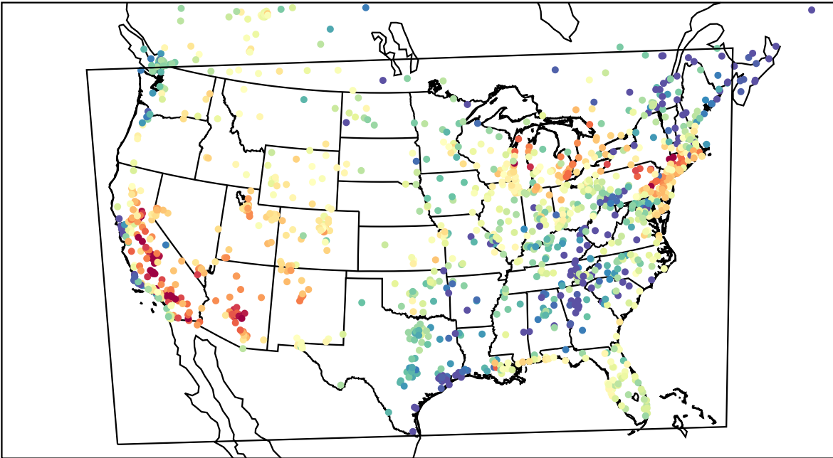
AirNOW (2023-07-01_01:00:00)
