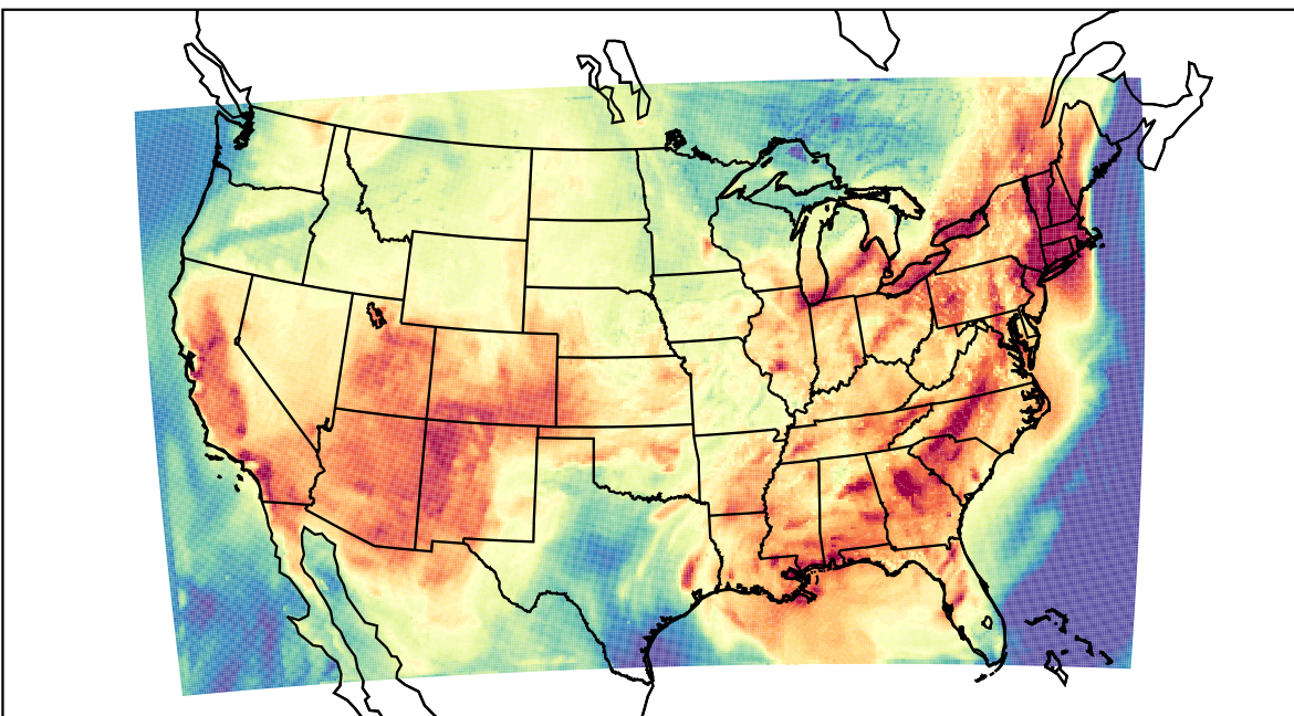
WRF (2023-07-01_20:00:00)
