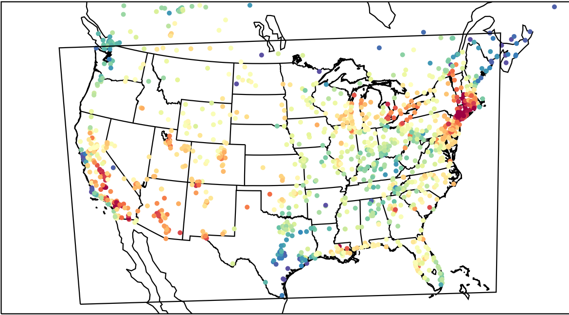
AirNOW (2023-07-01_18:00:00)
