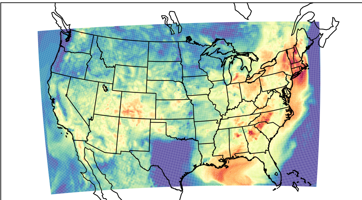
WRF (2023-07-01_14:00:00)
