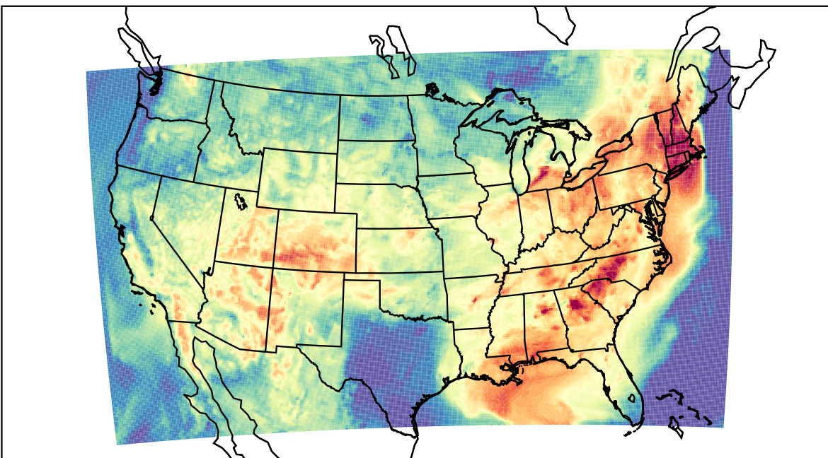
WRF (2023-07-01_15:00:00)
