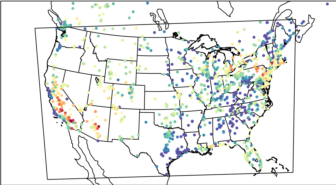
AirNOW (2023-07-01_03:00:00)
