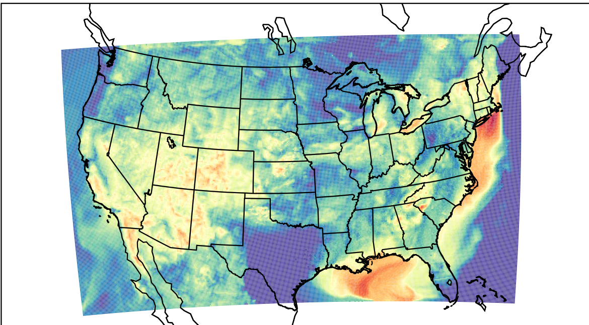
WRF (2023-07-01_11:00:00)
