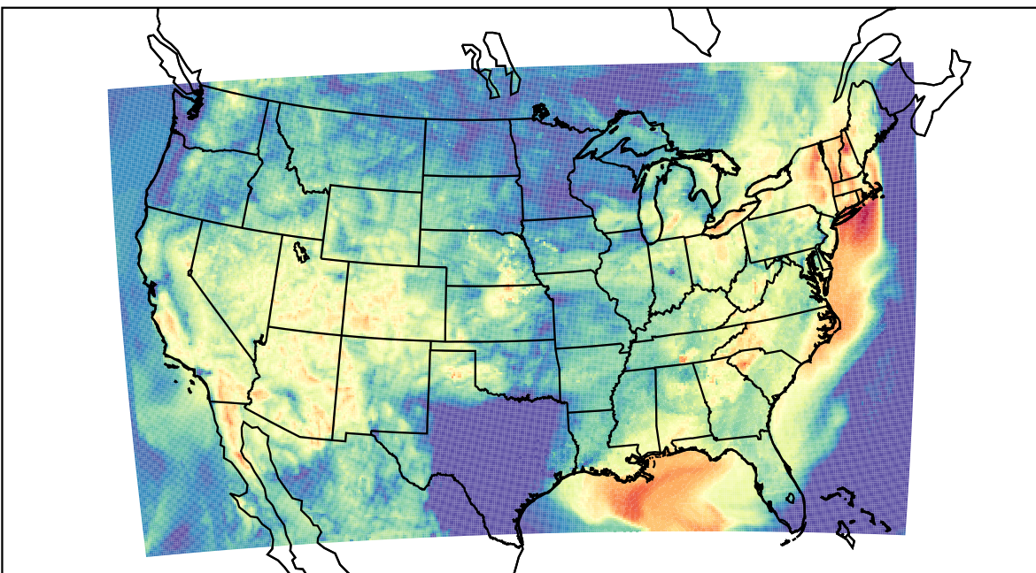
WRF (2023-07-01_13:00:00)
