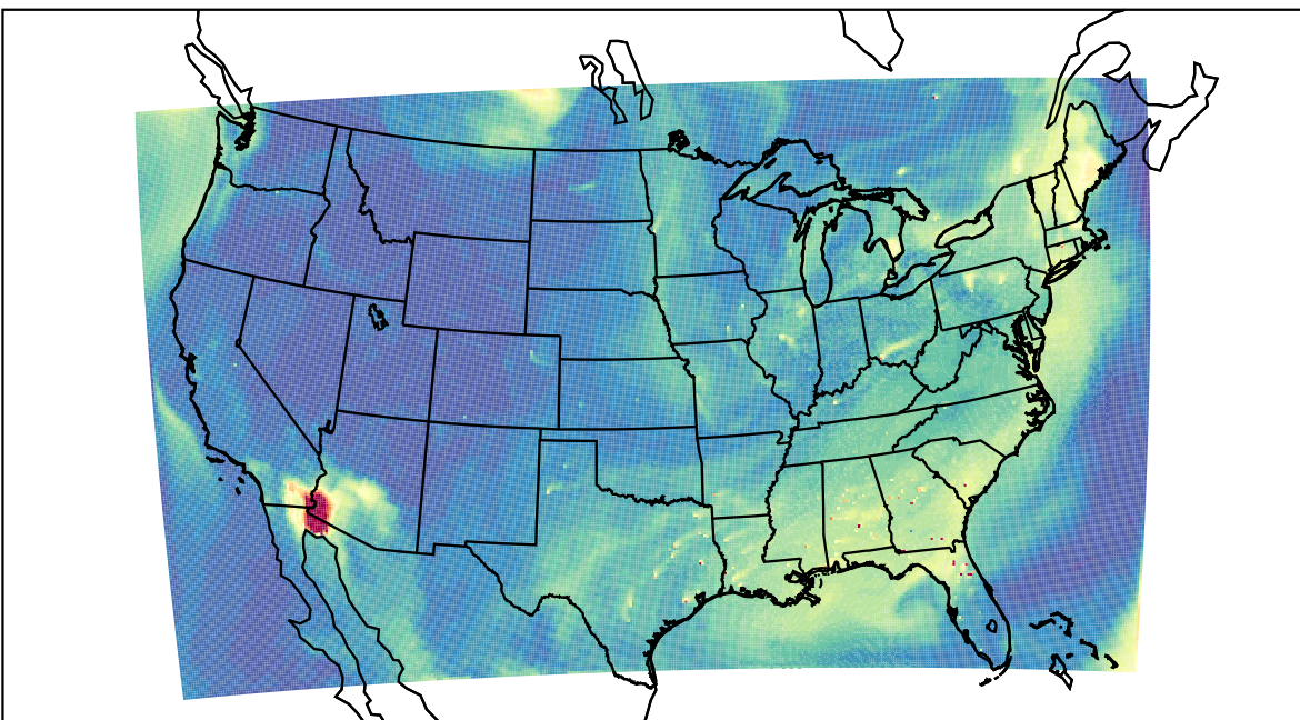
WRF 2023-07-02_19:00:00
