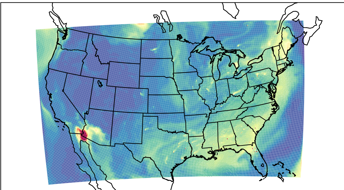
WRF 2023-07-02_18:00:00
