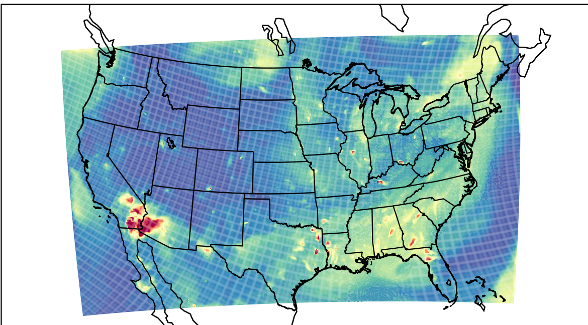
WRF 2023-07-03_04:00:00
