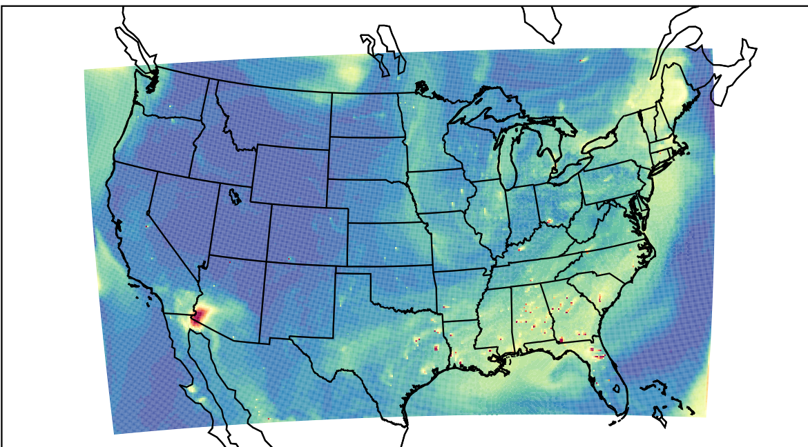
WRF 2023-07-02_23:00:00
