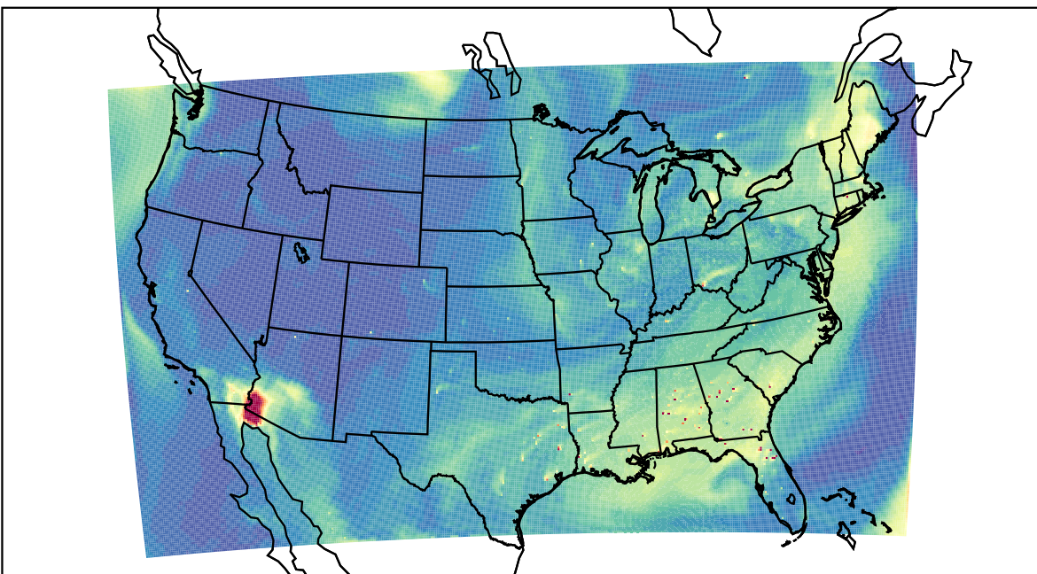
WRF 2023-07-02_20:00:00
