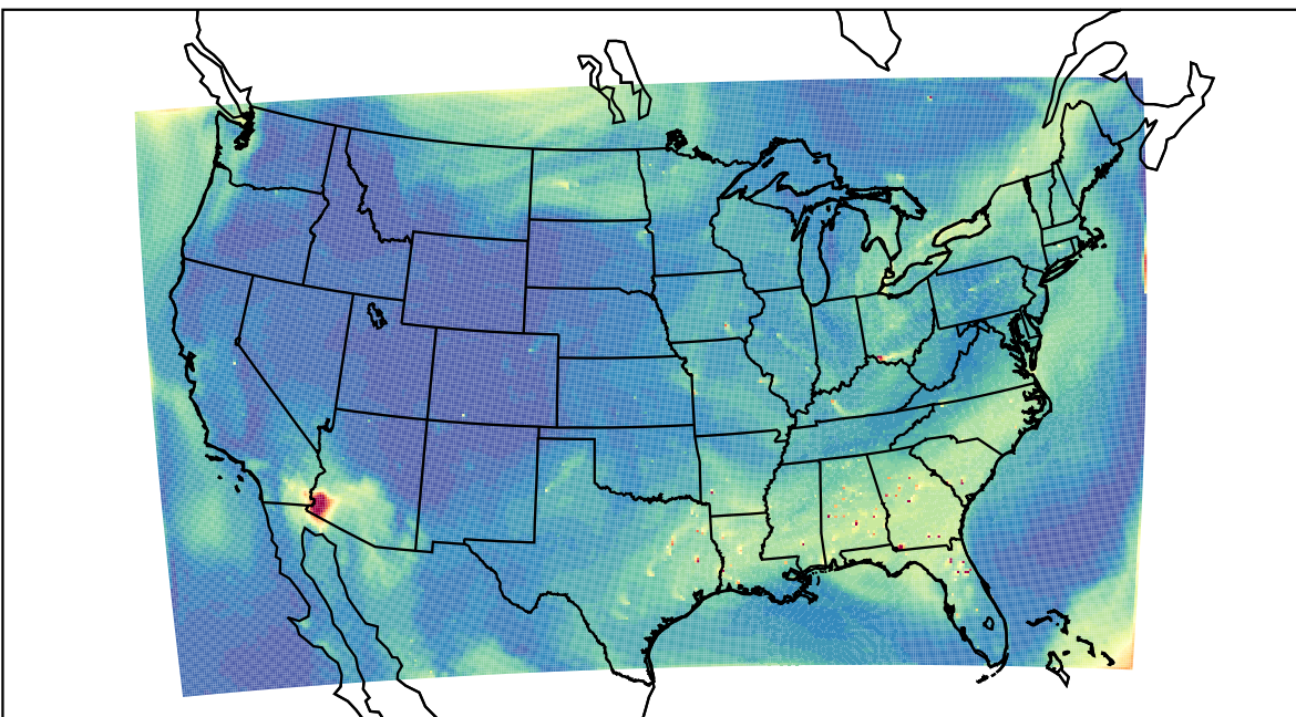
WRF 2023-07-03_20:00:00
