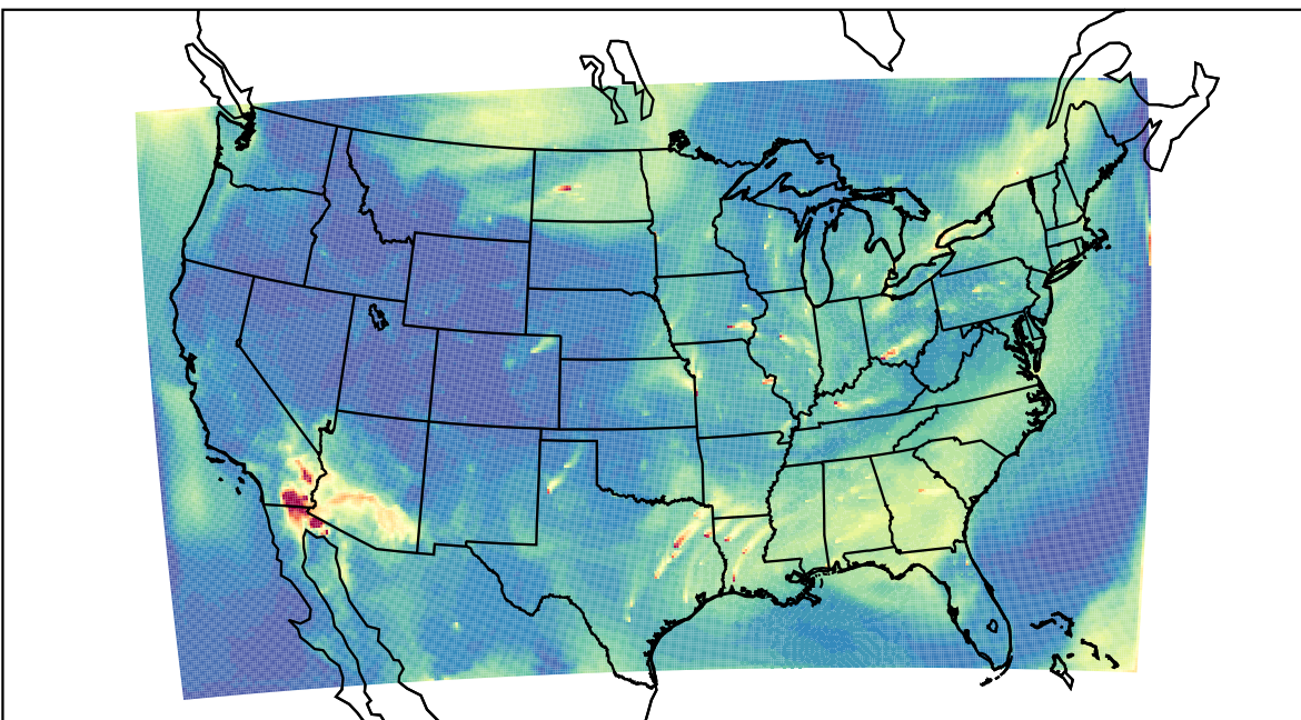
WRF 2023-07-03_14:00:00
