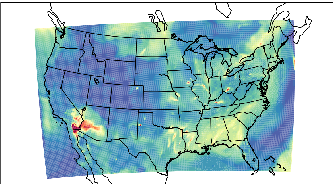
WRF 2023-07-03_10:00:00
