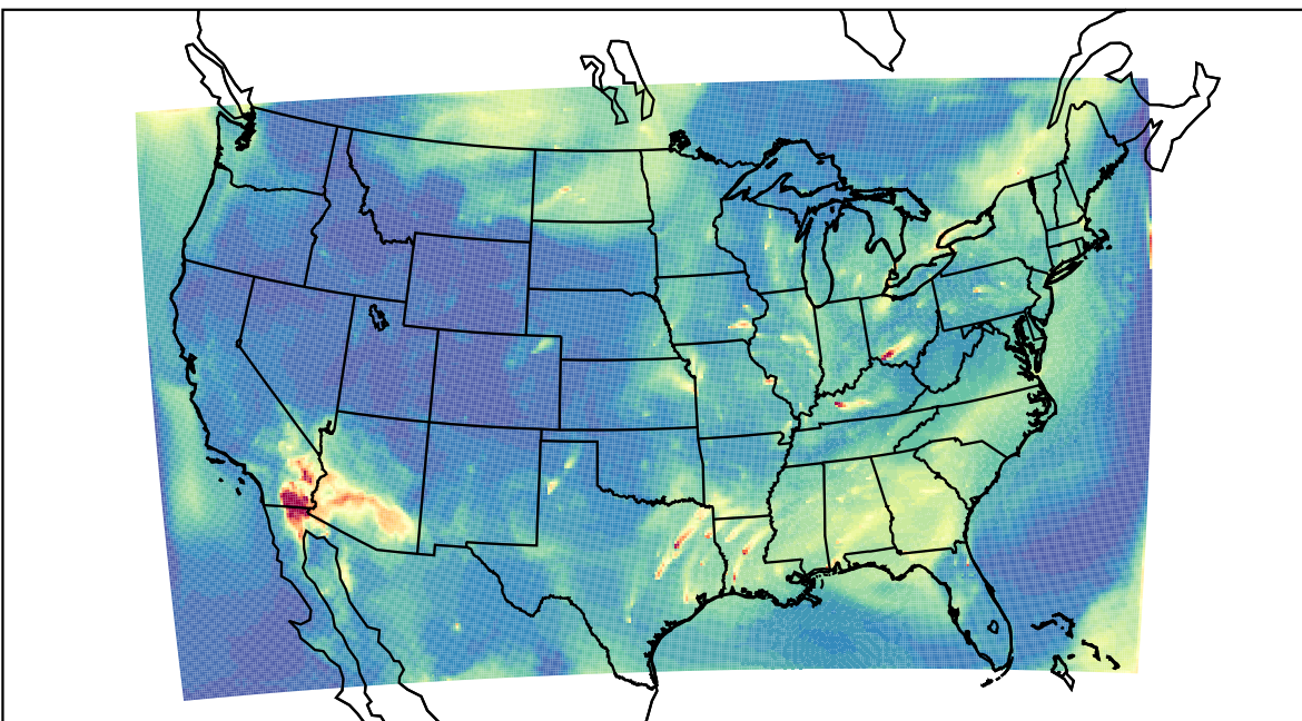
WRF 2023-07-03_13:00:00
