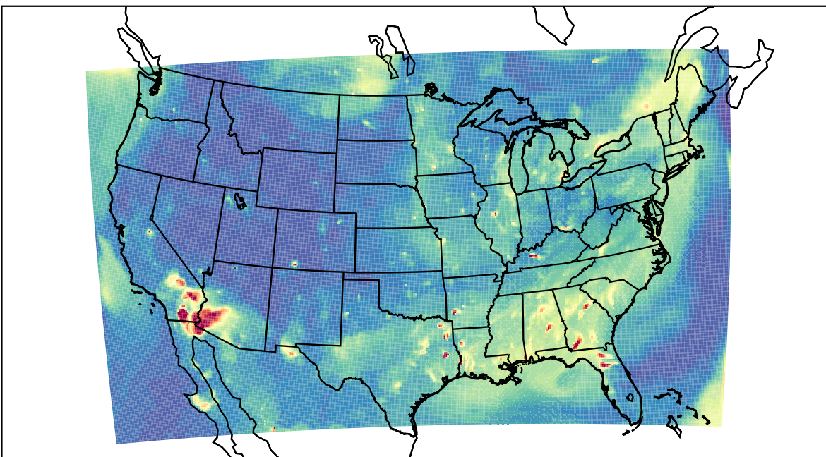
WRF 2023-07-03_03:00:00
