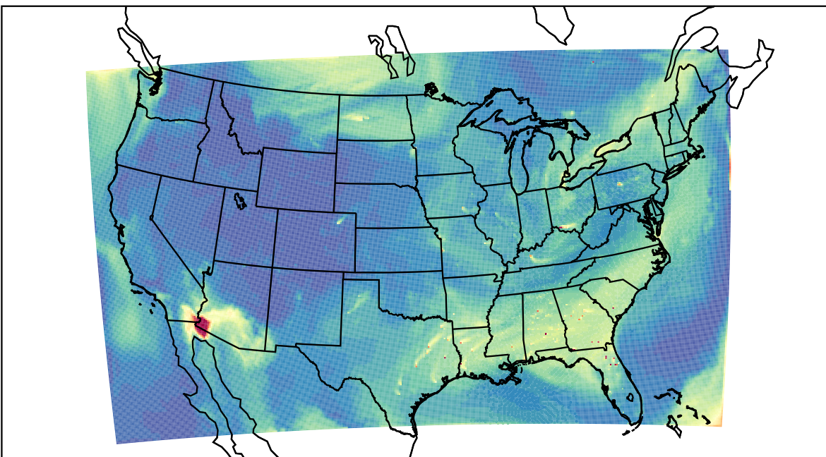
WRF 2023-07-03_18:00:00
