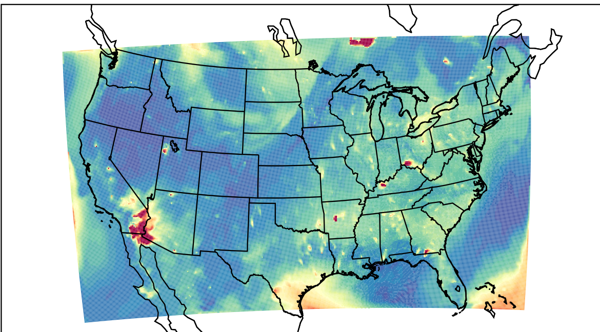
WRF 2023-07-05_03:00:00
