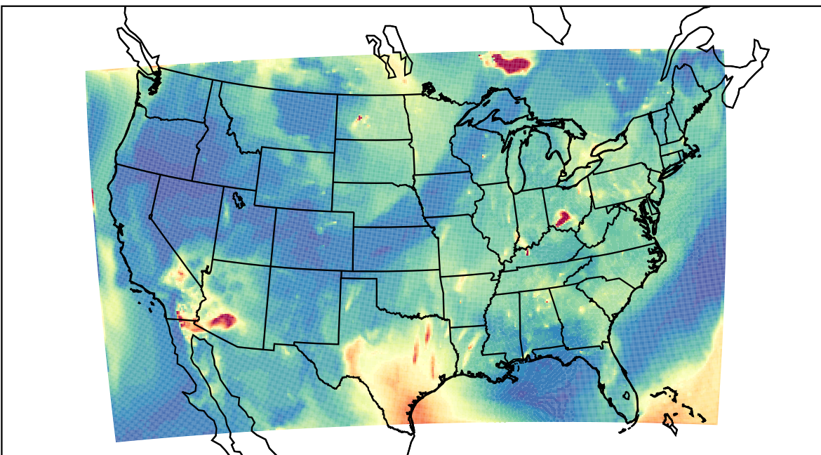
WRF 2023-07-05_10:00:00
