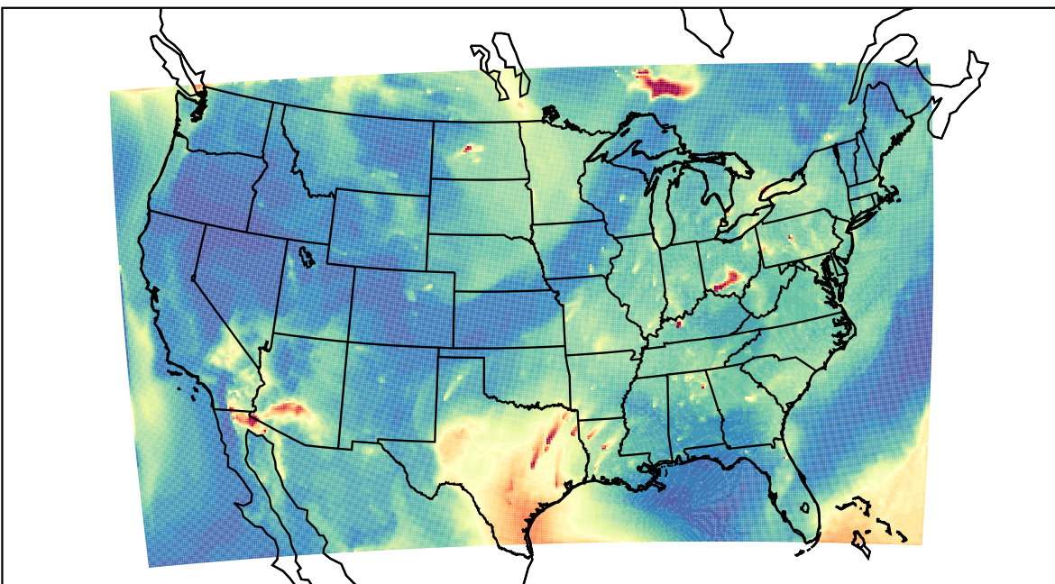
WRF 2023-07-05_13:00:00
