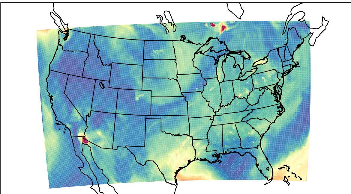
WRF 2023-07-05_18:00:00
