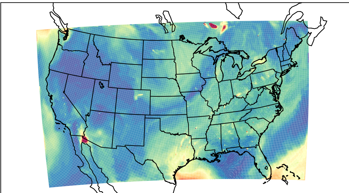
WRF 2023-07-05_20:00:00
