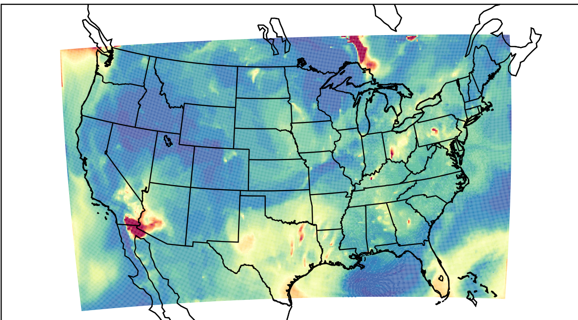
WRF 2023-07-06_10:00:00
