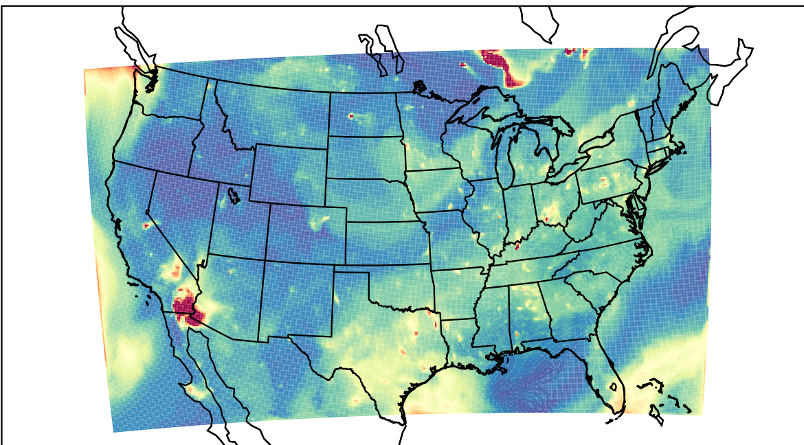
WRF 2023-07-06_03:00:00
