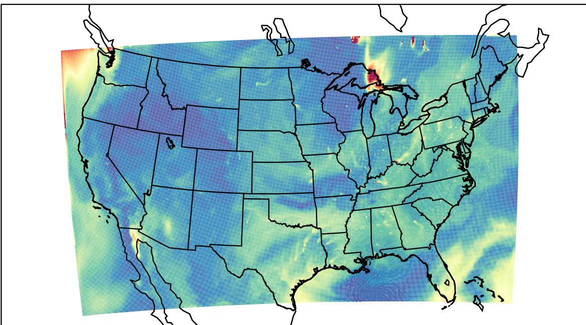
WRF 2023-07-06_20:00:00
