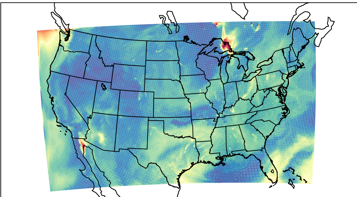
WRF 2023-07-06_18:00:00
