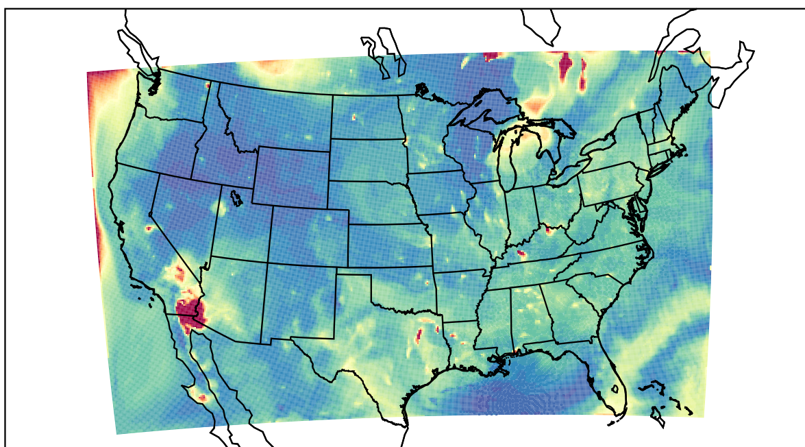
WRF 2023-07-07_04:00:00
