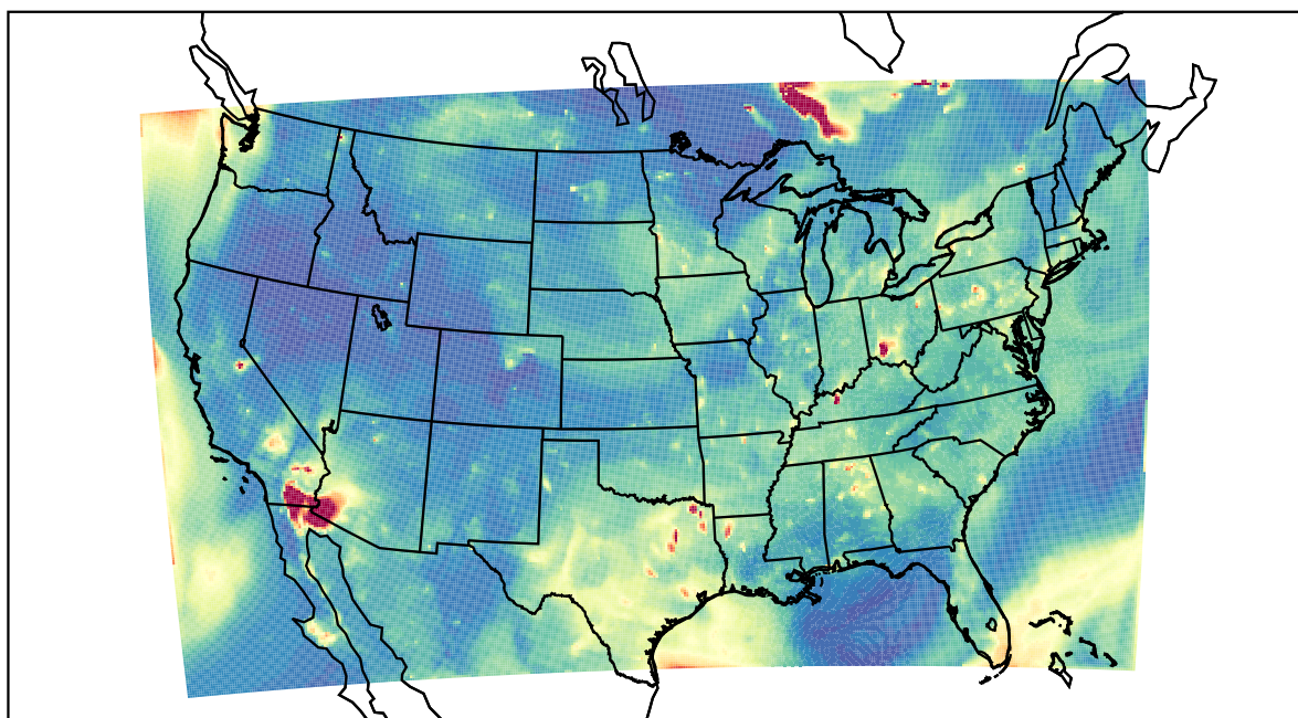
WRF 2023-07-06_03:00:00
