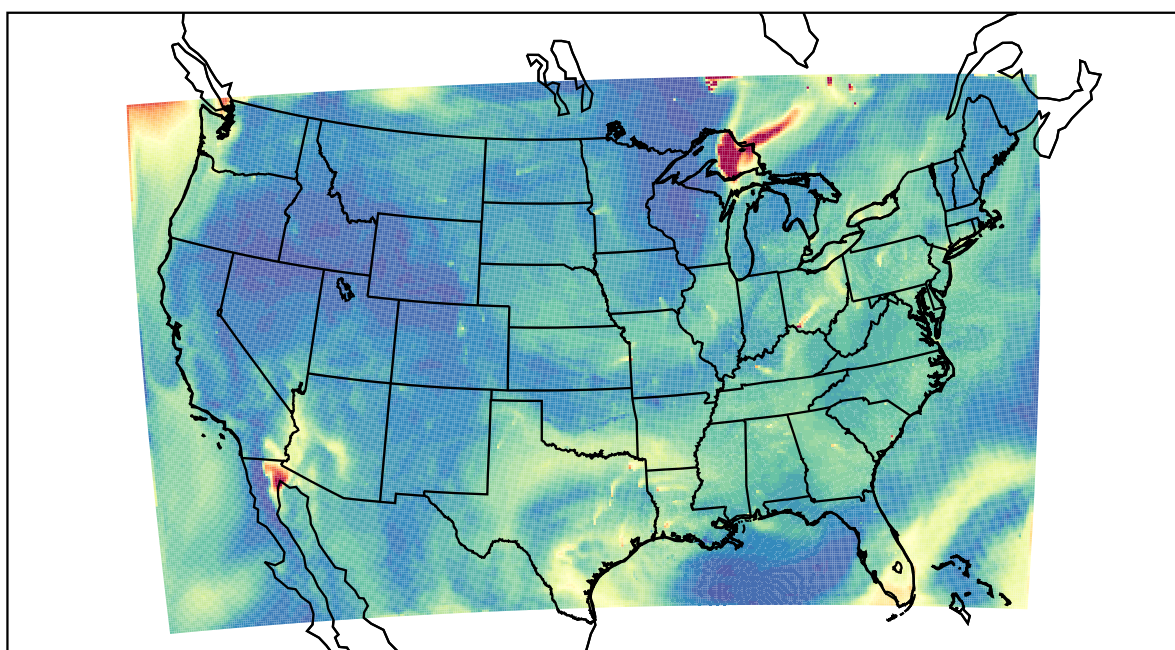
WRF 2023-07-06_18:00:00
