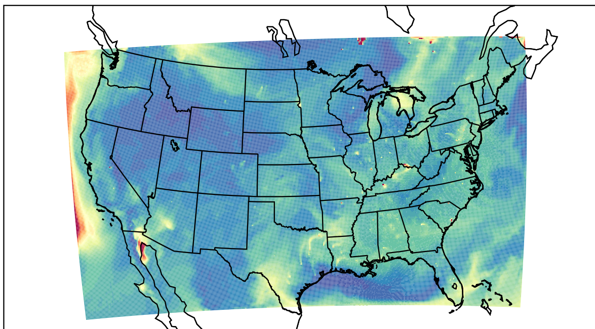
WRF 2023-07-07_20:00:00
