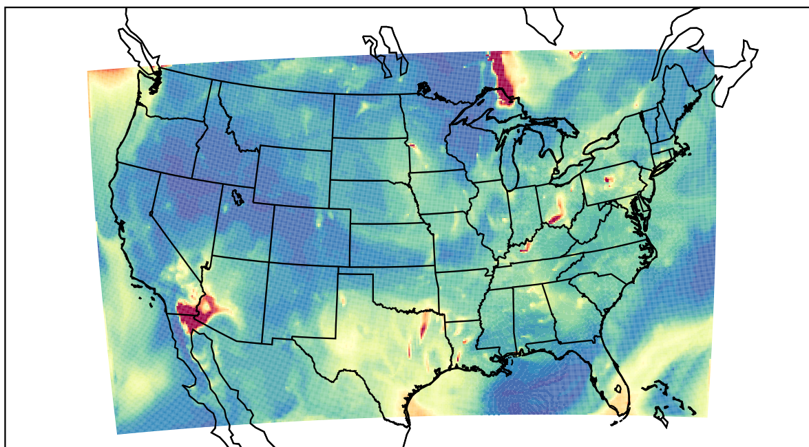
WRF 2023-07-06_10:00:00
