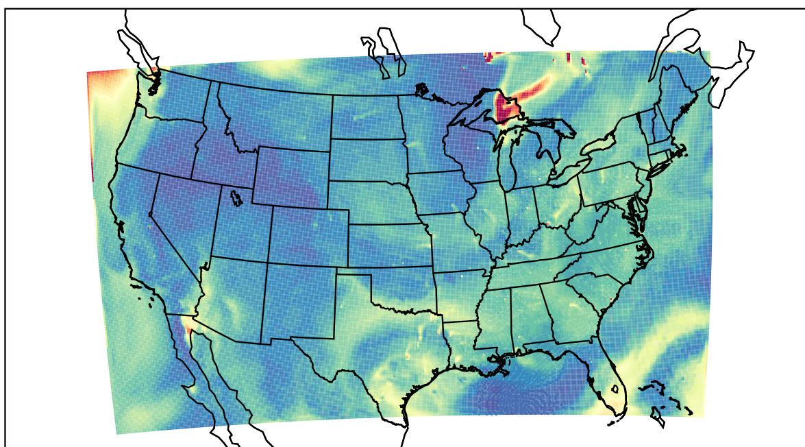
WRF 2023-07-06_20:00:00
