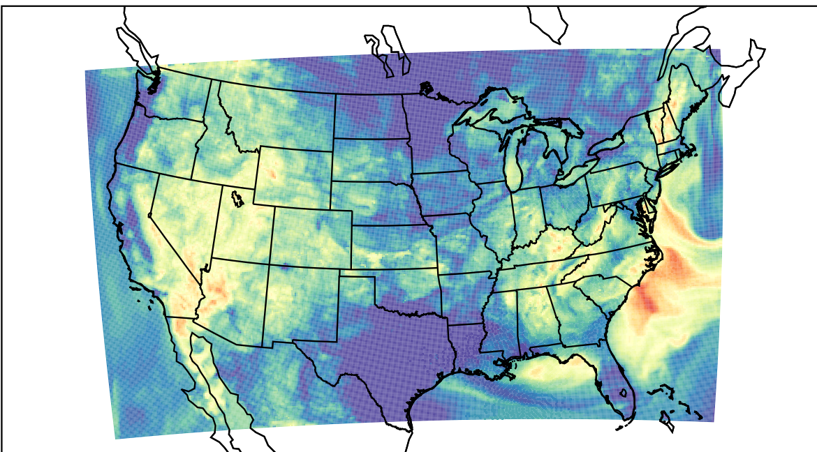
WRF (2023-07-08_10:00:00)
