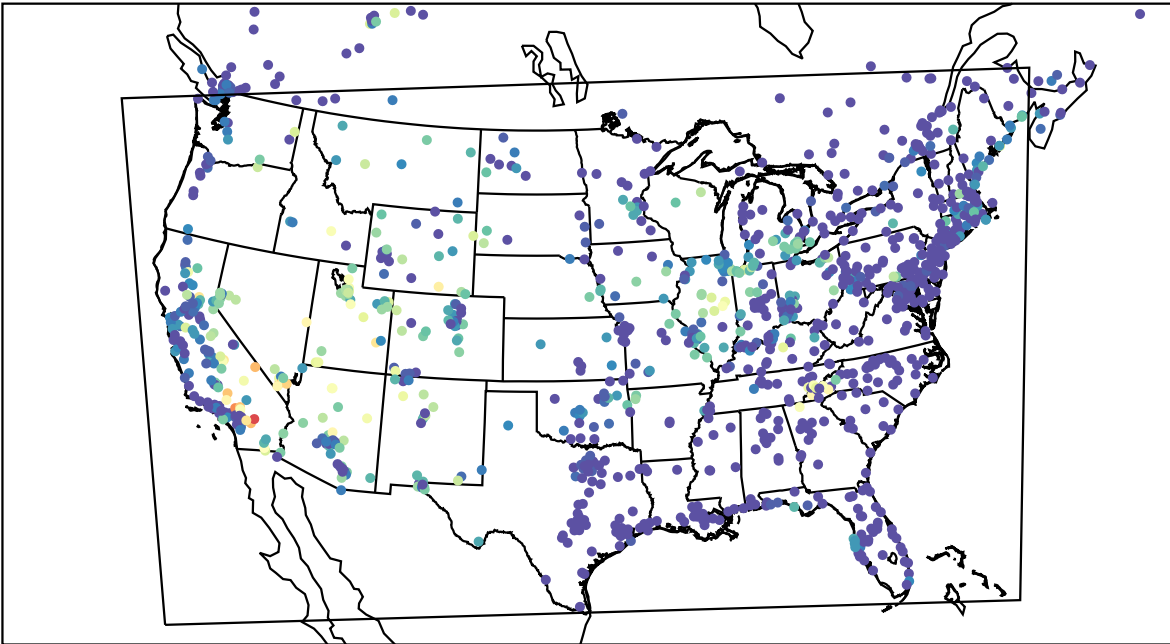
AirNOW (2023-07-08_10:00:00)
