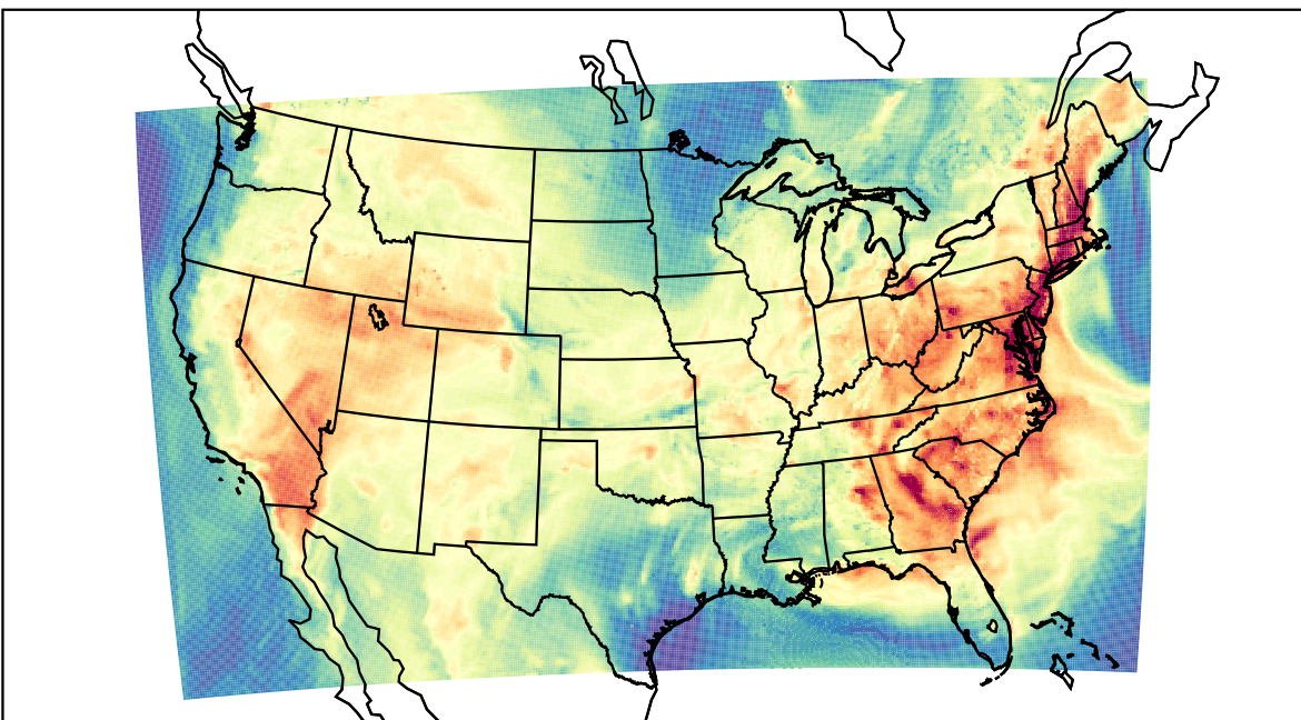
WRF (2023-07-08_19:00:00)
