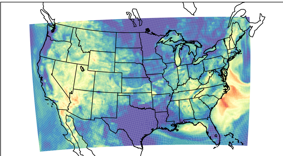
WRF (2023-07-08_11:00:00)
