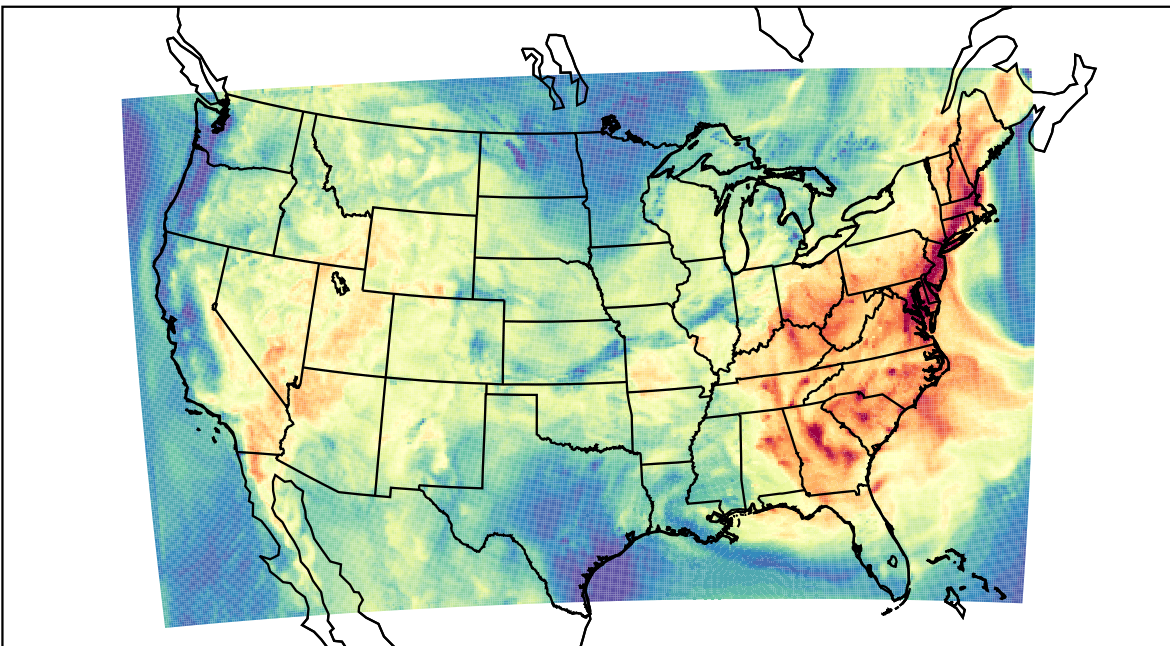
WRF (2023-07-08_16:00:00)
