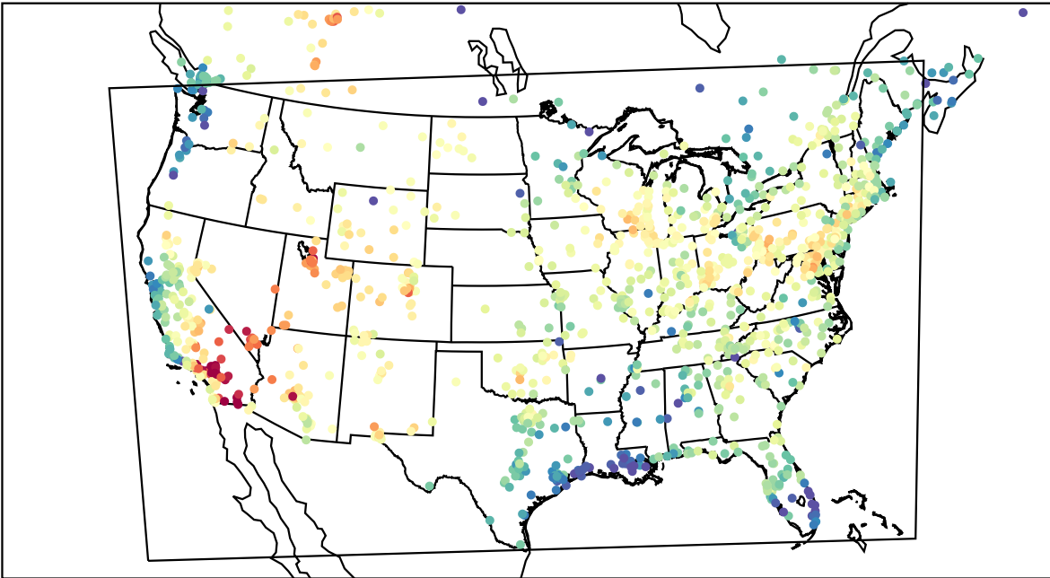
AirNOW (2023-07-08_20:00:00)
