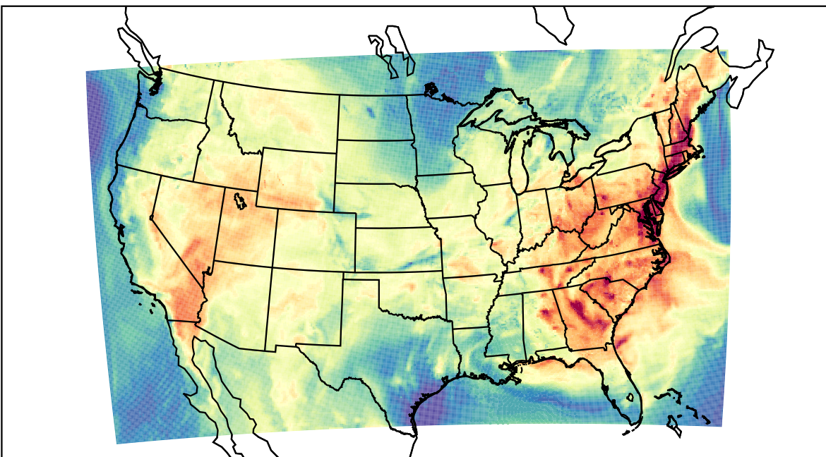
WRF (2023-07-08_18:00:00)
