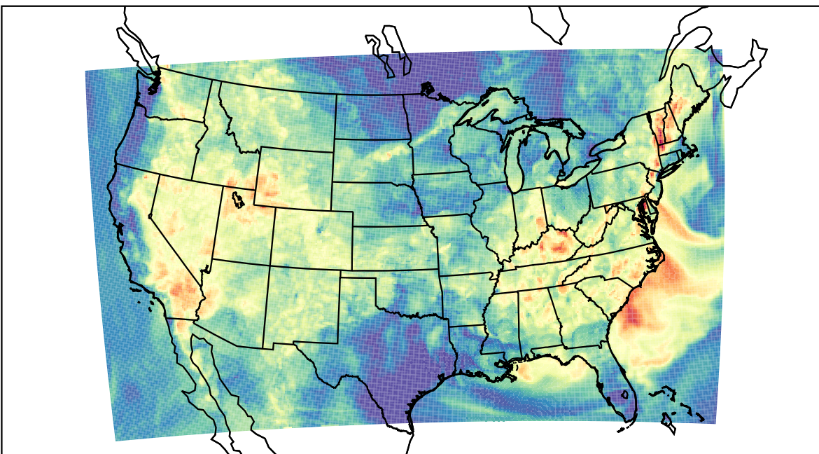
WRF (2023-07-08_04:00:00)
