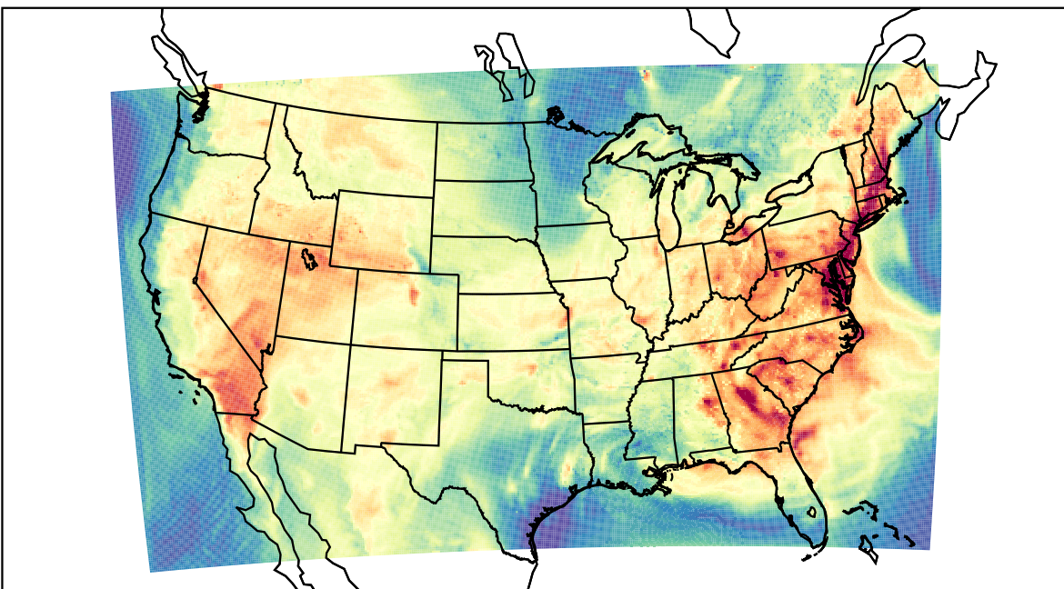
WRF (2023-07-08_20:00:00)
