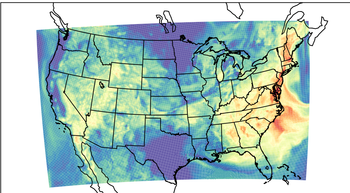
WRF (2023-07-08_14:00:00)
