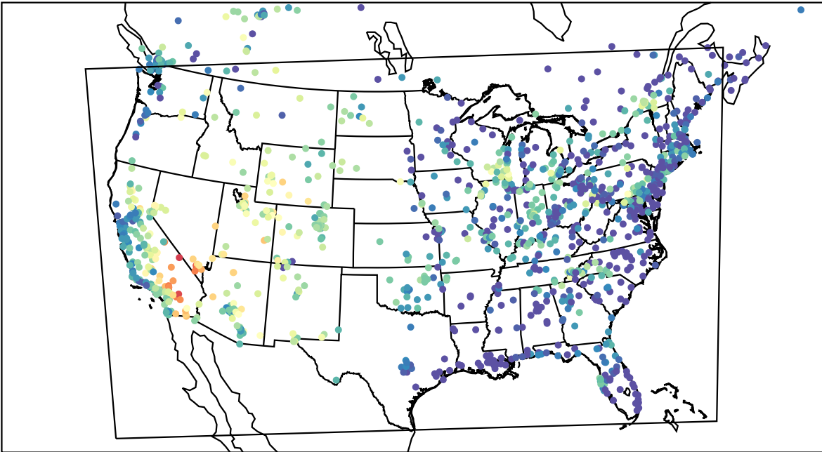
AirNOW (2023-07-09_04:00:00)
