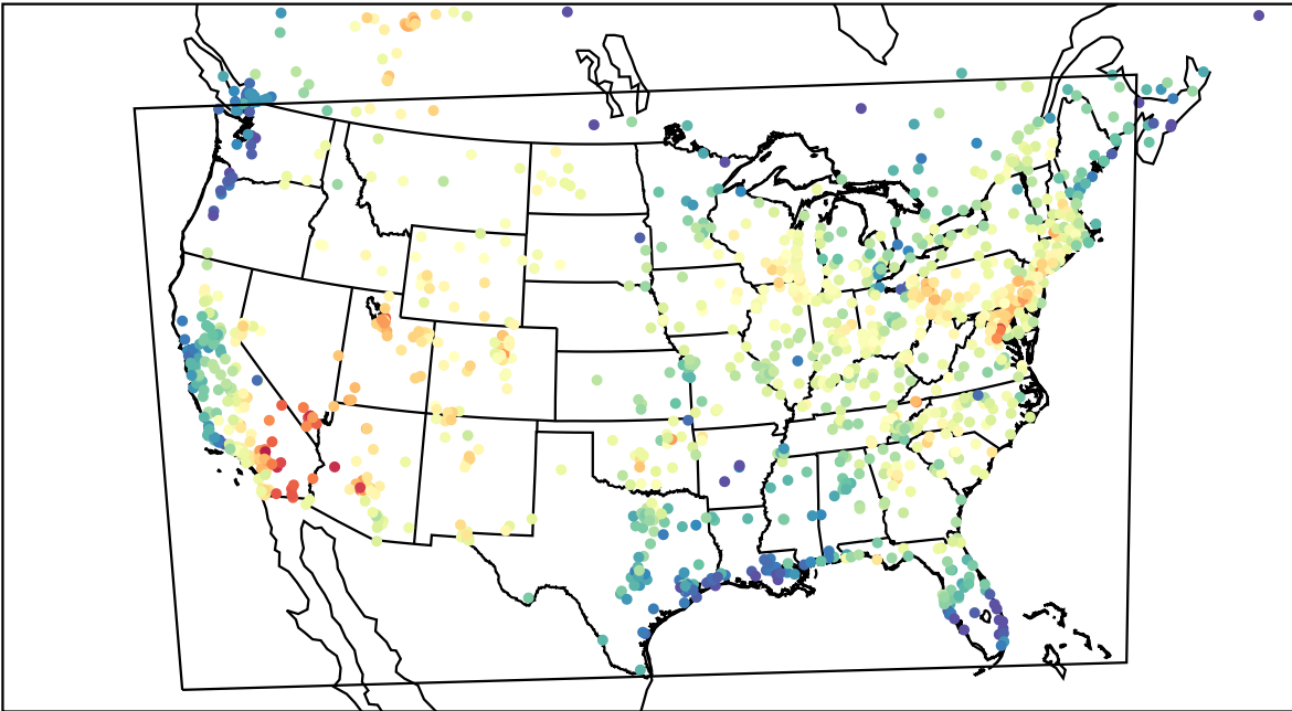
AirNOW (2023-07-08_18:00:00)
