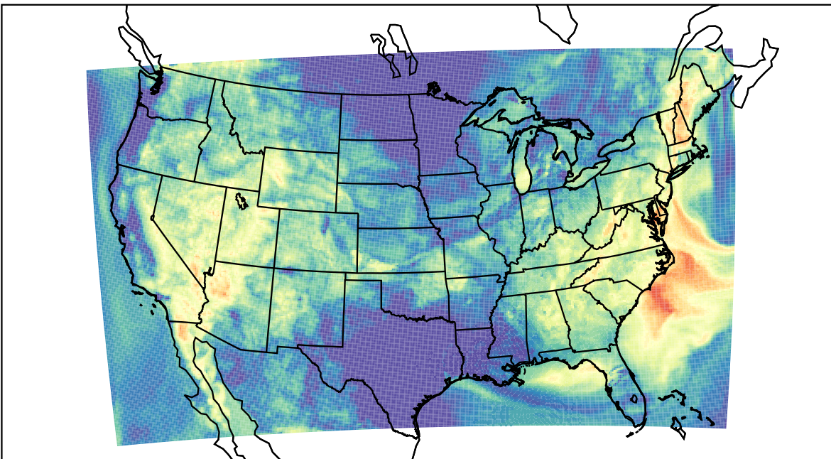
WRF (2023-07-08_13:00:00)
