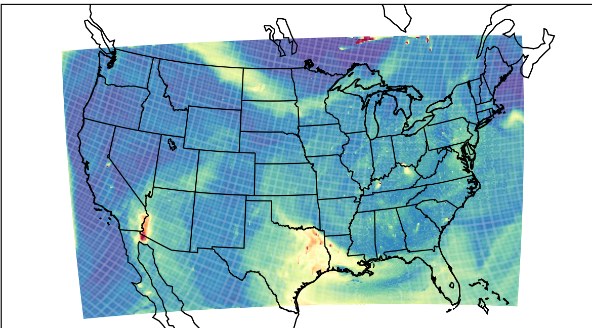
WRF 2023-07-10_23:00:00
