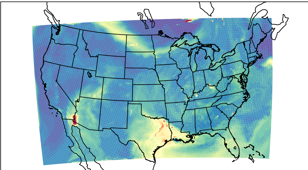
WRF 2023-07-10_20:00:00
