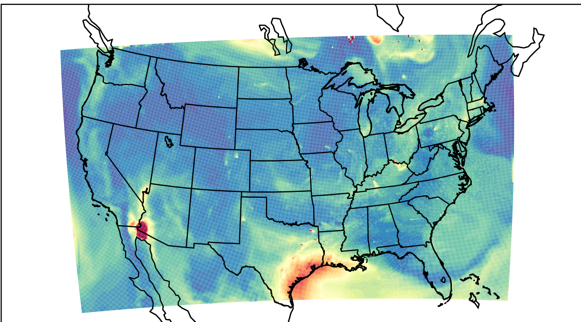
WRF 2023-07-09_18:00:00
