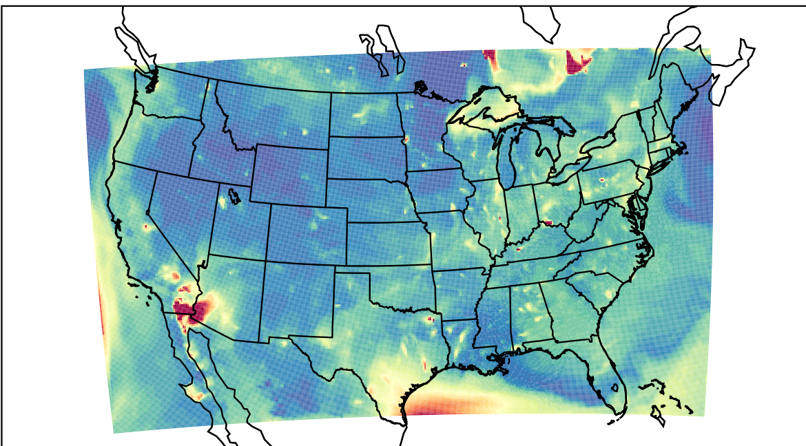
WRF 2023-07-09_04:00:00
