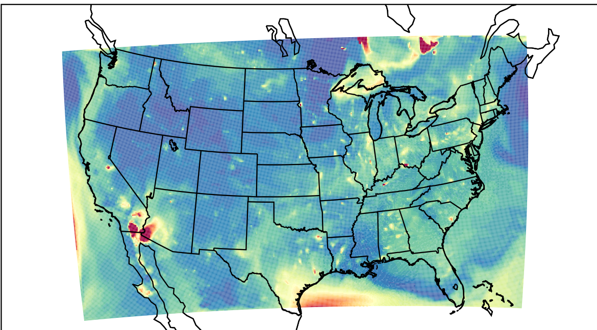
WRF 2023-07-09_03:00:00
