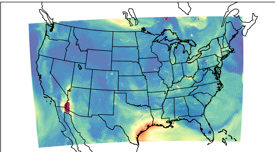
WRF 2023-07-09_20:00:00
