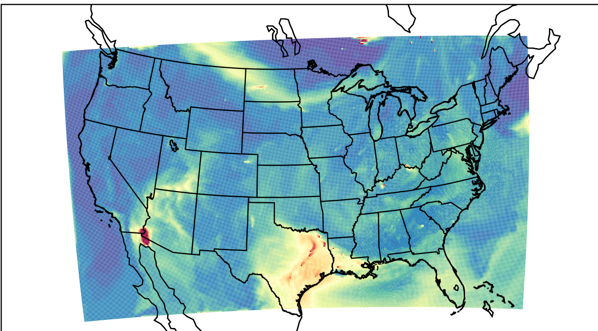
WRF 2023-07-10_18:00:00
