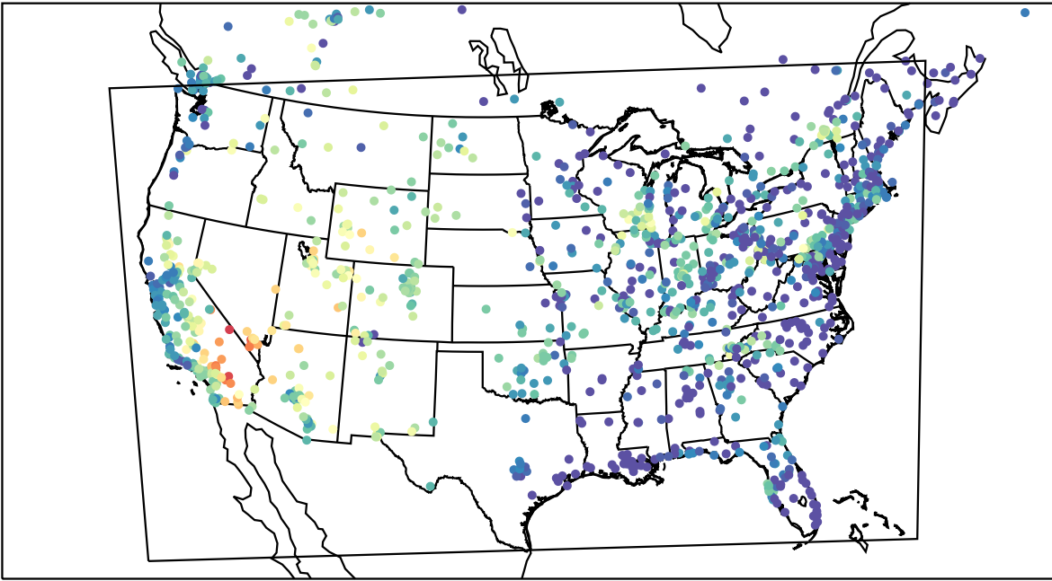
AirNOW (2023-07-09_04:00:00)
