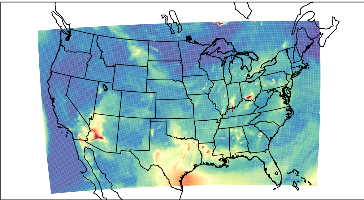
WRF 2023-07-11_11:00:00
