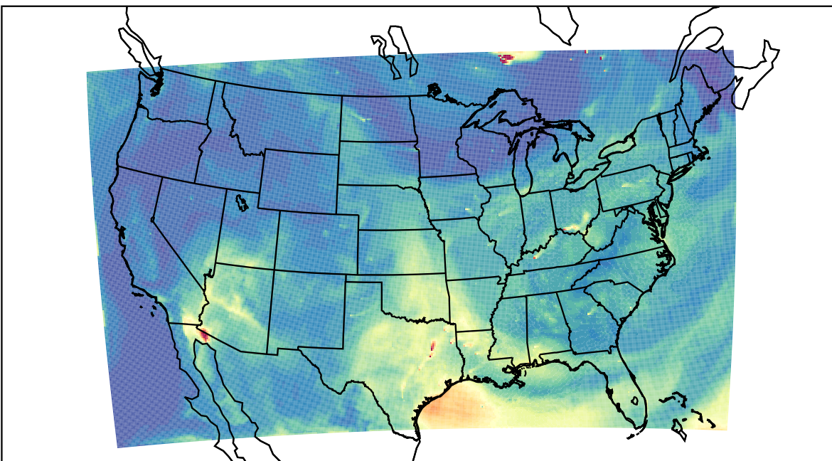
WRF 2023-07-11_18:00:00
