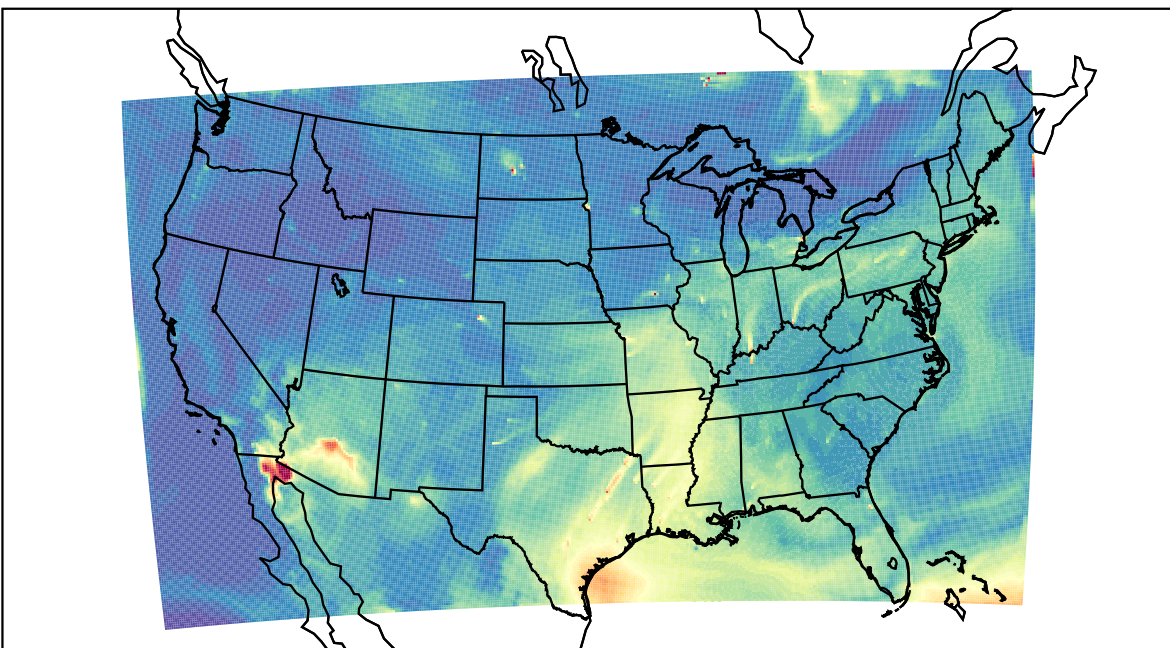
WRF 2023-07-12_16:00:00
