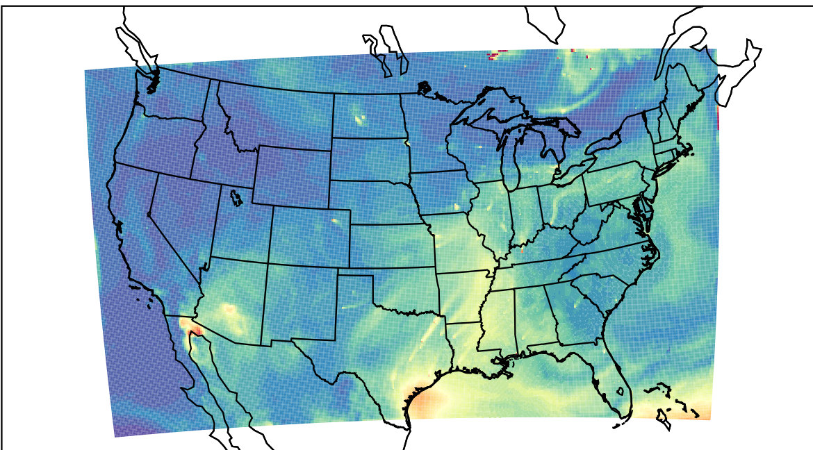
WRF 2023-07-12_18:00:00
