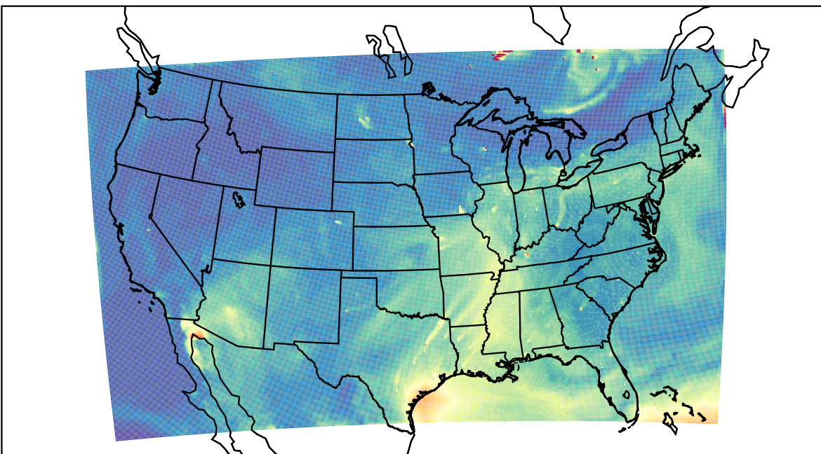
WRF 2023-07-12_19:00:00
