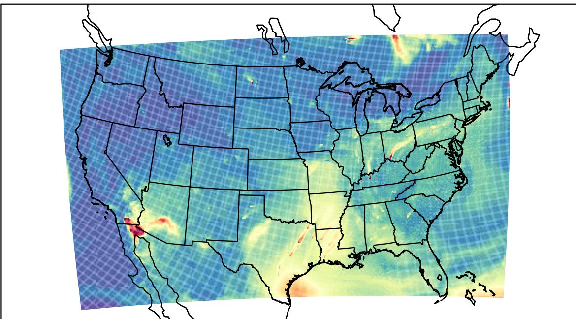
WRF 2023-07-12_14:00:00
