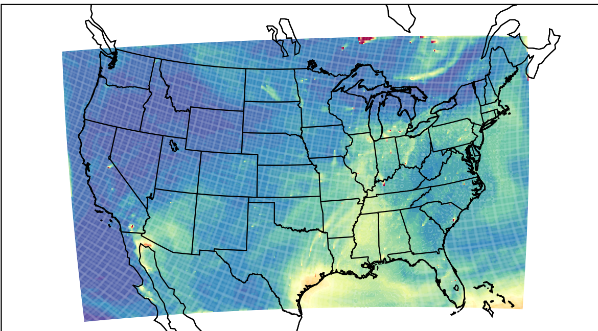
WRF 2023-07-12_23:00:00
