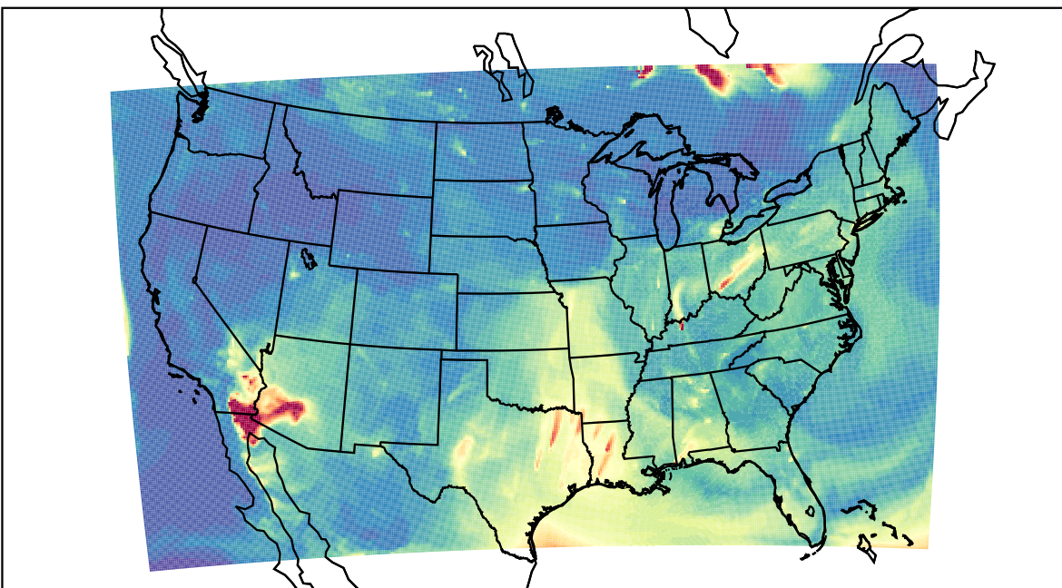
WRF 2023-07-12_10:00:00
