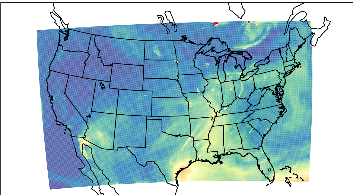
WRF 2023-07-12_20:00:00
