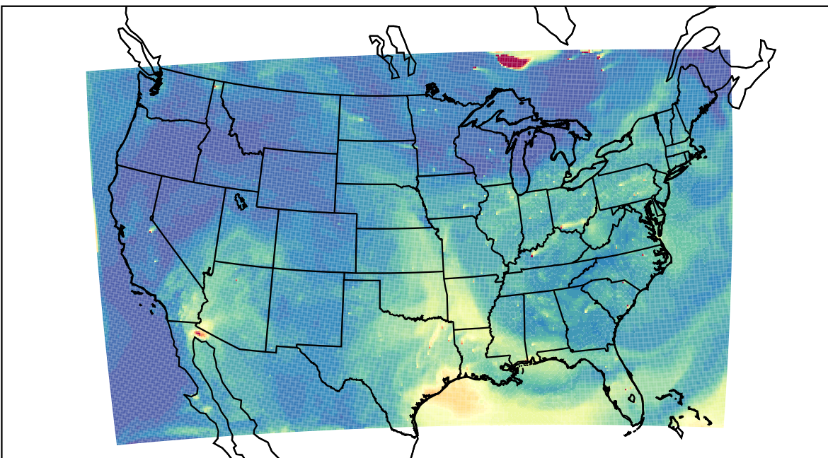
WRF 2023-07-11_23:00:00
