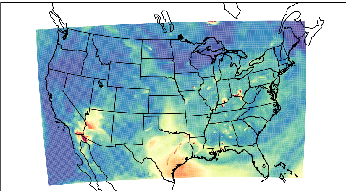
WRF 2023-07-11_14:00:00
