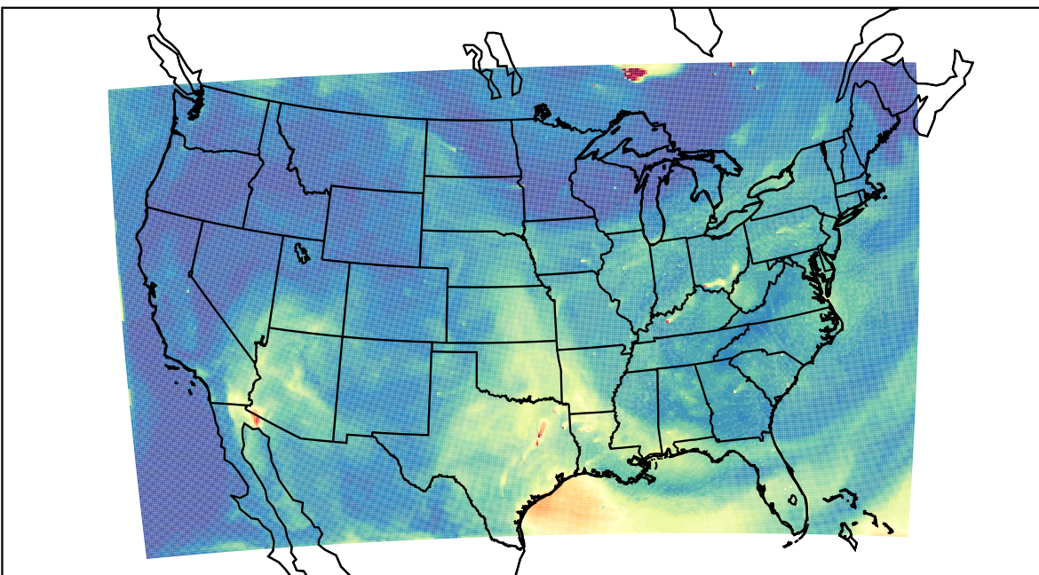
WRF 2023-07-11_19:00:00
