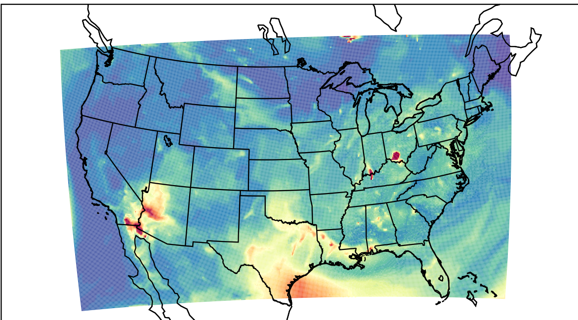
WRF 2023-07-11_11:00:00
