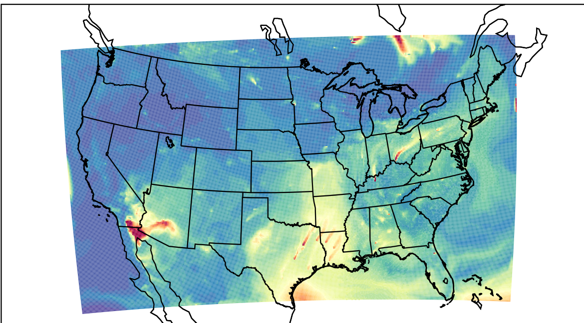
WRF 2023-07-12_13:00:00
