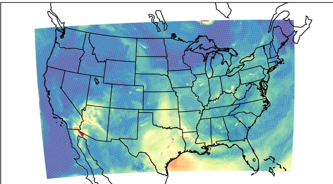
WRF 2023-07-11_16:00:00
