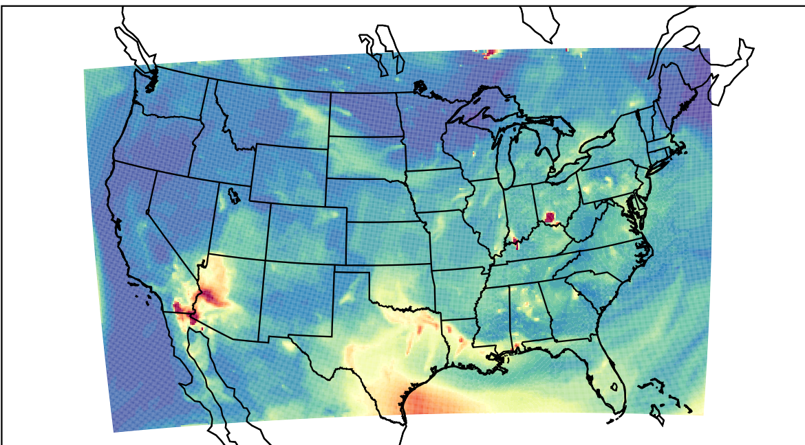
WRF 2023-07-11_10:00:00
