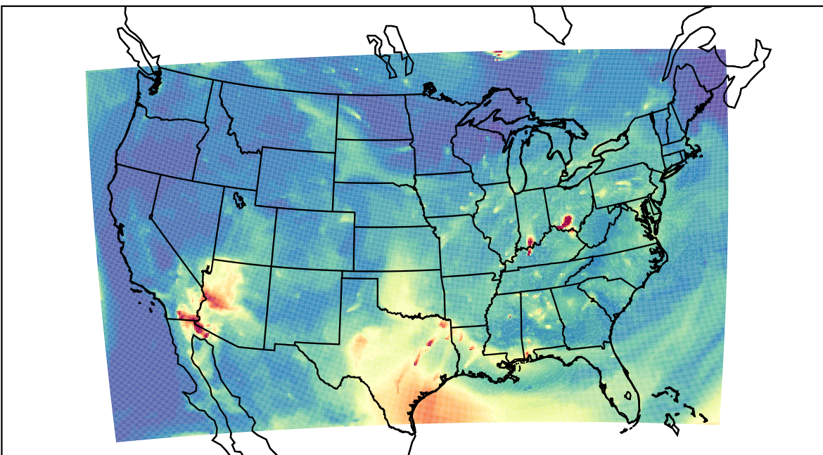
WRF 2023-07-11_13:00:00
