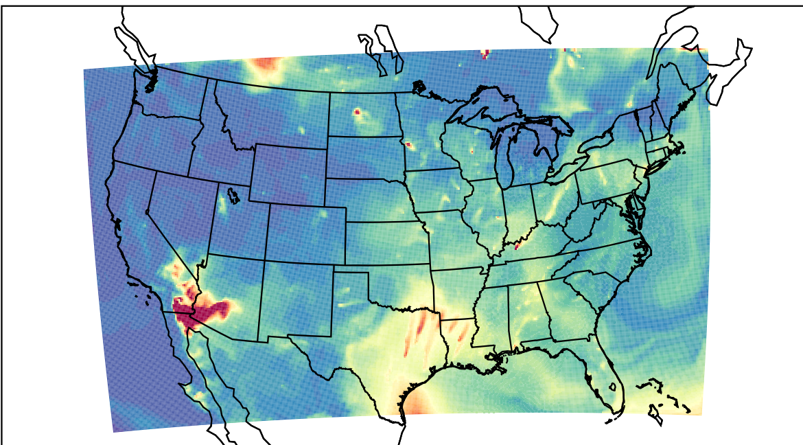
WRF 2023-07-13_10:00:00
