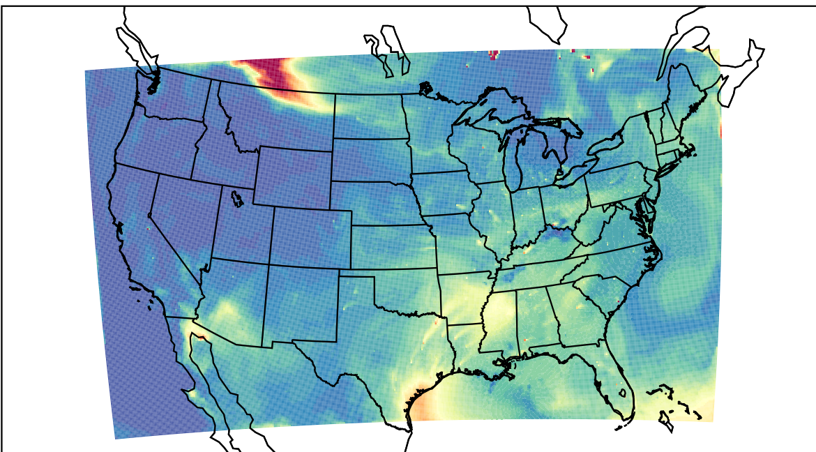
WRF 2023-07-13_20:00:00
