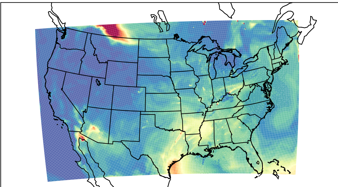
WRF 2023-07-13_18:00:00
