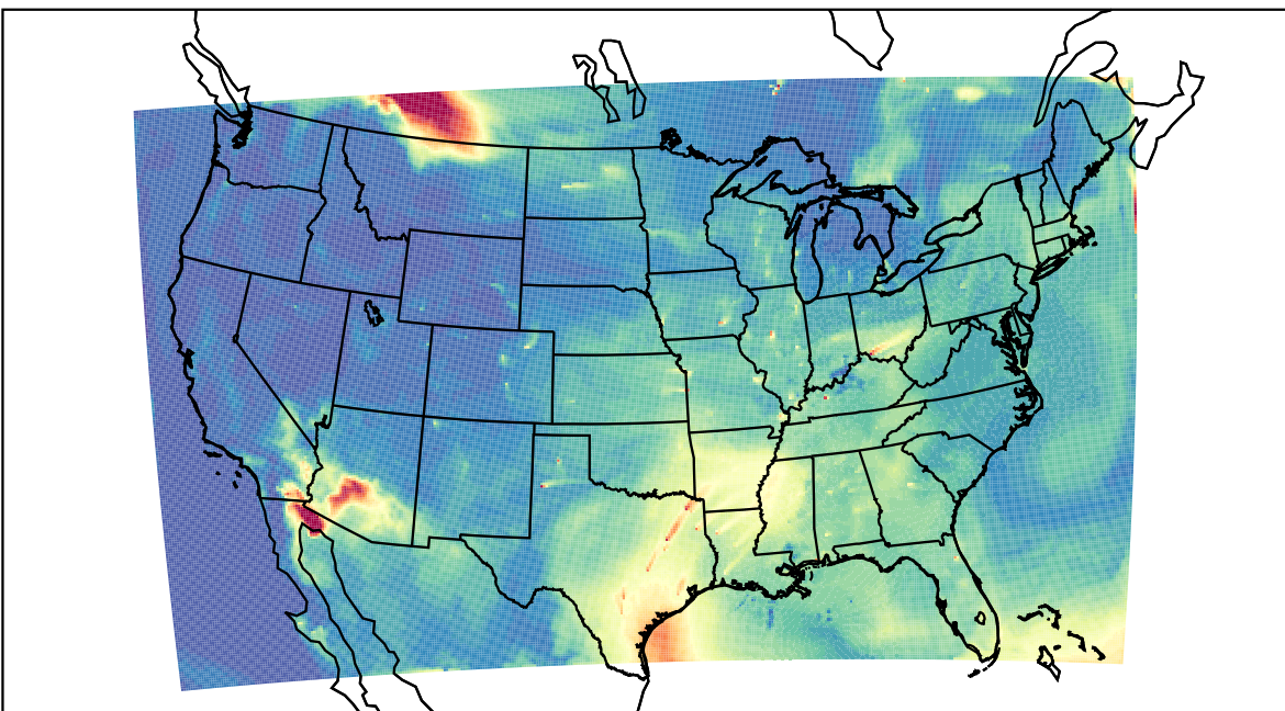
WRF 2023-07-13_16:00:00
