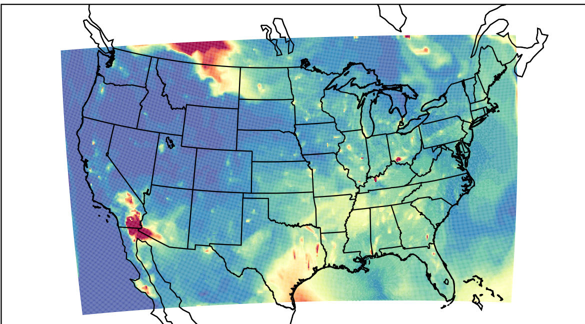
WRF 2023-07-14_04:00:00
