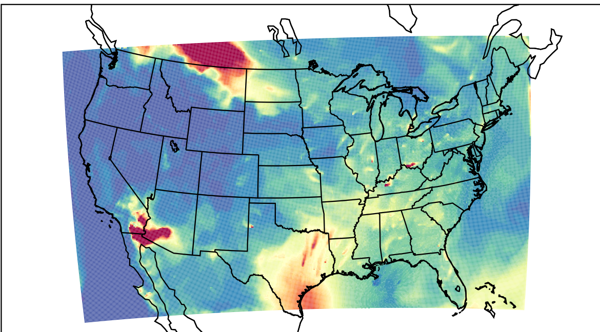
WRF 2023-07-14_10:00:00
