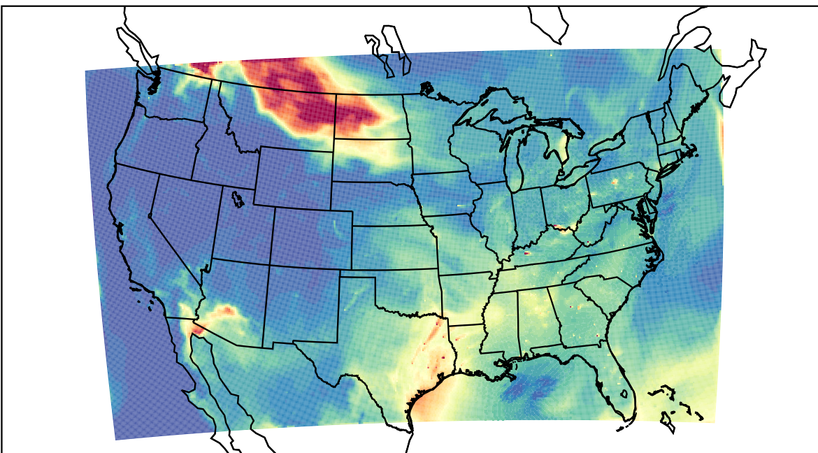
WRF 2023-07-14_18:00:00
