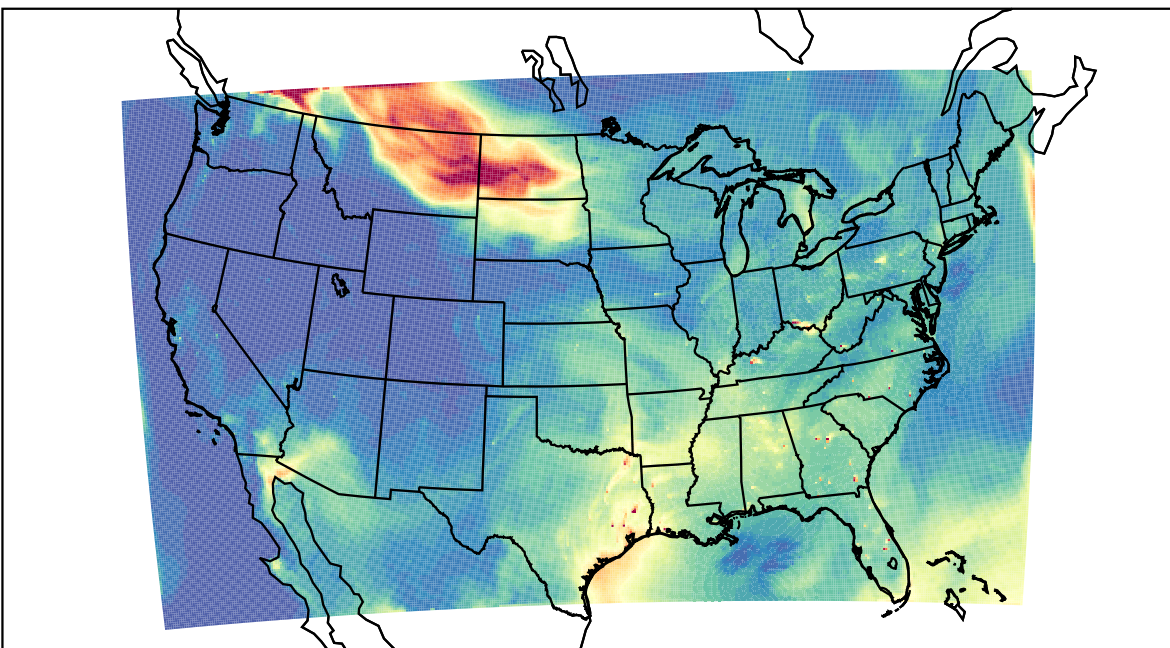
WRF 2023-07-14_20:00:00
