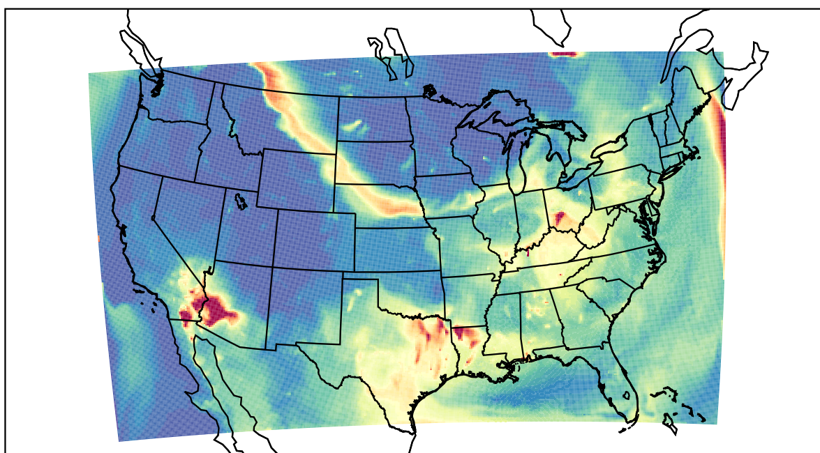
WRF 2023-07-17_08:00:00
