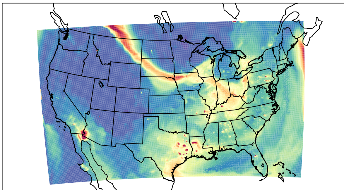
WRF 2023-07-17_01:00:00
