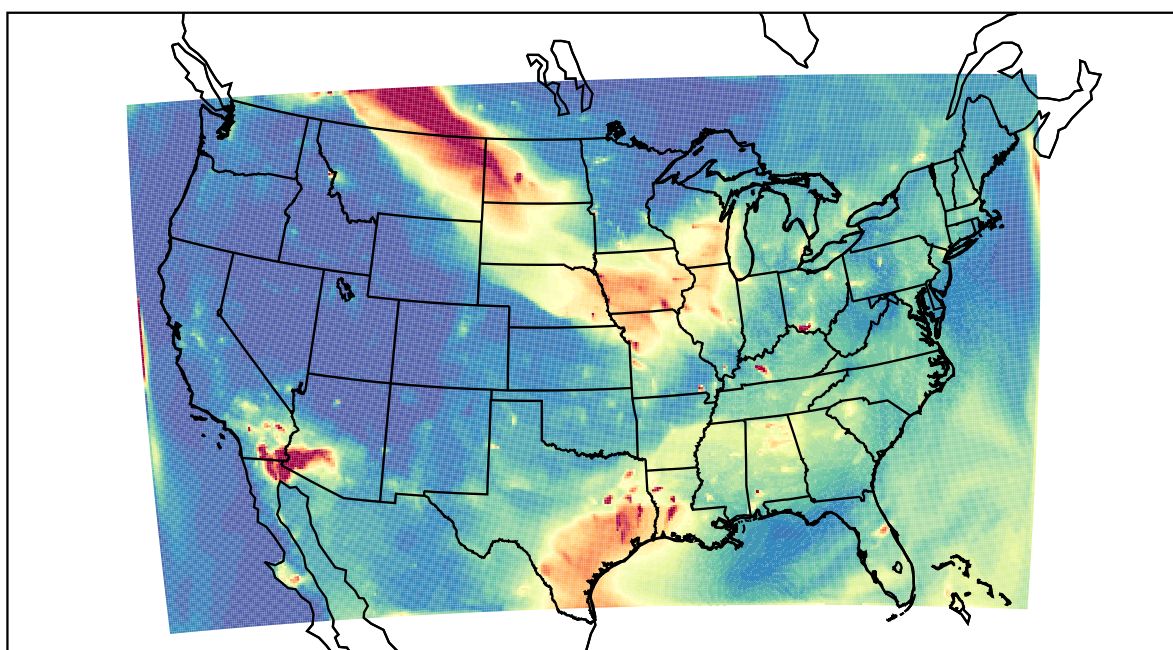
WRF 2023-07-16_04:00:00
