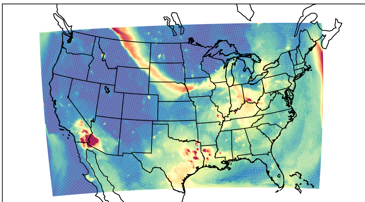
WRF 2023-07-17_04:00:00
