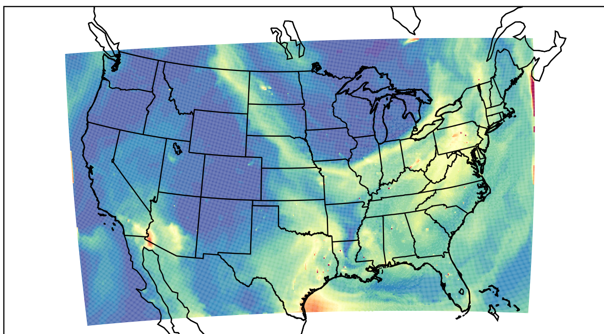
WRF 2023-07-17_20:00:00
