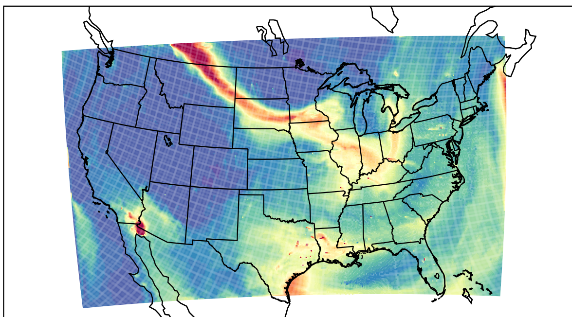
WRF 2023-07-16_20:00:00
