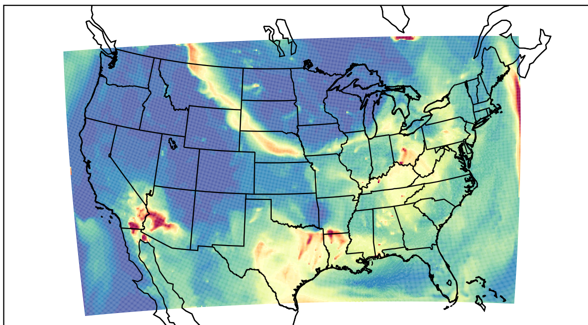
WRF 2023-07-17_10:00:00
