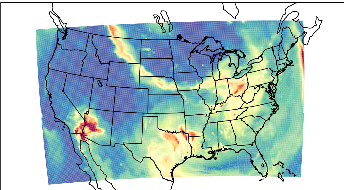
WRF 2023-07-17_10:00:00
