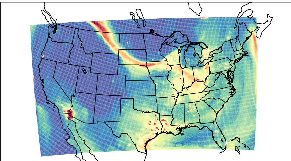
WRF 2023-07-17_01:00:00
