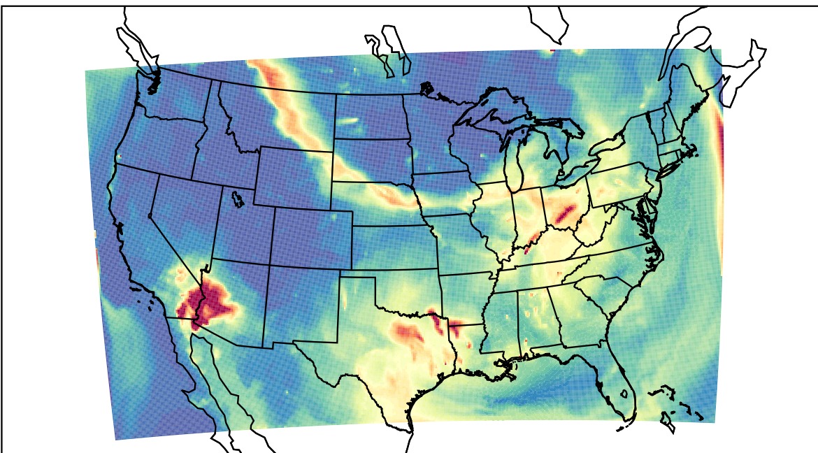
WRF 2023-07-17_08:00:00
