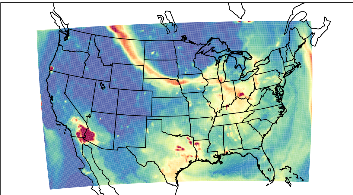
WRF 2023-07-17_04:00:00
