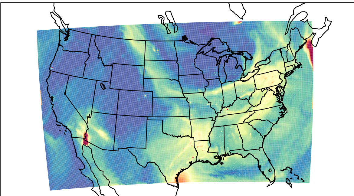
WRF 2023-07-17_20:00:00
