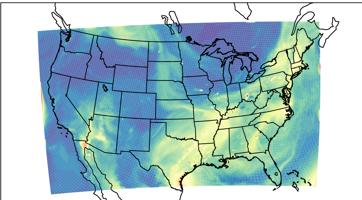
WRF 2023-07-18_18:00:00
