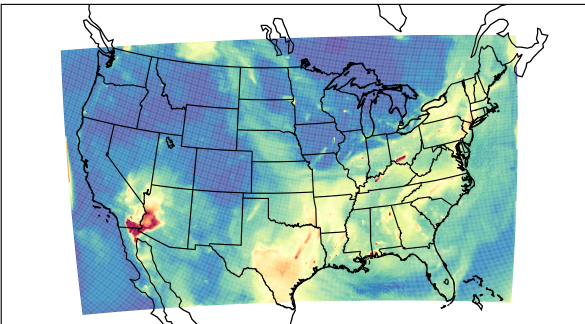
WRF 2023-07-18_10:00:00
