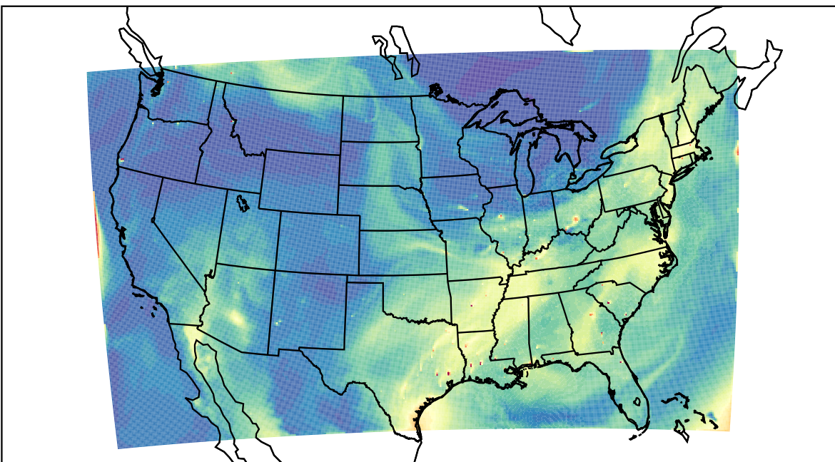
WRF 2023-07-18_20:00:00
