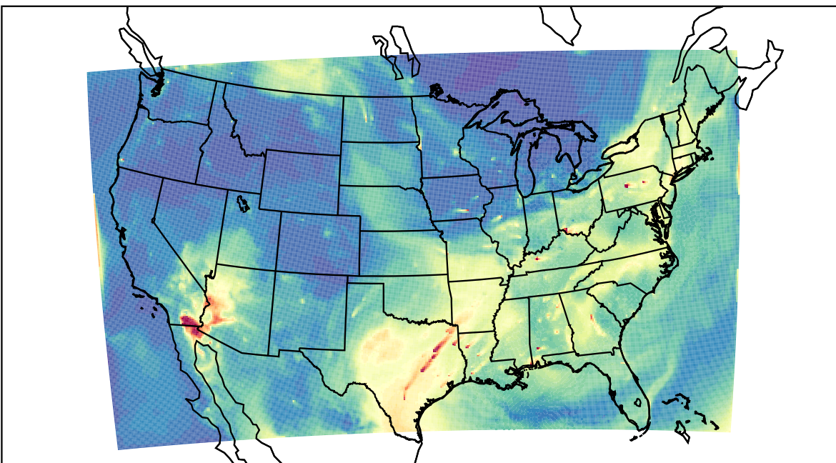
WRF 2023-07-18_14:00:00
