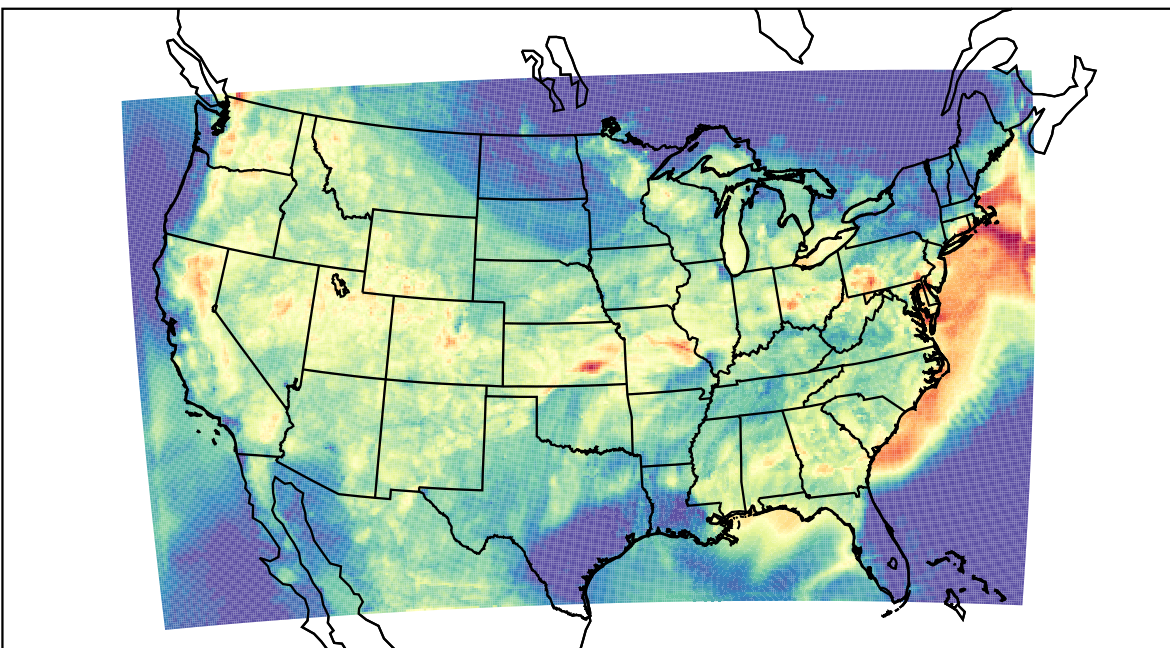
WRF (2023-07-20_04:00:00)
