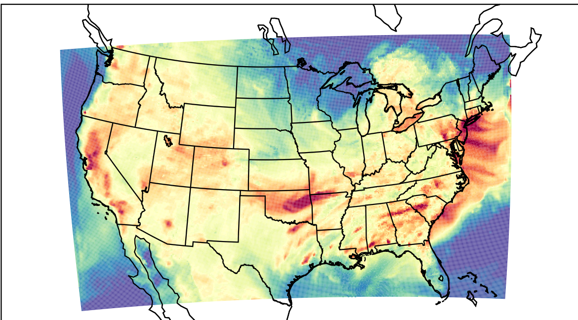
WRF (2023-07-20_23:00:00)
