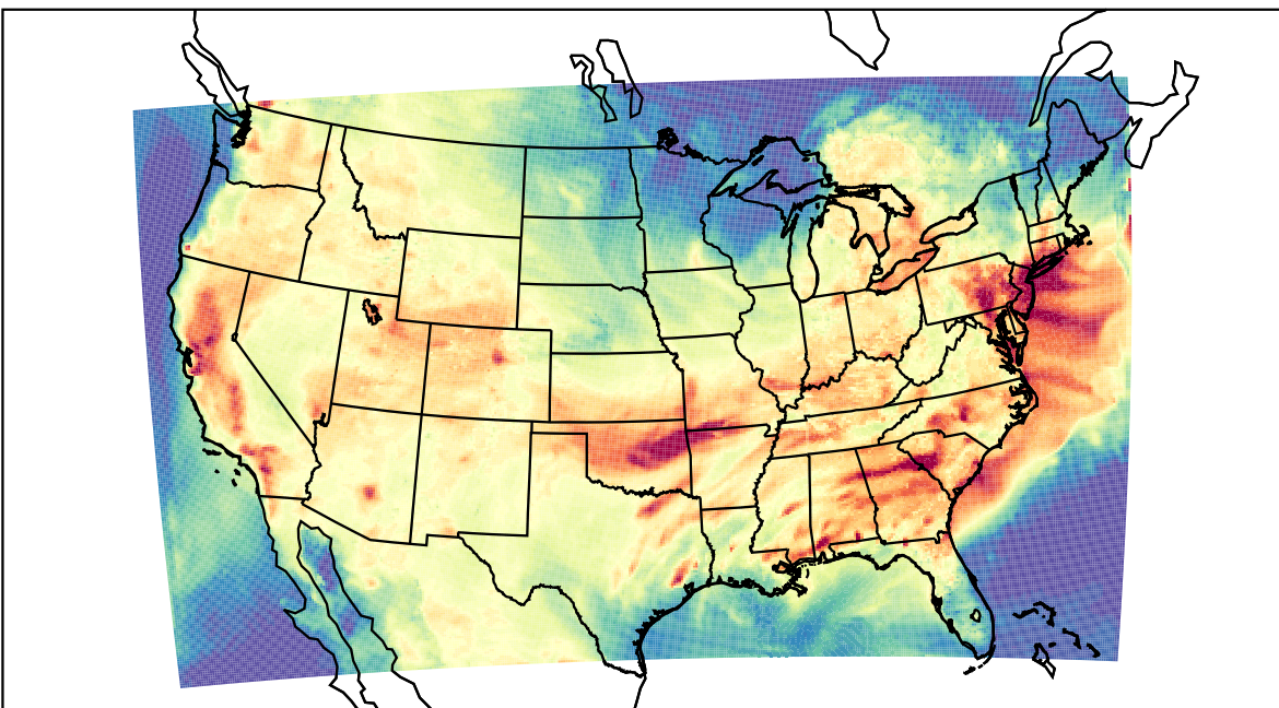
WRF (2023-07-20_22:00:00)
