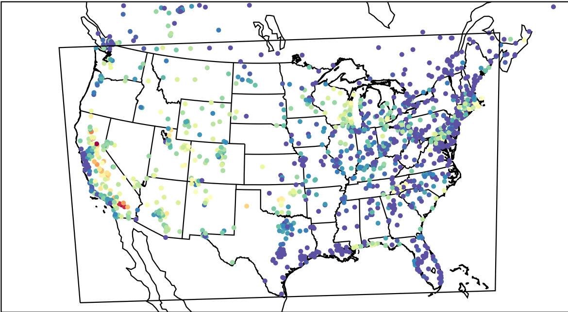
AirNOW (2023-07-20_04:00:00)
