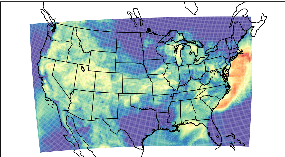
WRF (2023-07-20_10:00:00)
