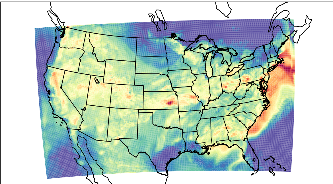
WRF (2023-07-20_03:00:00)
