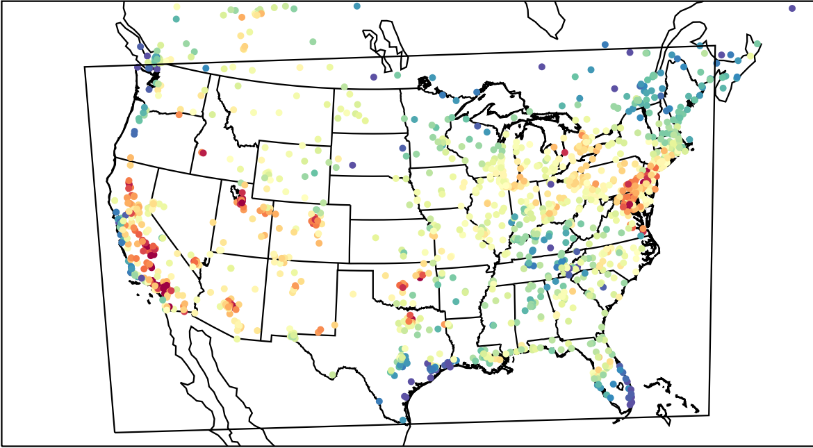
AirNOW (2023-07-20_20:00:00)
