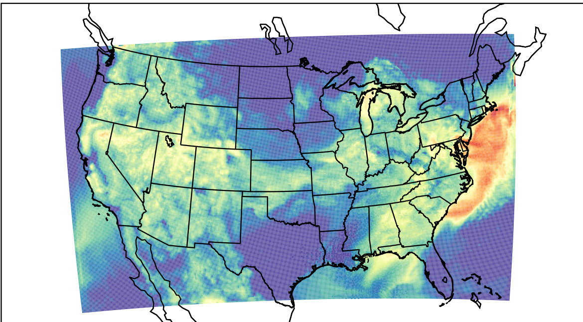
WRF (2023-07-20_13:00:00)
