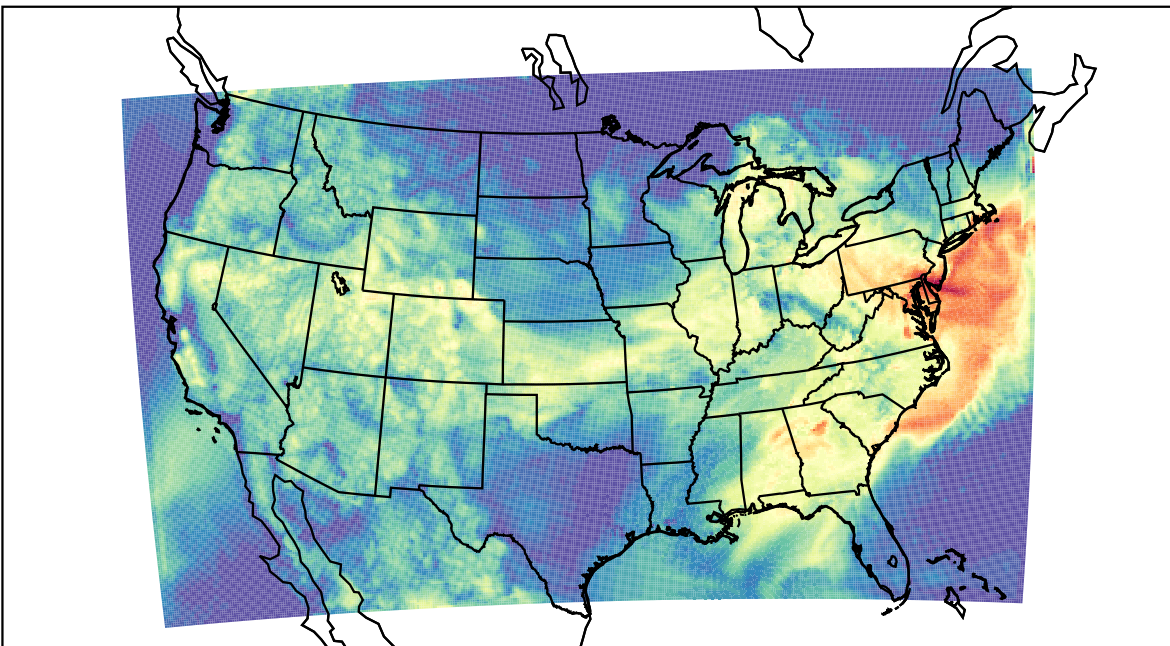
WRF (2023-07-20_14:00:00)
