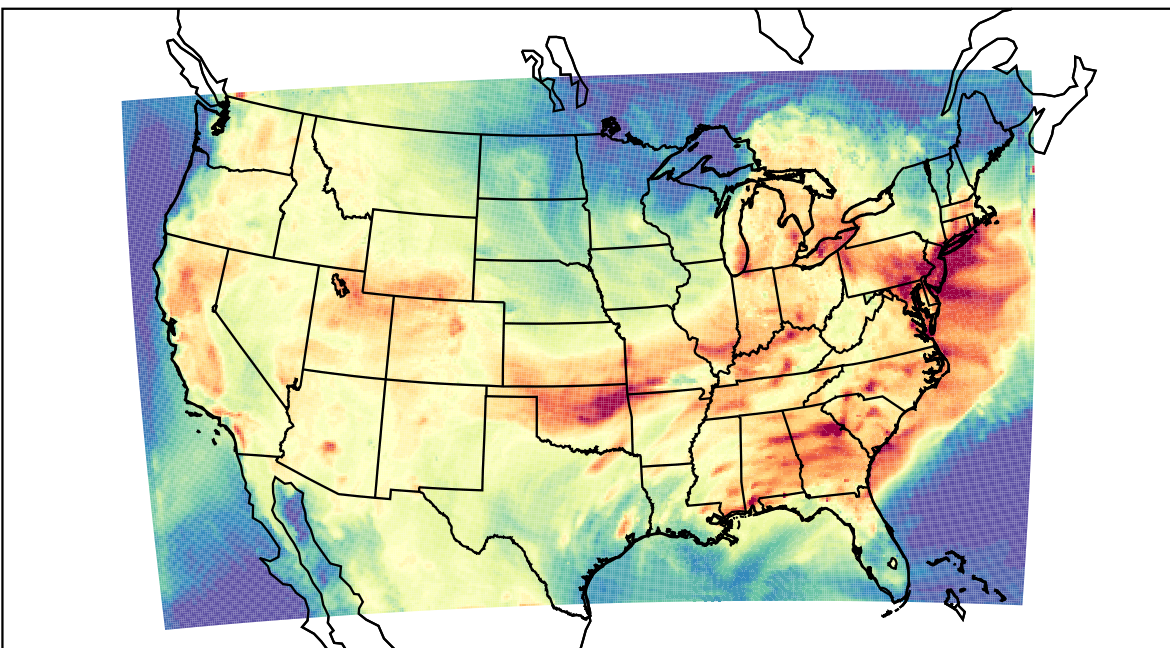
WRF (2023-07-20_19:00:00)
