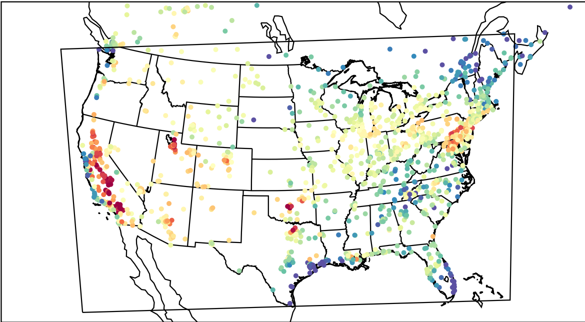
AirNOW (2023-07-20_23:00:00)
