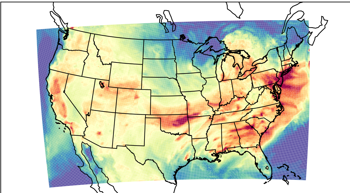
WRF (2023-07-20_20:00:00)
