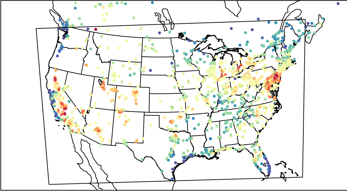
AirNOW (2023-07-20_18:00:00)
