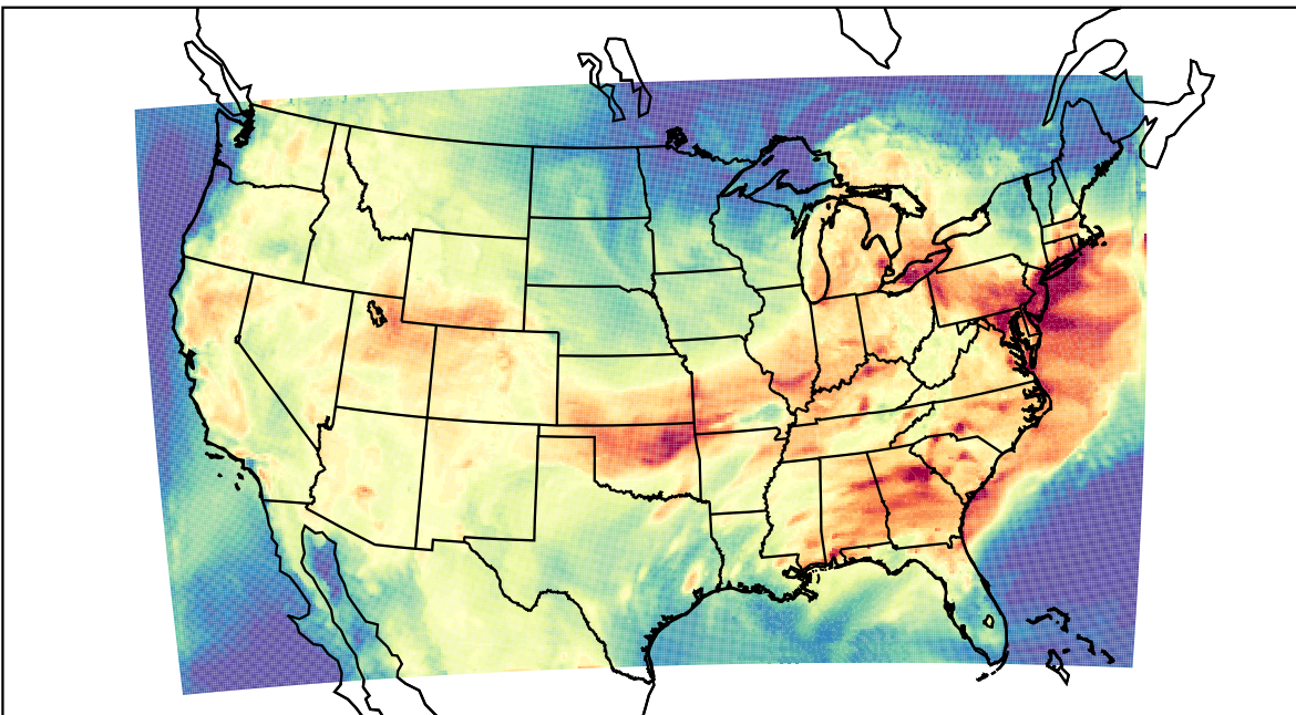
WRF (2023-07-20_18:00:00)
